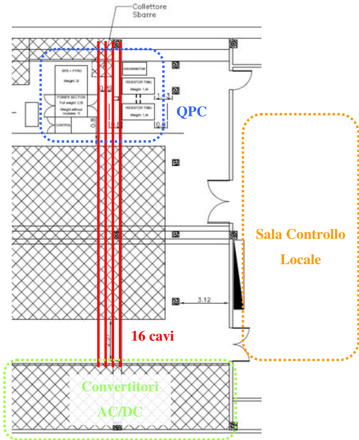
Figura 3 – Pianta luogo installazione
