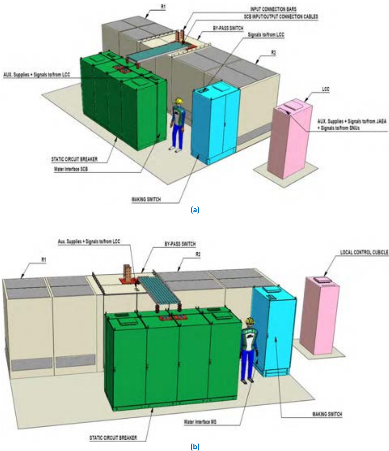
Figura 6. Due diverse angolazioni 3D in scala del prototipo di SNU nella sua configurazione definitiva.
