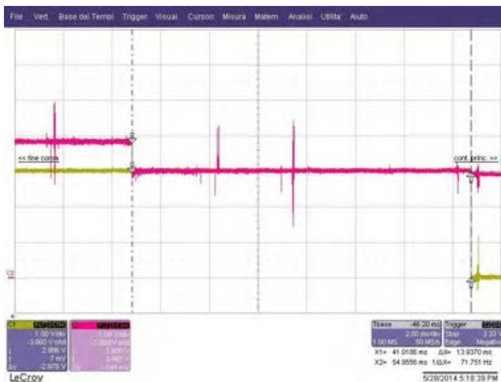
Figura 16. Schermata dell'oscilloscopio per la misura del tempo di apertura meccanica del BPS. In questo caso, il tempo di apertura stimato è intorno al valore medio tra le ripetizioni (circa 14 ms).
