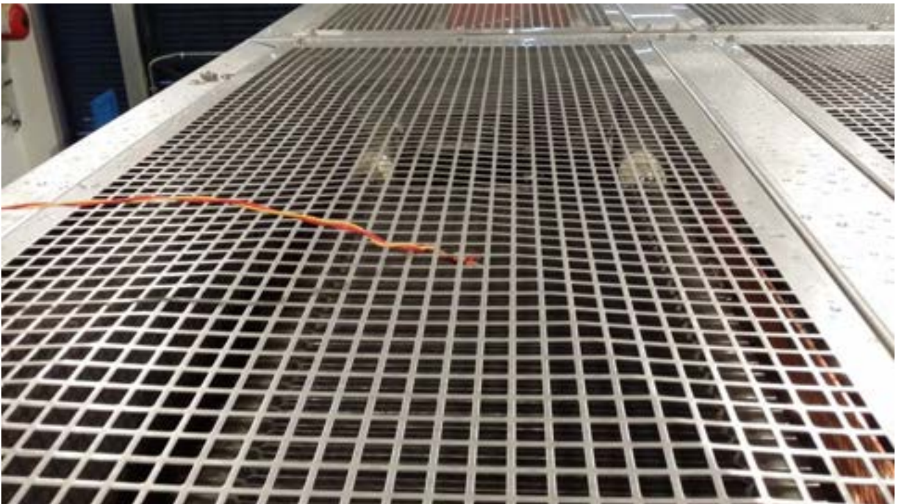
Figura 27. Termocoppia per la misura di temperatura dell'aria in uscita dai resistori durante i temperature rise test.
