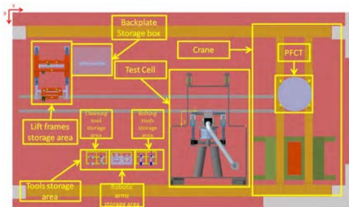
Figura 18. Layout DRP
