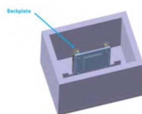
Figura 13. Modello 3d Cassa di Stoccaggio con Backplate
