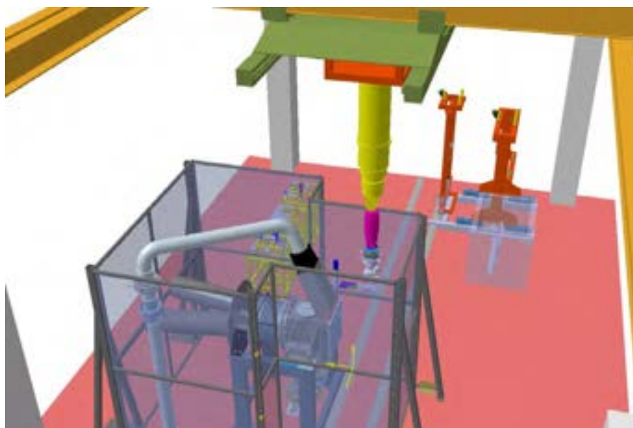
Figura 22. Fissaggio Backplate.
