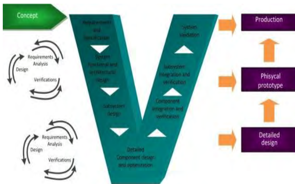
Fig. 1 – V model.
