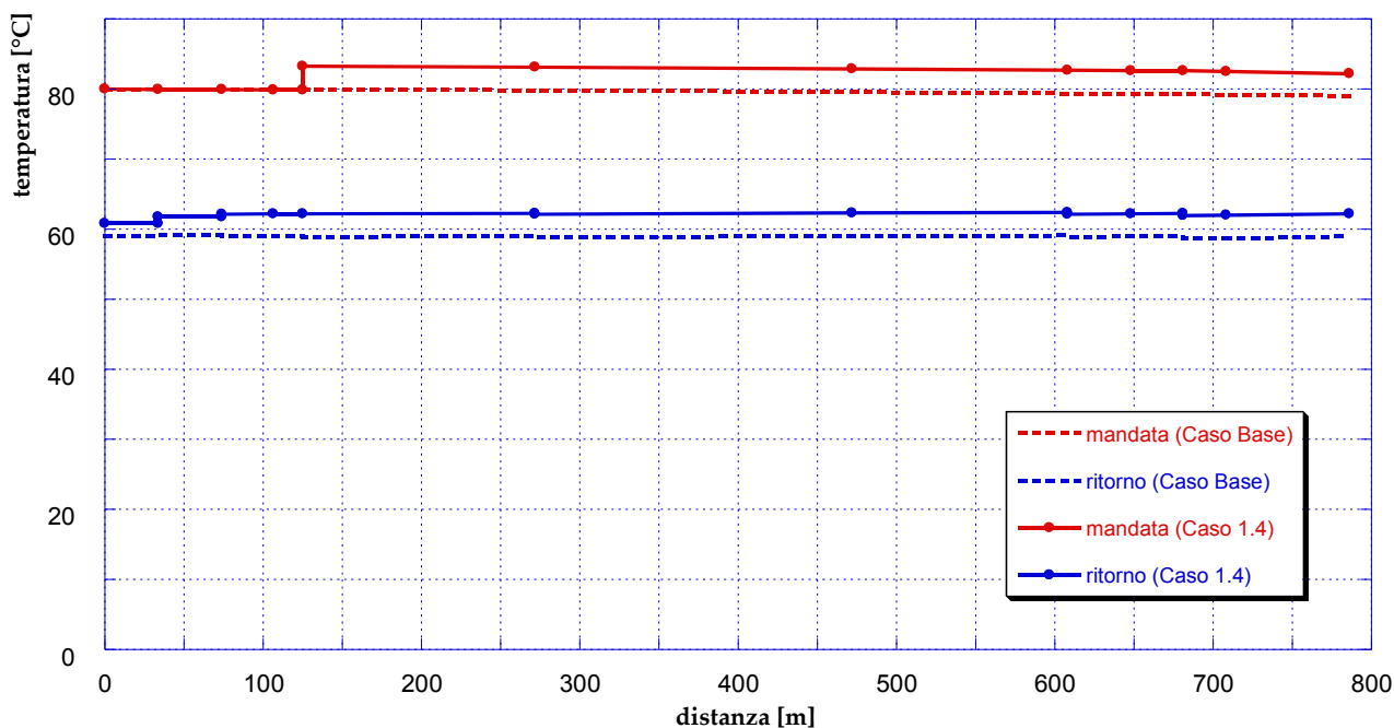
Figura 68 - Temperature lungo il percorso critico (caso 1.4 – Q_{TH,U}/Q_{TH,SP} = 0.0 )
