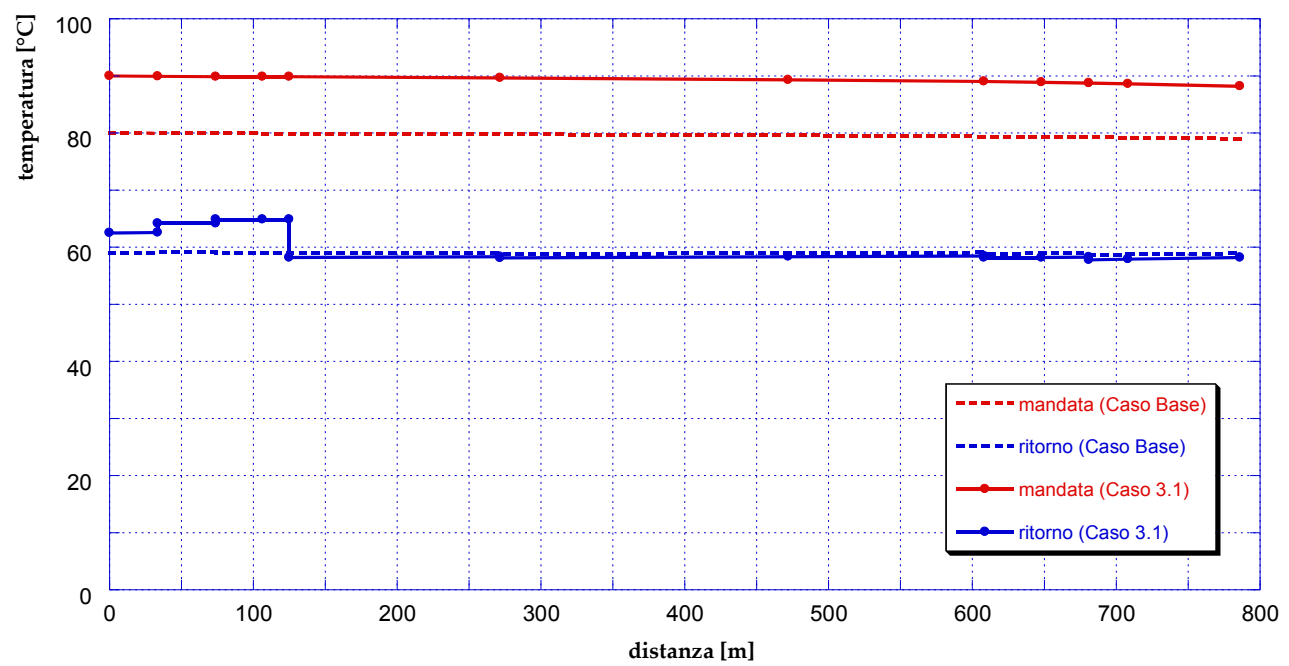
Figura 86 - Temperature lungo il percorso critico (caso 3.1 – Q_{TH,U}/Q_{TH,SP} = 0.0 )
