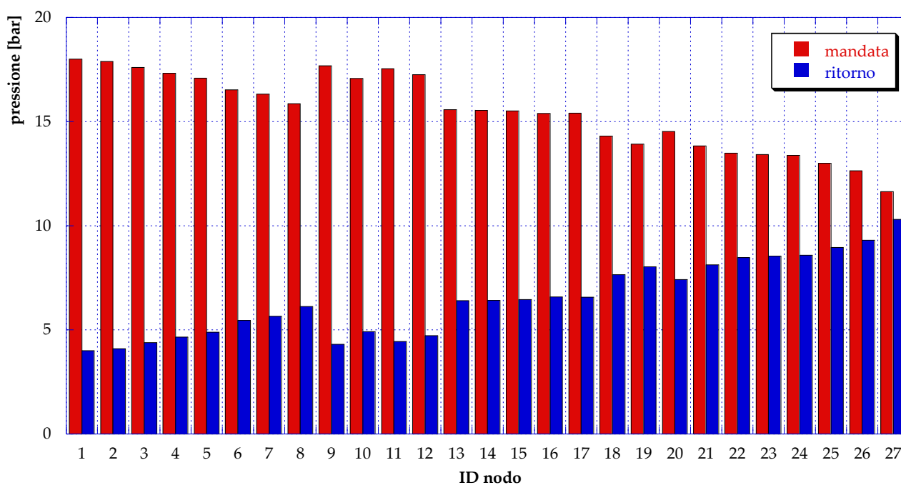
Figura 50 – pressioni sui nodi della rete (caso base)
