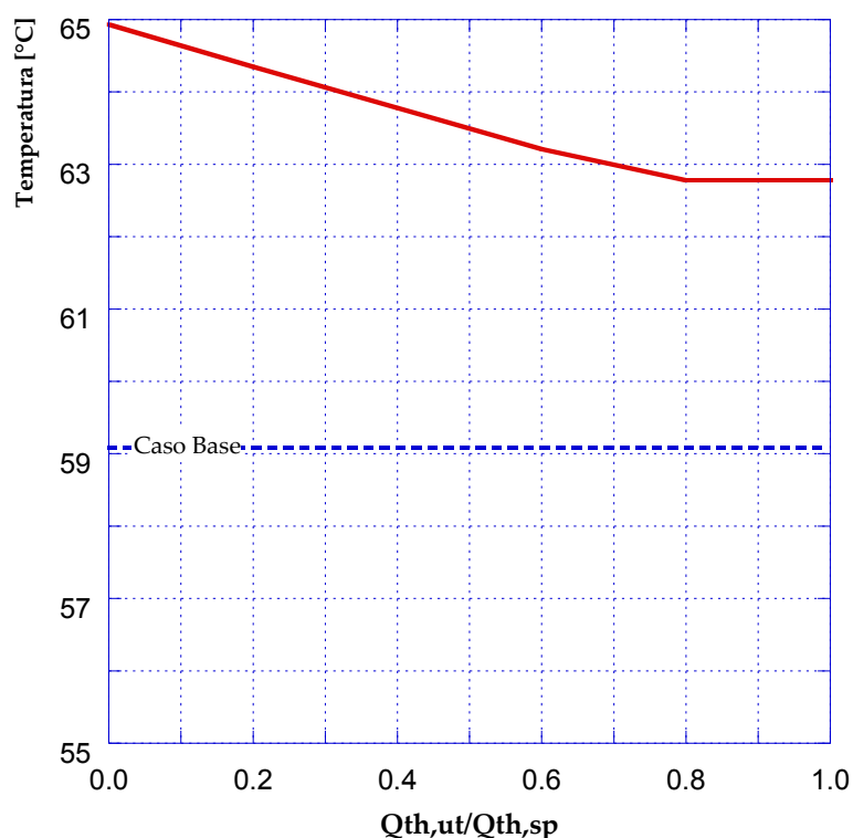
Figura 88 - Temperatura nodo (ritorno) utenza attiva (caso 3.1)
