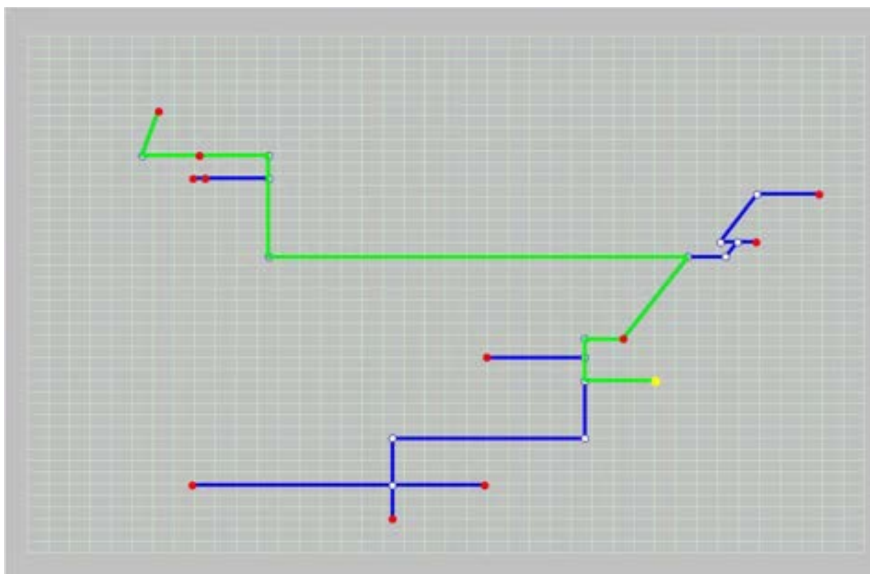
Figura 53 – Percorso critico (dalla centrale all'utenza 27)
