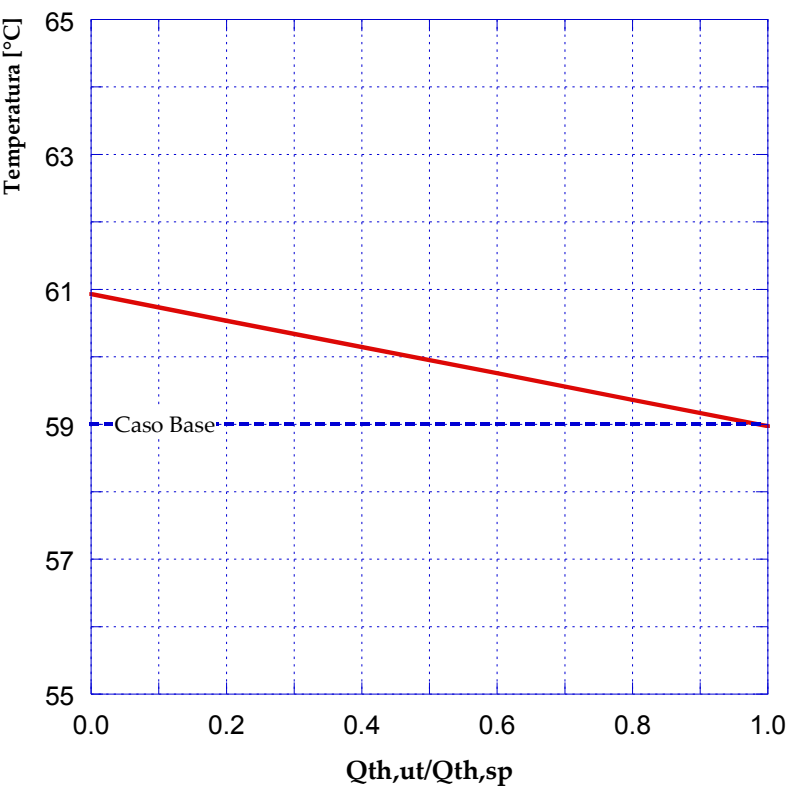
Figura 61 - Temperatura ritorno in centrale (caso 1.2)
