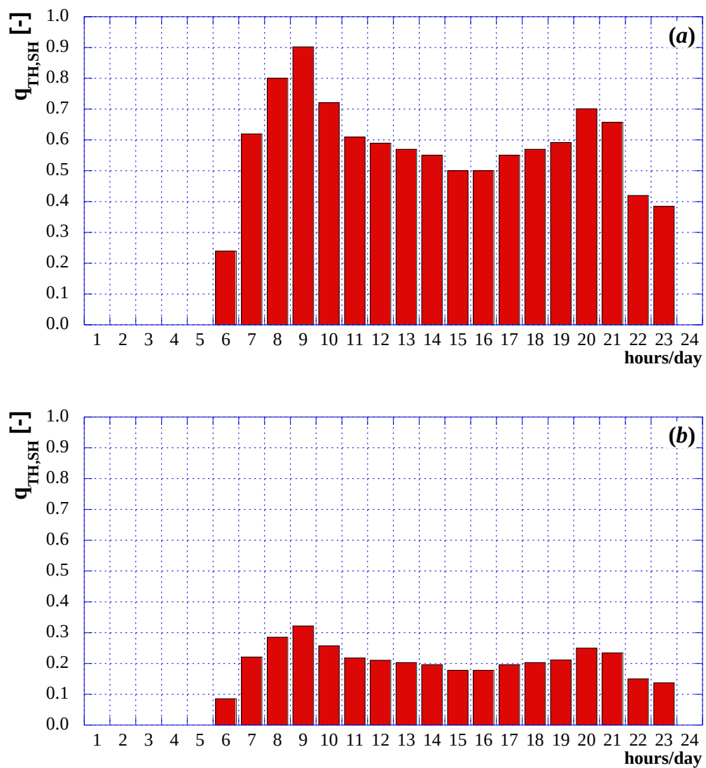
Figura 103 – Curva di carico giornaliera, adimensionalizzata rispetto al carico massimo, per il riscaldamento invernale in un giorno di dicembre (a) e ottobre (b)
