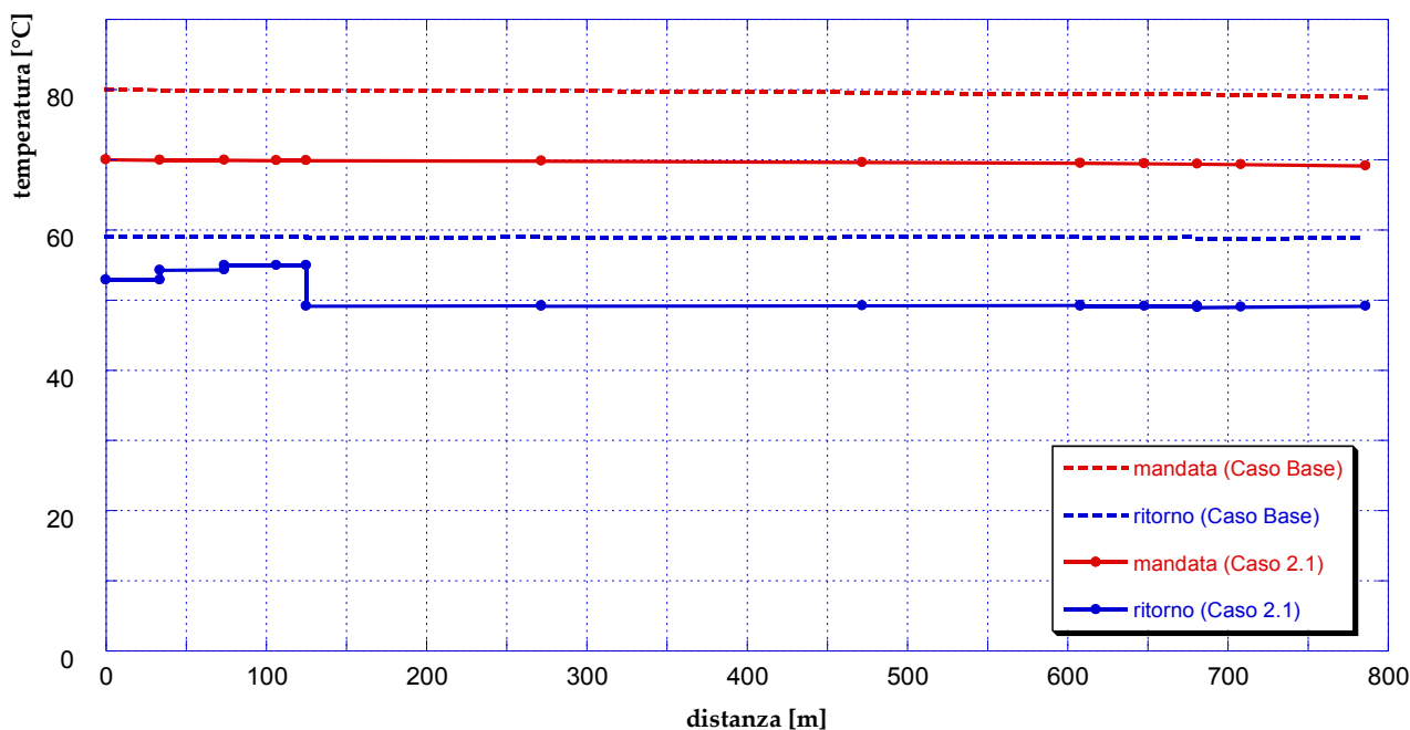
Figura 71 - Temperature lungo il percorso critico (caso 2.1 – Q_{TH,U}/Q_{TH,SP} = 0.0 )
