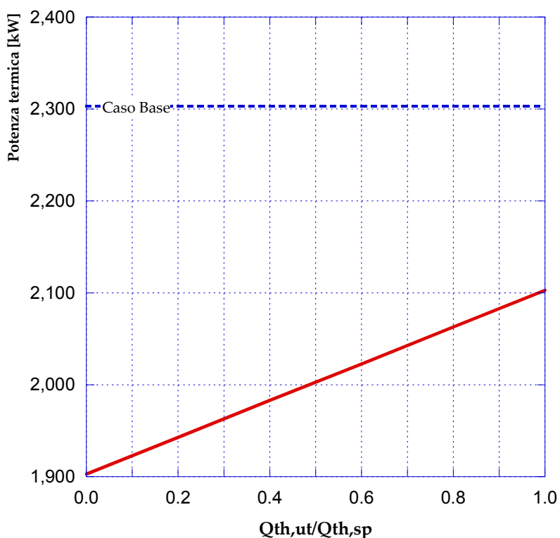
Figura 67 - Potenza termica fornita dalla sorgente (caso 1.3)
