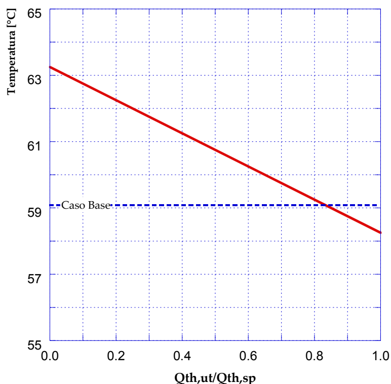
Figura 96 - Temperatura nodo (ritorno) utenza attiva (caso 3.3)
