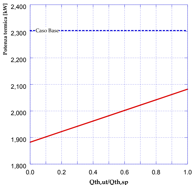
Figura 74 - Potenza termica fornita dalla sorgente (caso 2.1)
