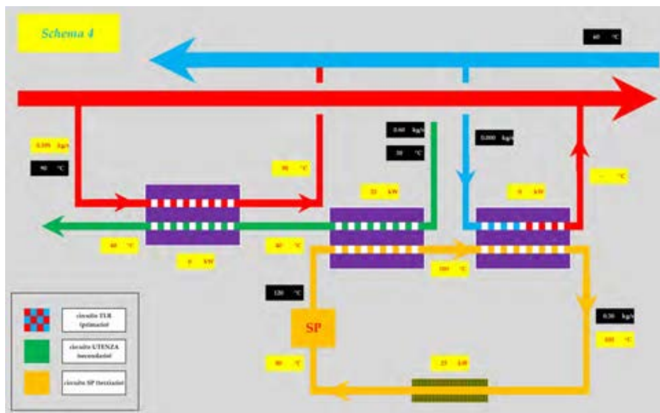
Figura 35 – Interfaccia utente del software IHENA per il fitting dell'utenza nel caso di utenza attiva (schema4)
