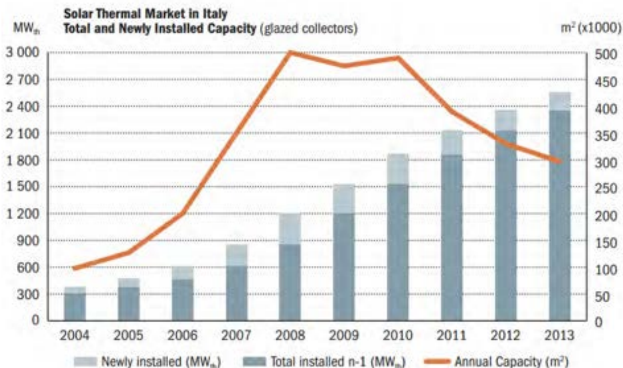
Figura 23 – Potenza totale e nuova installata in collettori solari in Italia
