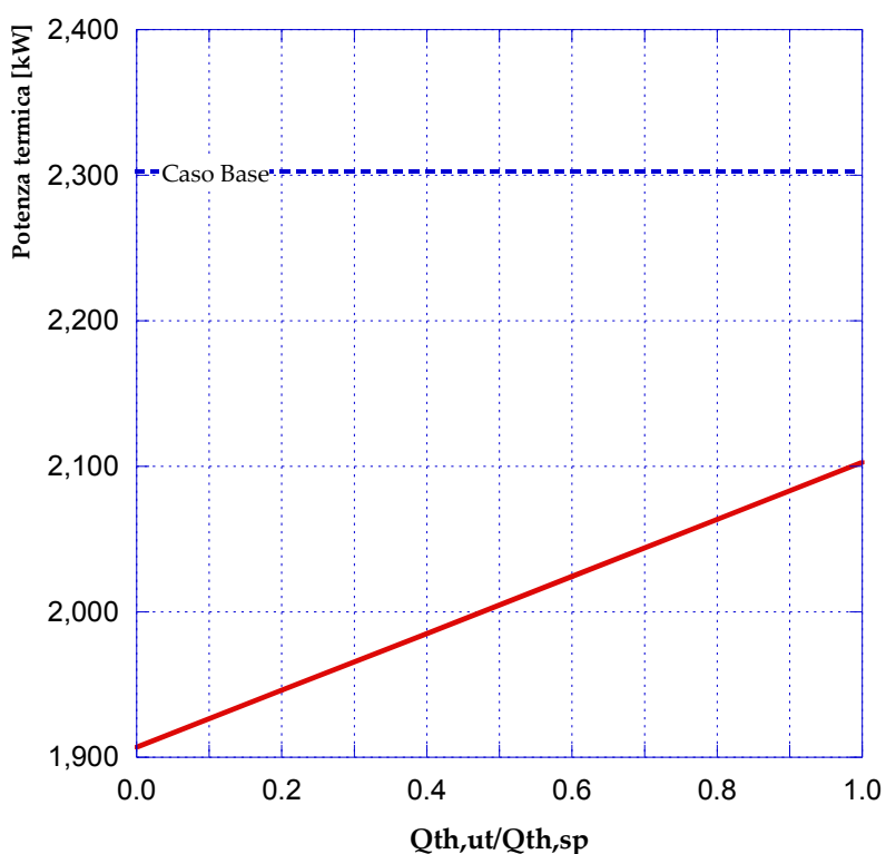
Figura 63 - Potenza termica fornita dalla sorgente (caso 1.2)
