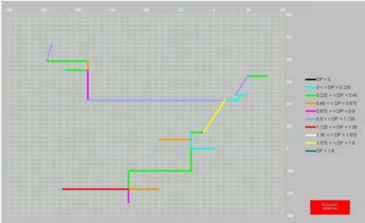
Figura 48 – Distribuzione perdite di carico [bar] (caso base)
