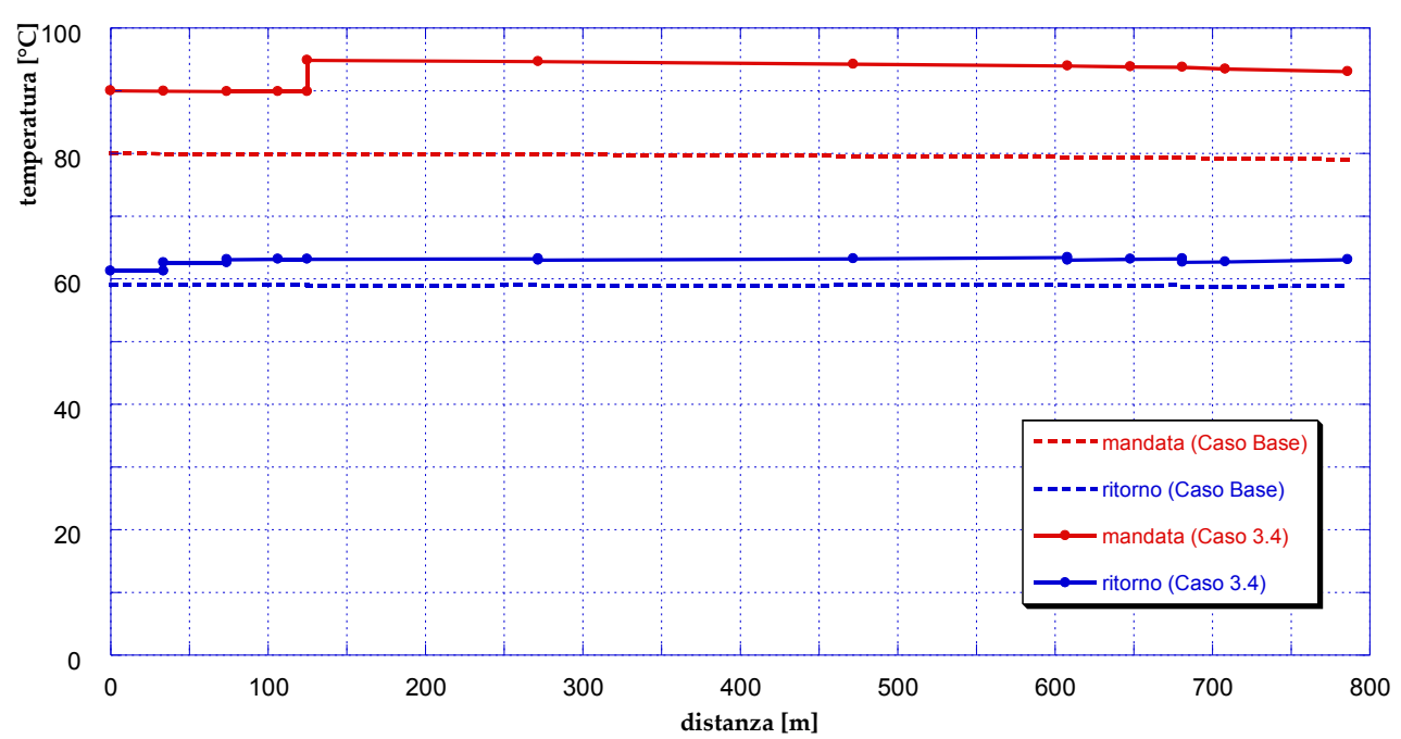
Figura 98 - Temperature lungo il percorso critico (caso 3.4 – Q_{TH,U}/Q_{TH,SP} = 0.0 )
