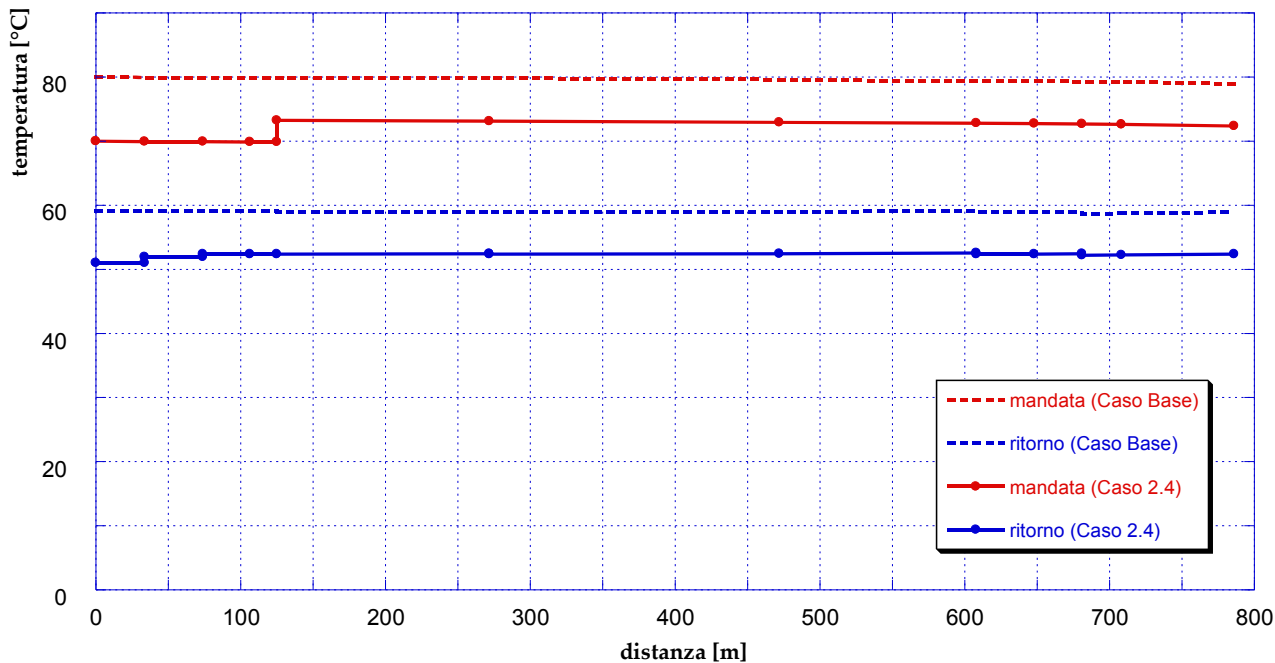
Figura 83 - Temperature lungo il percorso critico (caso 2.4 - Q_{TH,U}/Q_{TH,SP} = 0.0 )
