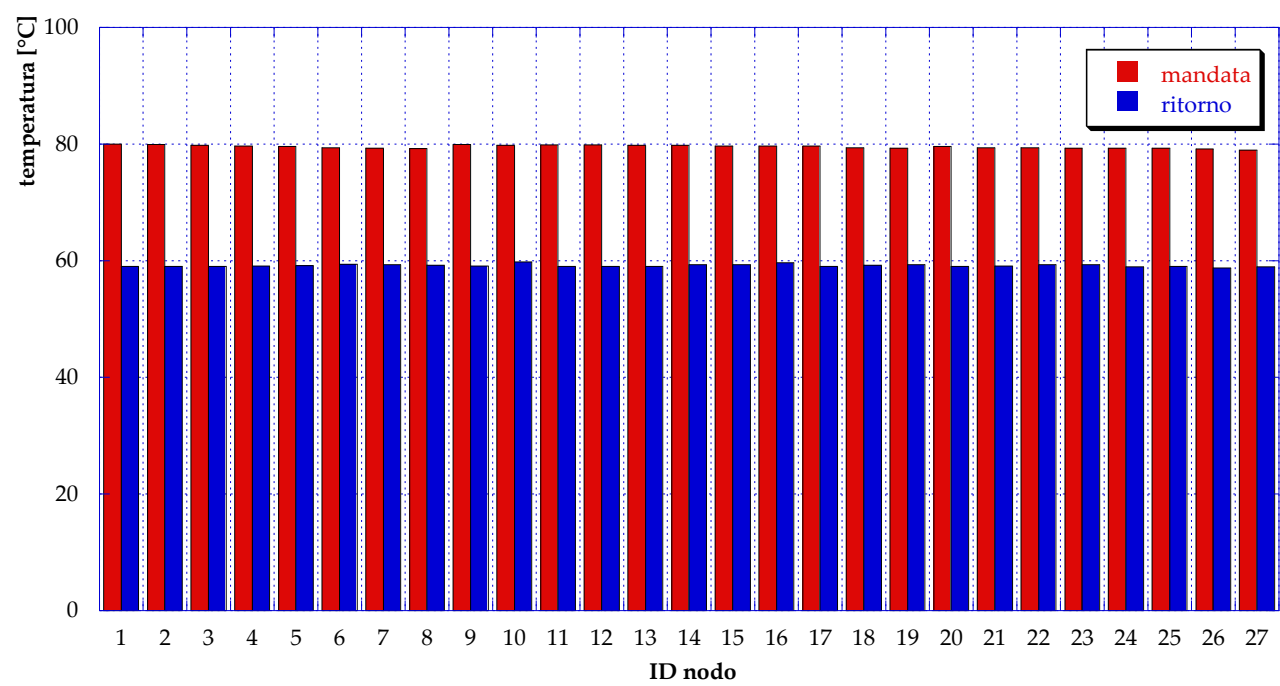
Figura 51 – Temperature sui nodi della rete (caso base)
