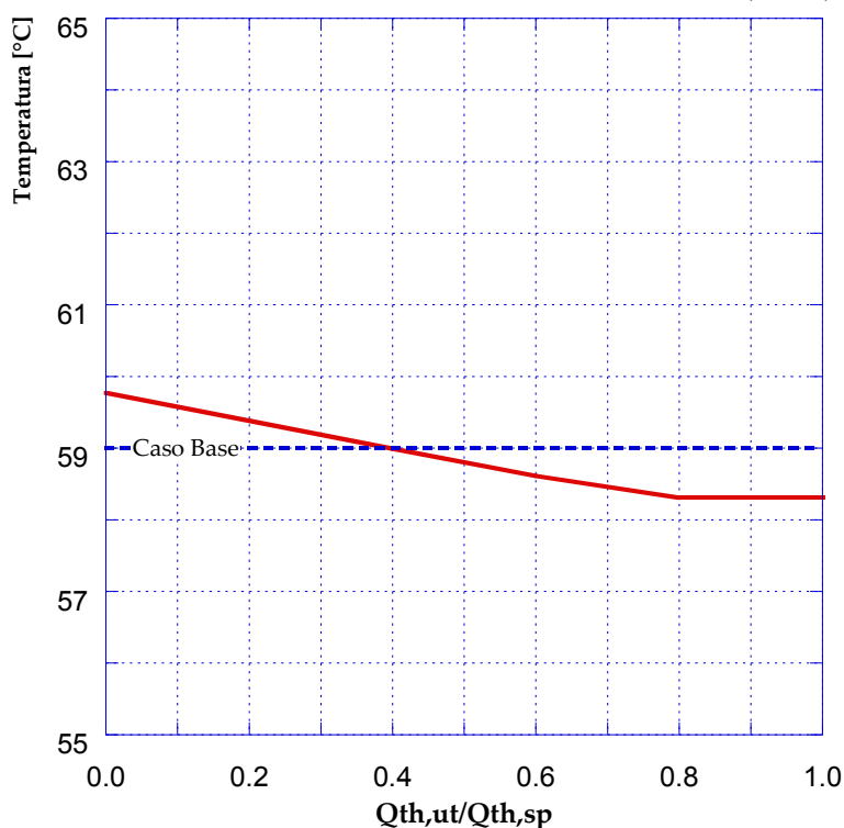
Figura 91 - Temperatura ritorno in centrale (caso 3.2)
