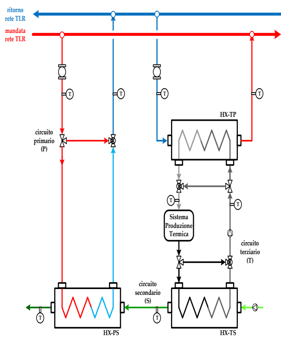
Schema 2
