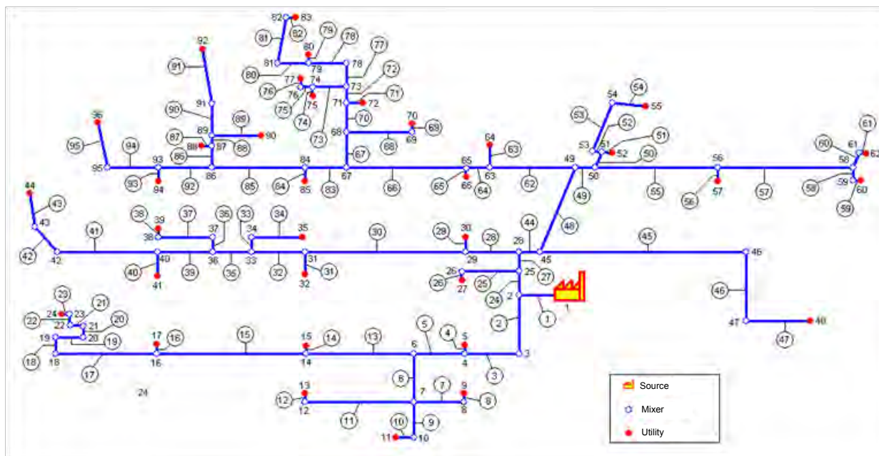
Figura 27 – Rete di teleriscaldamento impiegata per la validazione del Ca.R.Di.F.
