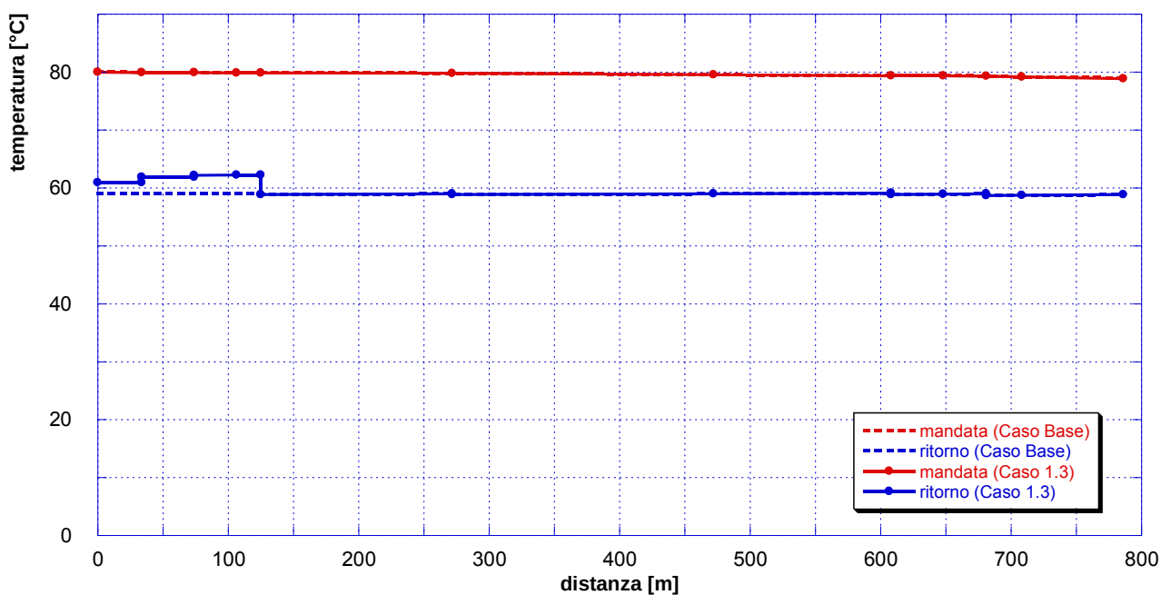
Figura 64 - Temperature lungo il percorso critico (caso 1.3 – Q_{TH,U}/Q_{TH,SP} = 0.0 )
