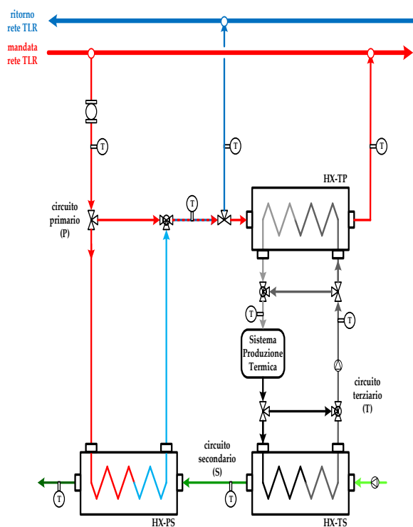
Schema 2
