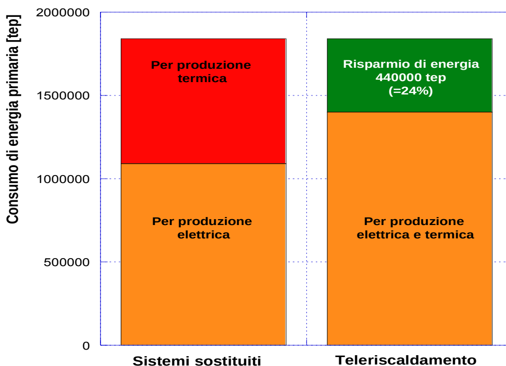
Figura 10 – Risparmio di energia primaria fossile conseguita dalle reti di Teleriscaldamento (anno 2012) [4]
