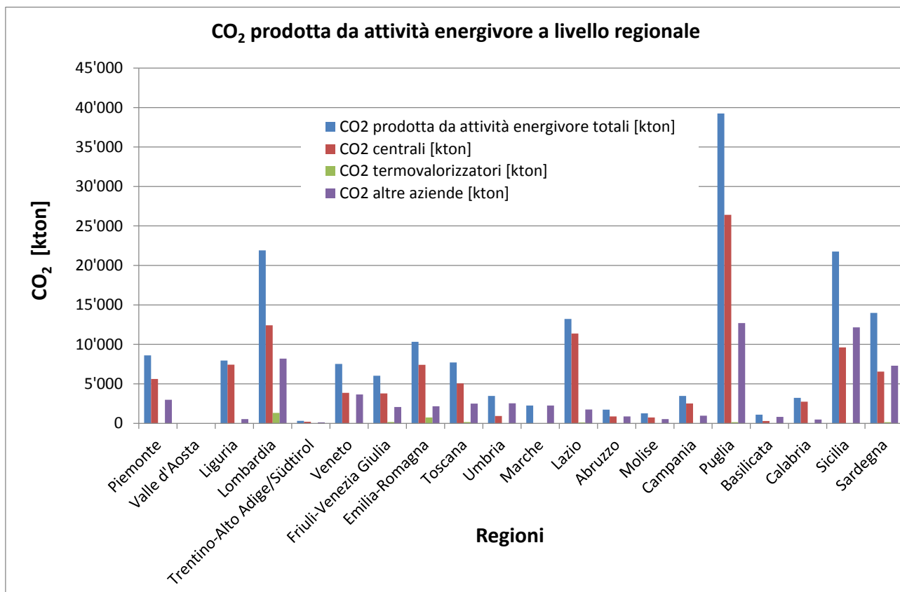
Figura 47 - CO 2 emessa da aziende energivore, elaborazione dati E-PRTR
