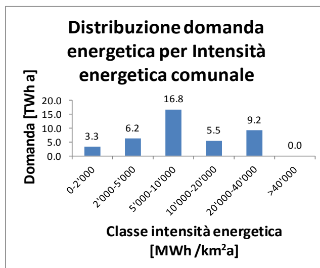
Figura 62 - Distribuzione della domanda di energia per il settore residenziale, per i comuni con reti TLR, in funzione della classe di intensità energetica
