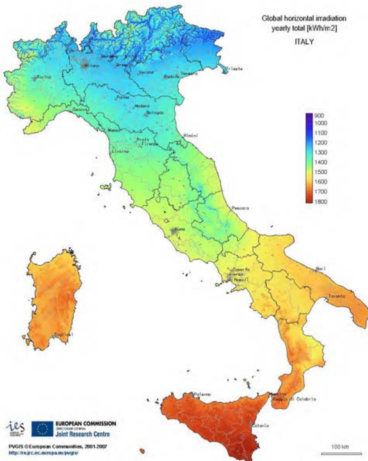
Figura 53 - Mappa della radiazione solare in Italia, dati JRC
