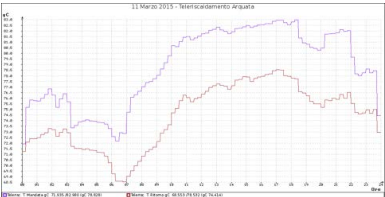
Figura 35 - Temperatura di mandata e di ritorno
