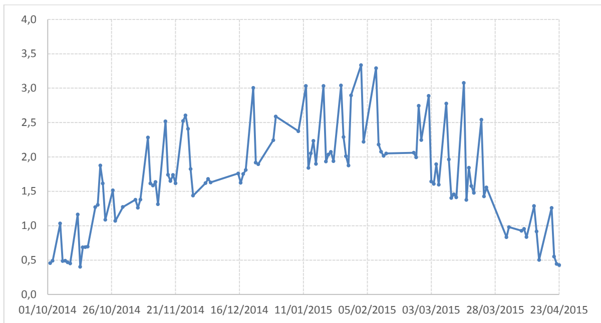
Figura 44 - Rapporto energia termica caldaie/cogeneratore
