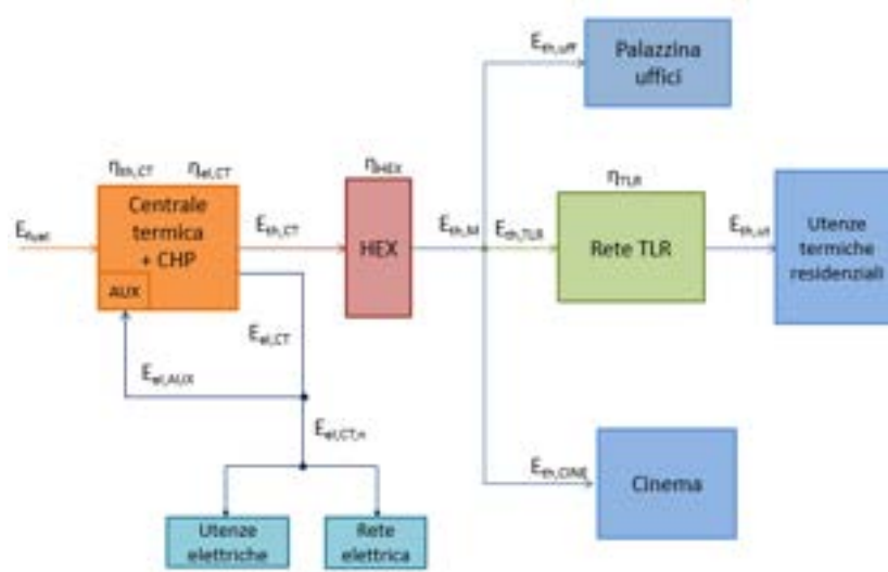
Figura 45 – Schema funzionale dell'impianto
