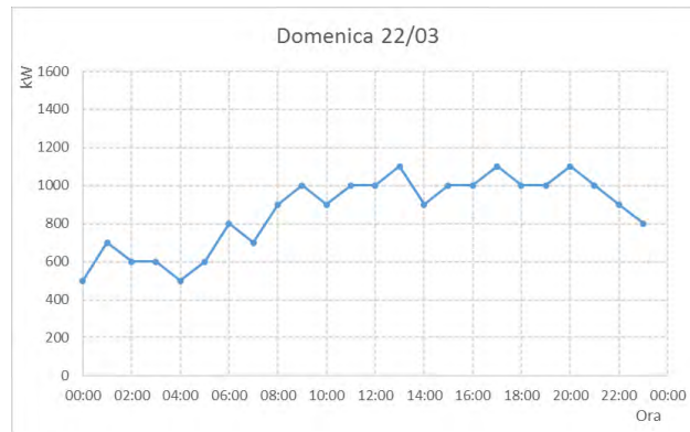
Figura 46 – Andamento giornaliero potenza termica
