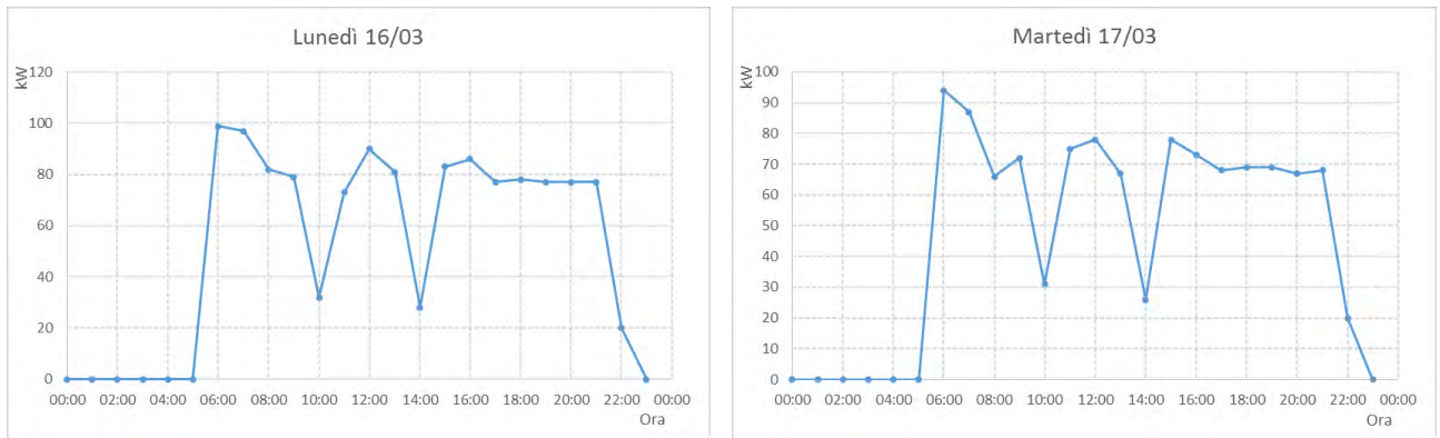
Figura 51 - Andamento potenza termica piè di stabile con allacciamento indiretto
