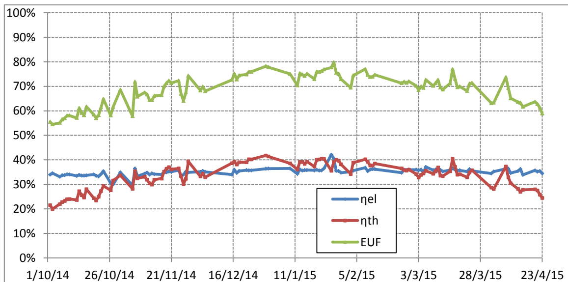
Figura 39 - Indici di performance energetica del cogeneratore sull'anno termico 2014-2015
