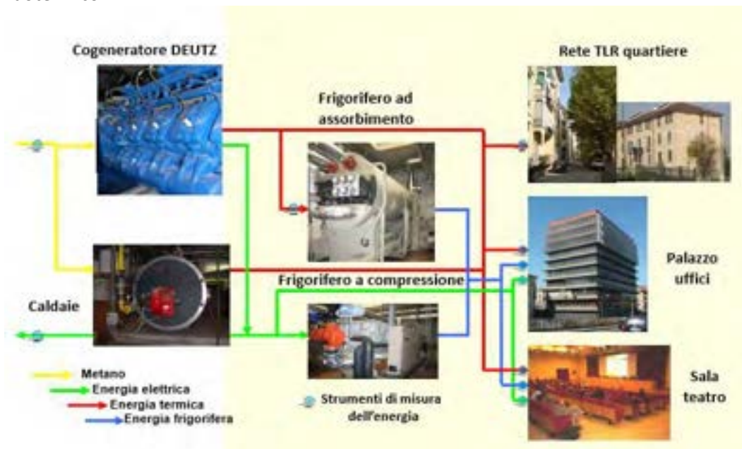
Figura 4 - Schema della Centrale Termica
