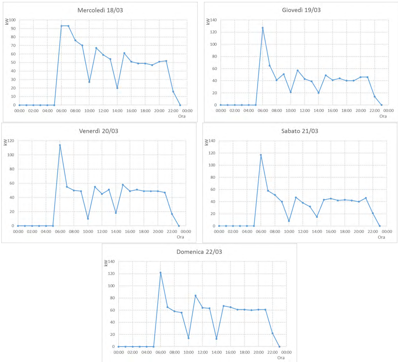
Figura 52 - Andamento potenza termica piè di stabile con allacciamento diretto
