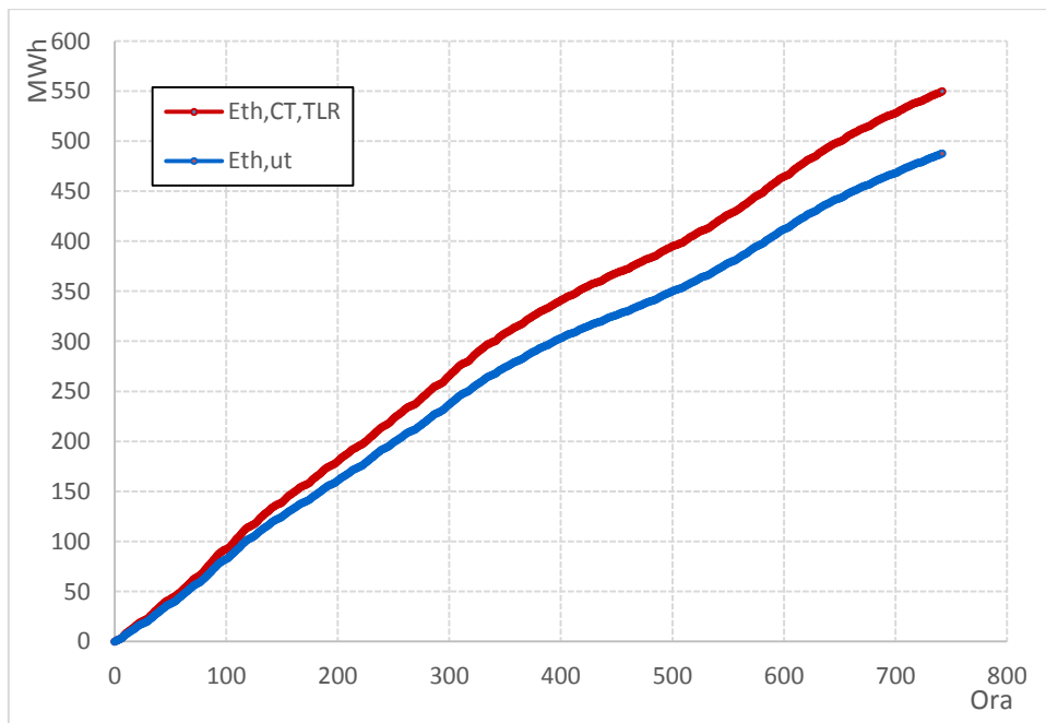
Figura 49 - Confronto progressivi energia termica
