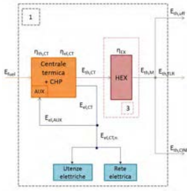
Figura 21 - Volume di controllo 1
