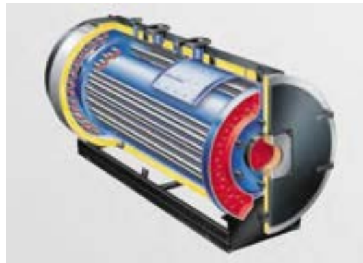
Figura 8 - Sezione di caldaia Vitomax 200
