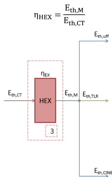
Figura 22 - Volume di controllo 3
