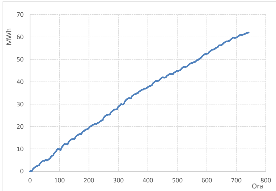
Figura 50 - Perdite sulla rete e nello scambiatore di calore
