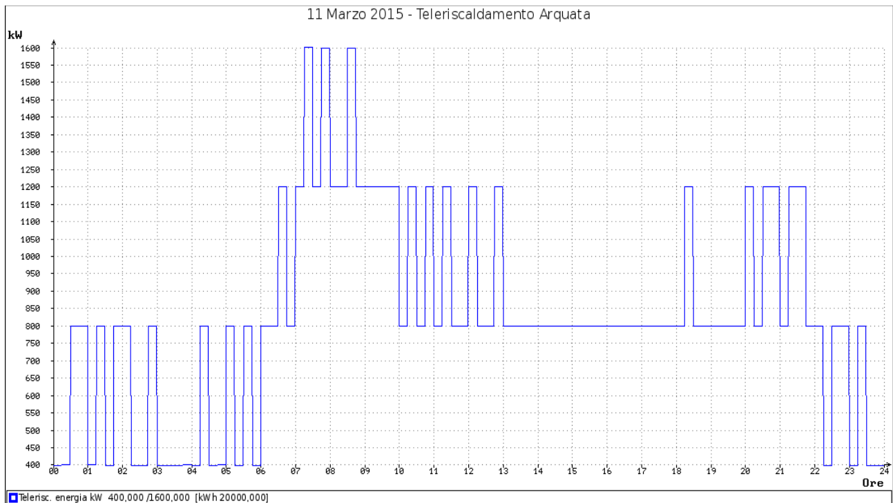
Figura 33 - Potenza TLR
