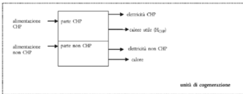
Figura 42 - Macchina virtuale unità cogenerativa
