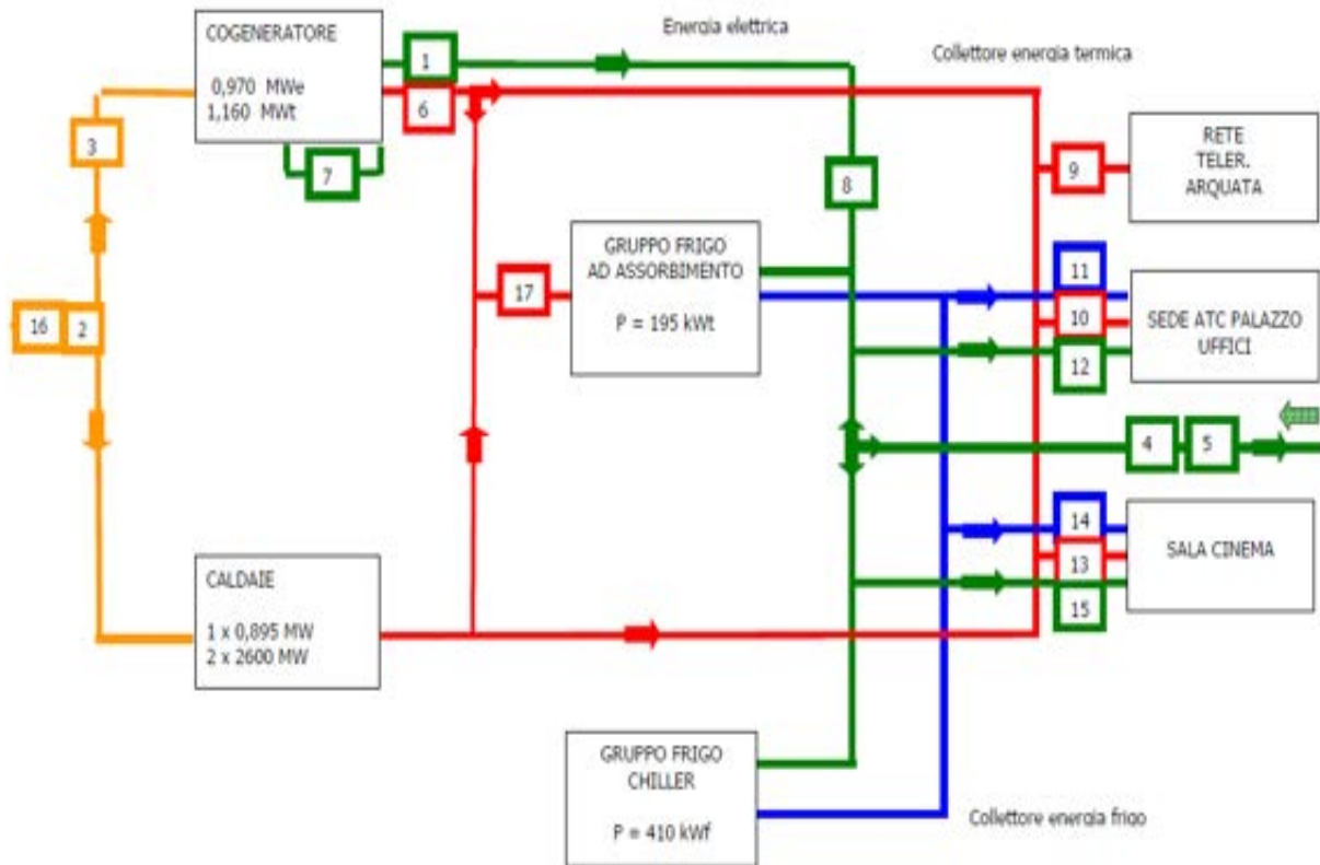
Figura 9 - Schema sensori dell'impianto
