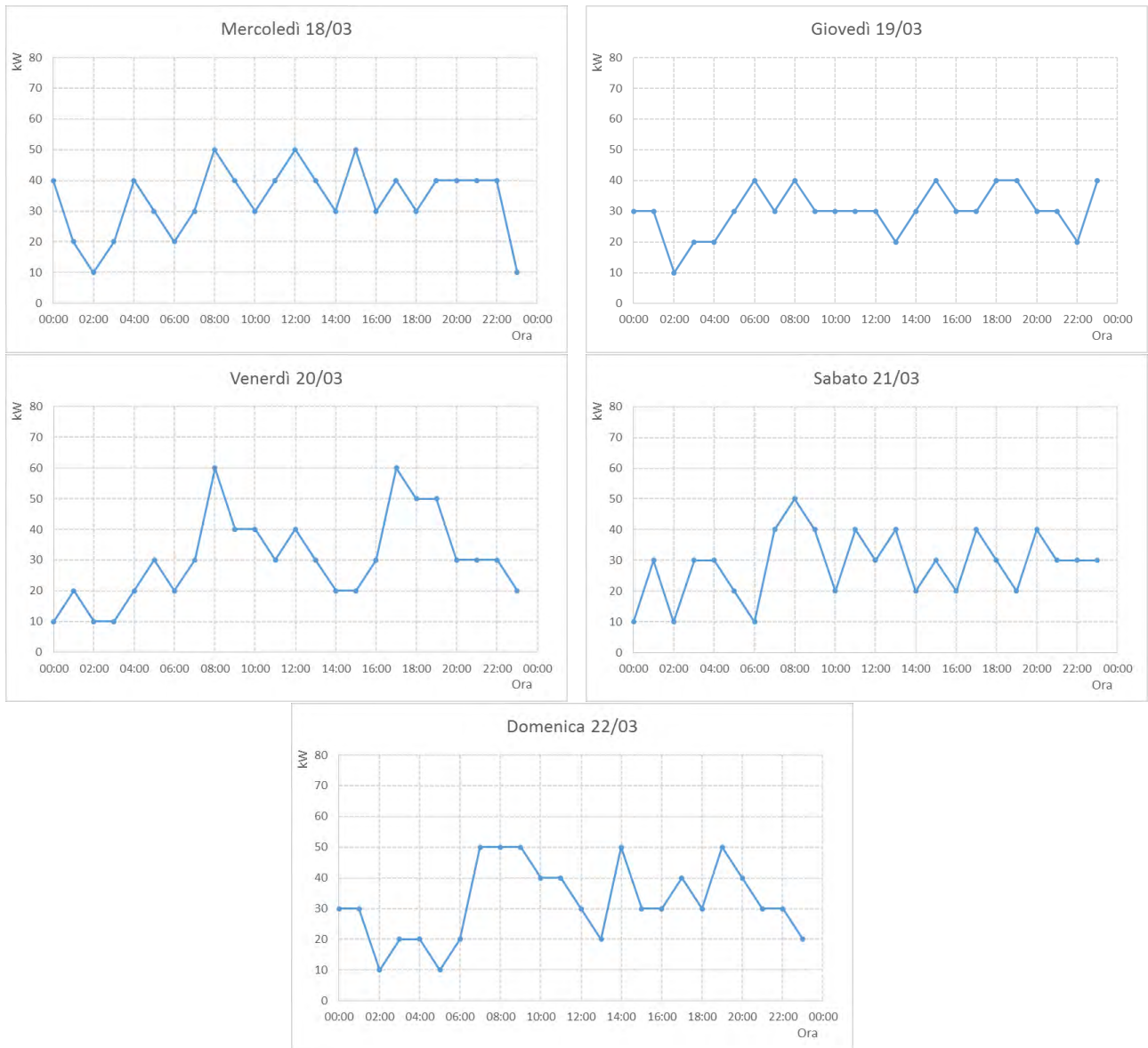
Figura 51 - Andamento potenza termica piè di stabile con allacciamento indiretto
