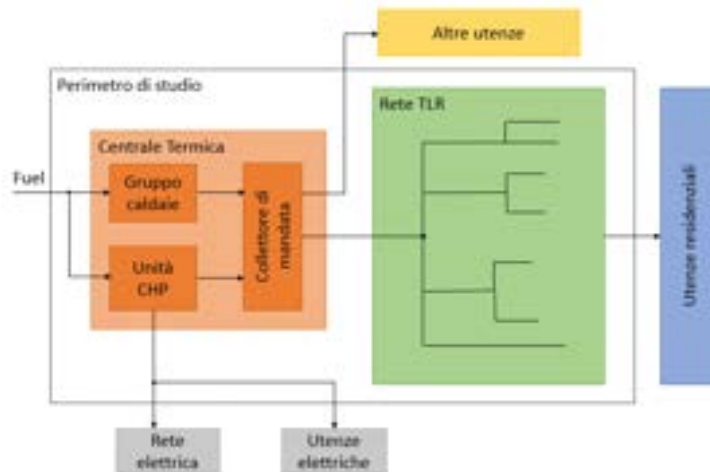
Figura 3 – Schema a blocchi dell’intero impianto con annessa rete di teleriscaldamento
