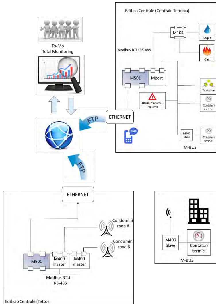
Figura 23 - Architettura sistema di monitoraggio
