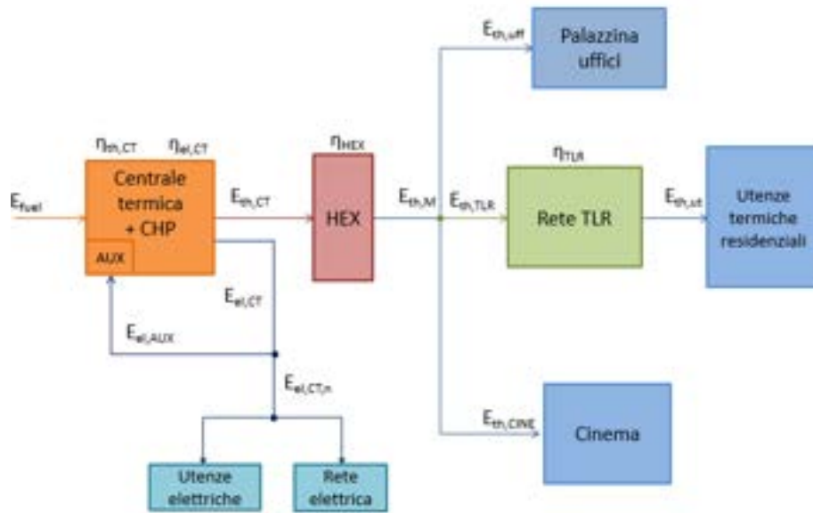
Figura 18 - Schema semplificato di impianto
