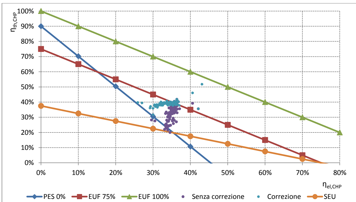
Figura 43 - Punti di funzionamento impianto
