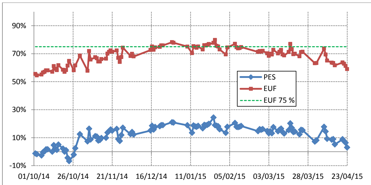
Figura 41 - Andamento PES e EUF
