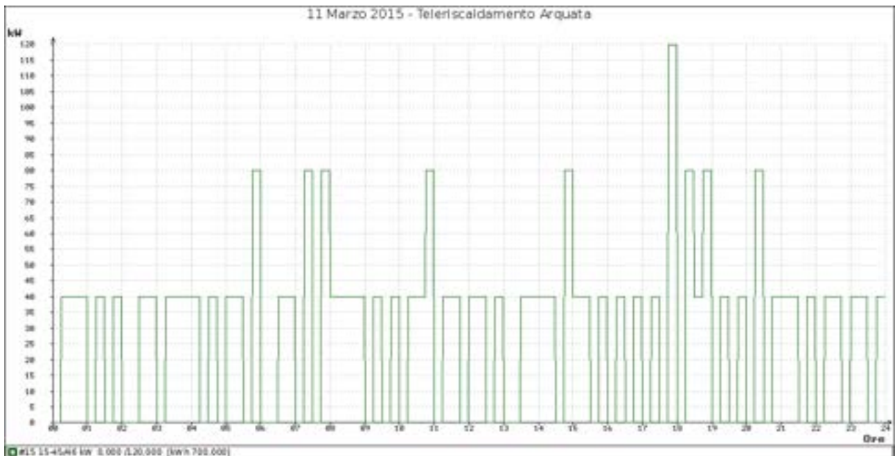
Figura 37 - Potenza termica misurata a un piè di stabile
