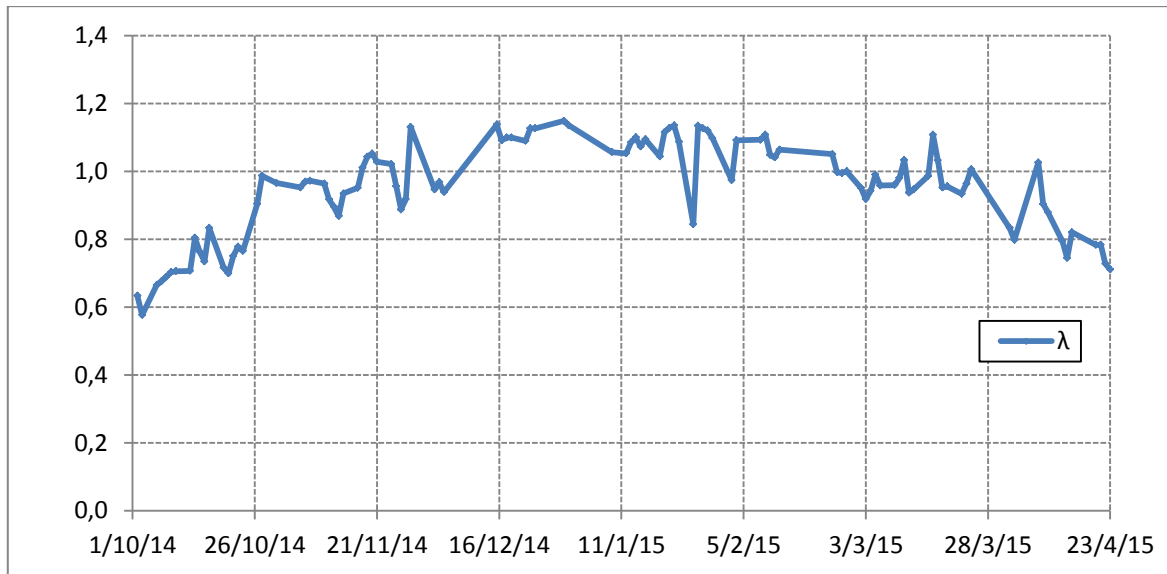
Figura 40 - Rapporto di cogenerazione
