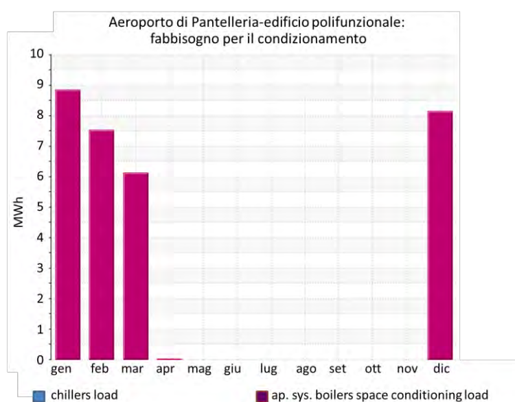
Figura 20 Fabbisogno termico per raffrescamento e riscaldamento dell'aerostazione di Pantelleria. Edificio Polifunzionale. Report Software IES VE
