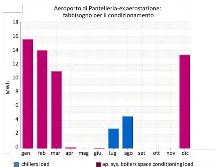
Figura 21 Fabbisogno termico per raffrescamento e riscaldamento dell'aerostazione di Pantelleria. Ex-aerostazione. Report Software IES VE
