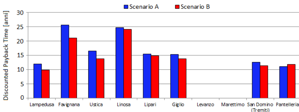
Figura 105 Discounted Payback Time per tutte le isole
