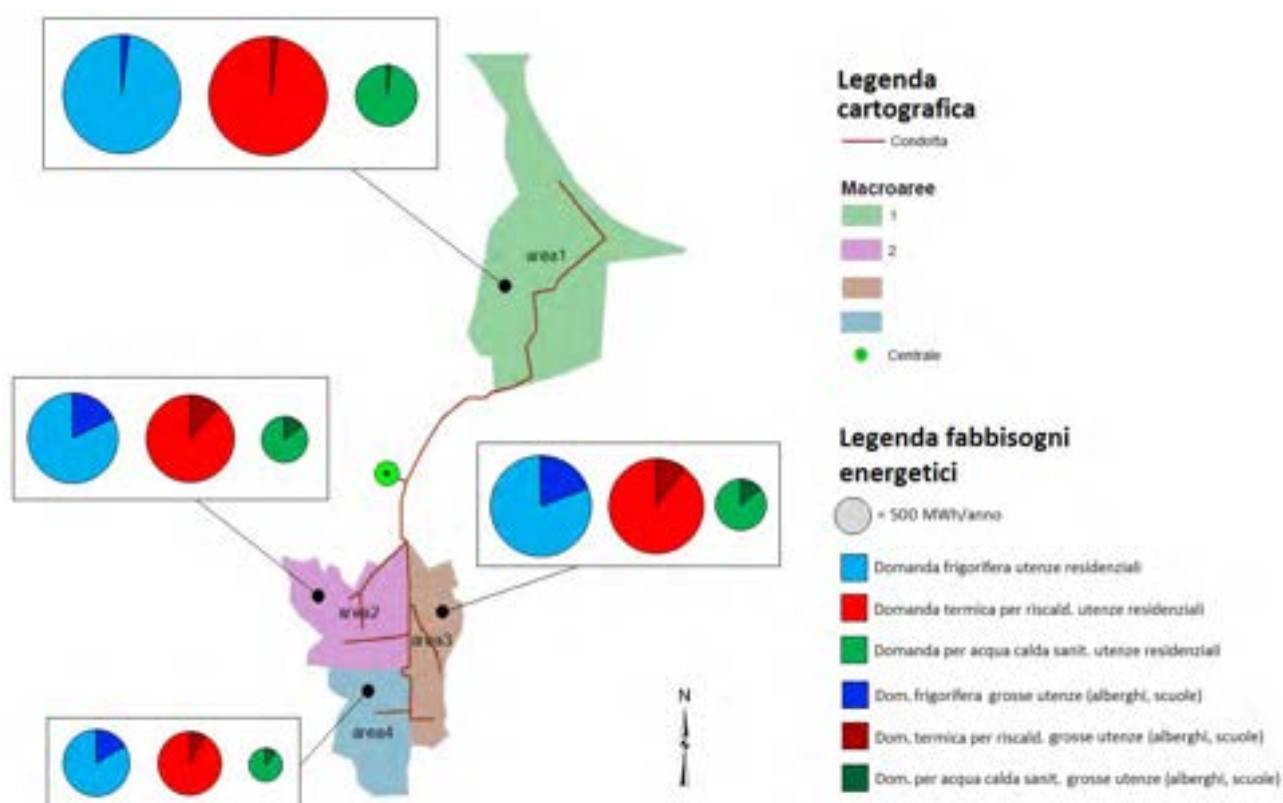
Figura 82 Rappresentazione semplificata delle aree di riferimento e della geometria delle possibili dorsali principali di distribuzione
