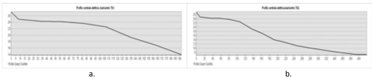
Figura 41 Sviluppo altimetrico delle condotte di trasporto, lungo i rami di dorsale principale, che collegano la centrale elettrica alle diverse aree
