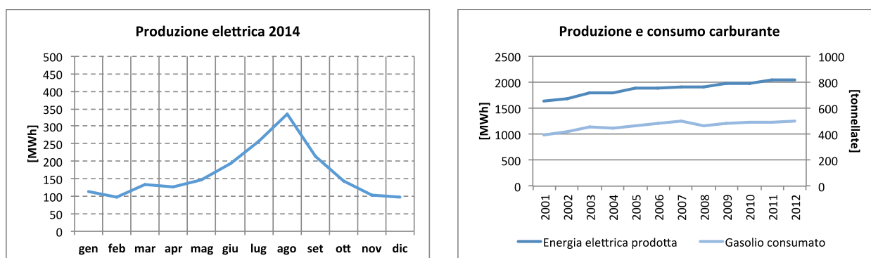
Figura 59 Centrale elettrica. A sinistra, produzione mensile. A destra, serie storica.
