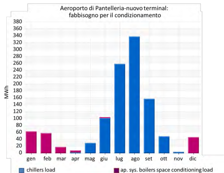
Figura 19 Fabbisogno termico per raffrescamento e riscaldamento dell'aerostazione di Pantelleria Nuovo terminal. Report Software IES VE
