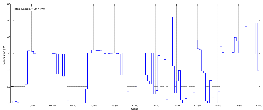
Figura 64: Potenza Attiva misurata il 24/07/2015 dalle ore 10:00
