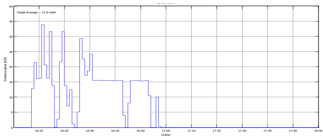
Figura 44: Potenza Attiva misurata il 20/07/2015 dalle ore 16:00
