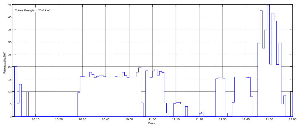
Figura 41: Potenza Attiva misurata il 20/07/2015 dalle ore 10:00
