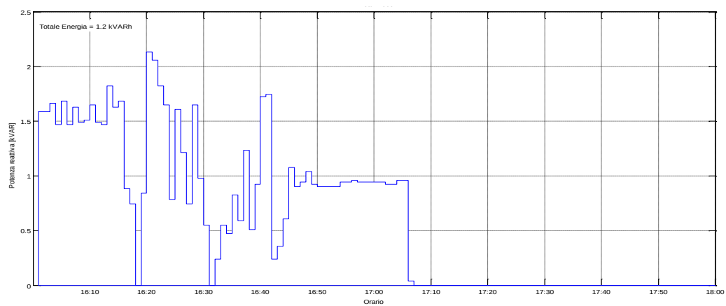
Figura 100: Potenza Reattiva misurata il 22/07/2015 dalle ore 16:00
