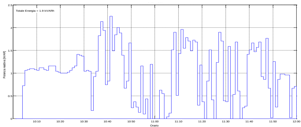
Figura 91: Potenza Reattiva misurata il 21/07/2015 dalle ore 10:00
