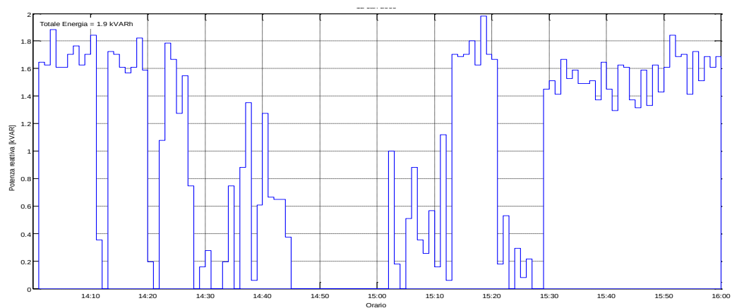
Figura 87: Potenza Reattiva misurata il 20/07/2015 dalle ore 14:00
