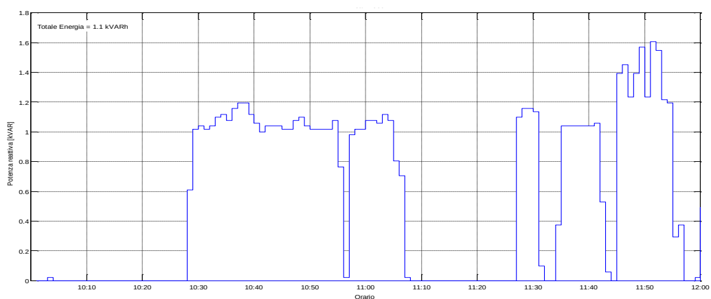
Figura 85: Potenza Reattiva misurata il 20/07/2015 dalle ore 10:00
