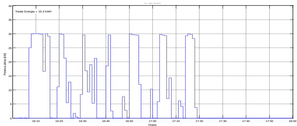
Figura 73: Potenza Attiva misurata il 25/07/2015 dalle ore 16:00
