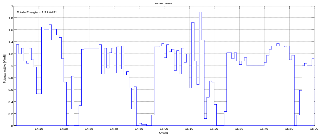
Figura 105: Potenza Reattiva misurata il 23/07/2015 dalle ore 14:00
