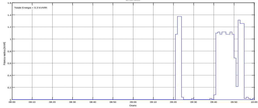
Figura 76: Potenza Reattiva misurata il 18/07/2015 dalle ore 08:00
