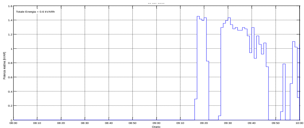
Figura 108: Potenza Reattiva misurata il 24/07/2015 dalle ore 08:00
