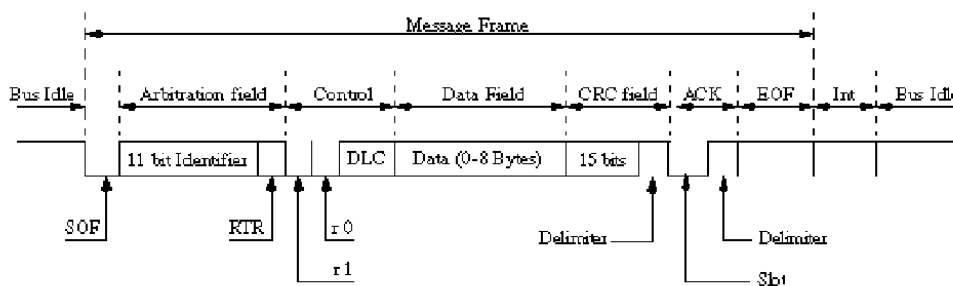
Figura 5: Struttura messaggio nel protocollo CAN 2.0
