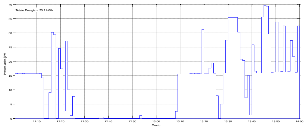
Figura 42: Potenza Attiva misurata il 20/07/2015 dalle ore 12:00
