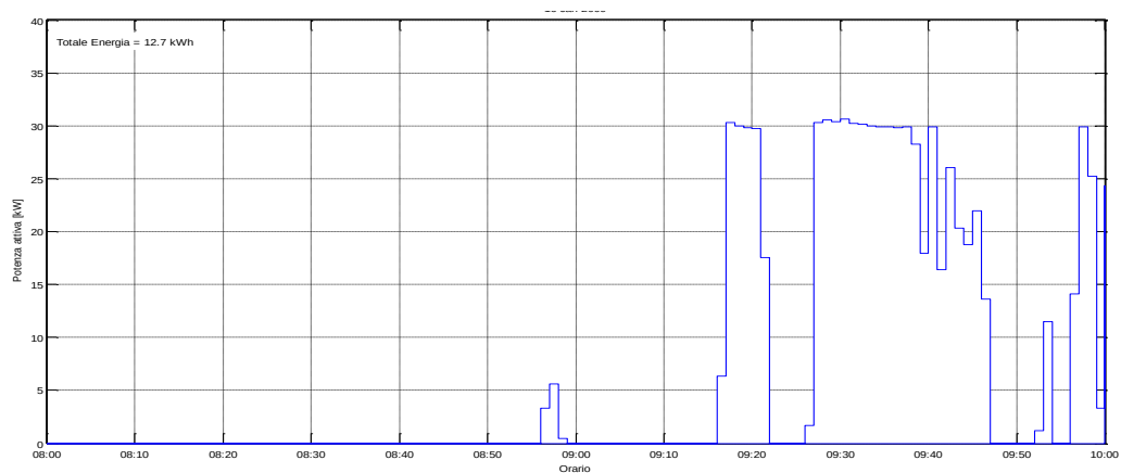
Figura 63: Potenza Attiva misurata il 24/07/2015 dalle ore 08:00
