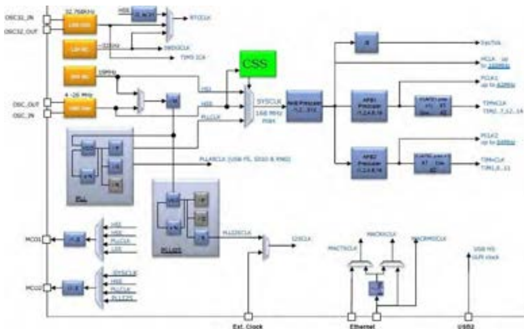
Figura 16: Schema del Clock del microcontrollore ARM Cortex M4
