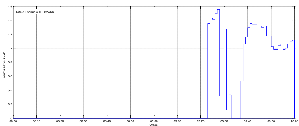
Figura 96: Potenza Reattiva misurata il 22/07/2015 dalle ore 08:00
