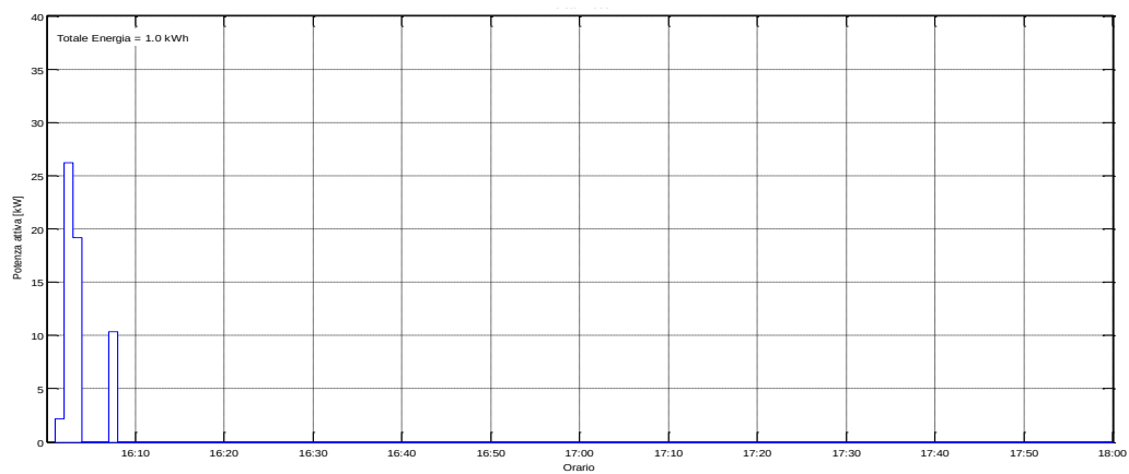
Figura 36: Potenza Attiva misurata il 18/07/2015 dalle ore 16:00
