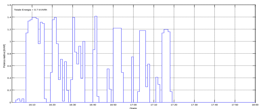
Figura 118: Potenza Reattiva misurata il 25/07/2015 dalle ore 16:00
