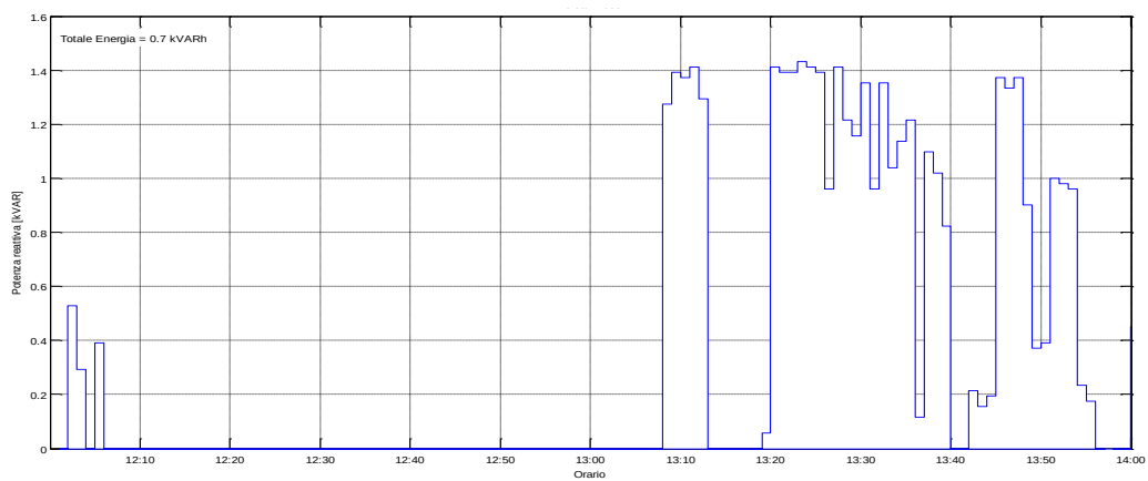
Figura 110: Potenza Reattiva misurata il 24/07/2015 dalle ore 12:00
