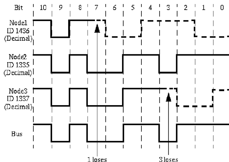
Figura 4: Esempio di arbitraggio nell'accesso al bus CAN
