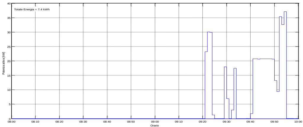
Figura 32: Potenza Attiva misurata il 18/07/2015 dalle ore 08:00
