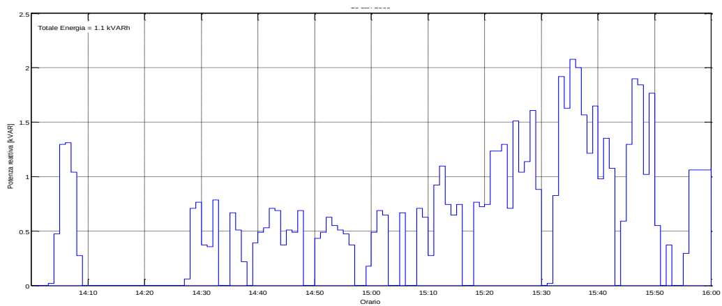
Figura 111: Potenza Reattiva misurata il 24/07/2015 dalle ore 14:00
