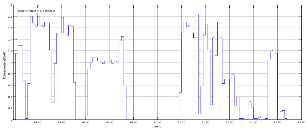
Figura 97: Potenza Reattiva misurata il 22/07/2015 dalle ore 10:00
