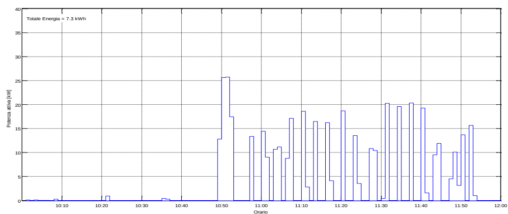
Figura 33: Potenza Attiva misurata il 18/07/2015 dalle ore 10:00
