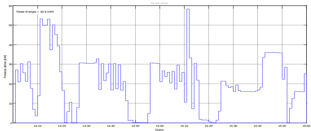
Figura 60: Potenza Attiva misurata il 23/07/2015 dalle ore 14:00
