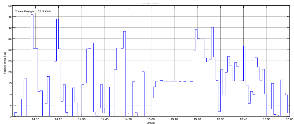
Figura 48: Potenza Attiva misurata il 21/07/2015 dalle ore 14:00
