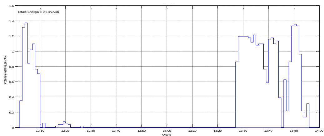
Figura 116: Potenza Reattiva misurata il 25/07/2015 dalle ore 12:00
