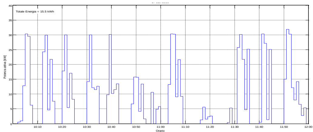
Figura 70: Potenza Attiva misurata il 25/07/2015 dalle ore 10:00
