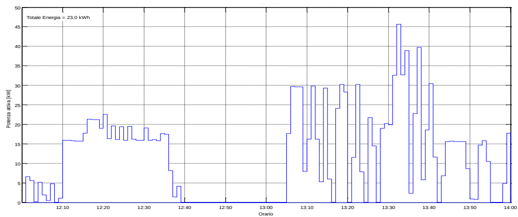
Figura 53: Potenza Attiva misurata il 22/07/2015 dalle ore 12:00
