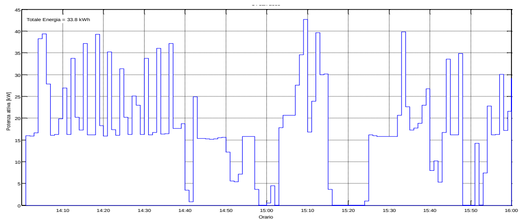
Figura 54: Potenza Attiva misurata il 22/07/2015 dalle ore 14:00
