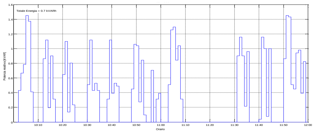
Figura 115: Potenza Reattiva misurata il 25/07/2015 dalle ore 10:00
