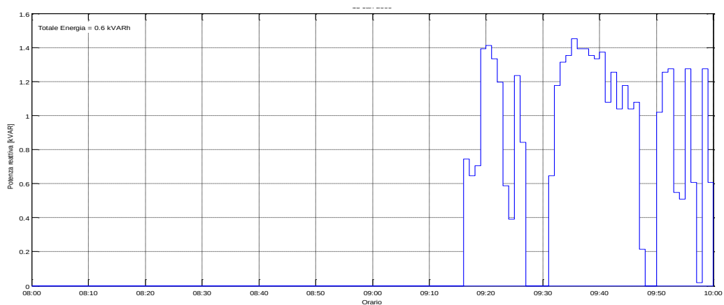
Figura 90: Potenza Reattiva misurata il 21/07/2015 dalle ore 08:00
