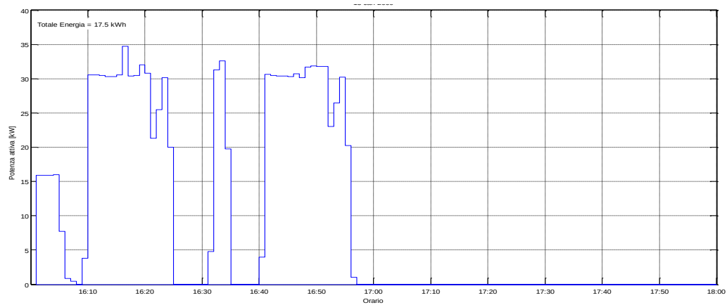
Figura 61: Potenza Attiva misurata il 23/07/2015 dalle ore 16:00
