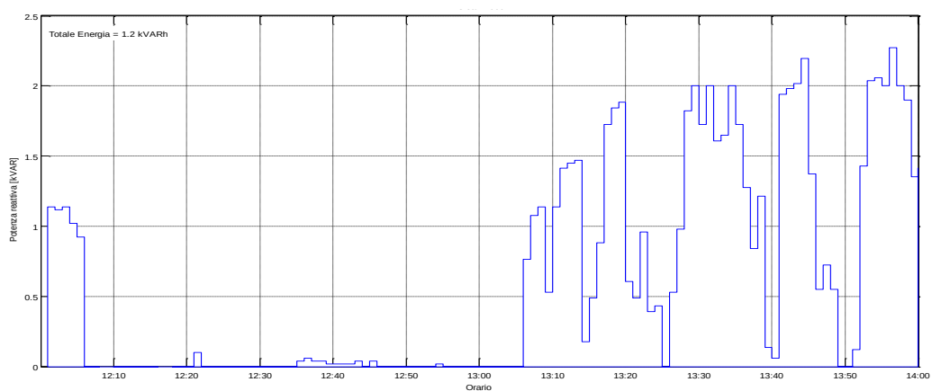
Figura 104: Potenza Reattiva misurata il 23/07/2015 dalle ore 12:00
