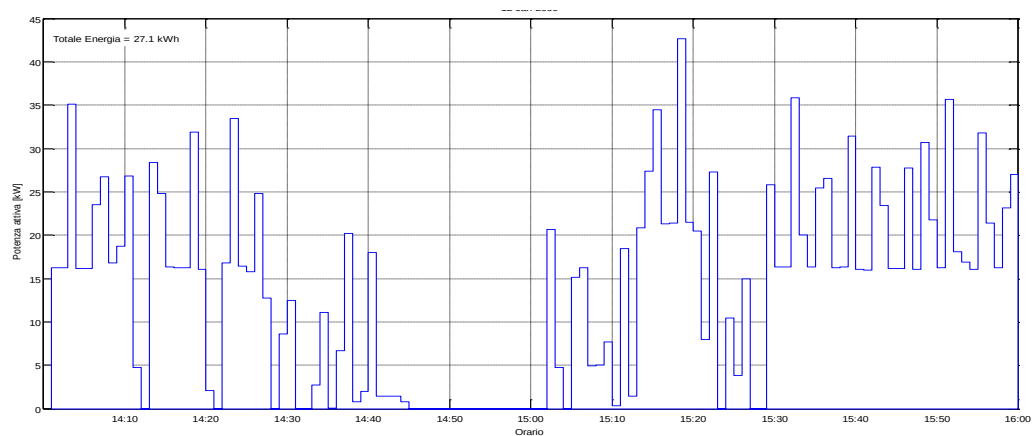
Figura 43: Potenza Attiva misurata il 20/07/2015 dalle ore 14:00
