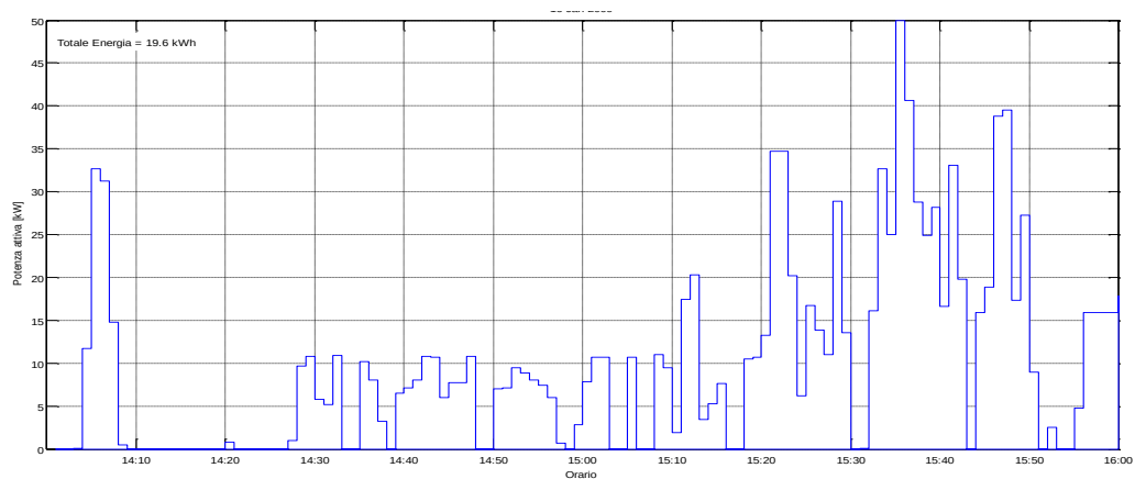
Figura 66: Potenza Attiva misurata il 24/07/2015 dalle ore 14:00
