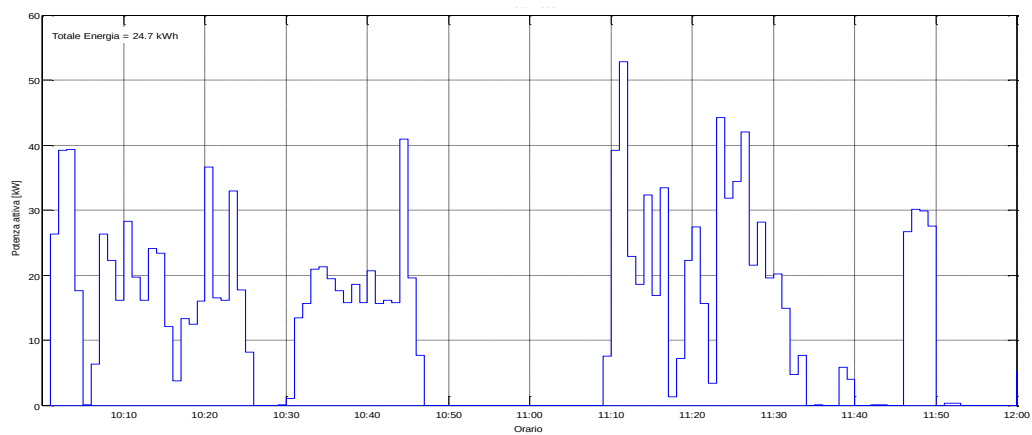
Figura 52: Potenza Attiva misurata il 22/07/2015 dalle ore 10:00
