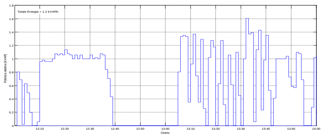
Figura 98: Potenza Reattiva misurata il 22/07/2015 dalle ore 12:00
