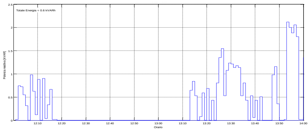
Figura 92: Potenza Reattiva misurata il 21/07/2015 dalle ore 12:00
