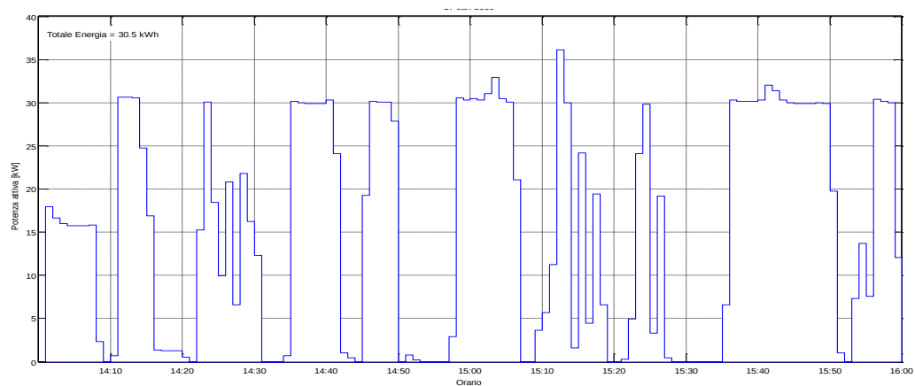
Figura 72: Potenza Attiva misurata il 25/07/2015 dalle ore 14:00
