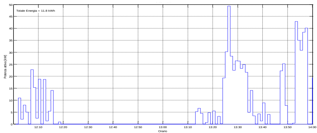
Figura 47: Potenza Attiva misurata il 21/07/2015 dalle ore 12:00
