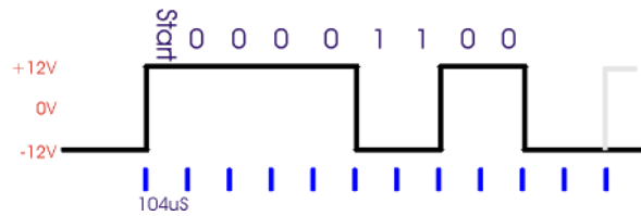
Figura 2: Esempio segnale RS-232
