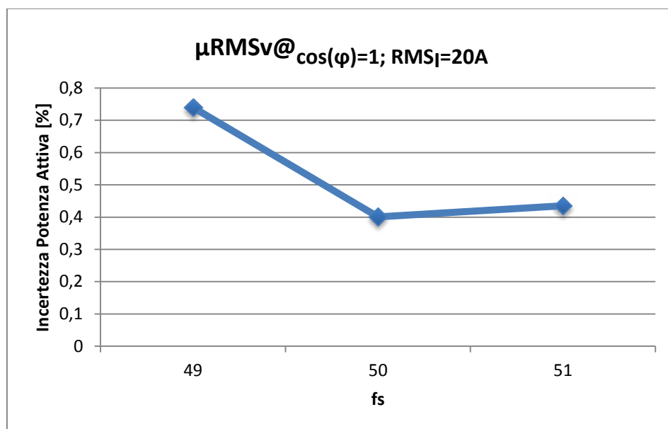
Figura 25: Incertezza nella misura di potenza rispetto alla frequenza
