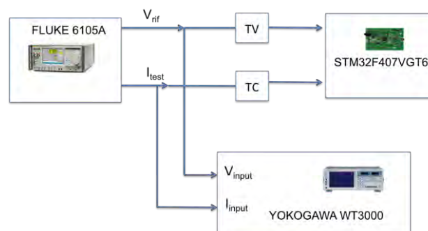
Figura 21: Connessione strumentazione per caratterizzazione SM
