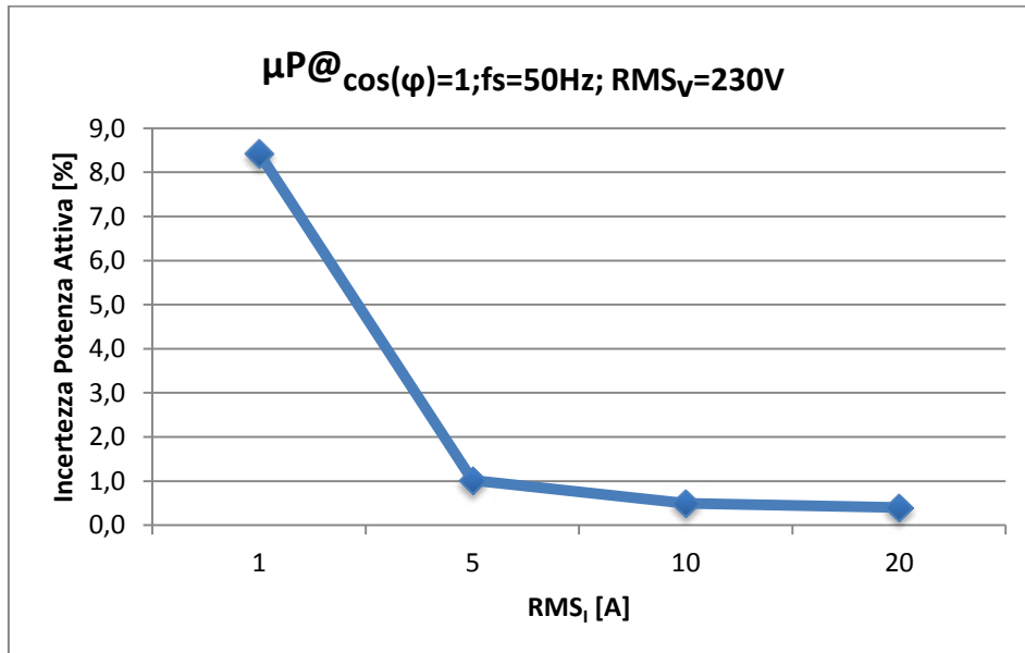
Figura 23: Incertezza nella misura di potenza rispetto alla corrente
