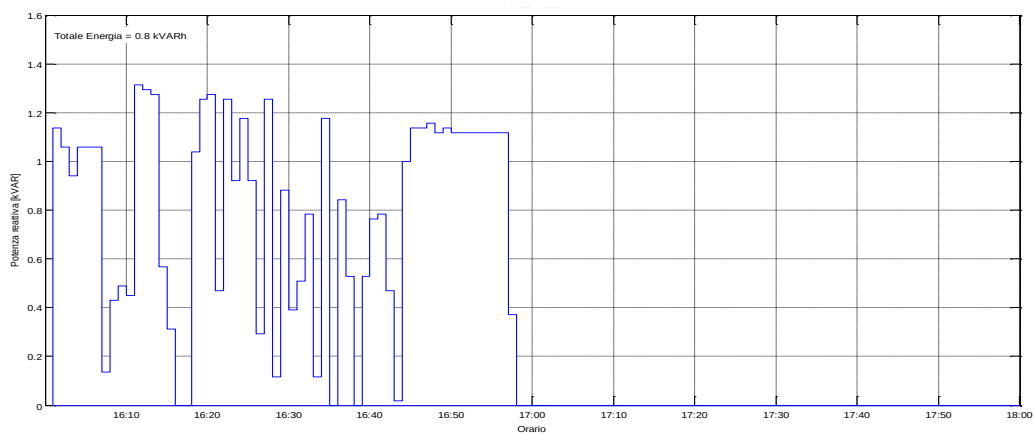
Figura 112: Potenza Reattiva misurata il 24/07/2015 dalle ore 16:00
