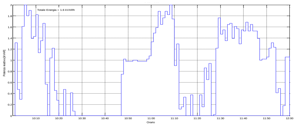
Figura 103: Potenza Reattiva misurata il 23/07/2015 dalle ore 10:00
