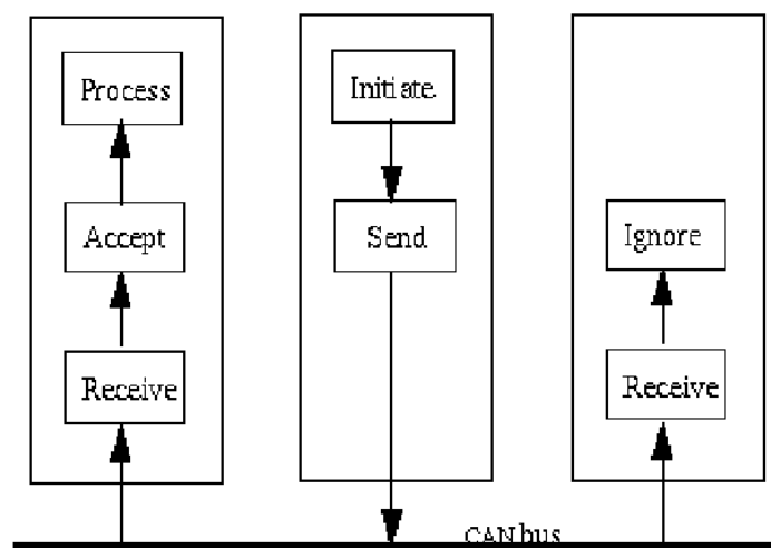
Figura 3: Esempio di message filtering: l'informazione del nodo 2 è ricevuta dal nodo 1 ma ignorata dal nodo 3
