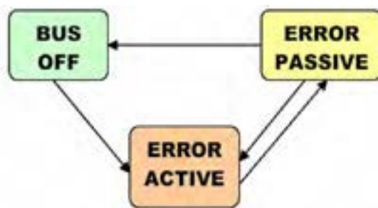
Figura 6: Stati di un nodo CAN
