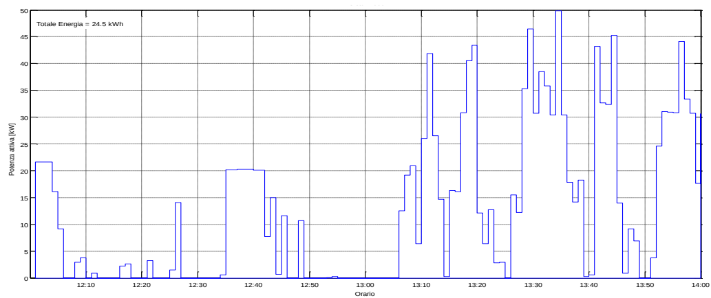
Figura 59: Potenza Attiva misurata il 23/07/2015 dalle ore 12:00
