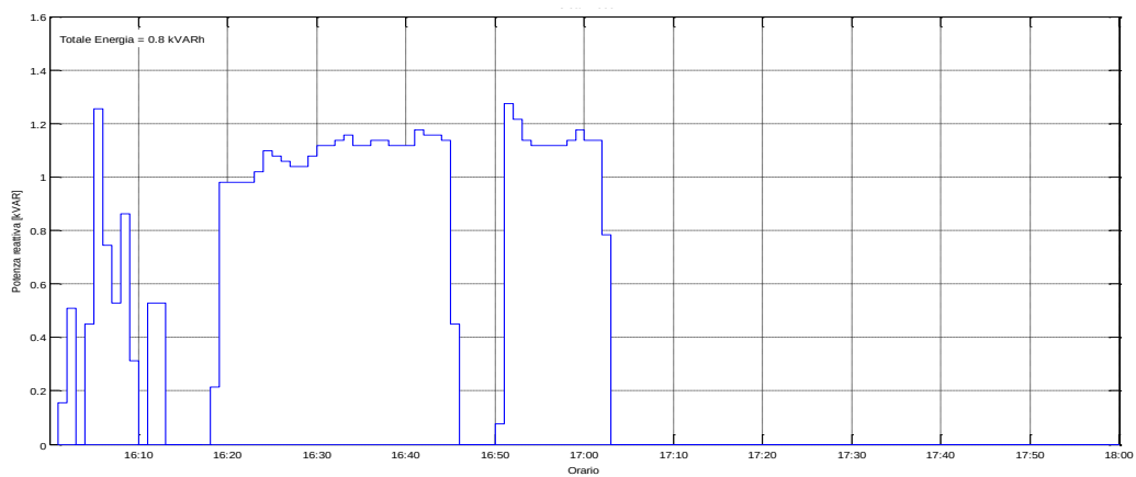
Figura 94: Potenza Reattiva misurata il 21/07/2015 dalle ore 16:00
