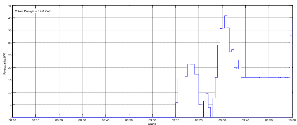
Figura 57: Potenza Attiva misurata il 23/07/2015 dalle ore 08:00
