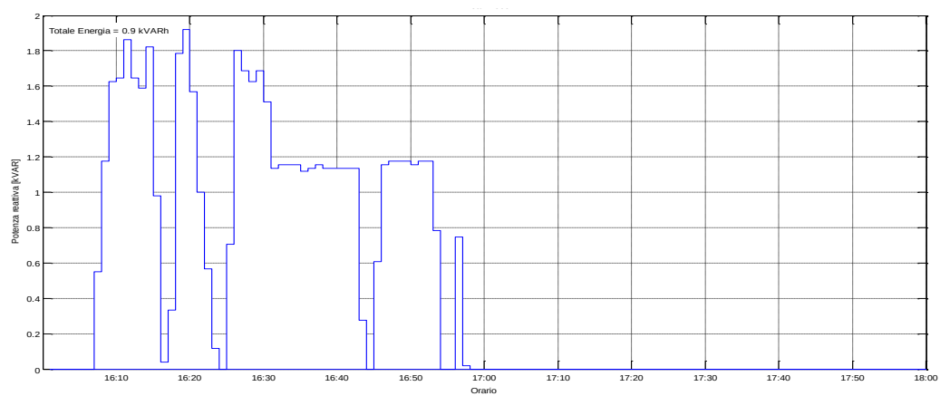
Figura 88: Potenza Reattiva misurata il 20/07/2015 dalle ore 16:00
