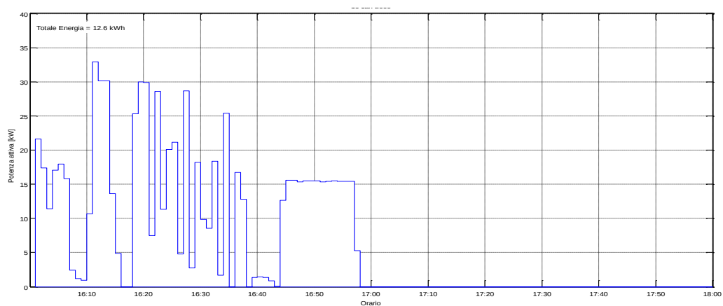
Figura 67: Potenza Attiva misurata il 24/07/2015 dalle ore 16:00
