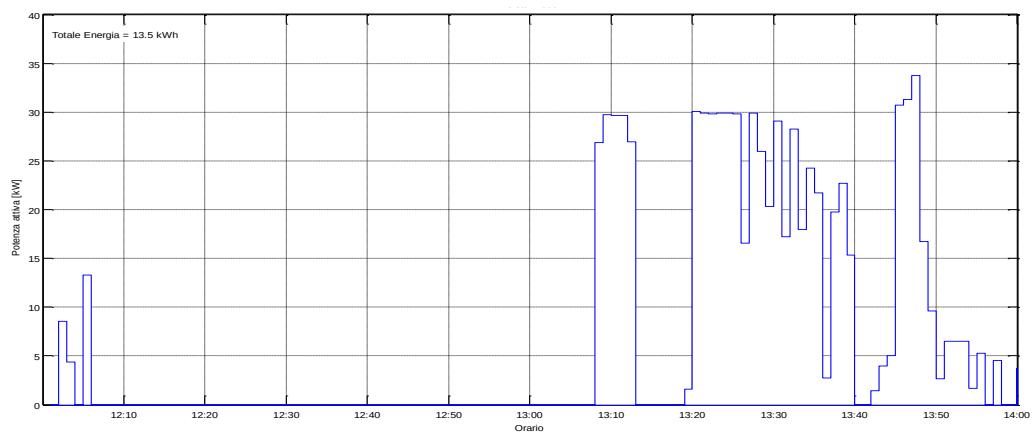
Figura 65: Potenza Attiva misurata il 24/07/2015 dalle ore 12:00
