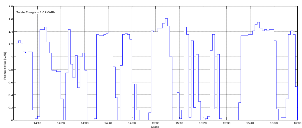
Figura 117: Potenza Reattiva misurata il 25/07/2015 dalle ore 14:00
