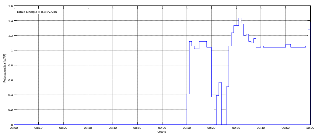
Figura 102: Potenza Reattiva misurata il 23/07/2015 dalle ore 08:00
