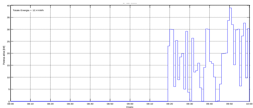
Figura 69: Potenza Attiva misurata il 25/07/2015 dalle ore 08:00
