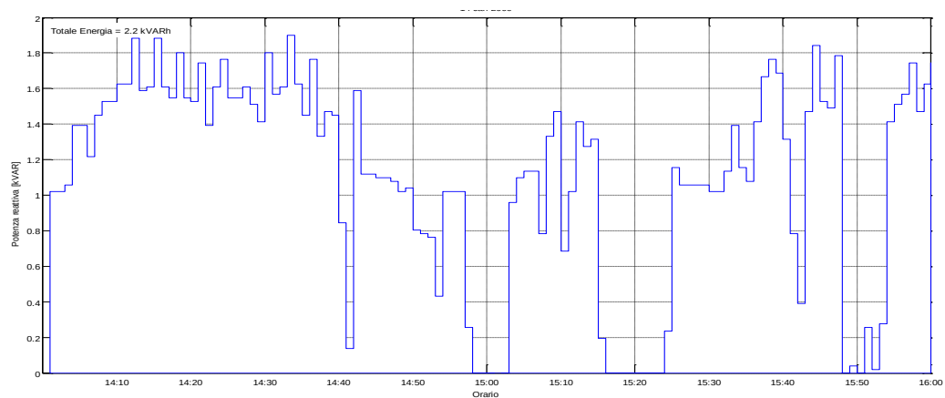
Figura 99: Potenza Reattiva misurata il 22/07/2015 dalle ore 14:00
