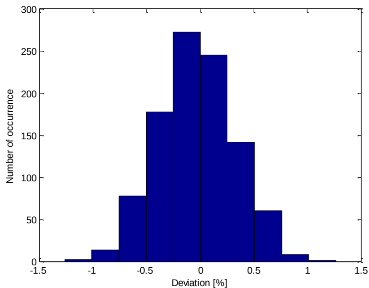
Figura 28: Scostamenti percentuali nelle misure di Potenza Reattiva
