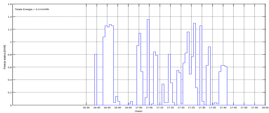
Figura 74: Potenza Reattiva misurata il 17/07/2015 dalle ore 16:35
