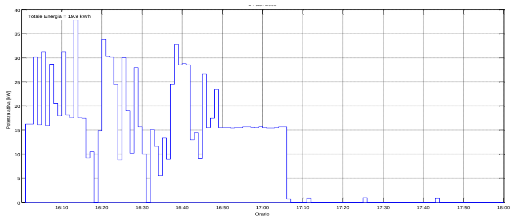
Figura 55: Potenza Attiva misurata il 22/07/2015 dalle ore 16:00
