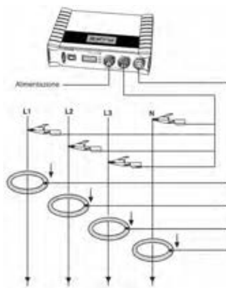
Figura 26: Inserzione del misuratore commerciale
