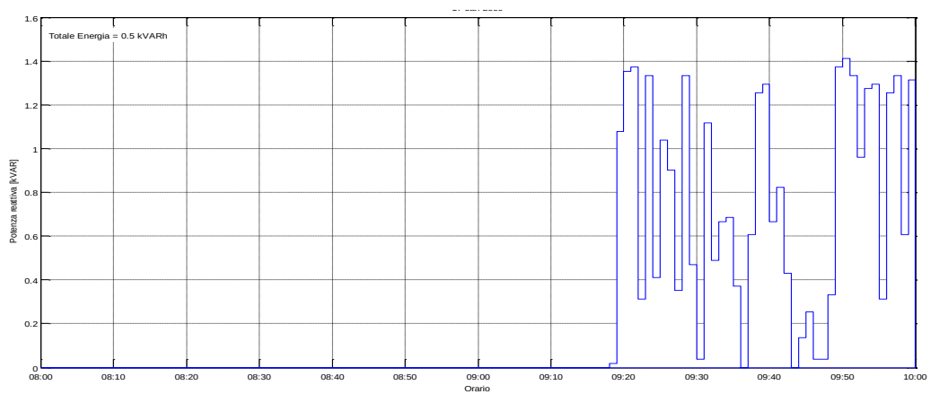
Figura 114: Potenza Reattiva misurata il 25/07/2015 dalle ore 08:00
