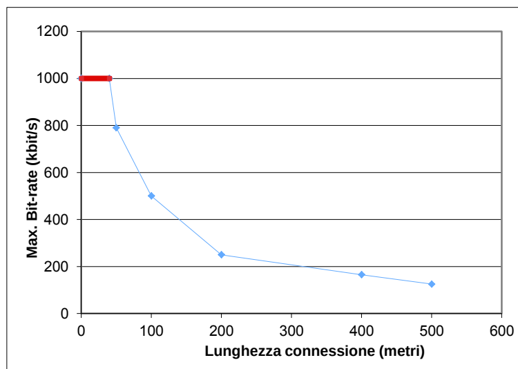
Figura 7: Velocità di trasmissione in funzione della lunghezza del bus
