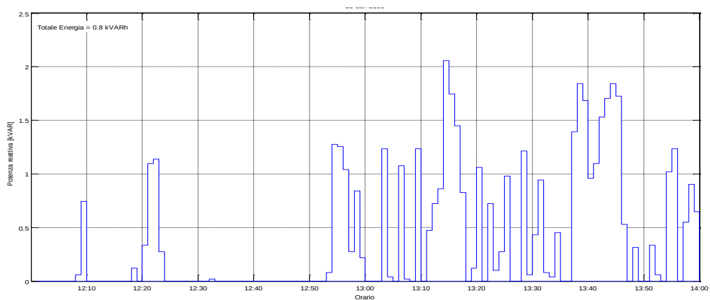
Figura 78: Potenza Reattiva misurata il 18/07/2015 dalle ore 12:00
