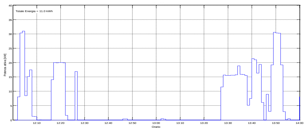
Figura 71: Potenza Attiva misurata il 25/07/2015 dalle ore 12:00
