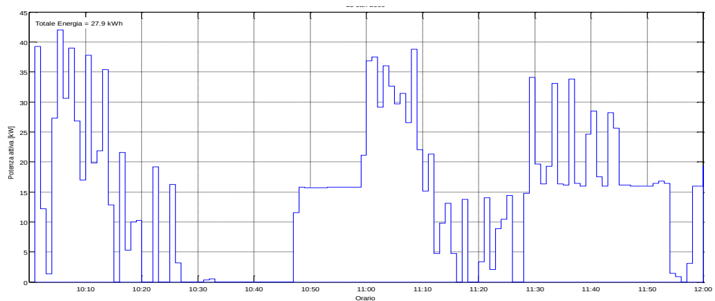
Figura 58: Potenza Attiva misurata il 23/07/2015 dalle ore 10:00
