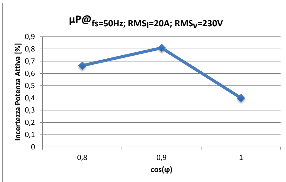
Figura 24: Incertezza nella misura di potenza rispetto al fattore di potenza
