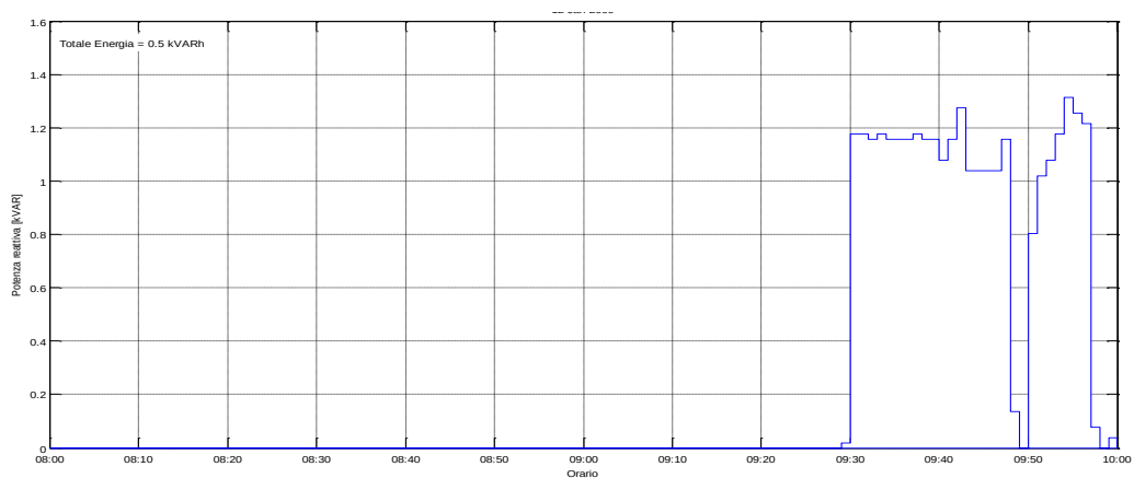
Figura 84: Potenza Reattiva misurata il 20/07/2015 dalle ore 08:00
