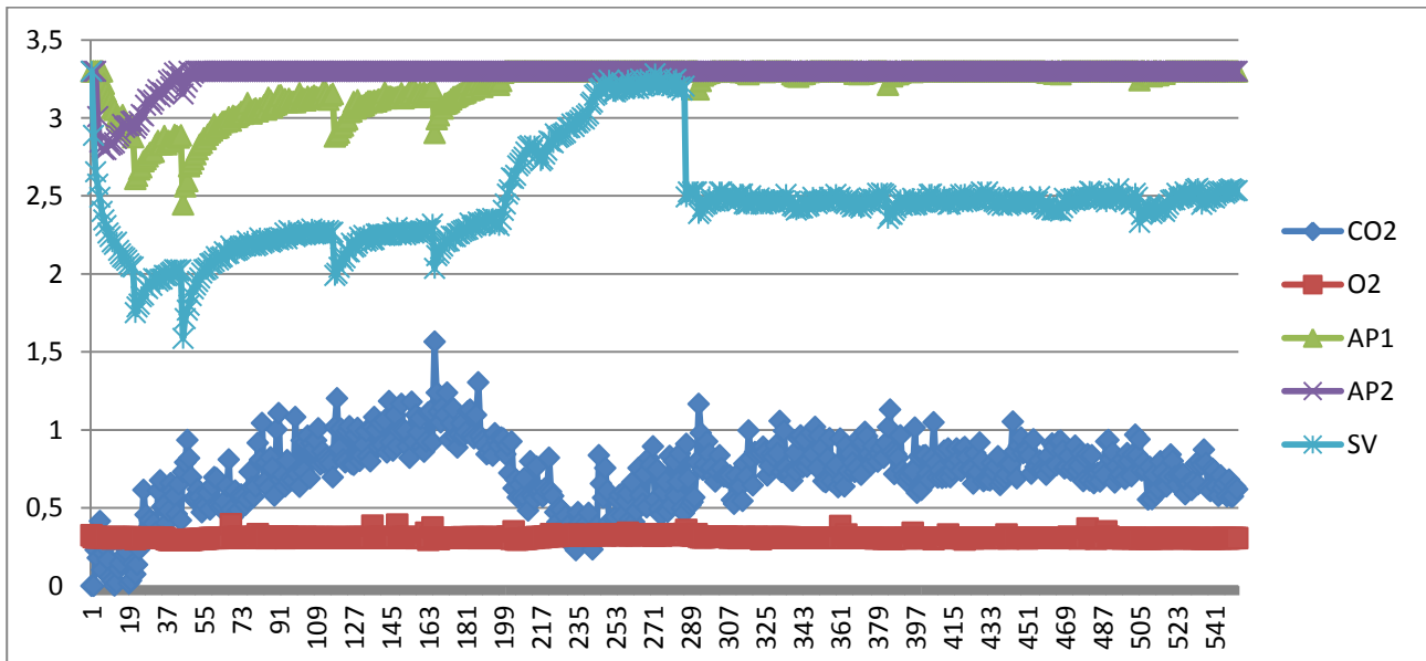
Figura 2.56: Nodo sensoriale 3, pere conservate a 151°C, acquisizioni effettuate con frequenza oraria per i 3 sensori aspecifici e per i sensori di ossigeno e anidride carbonica.
