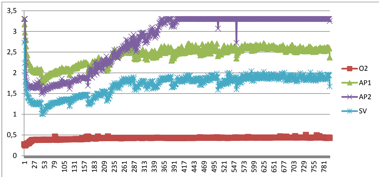
Figura 2.55: Nodo sensoriale 2, pere conservate a 11°C, acquisizioni effettuate con frequenza oraria per i 3 sensori aspecifici e per il sensore di ossigeno.
