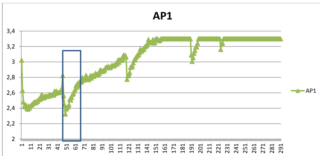
Figura 2.21: sensore AP1 Libelium, susine. Andamento del sensore AP1 di un nodo sensoriale per le susine con tempi di trasmissione di 1 ora. Il rettangolo indica il lasso temporale di 24 ore, periodo di recupero del livello di composti volatili dello spazio di testa.
