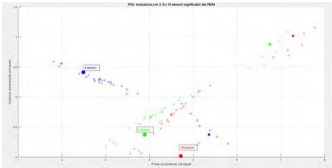
Figura 2.8: susine a 5 °C in camera. PCA utilizzando tutti i 10 sensori , i 6 maggiormente significativi , e i 3 sensori maggiormente significativi . Cerchi pieni più grandi punti di partenza, cerchi pieni piccoli punti di arrivo.
