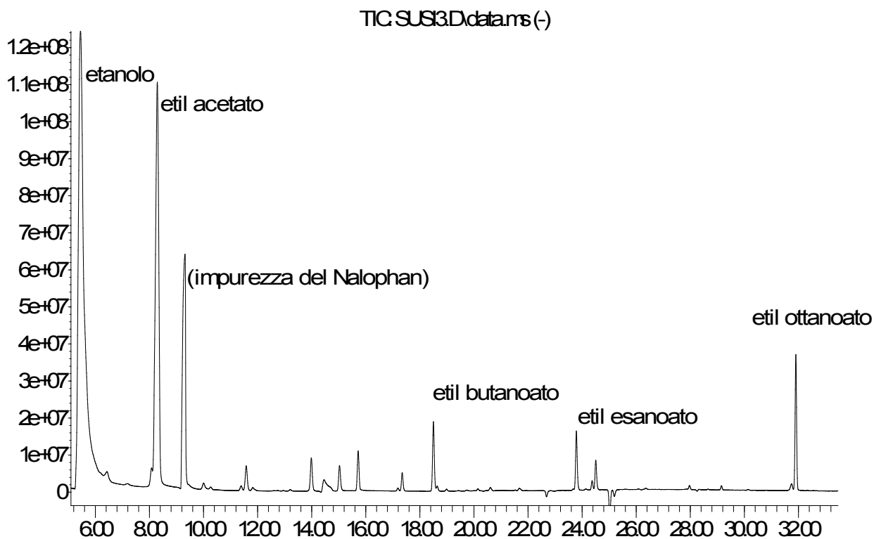
Figura 2.22: Meta-cromatogramma generato dalla differenza tra i cromatogrammi relativi alle emissioni di alcune susine conservate in busta di Nalophan a distanza di alcuni giorni a temperatura ambiente;
