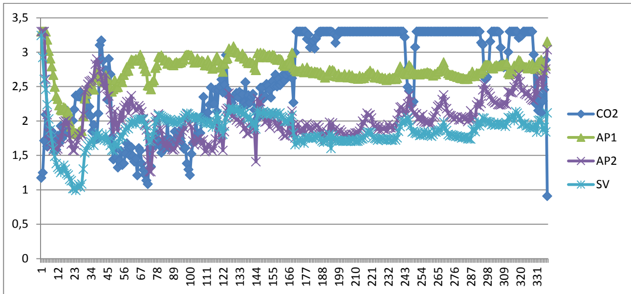
Figura 2.57: Nodo sensoriale 4, pere conservate a temperatura ambiente in laboratorio, acquisizioni effettuate con frequenza oraria per i 3 sensori aspecifici e per il sensore di anidride carbonica.
