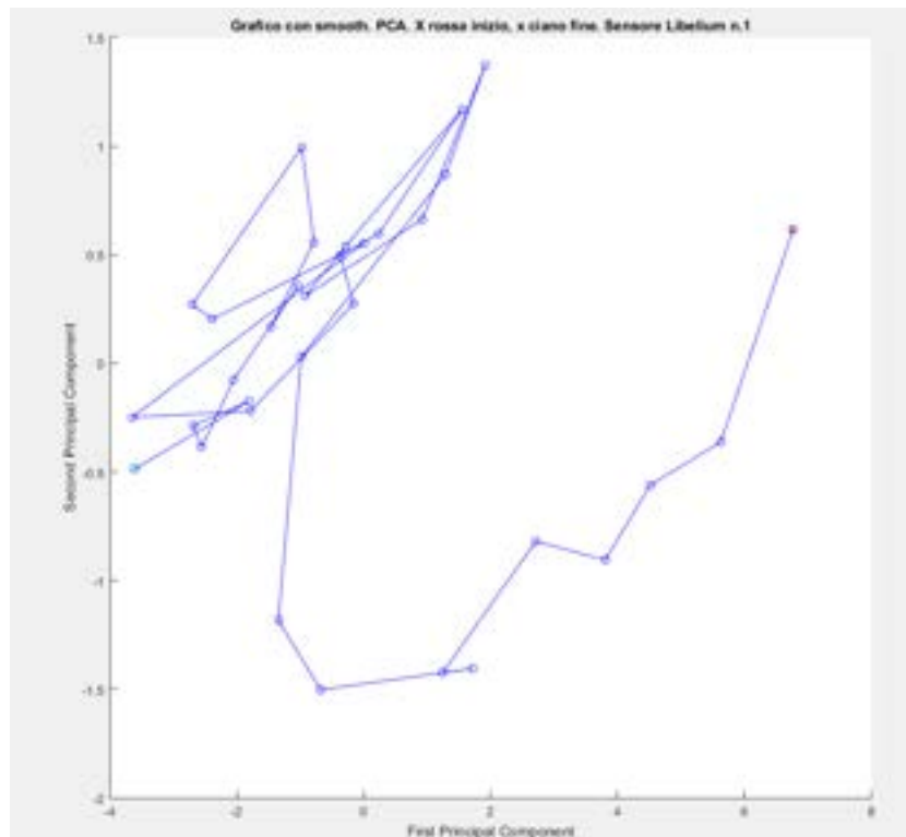
Figura 2.62: PCA, pere. Andamento della PCA utilizzando 7 sensori e con media su 5 campioni precedenti e decimazione di valore 24.
