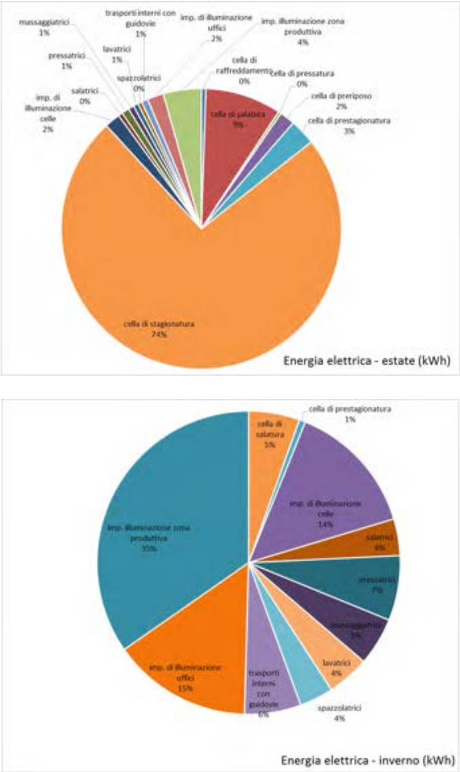
Figura 8 – Rappresentazione grafica dei consumi elettrici estate-inverno di un prosciuttificio tipo
