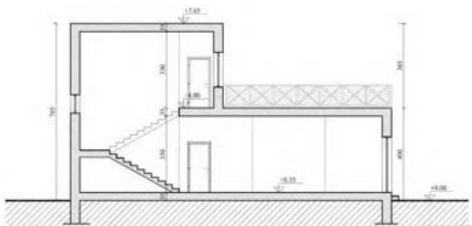
Figura 20 “Piccola palazzina per uffici. Sezione A-A”
