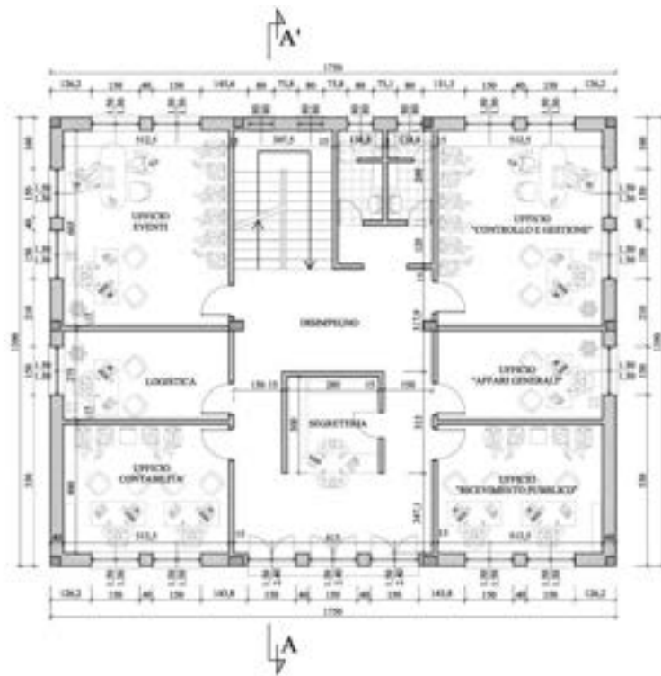
Figura 14 "Piccola palazzina per uffici. Pianta Piano Terra"
