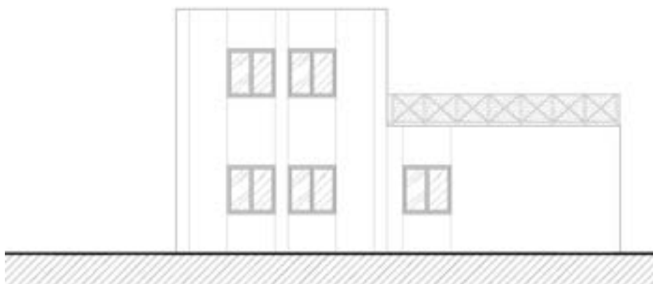
Figura 19 “Piccola palazzina per uffici. Prospetto Ovest”
