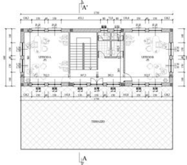
Figura 15 "Piccola palazzina per uffici. Pianta Piano primo"
