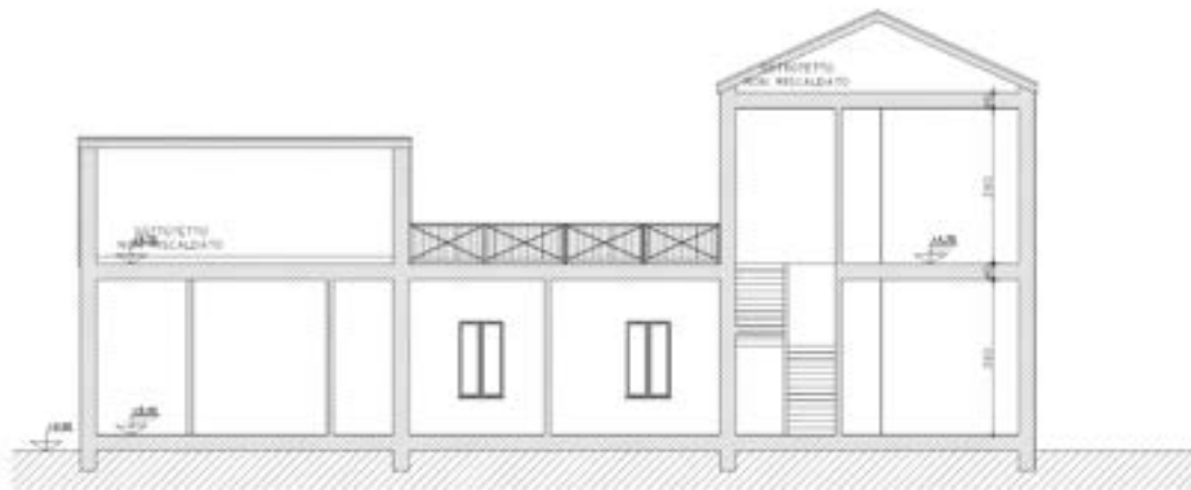
Figura 12 "Casolare di montagna di modesta entità. Sezione A-A"
