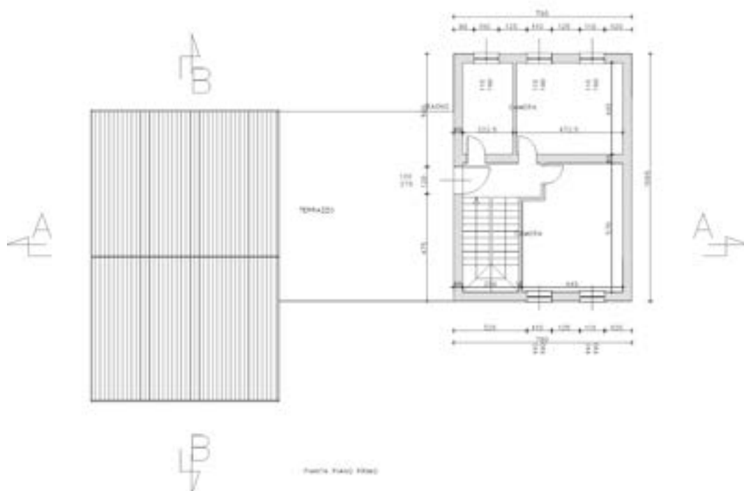
Figura 7 “Casolare di montagna di modesta entità. Pianta Piano primo”
