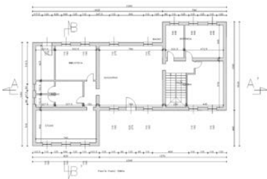
Figura 6 “Casolare di montagna di modesta entità. Pianta Piano Terra”
