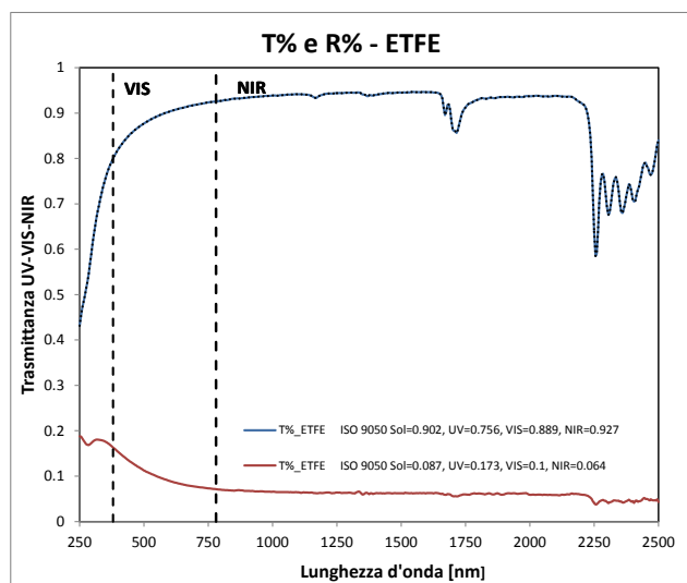
Fig. 38 - Trasmittanza e riflettanza spettrale di campione di ETFE non trattato – trasparente – 200 μm
