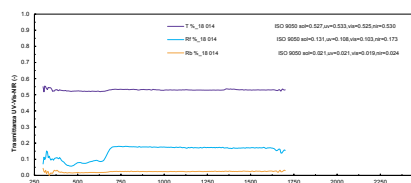
18014 – Tessuto in PET tridimensionale
