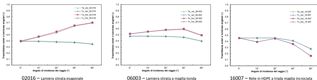
Fig. 26 - \tau_v e \tau_e al variare dell'orientamento del campione e dell'angolo di incidenza della radiazione
