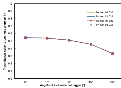
01033 – Tessuto in PET nero con coating in Ti
