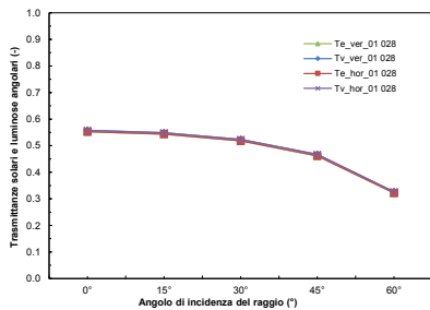
01028 – Tessuto in PET nero con coating in Cr
