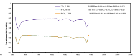
17008 – Tessuto in PES tridimensionale spesso
