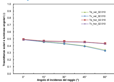
02010 – Lamiera in alluminio forata con foro oblungho
