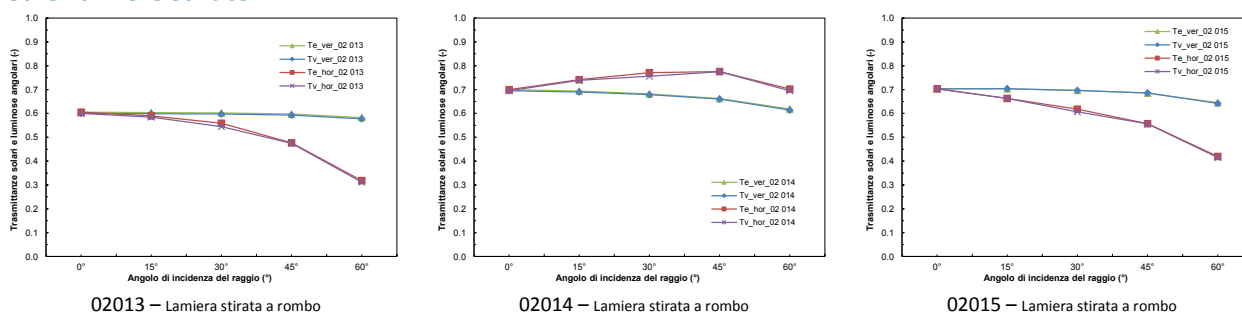
Fig. 25 - \tau_v e \tau_e al variare dell'orientamento del campione e dell'angolo d'incidenza della radiazione
