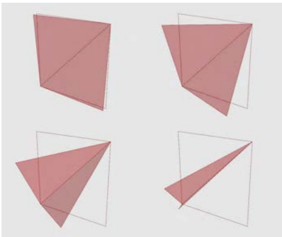
Fig. 76 – Modello C: Modello funzionale a elementi mobili rigidi, apertura massima 100%, presenza di elementi aggettanti
