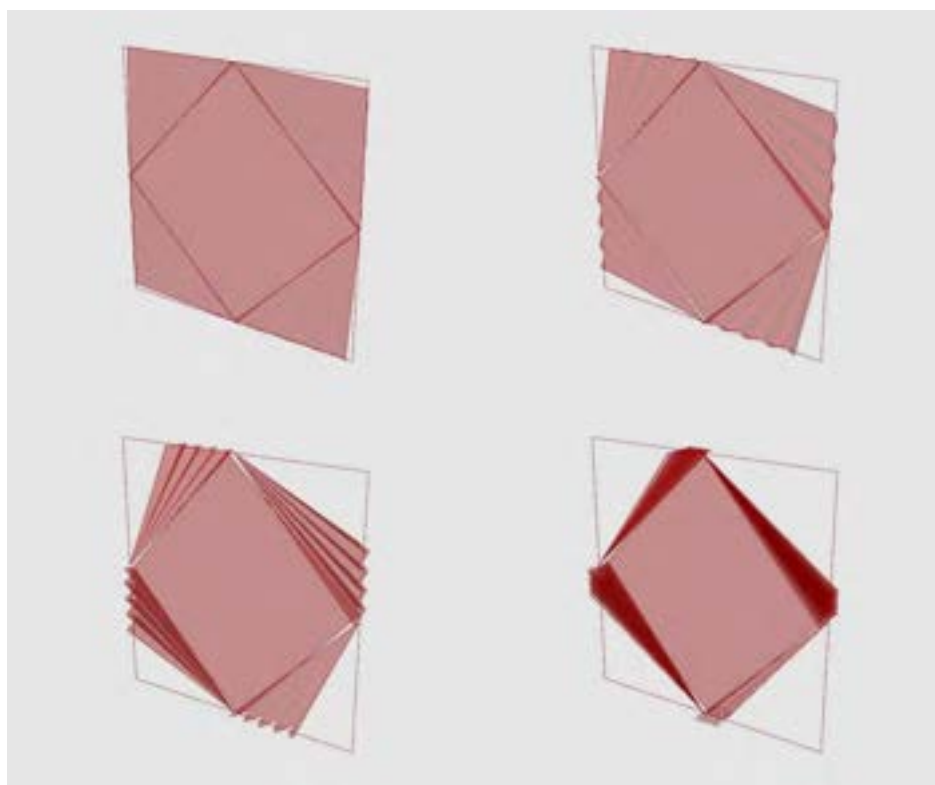
Fig. 81 – Modello H: Modello funzionale a 4 elementi flessibili plissettati ed elemento fisso centrale, apertura massima variabile, assenza di elementi aggettanti
