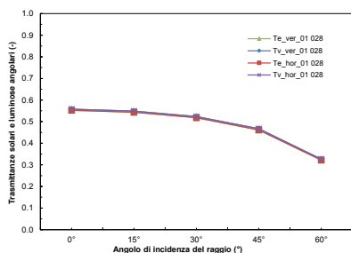
01028 – Tessuto in PET nero con coating in Cr
