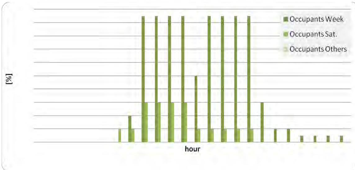
Figura 3. Profilo di occupazione dell'edificio di riferimento
