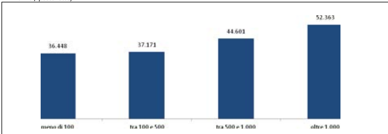
Figura 35 – Statistiche campionarie sui consumi termici specifici delle strutture ospedaliere per numero di posti letto (2012-2013, kwh annui/posto letto)
