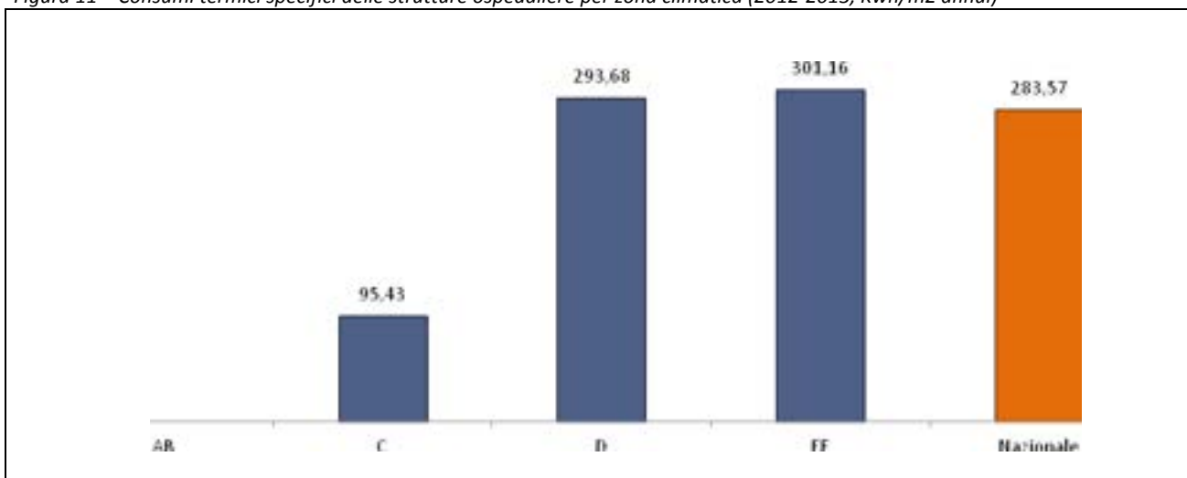
Figura 11 – Consumi termici specifici delle strutture ospedaliere per zona climatica (2012-2013, Kwh/m2 annui)
