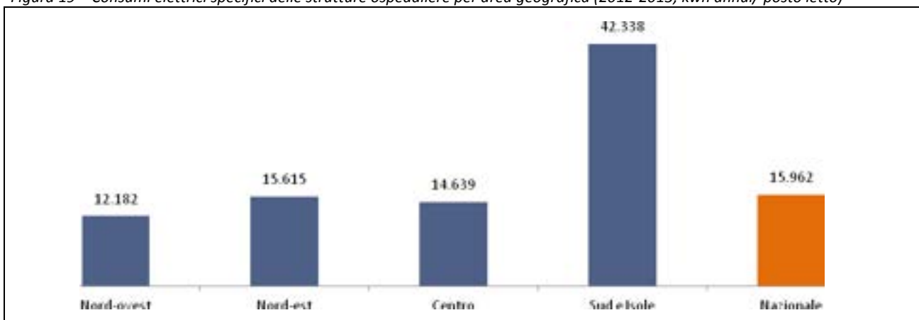
Figura 19 – Consumi elettrici specifici delle strutture ospedaliere per area geografica (2012-2013, kwh annui/ posto letto)
