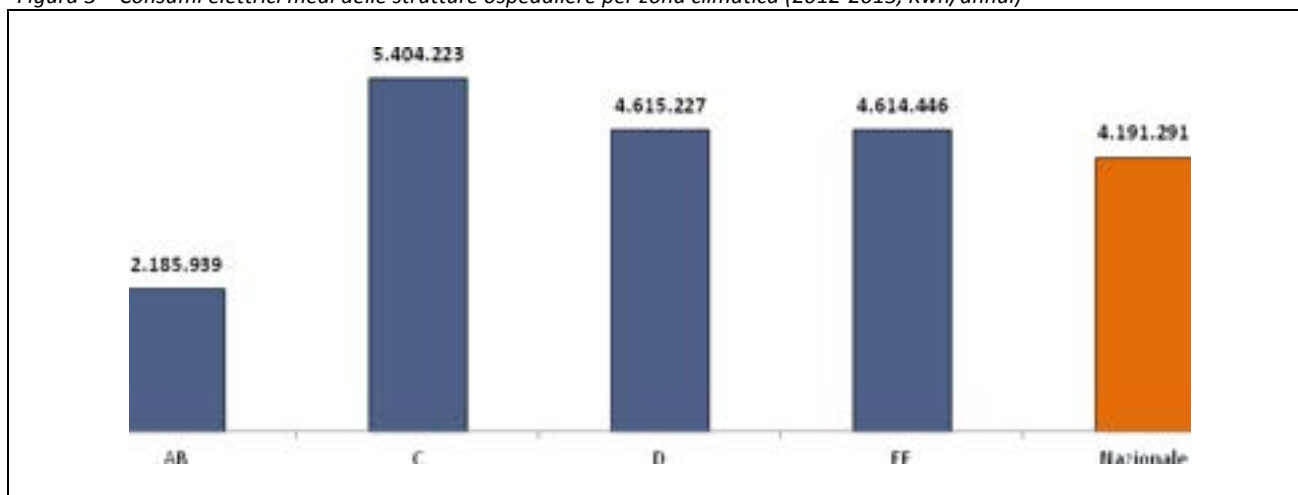
Figura 3 – Consumi elettrici medi delle strutture ospedaliere per zona climatica (2012-2013, Kwh/annui)
