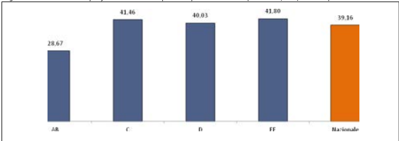
Figura 7 – Consumi elettrici specifici delle strutture ospedaliere per zona climatica (2012-2013, Kwh/m3 annui)
