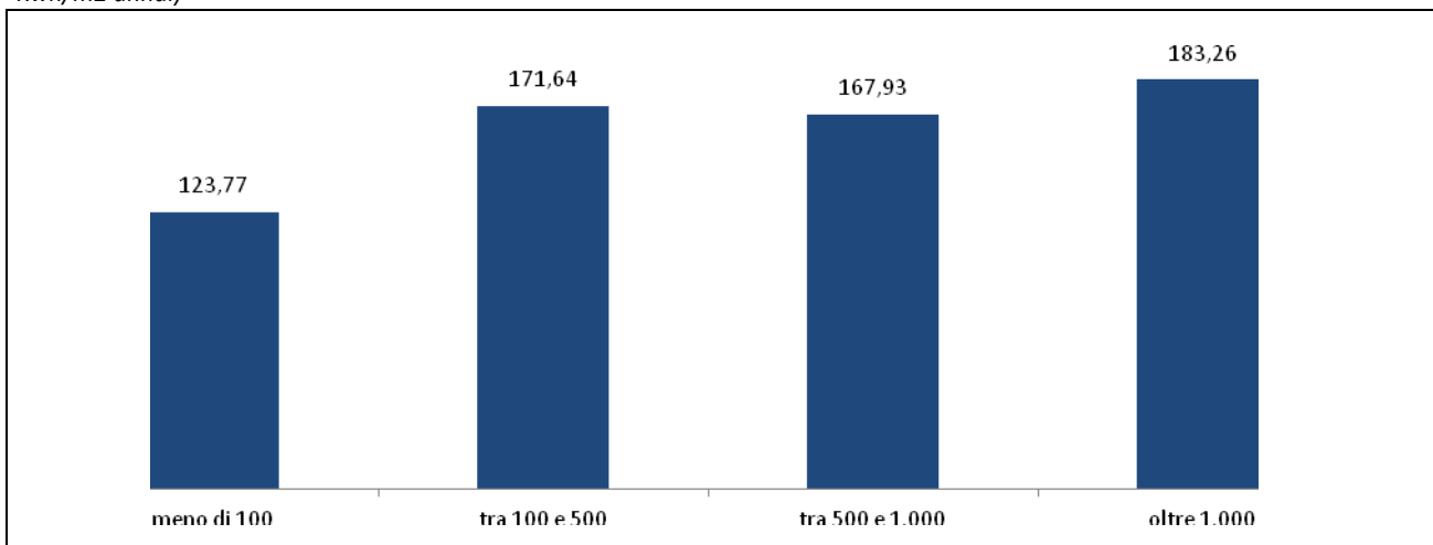
Figura 28 – Statistiche campionarie sui consumi elettrici specifici delle strutture ospedaliere per numero di posti letto (2012-2013, Kwh/m2 annui)
