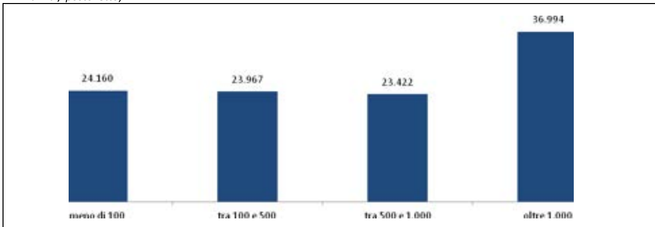
Figura 30 – Statistiche campionarie sui consumi elettrici specifici delle strutture ospedaliere per numero di posti letto (2012-2013, kwh annui/ posto letto)
