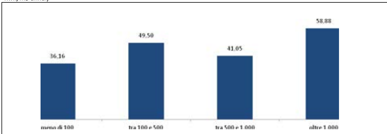
Figura 29 – Statistiche campionarie sui consumi elettrici specifici delle strutture ospedaliere per numero di posti letto (2012-2013, Kwh/m3 annui)
