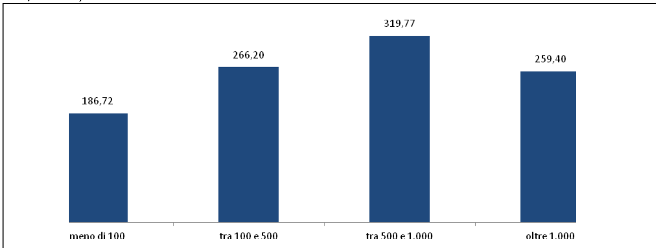
Figura 33 – Statistiche campionarie sui consumi termici specifici delle strutture ospedaliere per numero di posti letto (2012-2013, Kwh/m2 annui)
