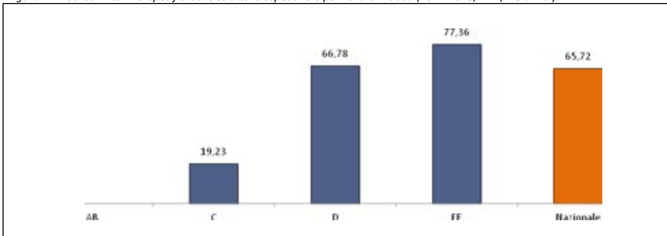
Figura 12 – Consumi termici specifici delle strutture ospedaliere per zona climatica (2012-2013, Kwh/m3 annui)
