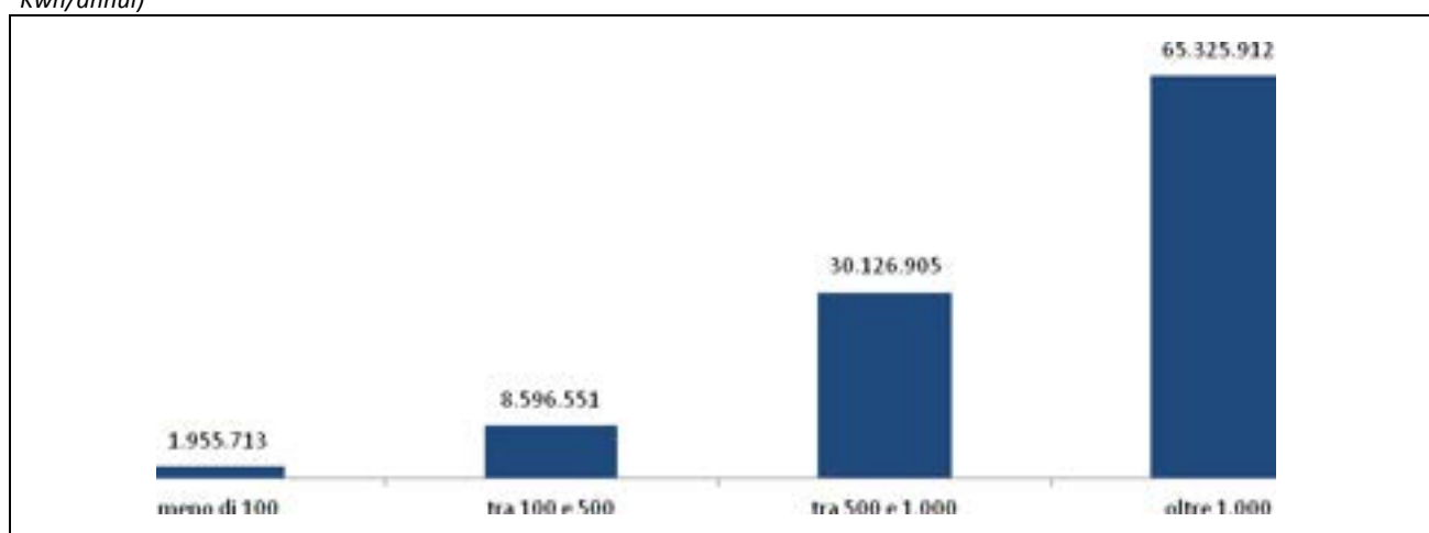
Figura 31 – Statistiche campionarie sui consumi termici delle strutture ospedaliere per numero di posti letto (2012-2013, Kwh/annui)
