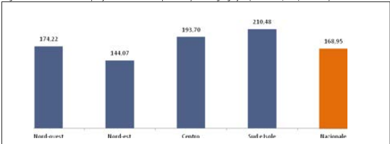
Figura 17 – Consumi elettrici specifici delle strutture ospedaliere per area geografica (2012-2013, Kwh/m2 annui)
