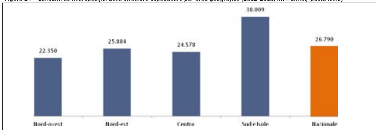
Figura 24 – Consumi termici specifici delle strutture ospedaliere per area geografica (2012-2013, kwh annui/ posto letto)
