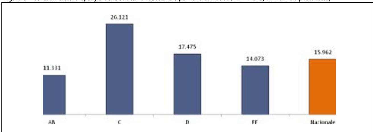
Figura 8 – Consumi elettrici specifici delle strutture ospedaliere per zona climatica (2012-2013, kwh annui/ posto letto)
