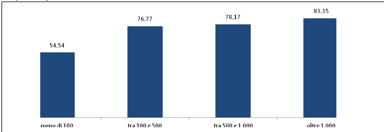
Figura 34 – Statistiche campionarie sui consumi termici specifici delle strutture ospedaliere per numero di posti letto (2012-2013, Kwh/m3 annui)
