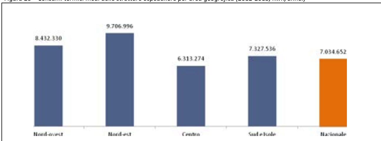
Figura 20 – Consumi termici medi delle strutture ospedaliere per area geografica (2012-2013, Kwh/annui)
