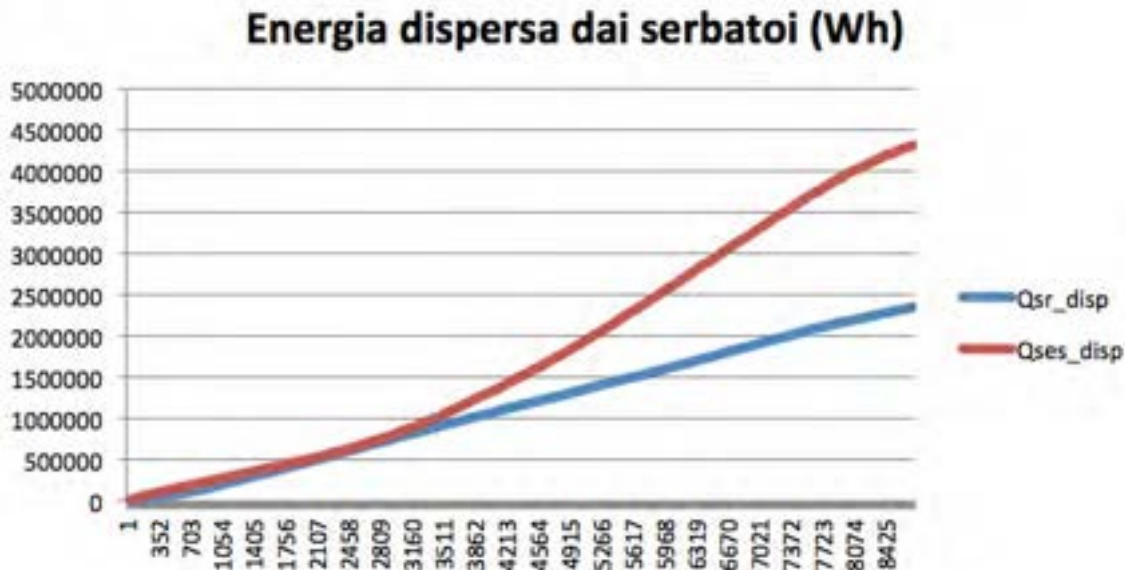
Figura 14. Valore cumulativo dell'energia persa tramite dispersioni di calore da parte dei serbatoi di accumulo (ora 1 = prima ora del primo di gennaio). Valido per edificio A, configurazione impiantistica 4, campo solare 40 m 2 , accumulo stagionale 170 m 3
