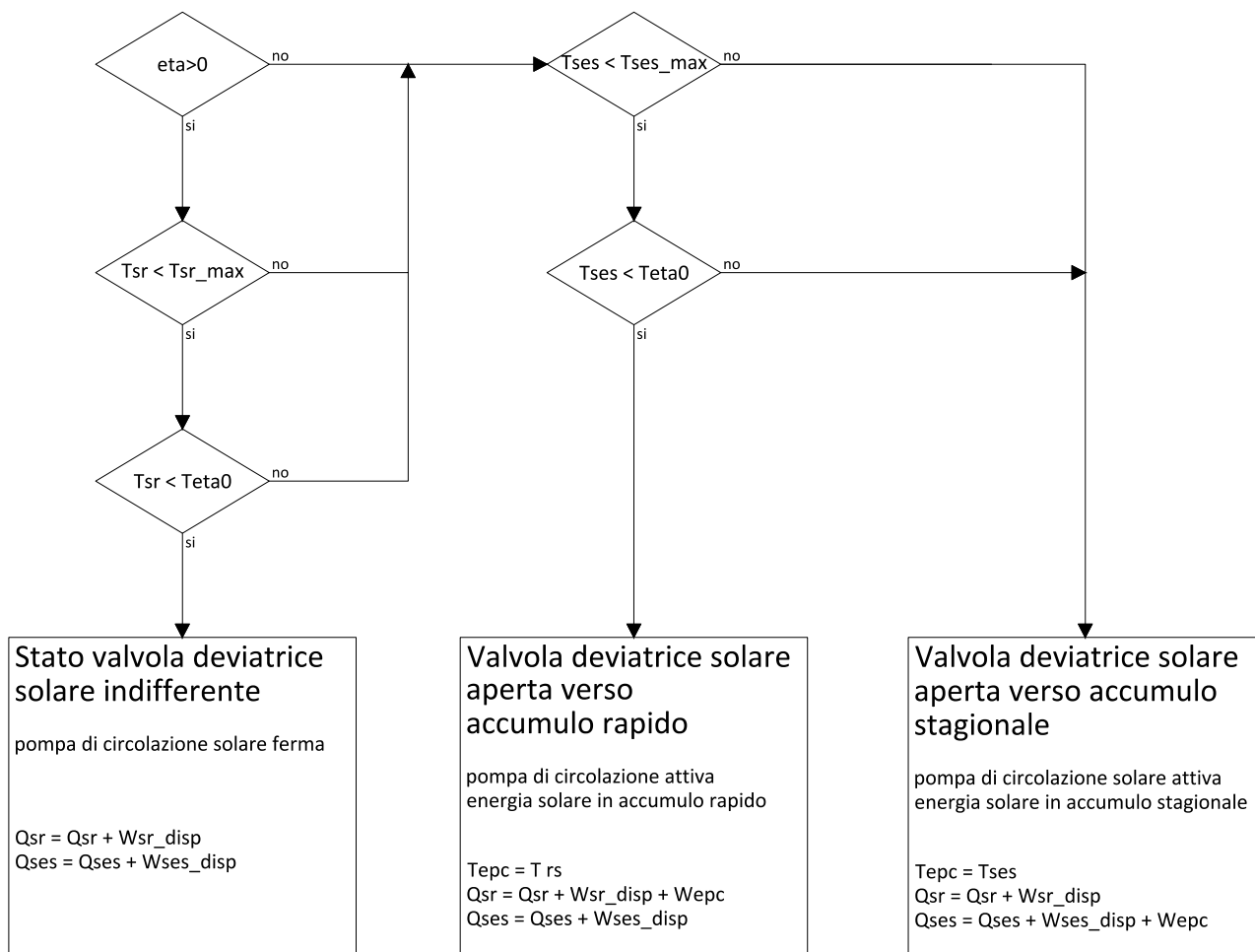
Figura 9. Rappresentazione logica della routine di gestione dell'energia proveniente dal circuito solare
