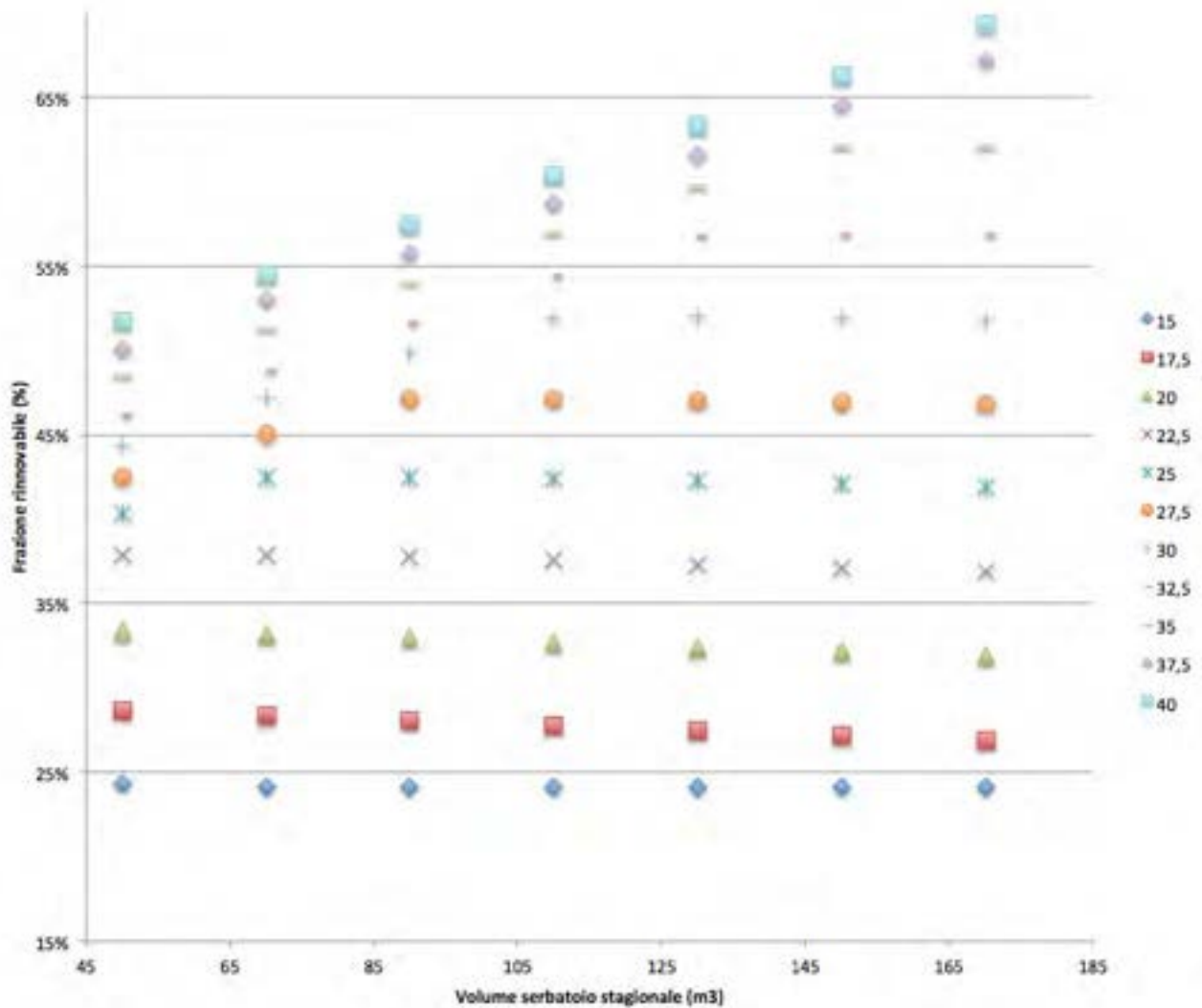
Figura 20: percentuale del fabbisogno energetico annuale dell'edificio soddisfatta tramite fonti rinnovabili in funzione delle dimensioni del serbatoio stagionale per diverse superfici complessive di apertura dell'accumulo (località Roma, edificio B, configurazione impiantistica 3)
