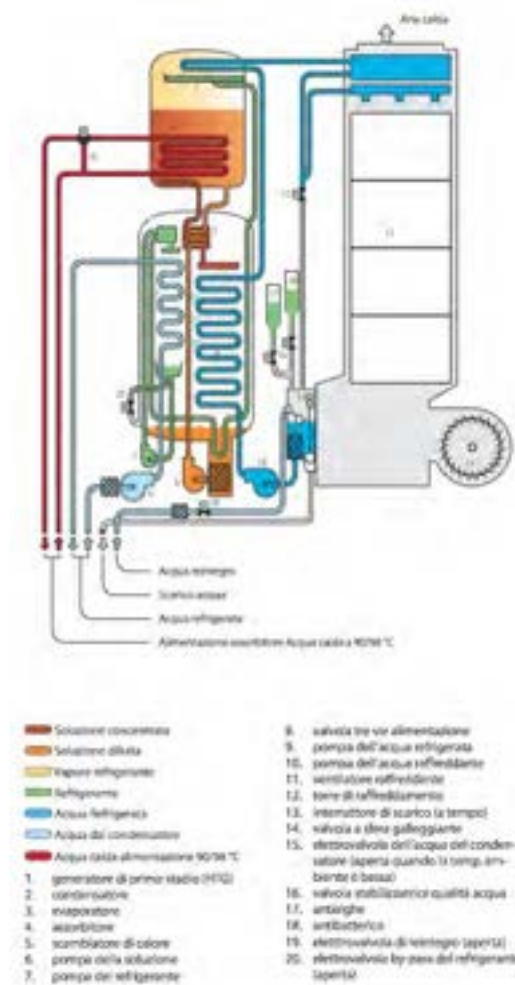
Figura 8: schema tipico di una macchina ad assorbimento a bromuro di litio [22]
