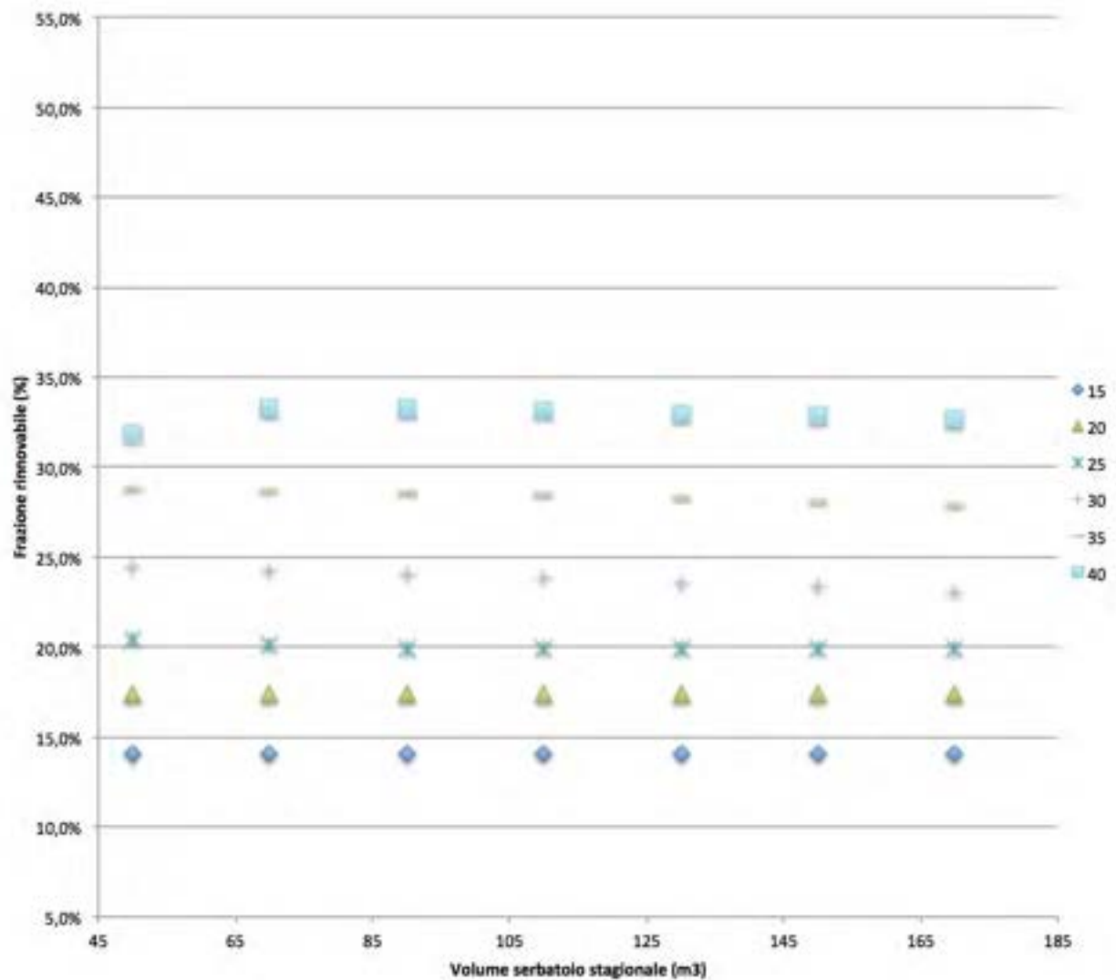
Figura 22: percentuale del fabbisogno energetico annuale dell'edificio soddisfatta tramite fonti rinnovabili in funzione delle dimensioni del serbatoio stagionale per diverse superfici complessive di apertura dell'accumulo (località Milano, edificio B, configurazione impiantistica 3)
