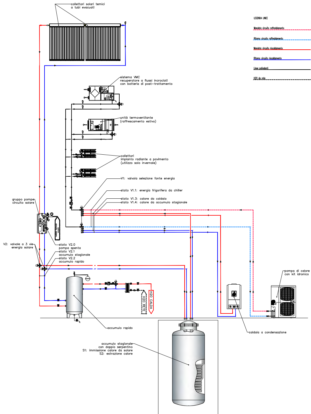
Figura 26: configurazione impiantistica 1 (adottata sia nell'edificio A, sia nell'edificio B)
