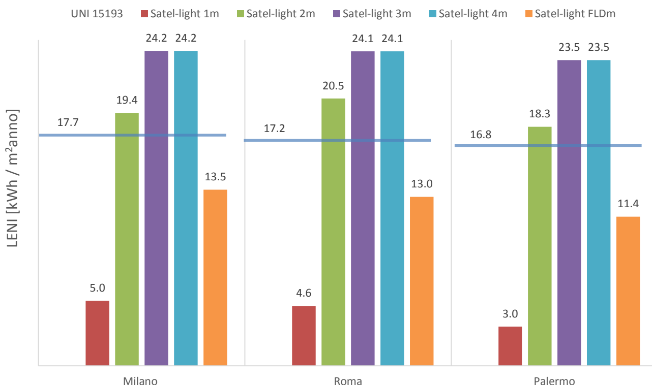
Figura 21. Calcolo del LENI per l'edificio F51 per livelli di illuminamento mantenuto di 750 lux - confronto dei risultati con i diversi metodi
