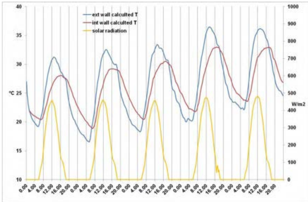
Fig.2.1.4: Simulazione dell'andamento della temperatura interna ed esterna della parete verticale ricoperta da Rhyncospermum jasminoides utilizzando i dati climatici misurati durante la prova sperimentale condotta presso il campo sperimentale di Valenzano dal 8 al 12 Agosto 2014 e andamento della radiazione solare incidente.
