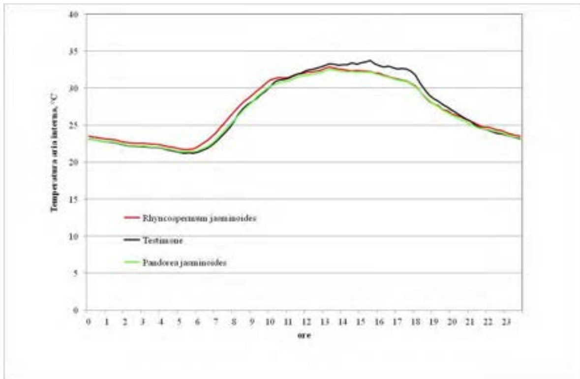
Figura 2.2.16: Andamento della temperatura dell'aria interna della struttura retrostante ogni parete nel corso delle 24 ore nel giorno 27 Agosto 2014.
