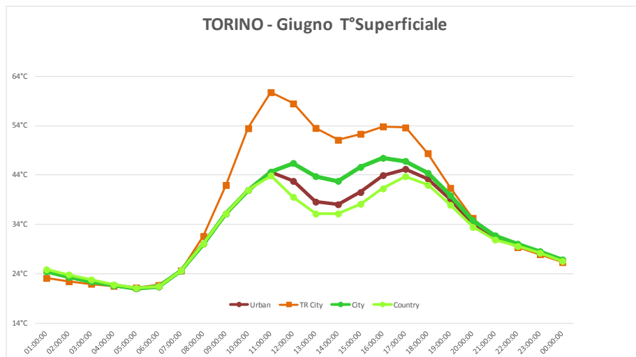
Fig. 5. Confronto fra le temperature superficiali del manto di copertura e dei Green-Roof, in relazione alla loro dislocazione. Località: Torino. Periodo:Giugno.
