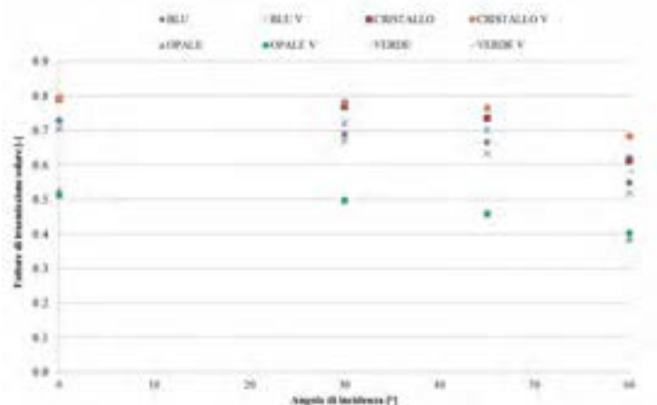
Figura 29 Fattore di trasmissione solare pannelli vuoti per diversi angoli di incidenza al variare dell’orientamento degli alveoli, orizzontali e verticali (V).
