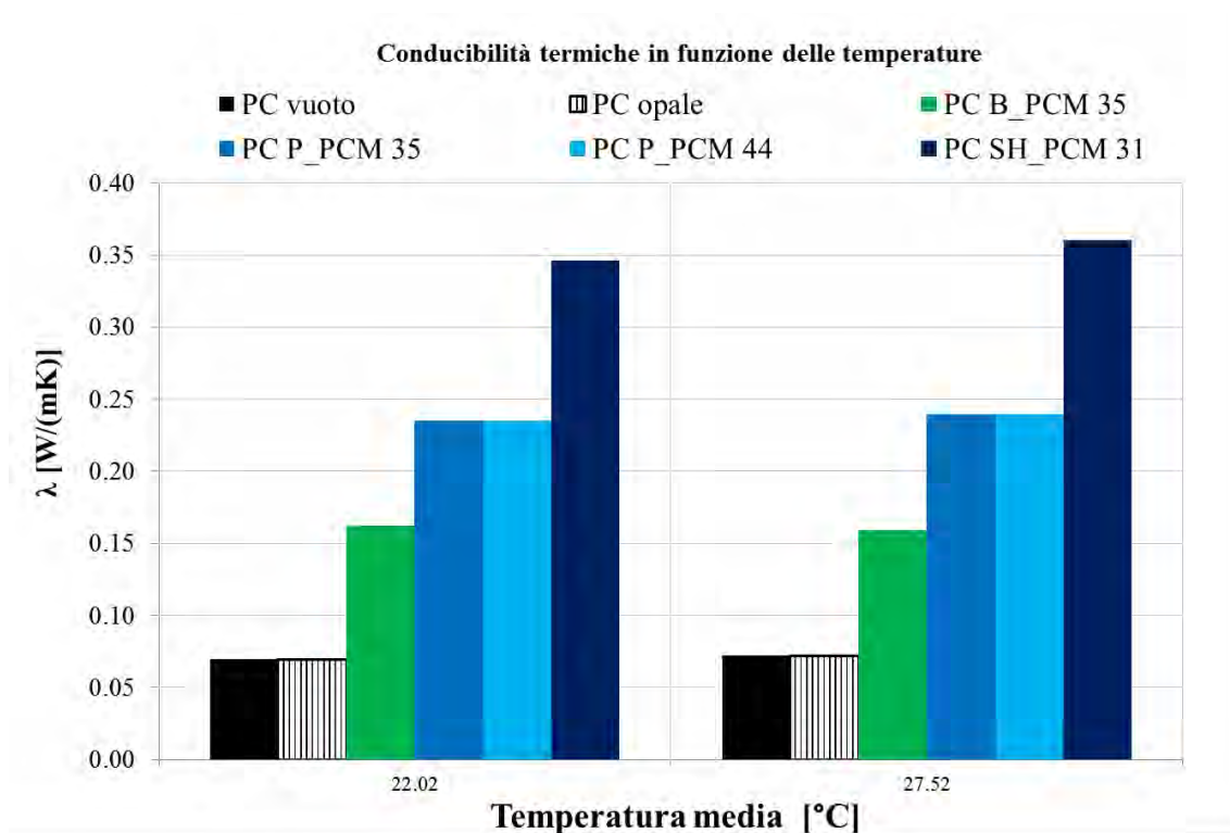
Figura 26 Quadro riassuntivo dei valori di conducibilità termica misurati.
