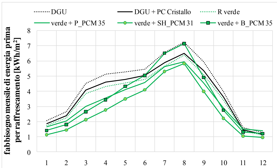
Fig.77 Fabbisogni di energia primaria per raffreddamento su base mensile
