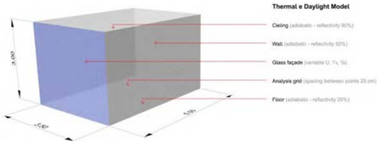
Fig. 67 Modello utilizzato per le analisi energetiche integrate.
