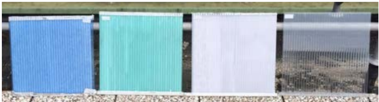
Figura 14 Configurazione 1-variante colore con PCM a base paraffina, temperatura di fusione 35°C. Da sinistra pannello Blu P_PCM 35, Verde P_PCM 35, Opale P_PCM 35 e il riferimento cristallo vuoto.
