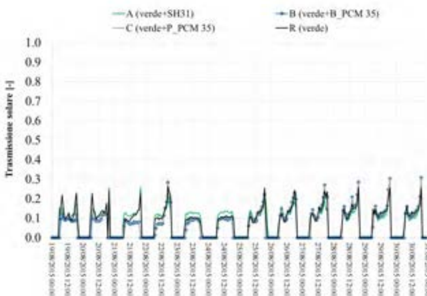
Figura 55 Andamento giornaliero, orario del coefficiente di trasmissione solare configurazione 2.
