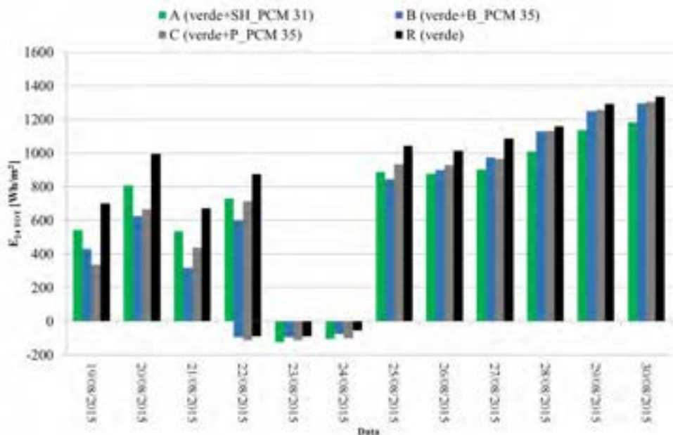
Figura 60 Configurazione 2. Energie totali giornaliere che attraversano globalmente vetrocamera + pannello schermante.
