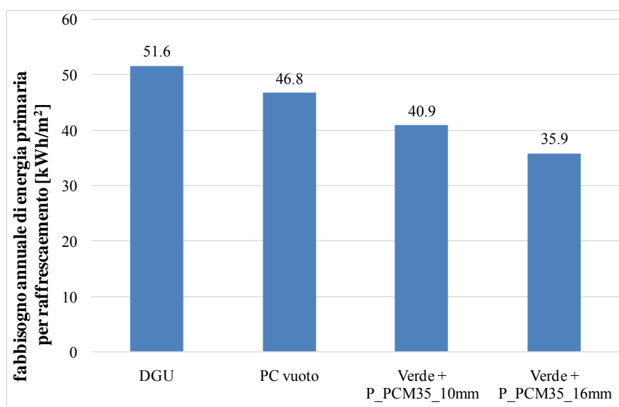
Fig.86 Fabbisogni annuale di energia primaria per raffreddamento
