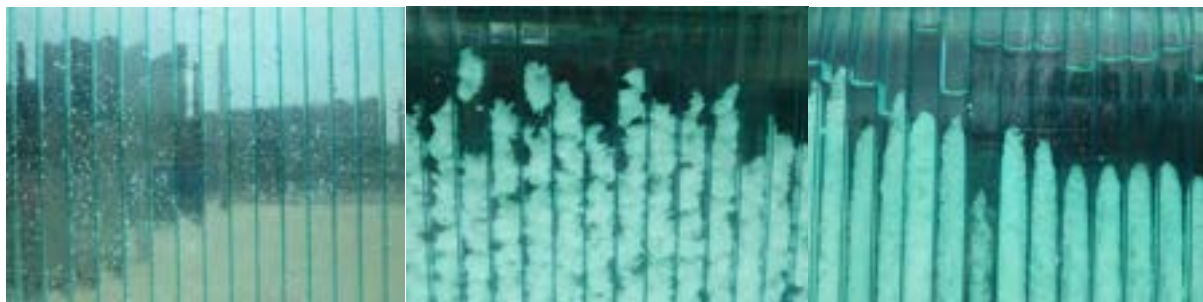
Figura 38 Configurazione 2. Analisi della transizione di fase. Policarbonato alveolare verde contenente SH_PCM 31 a). Policarbonato alveolare verde contenente B_PCM 35 b). Policarbonato alveolare verde contenente P_PCM 35 c).
