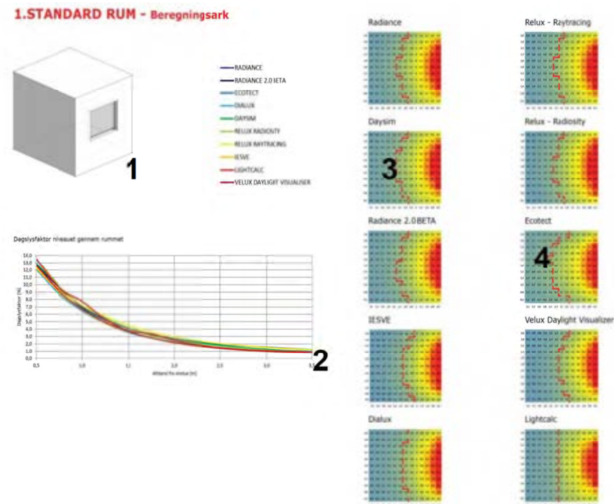
Figura 13. Calcolo di FLD con diversi software commerciali
