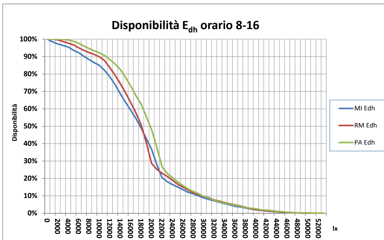
Figura 53 Curve di disponibilità E_{dh} MI-RM-PA.
