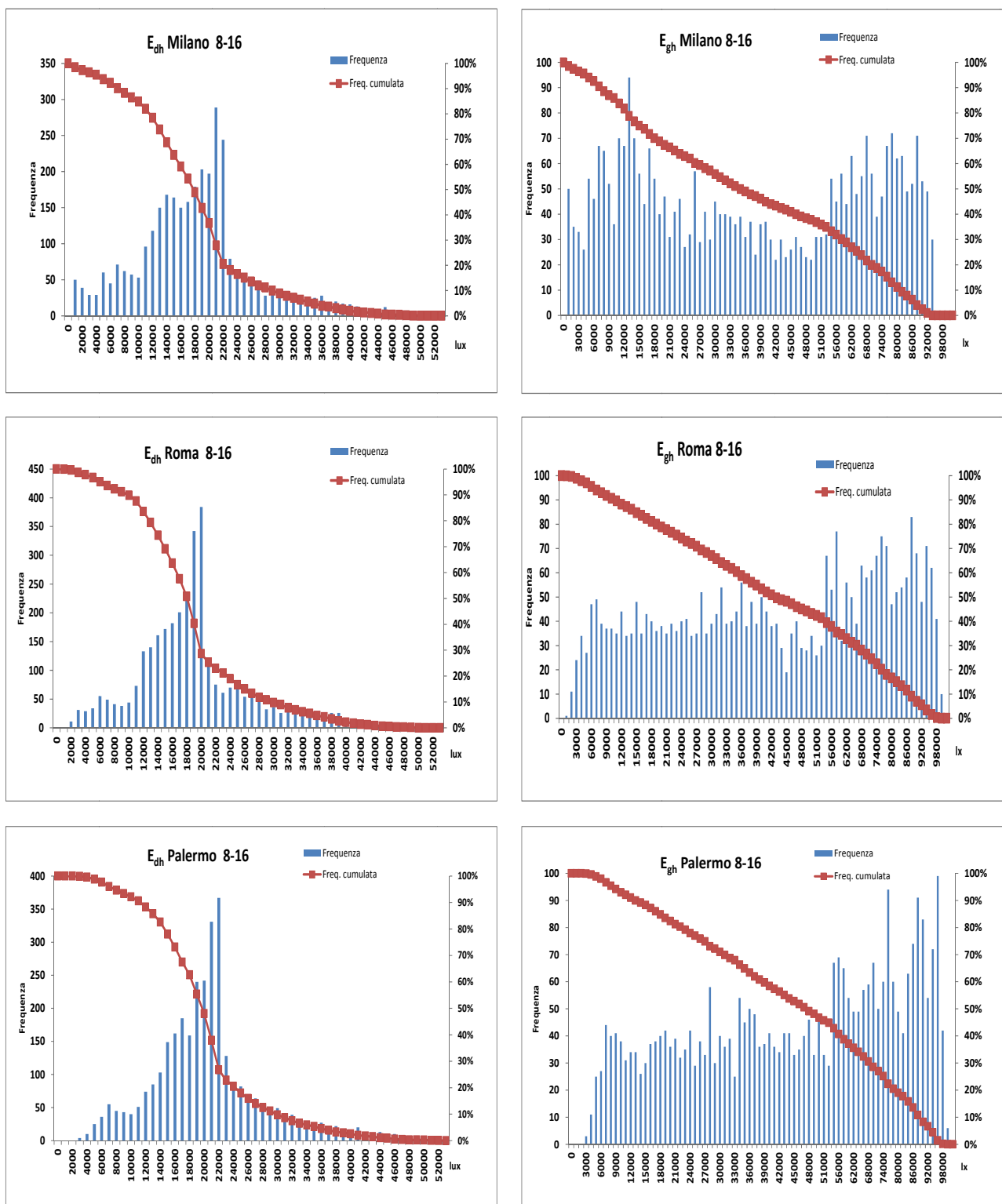
Figura 54 Distribuzioni in frequenza E_{dh} , E_{gh}
