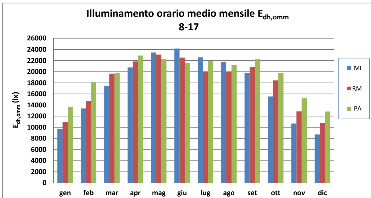
Figura 49. E_{dh,omm} tra le 8 e le 17 MI-RM-PA.
