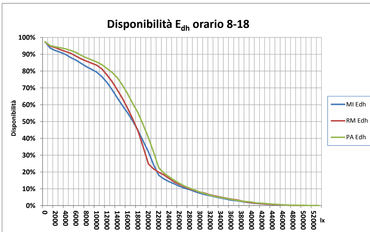
Figura 48. Curve di disponibilità E_{dh} MI-RM-PA.
