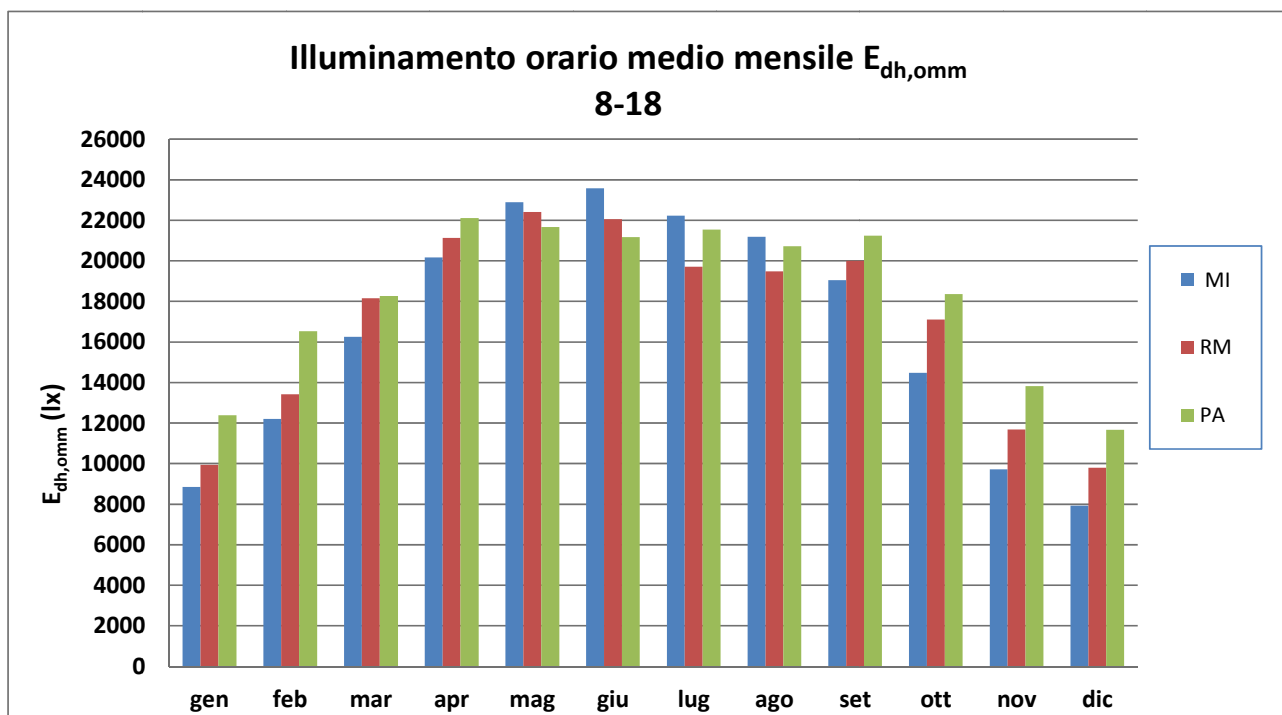
Figura 47. E_{dh,omm} tra le 8 e le 18 MI-RM-PA.
