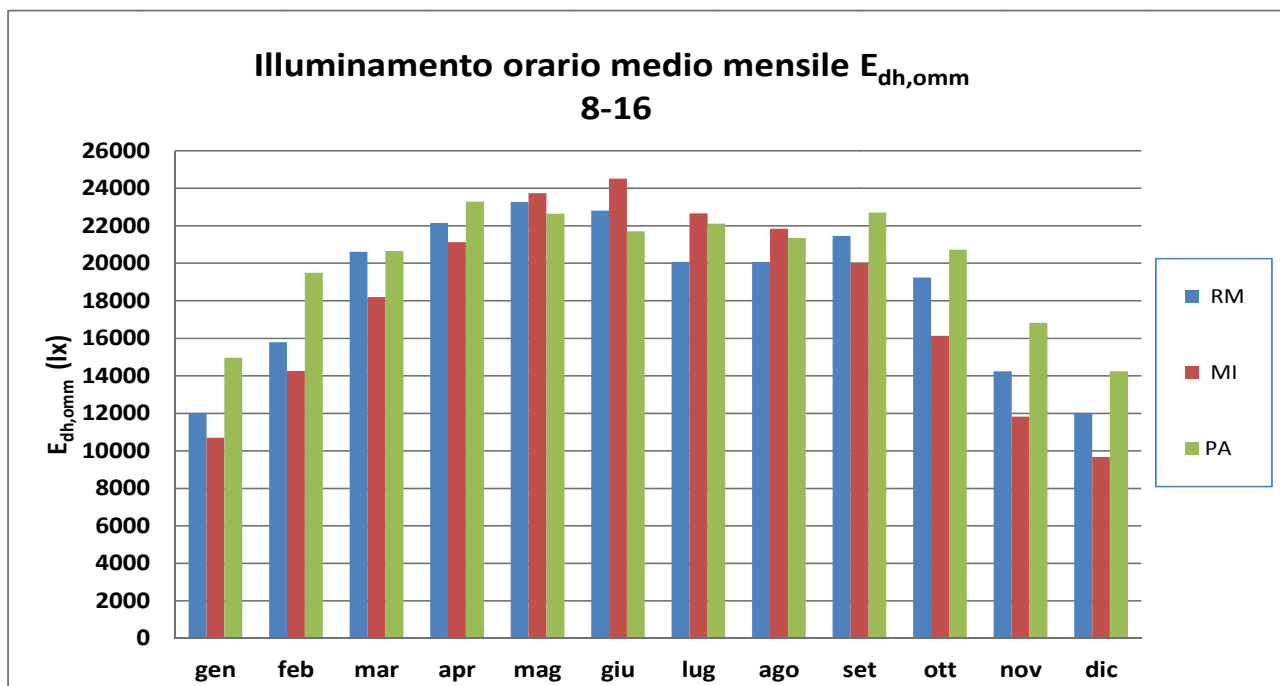
Figura 51. E_{dh,omm} tra le 8 e le 16 MI-RM-PA.
