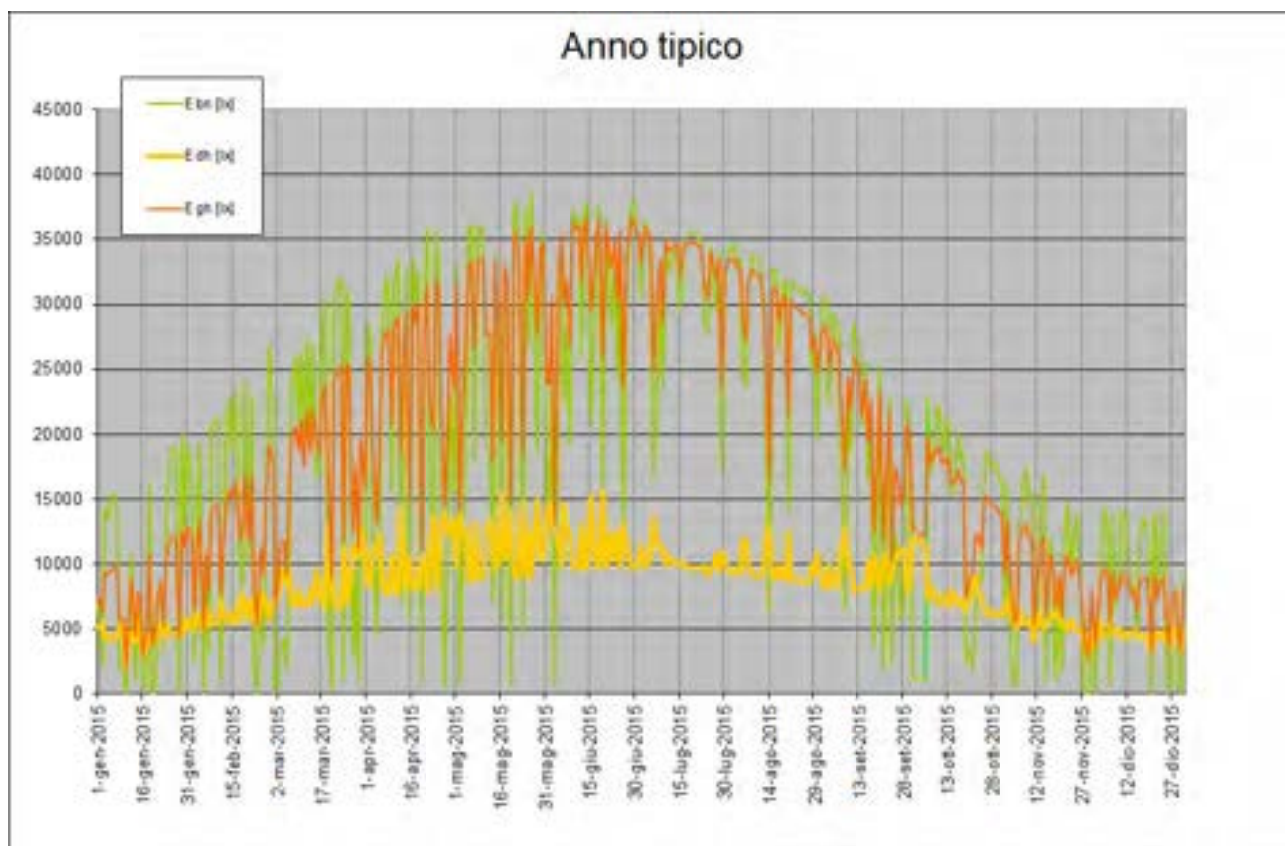
Figura 42. AMTIN: dati giornalieri — andamento annuale
