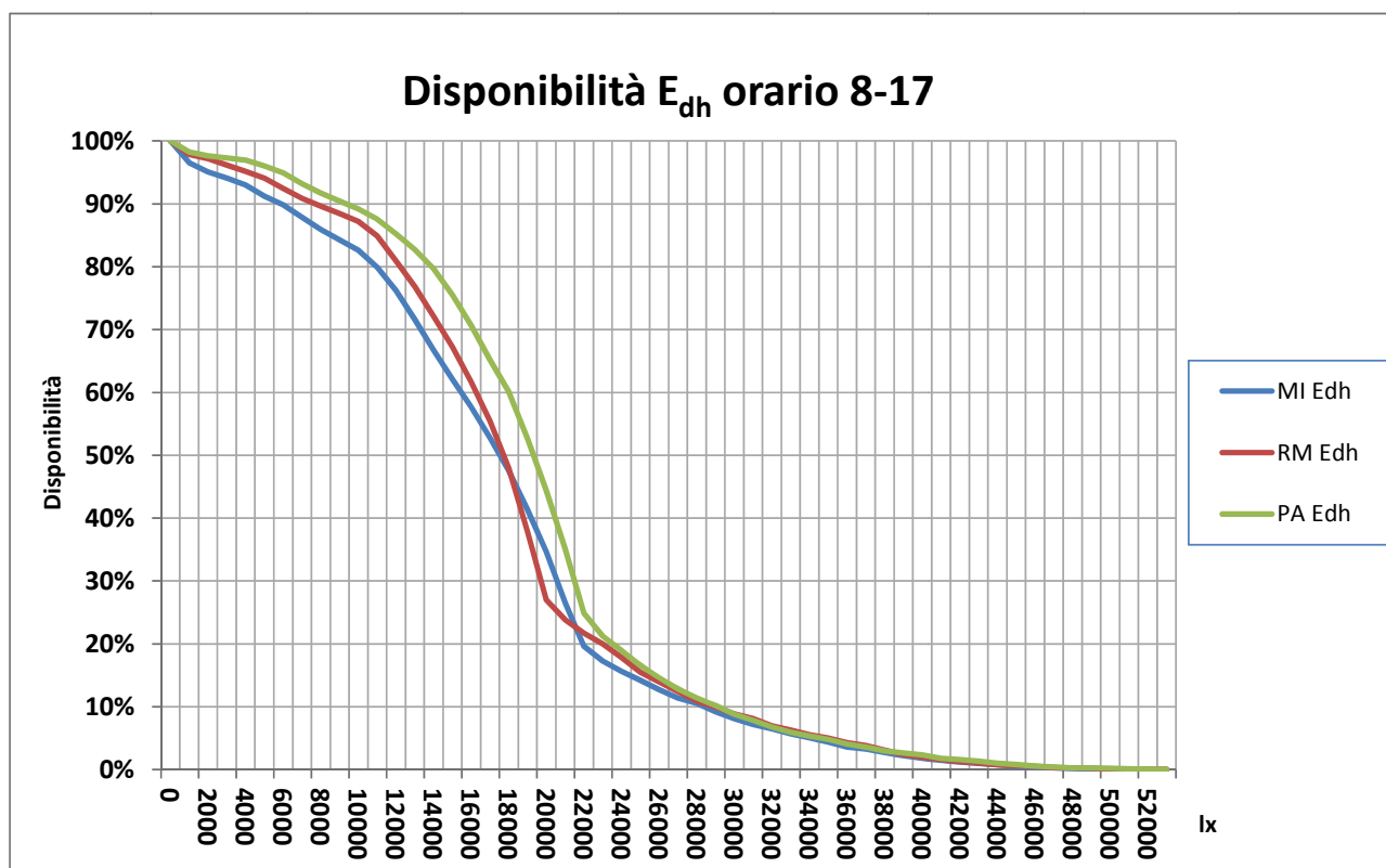
Figura 52. Curve di disponibilità E_{dh} MI-RM-PA.
