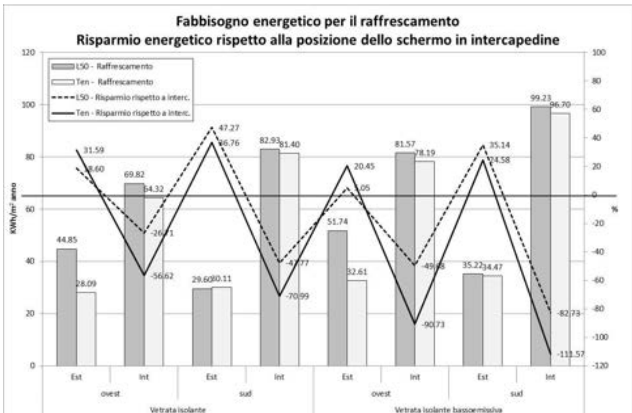
Graf.16 Comparazione di sistemi schermanti posti all'interno e all'esterno della vetrata isolante
