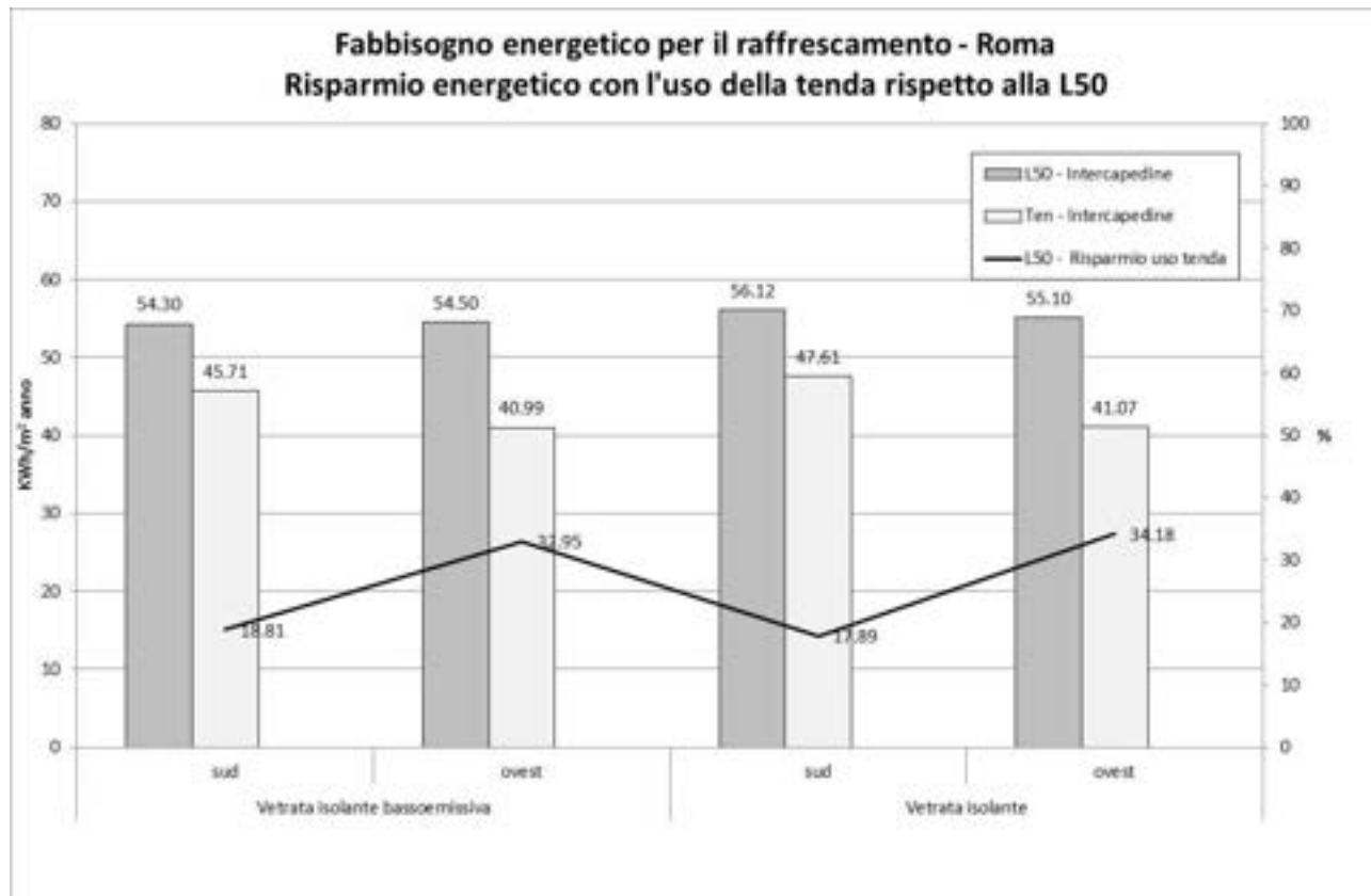
Fig.11 Comparazione di sistemi schermanti posti nell'intercapedine della vetrata isolante
