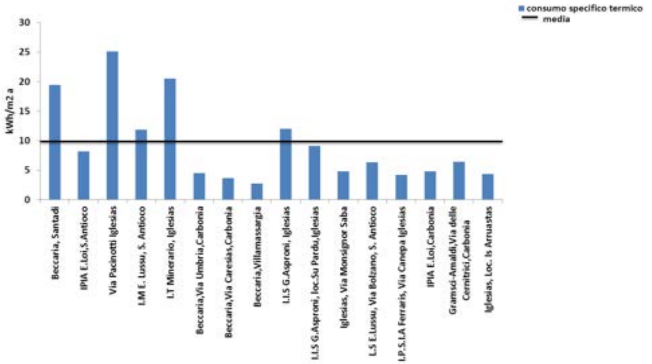
Figura 16: consumo termico specifico e medio in funzione della superficie degli edifici (scuole secondarie II°)
