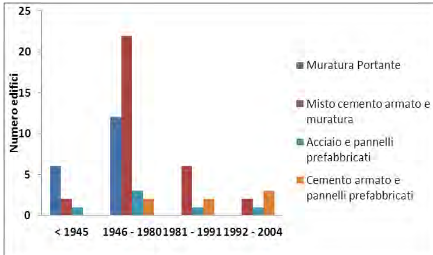
Figura 2 Anno di costruzione degli edifici scolastici per tipologia edilizia
