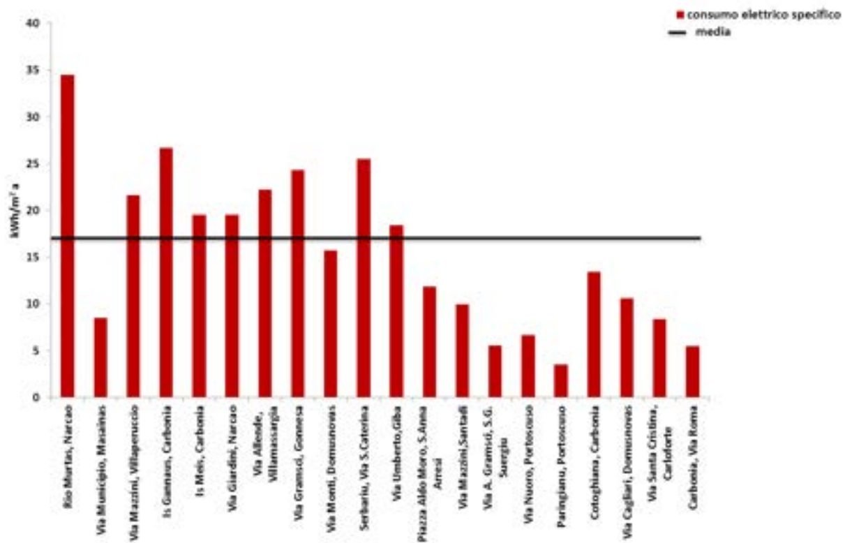
Figura 13 Consumo elettrico specifico e medio in funzione della superficie degli edifici (scuole primarie)
