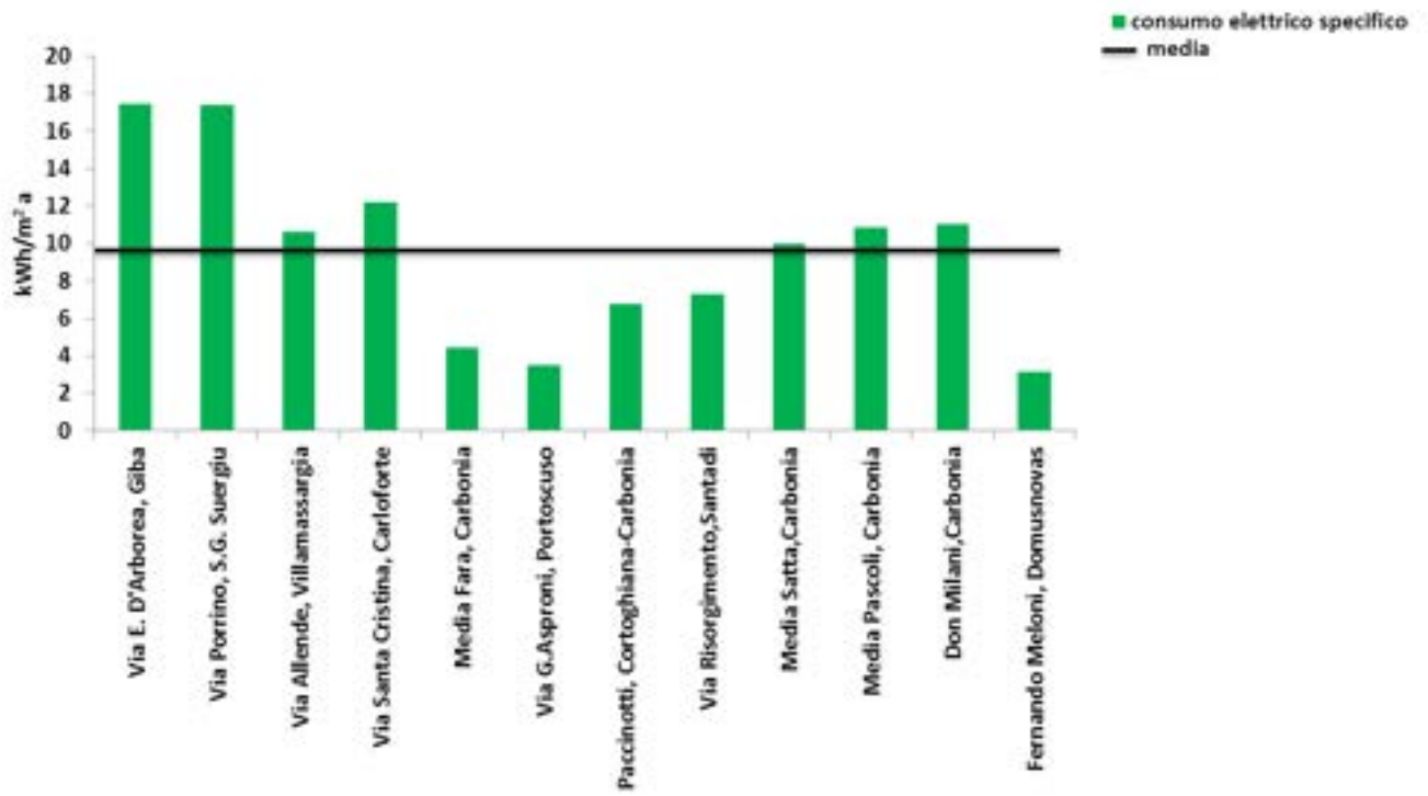
Figura 12 Consumo elettrico specifico e medio in funzione della superficie degli edifici (scuole secondarie I°)
