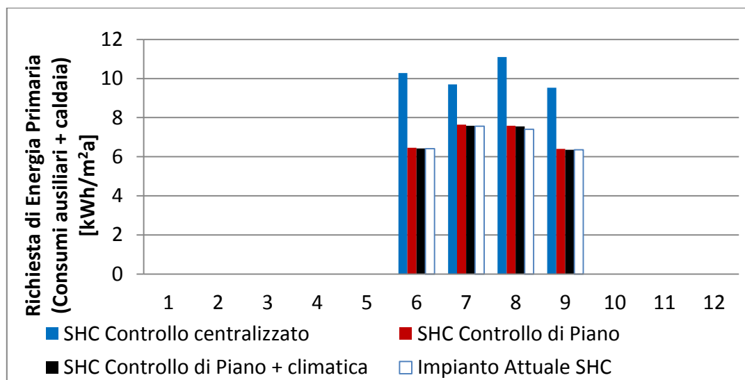
Figura 2.4.2 - Energia primaria richiesta, al variare della tipologia impiantistica, per la climatizzazione estiva di una superficie unitaria dell'edificio
