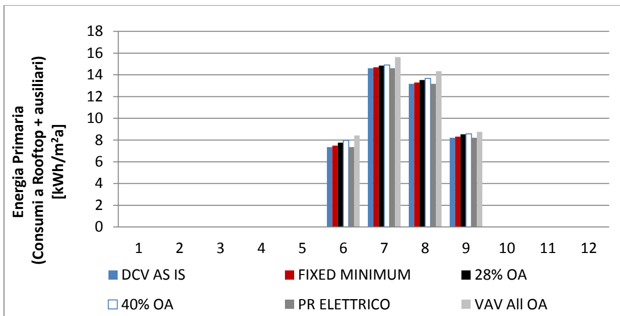
Figura 2.1.17 - Energia primaria richiesta, al variare della tipologia impiantistica, per la climatizzazione estiva di una superficie unitaria dell'edificio
