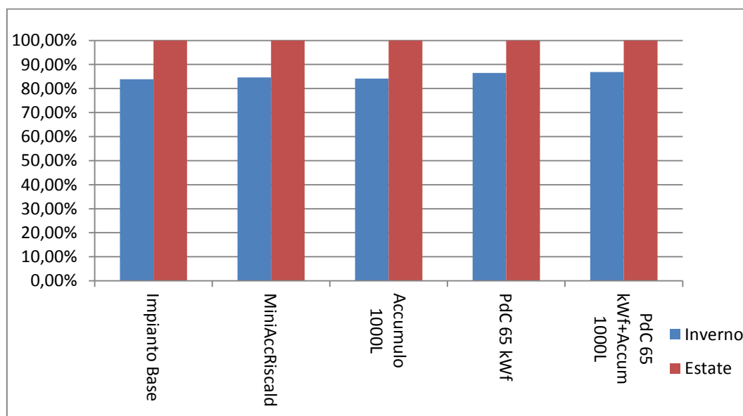
Figura 2.3.12 - Indicatori di Prestazione di temperatura, relativi alle intere stagioni di riscaldamento e raffreddamento, al variare della tipologia impiantistica
