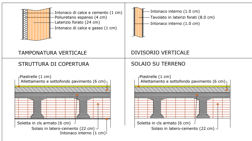
Figura 2.2.3 - Termofisica delle Strutture
