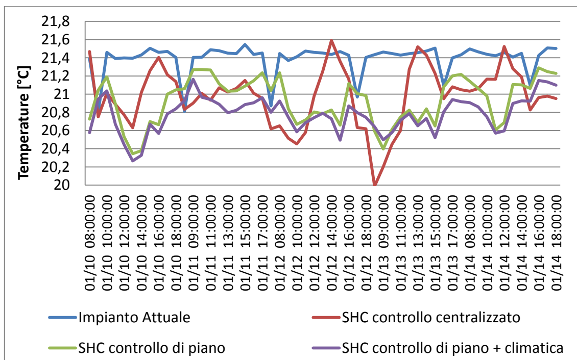
Figura 2.4.5 - Temperature invernali mediate (aula 1, aula 2, sala riunioni, area break) al variare della tipologia Impiantistica (periodo di riferimento: 10-14 Gennaio)
