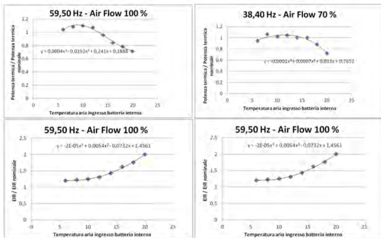
Figura 2.1.11 - Costruzione, per regressione, delle curve cubiche per la modellazione del funzionamento della PdC a CO 2 in EnergyPlus in inverno
