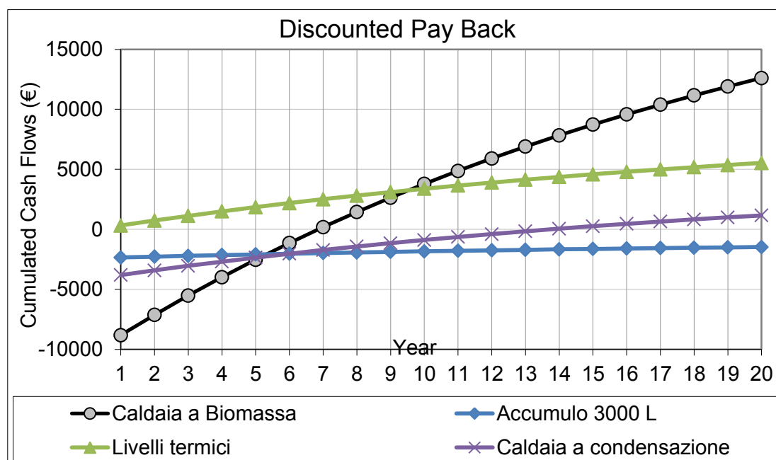
Figura 2.2.17 - Andamento dei flussi di cassa e valore del DPB per le differenti soluzioni impiantistiche alternative proposte
