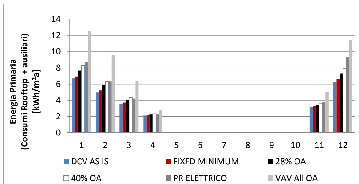
Figura 2.1.16 - Energia primaria richiesta, al variare della tipologia impiantistica, per la climatizzazione invernale di una superficie unitaria dell'edificio
