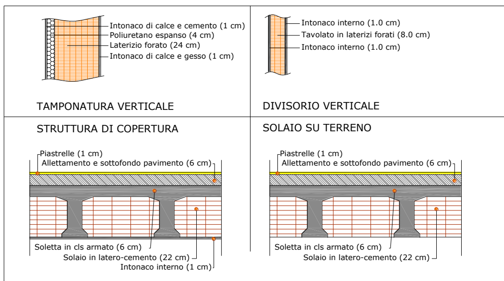
Figura 2.3.2 - Stratigrafia e termo-fisica delle strutture di confine
