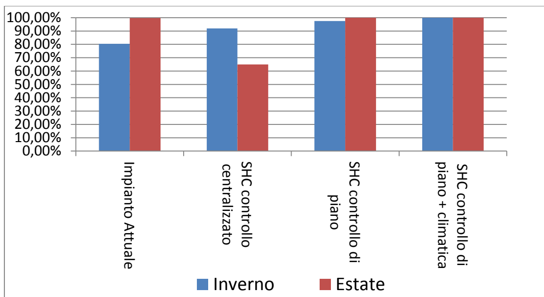
Figura 23 - Indicatori di Prestazione di temperatura, relativi alle intere stagioni di riscaldamento e raffreddamento, al variare della tipologia impiantistica
