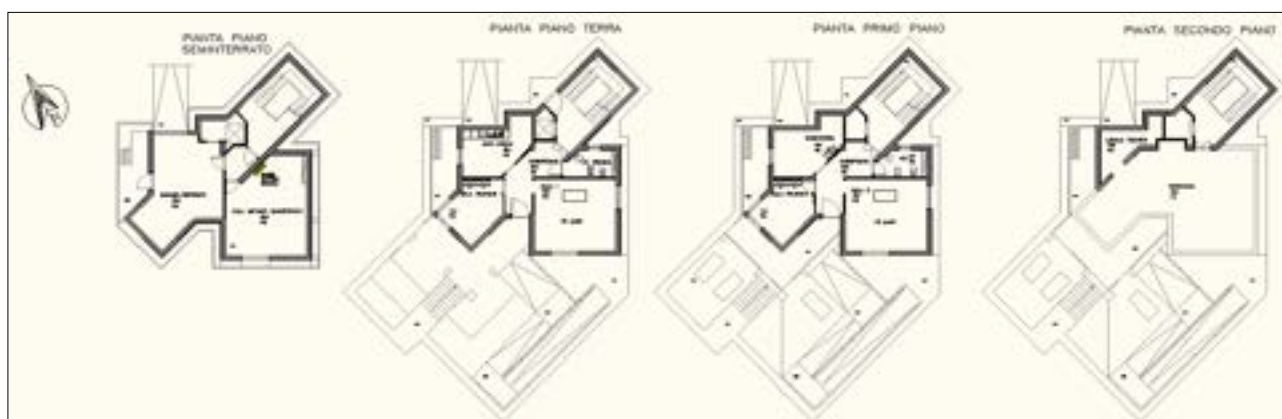
Figura 2.2.2 - Planimetrie in CAD per i diversi piani costituenti l'edificio
