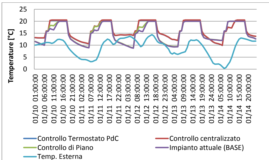
Figura 2.4.12 - Temperature invernali mediate (aula 1, aula 2, sala riunioni, area break) al variare della tipologia impiantistica (periodo di riferimento: 10-14 Gennaio)
