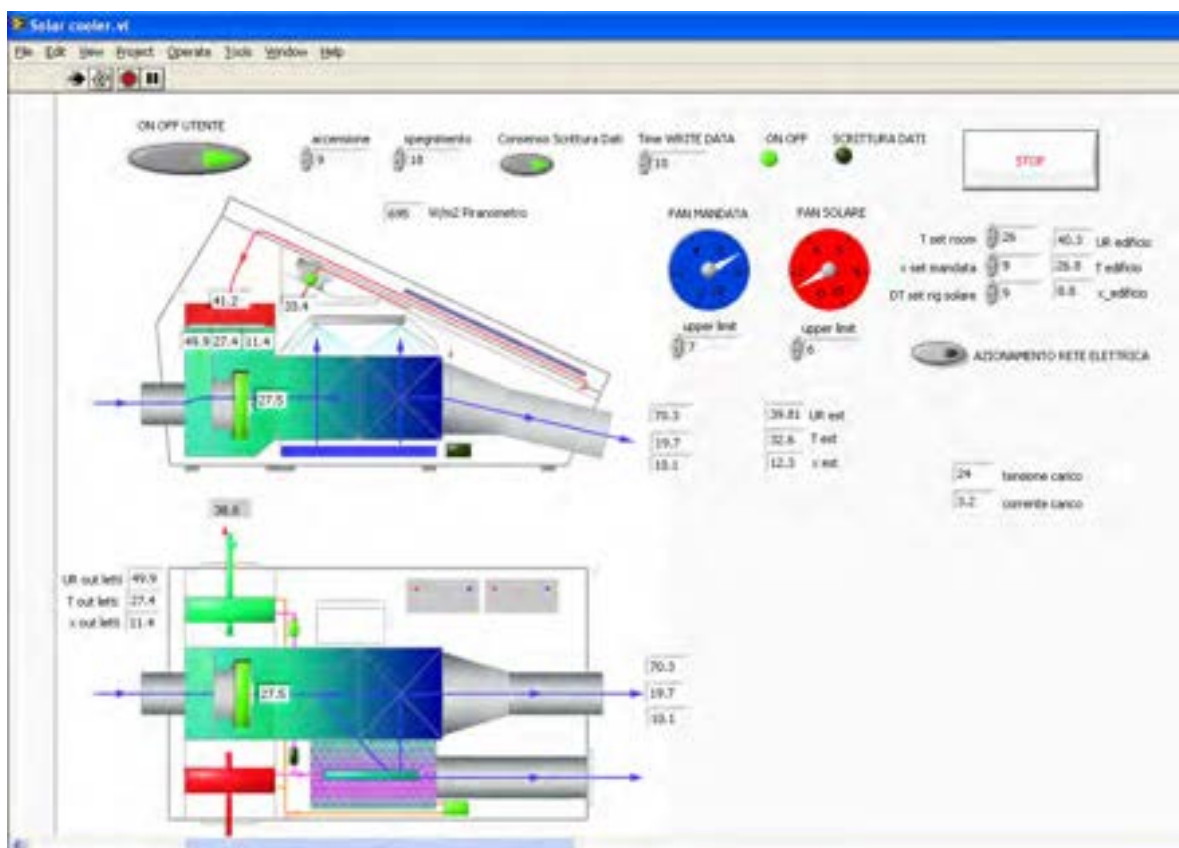
Figura 20: Valori di misura visualizzati sul pannello di controllo in Labview durante il funzionamento del sistema
