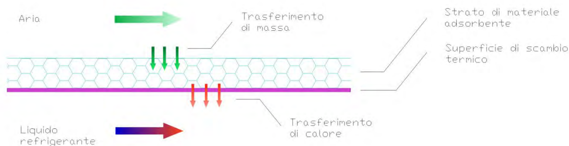
Figura 10: Schema trasferimento di calore e massa all'interno di uno scambiatore di calore con materiale adsorbente
