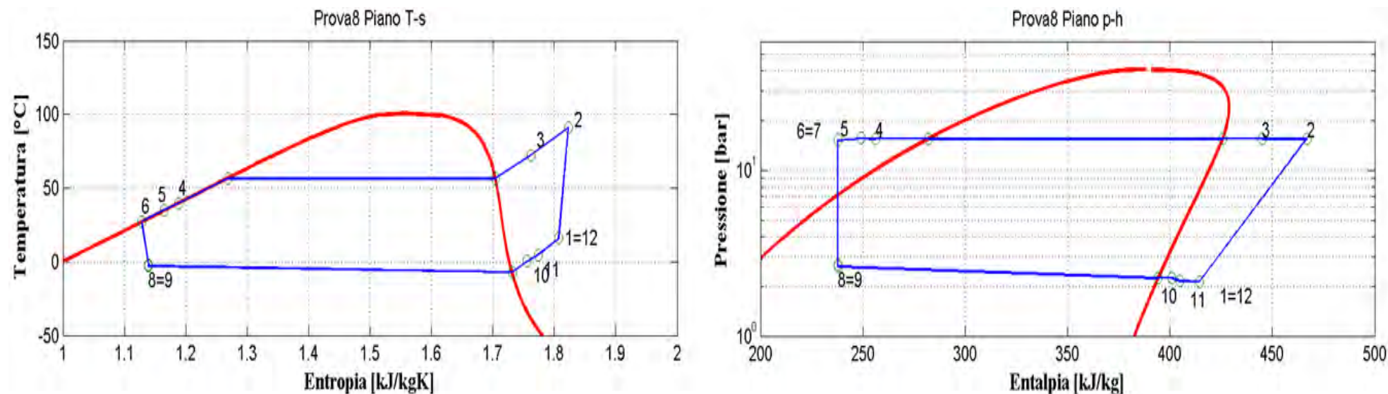
Figura 2.10: Piani T-s e p-h per la prova effettuata nelle condizioni 8 in modalità pompa di calore per il prototipo operante con R134a.
