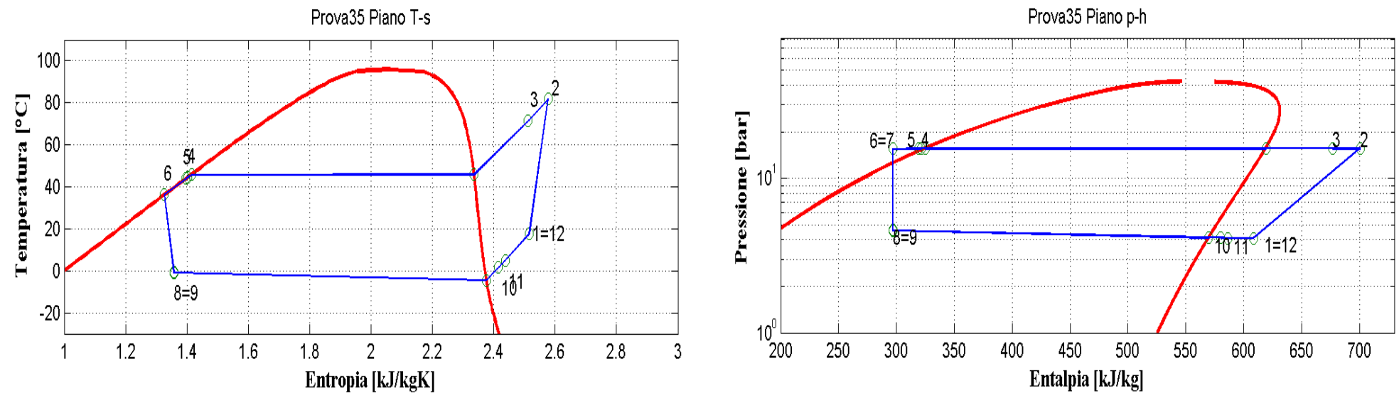
Figura 9.36: Piani T-s e p-h per la prova effettuata nelle condizioni 35 in modalità pompa di calore per il prototipo operante con R290.
