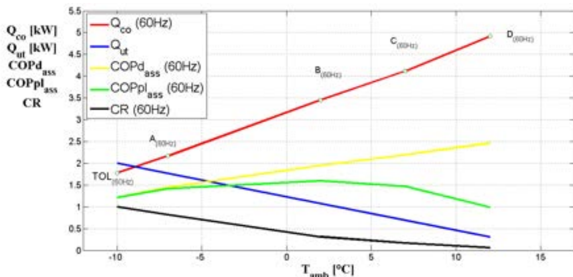
Figura 8.6: Andamento in funzione della temperatura esterna della potenza termica fornita dalla pompa di calore a R134a con compressore a 60 Hz (in rosso), quella richiesta dall'utenza (in blu), del COP dichiarato della pompa di calore (in giallo), del COP a carico parziale (in verde) e del fattore CR (in nero).
