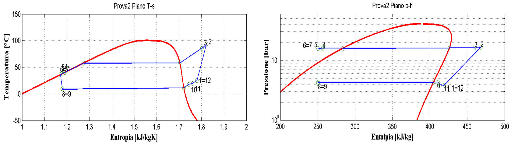
Figura 2.44: Piani T-s e p-h per la prova effettuata nelle condizioni 2 in modalità macchina frigorifera per il prototipo elaborante R134a.
