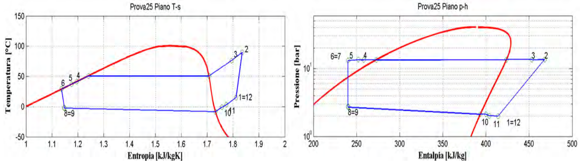
Figura 2.27: Piani T-s e p-h per la prova effettuata nelle condizioni 25 in modalità pompa di calore per il prototipo operante con R134a.
