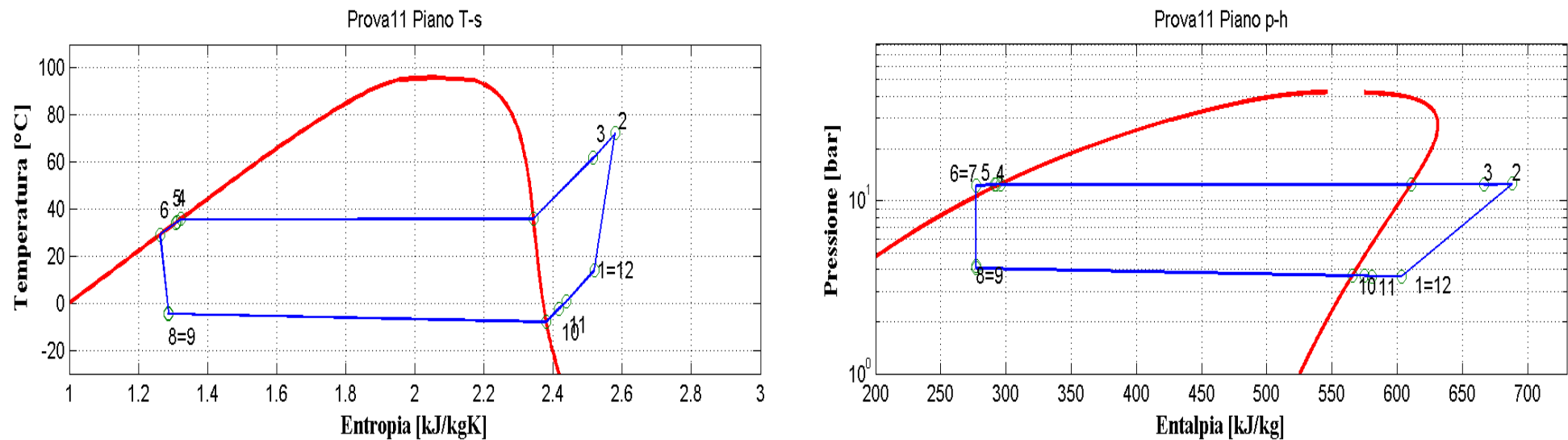
Figura 9.12: Piani T-s e p-h per la prova effettuata nelle condizioni 11 in modalità pompa di calore per il prototipo operante con R290.
