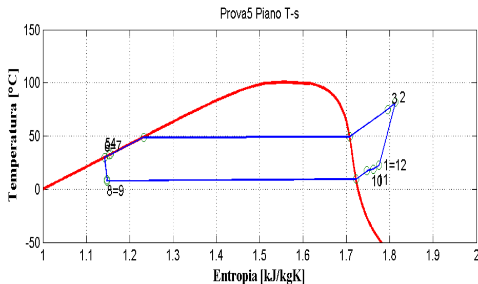
Figura 2.47: Piani T-s e p-h per la prova effettuata nelle condizioni 5 in modalità macchina frigorifera per il prototipo elaborante R134a.
