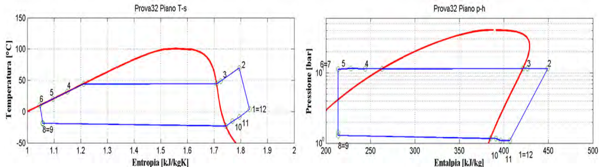
Figura 2.34: Piani T-s e p-h per la prova effettuata nelle condizioni 32 in modalità pompa di calore per il prototipo operante con R134a.
