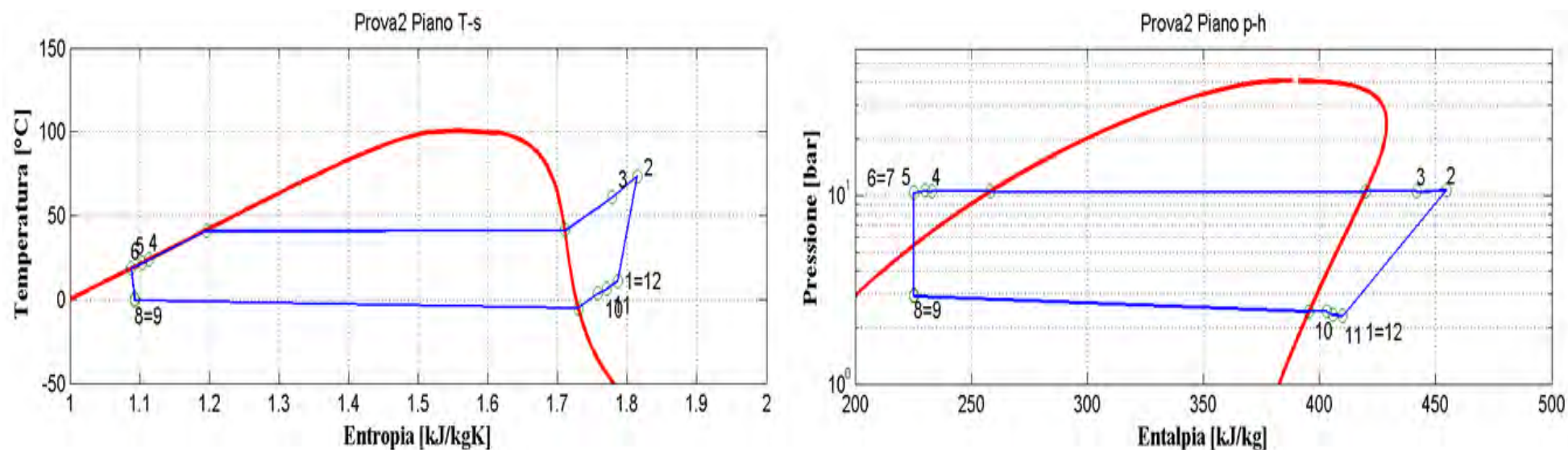
Figura 2.4: Piani T-s e p-h per la prova effettuata nelle condizioni 2 in modalità pompa di calore per il prototipo operante con R134a.
