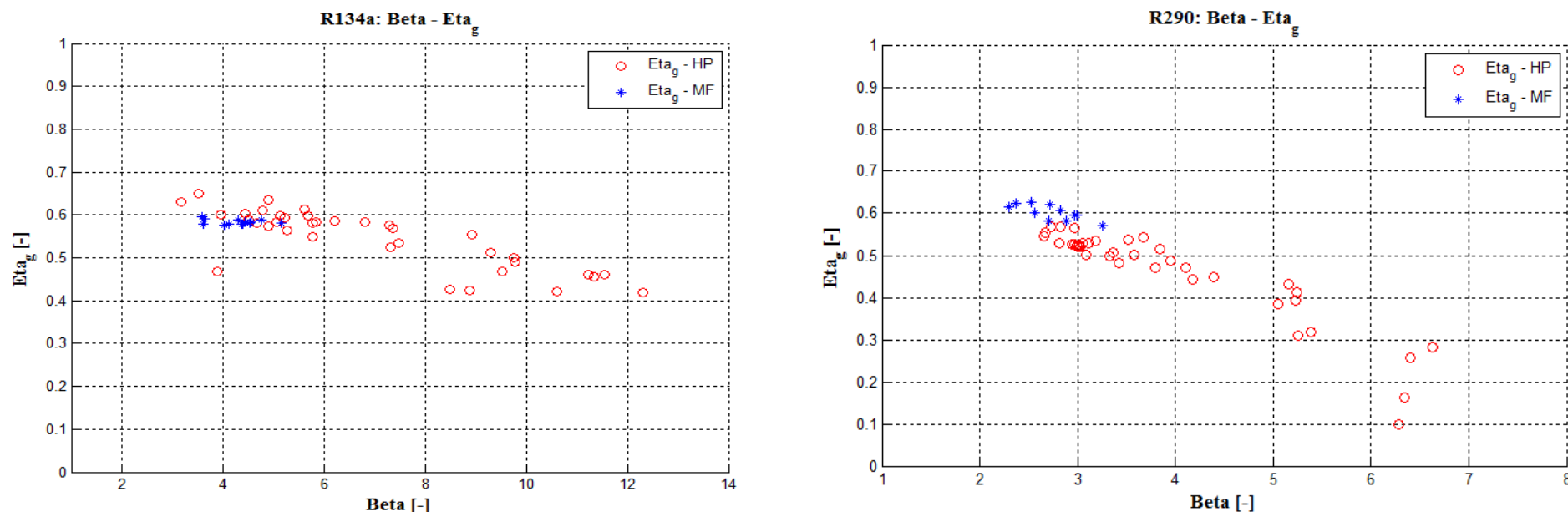
Figura 17.4 :Andamento del rendimento globale del compressore ( \eta_g ) in funzione del rapporto di compressione (Beta) per entrambi i prototipi nelle modalità di funzionamento pompa di calore (rosso) e macchina frigorifera (blu).
