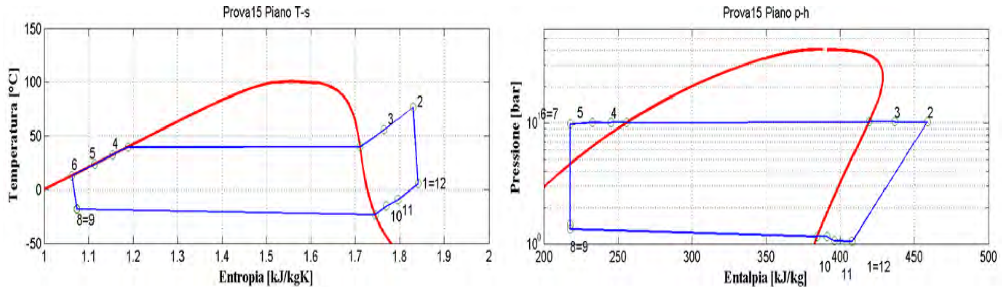
Figura 2.17: Piani T-s e p-h per la prova effettuata nelle condizioni 15 in modalità pompa di calore per il prototipo operante con R134a.
