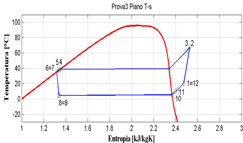
Figura 9.44: Piani T-s e p-h per la prova effettuata nelle condizioni 3 in modalità macchina frigorifera per il prototipo a propano (R290).
