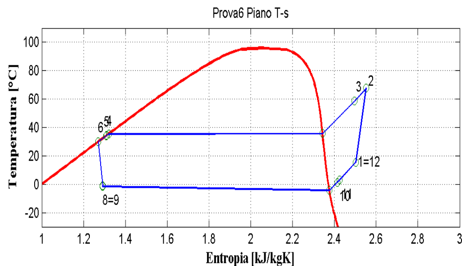
Figura 9.7: Piani T-s e p-h per la prova effettuata nelle condizioni 6 in modalità pompa di calore per il prototipo operante con R290.
