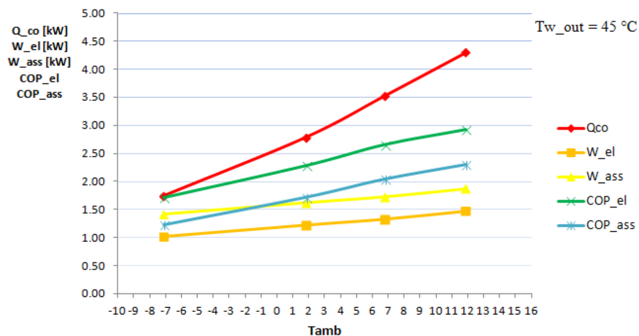
Figura 4.1: Andamento della \dot{Q}_{co} , W_{el} , W_{ass} , COP_{el} , COP_{ass} al variare della temperatura ambiente per una fissata temperatura dell'acqua in uscita dallo scambiatore per il prototipo operante con R134a in modalità pompa di calore.
