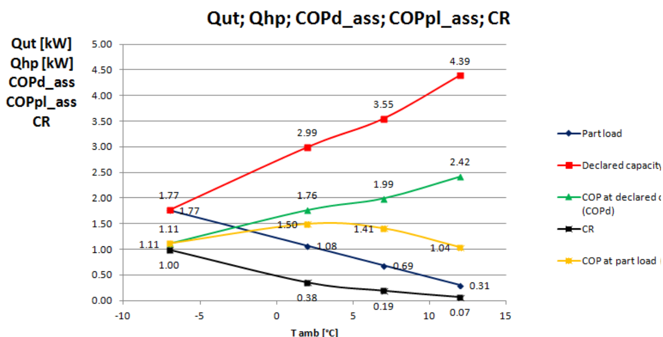
Figura 11.3: Andamento in funzione della temperatura esterna della potenza termica fornita dalla pompa di calore a propano (in rosso), della potenza richiesta dall'utenza (in blu), del rapporto di capacità CR (in nero), del COP dichiarato della pompa di calore (in verde) e del COP a carico parziale (in giallo) questi ultimi valutati considerando come spesa energetica la potenza elettrica assorbita dall'intero impianto.
