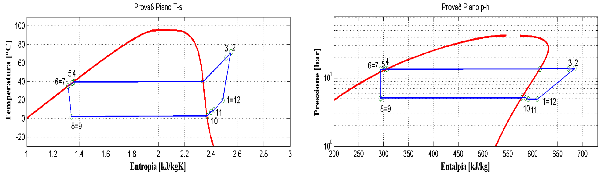
Figura 9.49: Piani T-s e p-h per la prova effettuata nelle condizioni 8 in modalità macchina frigorifera per il prototipo a propano (R290).
