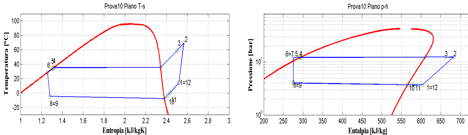
Figura 9.11: Piani T-s e p-h per la prova effettuata nelle condizioni 10 in modalità pompa di calore per il prototipo operante con R290.
