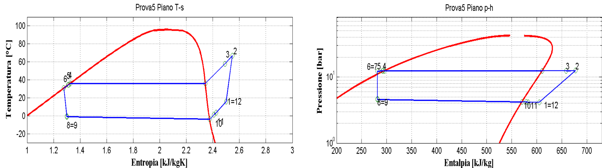
Figura 9.6: Piani T-s e p-h per la prova effettuata nelle condizioni 5 in modalità pompa di calore per il prototipo operante con R290.
