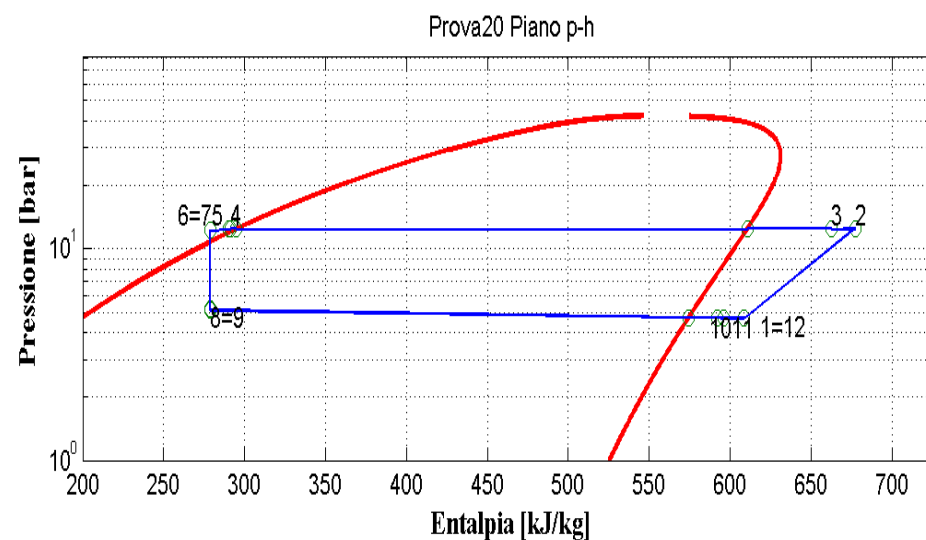
Figura 9.21: Piani T-s e p-h per la prova effettuata nelle condizioni 20 in modalità pompa di calore per il prototipo operante con R290.
