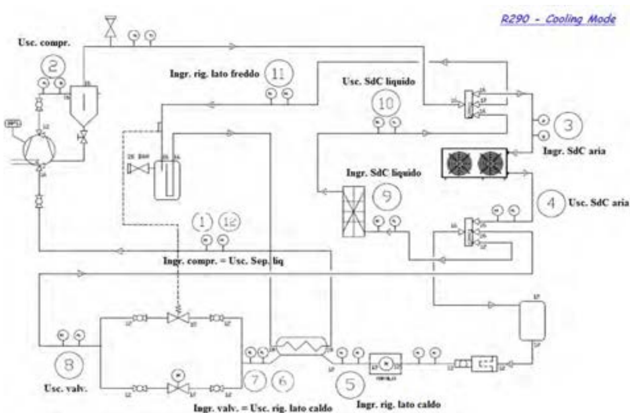
Figura 9.41: Schema d'impianto per il prototipo operante con R290 in modalità macchina frigo.
