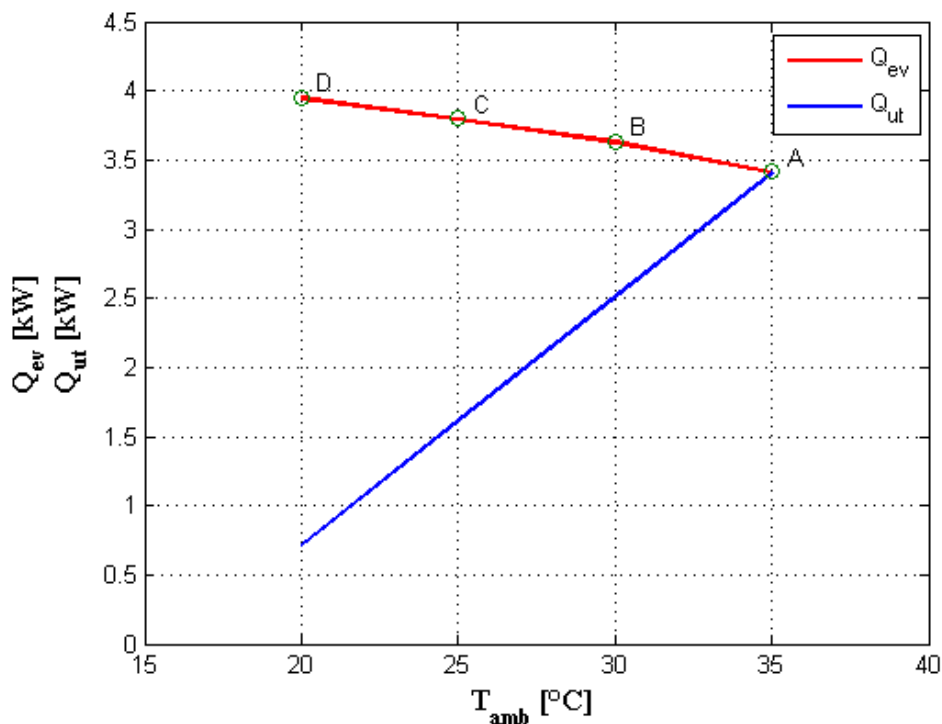
Figura 6.2.: Andamento in funzione della temperatura esterna della potenza frigo fornita dalla macchina frigorifera elaborante R134a (in rosso) e quella richiesta dall'utenza (in blu).
