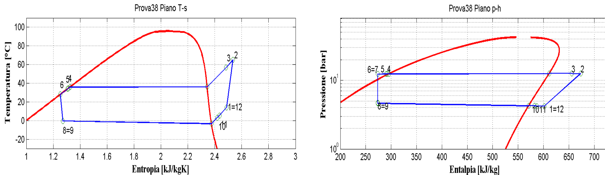
Figura 9.39: Piani T-s e p-h per la prova effettuata nelle condizioni 38 in modalità pompa di calore per il prototipo operante con R290.
