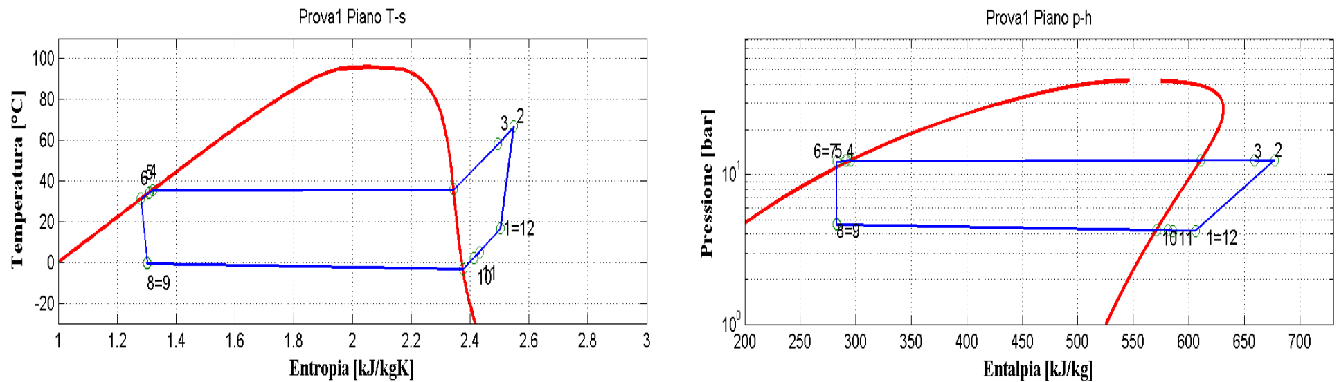
Figura 9.2: Piani T-s e p-h per la prova effettuata nelle condizioni 1 in modalità pompa di calore per il prototipo operante con R290.
