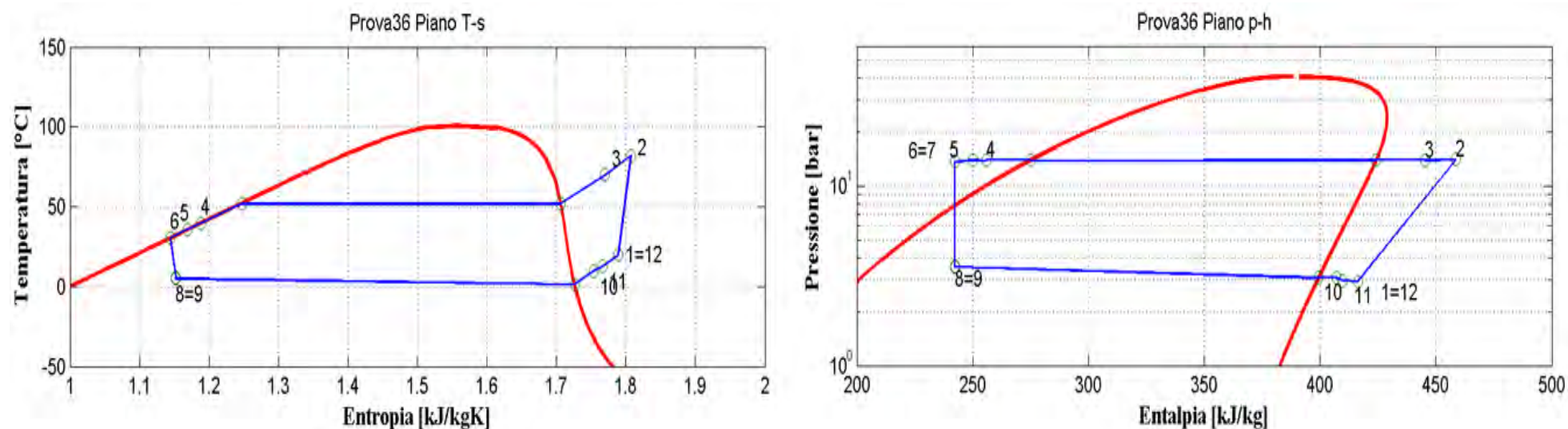
Figura 2.38: Piani T-s e p-h per la prova effettuata nelle condizioni 36 in modalità pompa di calore per il prototipo operante con R134a.
