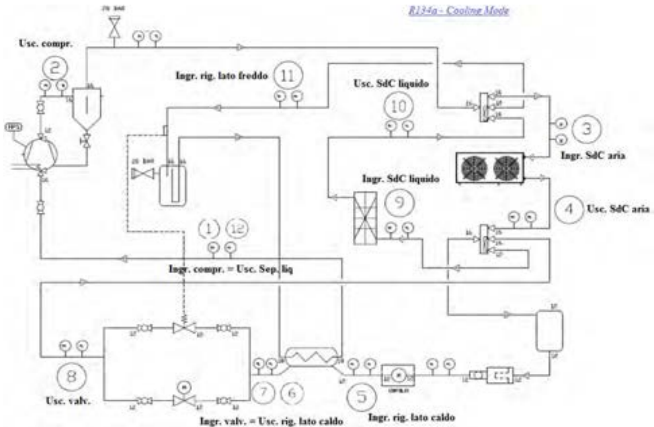
Figura 2.42: Schema d'impianto per il prototipo operante con R134a in modalità macchina frigo.
