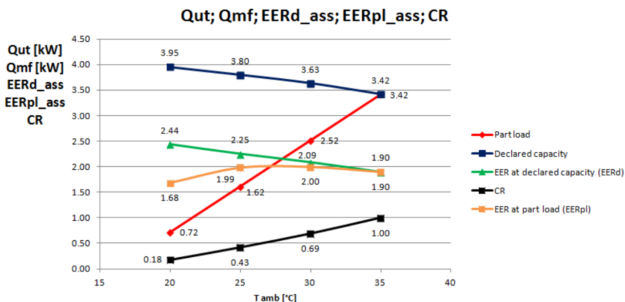
Figura 6.3: Andamento in funzione della temperatura esterna della potenza frigorifera fornita dalla macchina frigo a R134a (in blu), della potenza richiesta dall'utenza (in rosso), del rapporto di capacità CR (in nero), dell'EER dichiarato della macchina frigo (in verde) e dell'EER a carico parziale (in arancione), questi ultimi valutati considerando come spesa energetica la potenza elettrica assorbita dall'intero impianto
