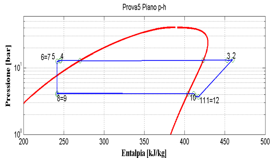
Figura 2.47: Piani T-s e p-h per la prova effettuata nelle condizioni 5 in modalità macchina frigorifera per il prototipo elaborante R134a.
