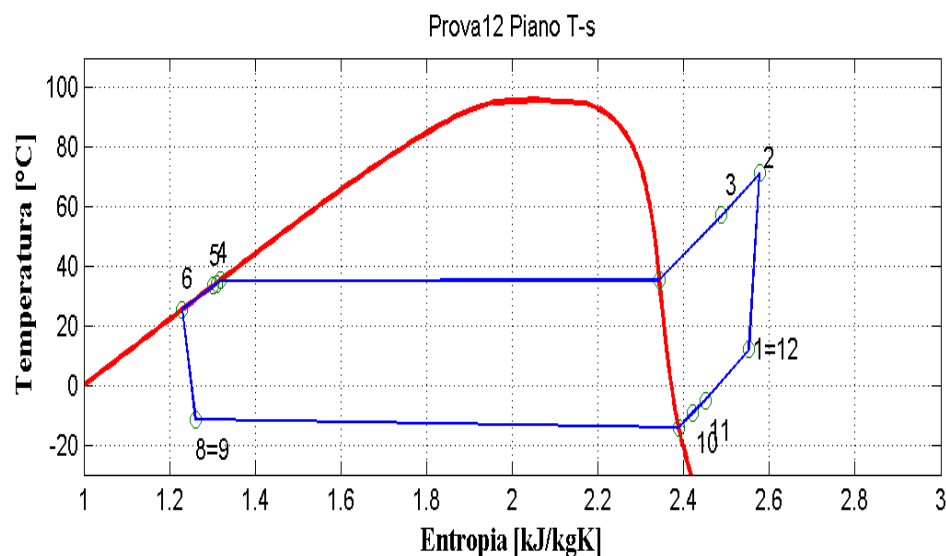
Figura 9.13: Piani T-s e p-h per la prova effettuata nelle condizioni 12 in modalità pompa di calore per il prototipo operante con R290.
