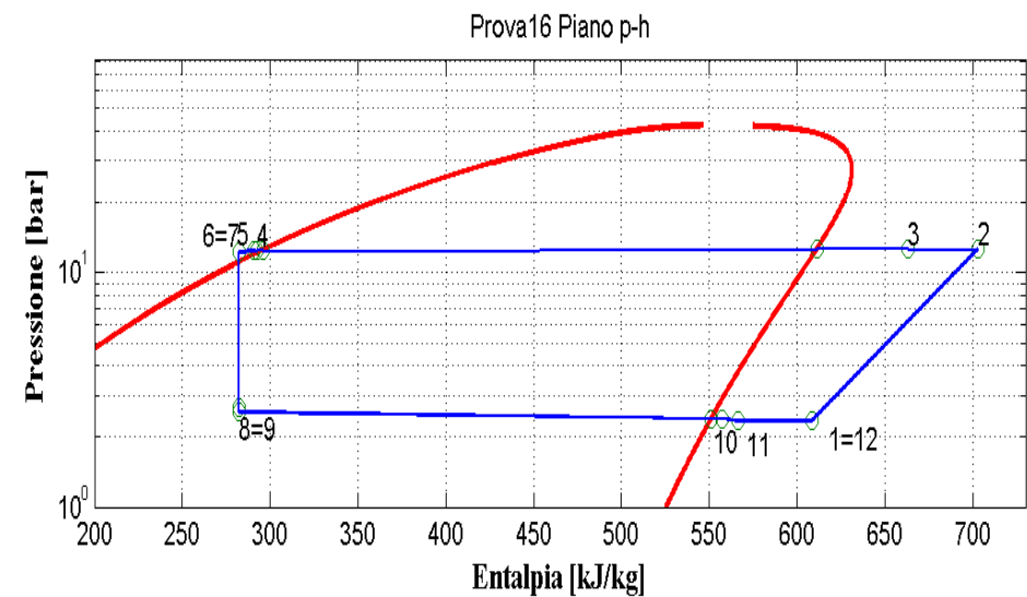
Figura 9.17: Piani T-s e p-h per la prova effettuata nelle condizioni 16 in modalità pompa di calore per il prototipo operante con R290.
