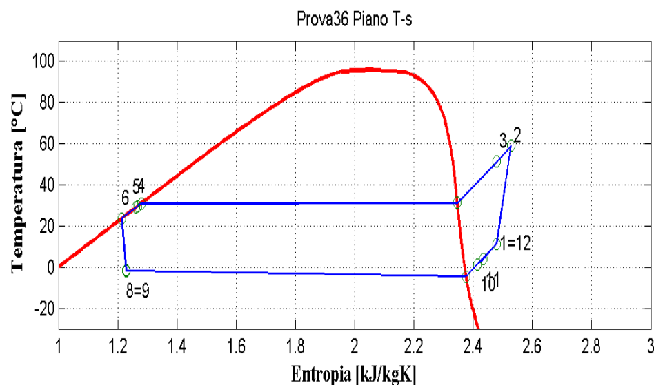
Figura 9.37: Piani T-s e p-h per la prova effettuata nelle condizioni 36 in modalità pompa di calore per il prototipo operante con R290.
