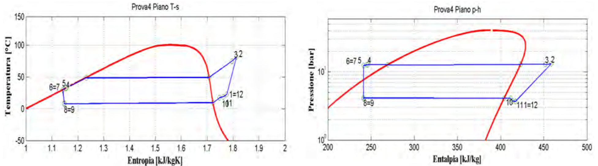
Figura 2.46: Piani T-s e p-h per la prova effettuata nelle condizioni 4 in modalità macchina frigorifera per il prototipo elaborante R134a.
