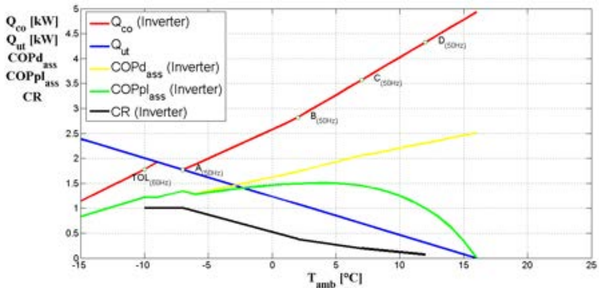
Figura 8.9: Andamento in funzione della temperatura esterna della potenza termica fornita dalla pompa di calore elaborante R134a con compressore funzionante con inverter tra 60 e 50 Hz (in rosso), quella richiesta dall'utenza (in blu), del COP dichiarato della pompa di calore (in giallo), del COP a carico parziale (in verde) e del fattore CR (in nero)
