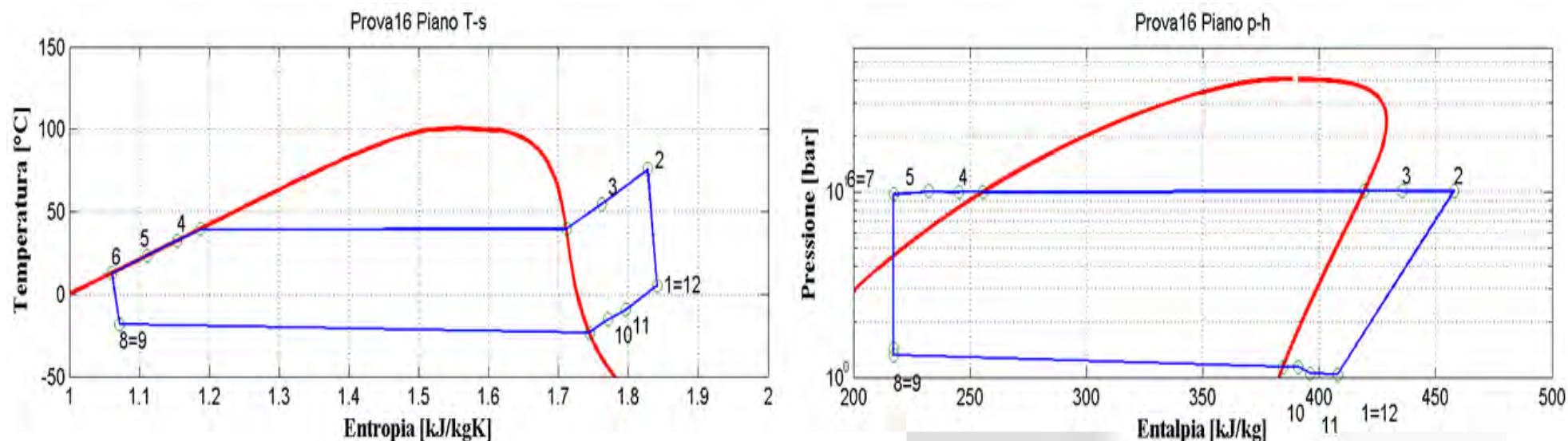
Figura 2.18: Piani T-s e p-h per la prova effettuata nelle condizioni 16 in modalità pompa di calore per il prototipo operante con R134a.
