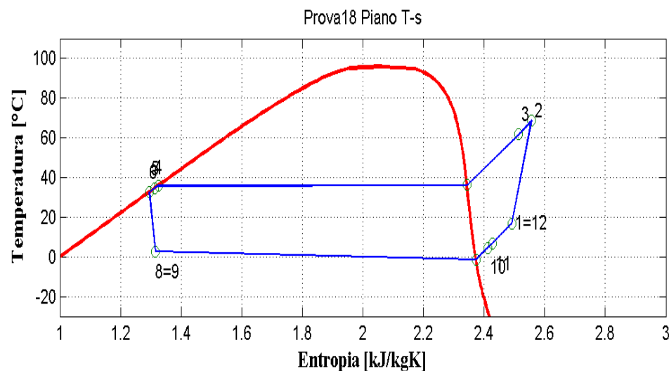
Figura 9.19: Piani T-s e p-h per la prova effettuata nelle condizioni 18 in modalità pompa di calore per il prototipo operante con R290.
