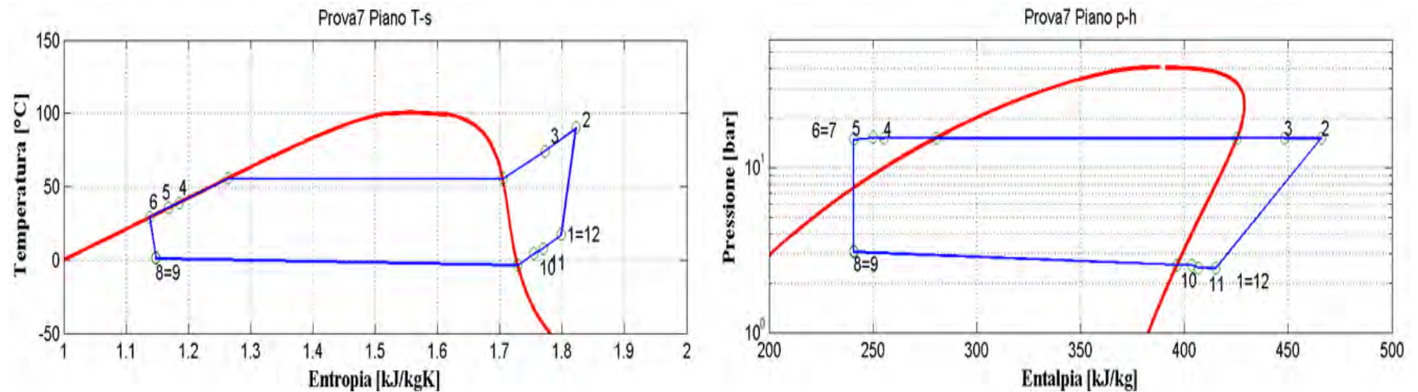
Figura 2.9: Piani T-s e p-h per la prova effettuata nelle condizioni 7 in modalità pompa di calore per il prototipo operante con R134a.
