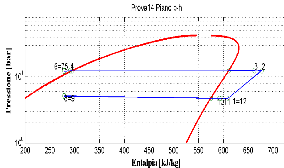
Figura 9.15: Piani T-s e p-h per la prova effettuata nelle condizioni 14 in modalità pompa di calore per il prototipo operante con R290.
