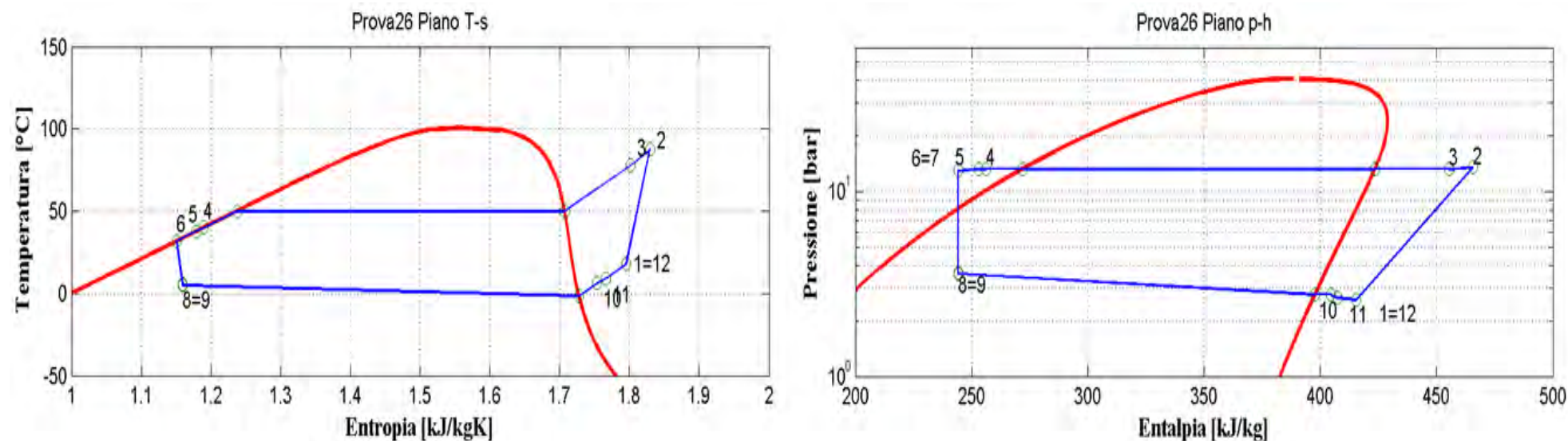
Figura 2.28: Piani T-s e p-h per la prova effettuata nelle condizioni 26 in modalità pompa di calore per il prototipo operante con R134a.
