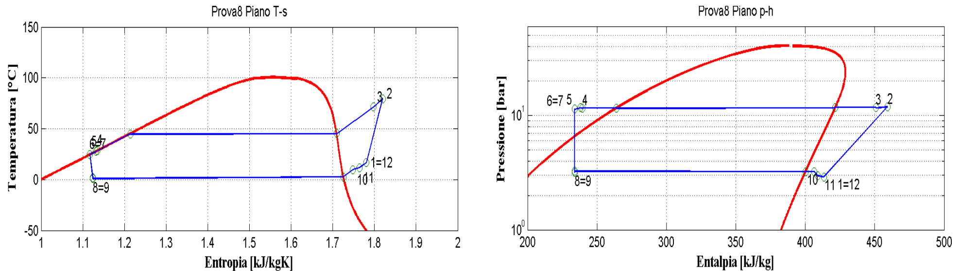
Figura 2.50: Piani T-s e p-h per la prova effettuata nelle condizioni 8 in modalità macchina frigorifera per il prototipo elaborante R134a.
