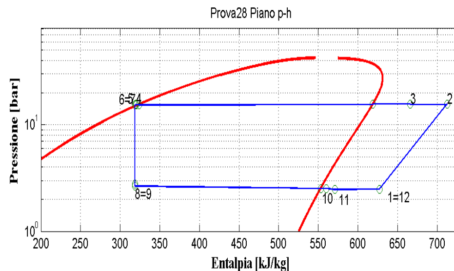
Figura 9.29: Piani T-s e p-h per la prova effettuata nelle condizioni 28 in modalità pompa di calore per il prototipo operante con R290.
