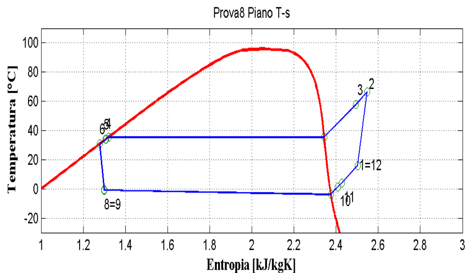
Figura 9.9: Piani T-s e p-h per la prova effettuata nelle condizioni 8 in modalità pompa di calore per il prototipo operante con R290.
