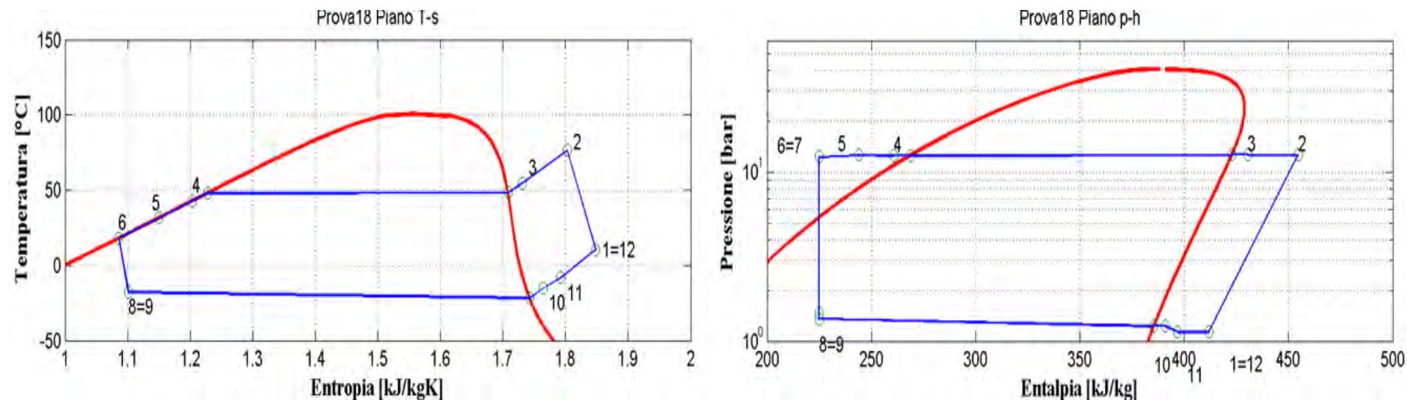
Figura 2.20: Piani T-s e p-h per la prova effettuata nelle condizioni 18 in modalità pompa di calore per il prototipo operante con R134a.
