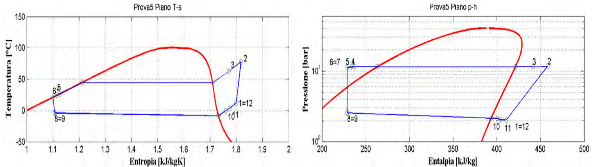
Figura 2.7: Piani T-s e p-h per la prova effettuata nelle condizioni 5 in modalità pompa di calore per il prototipo operante con R134a.
