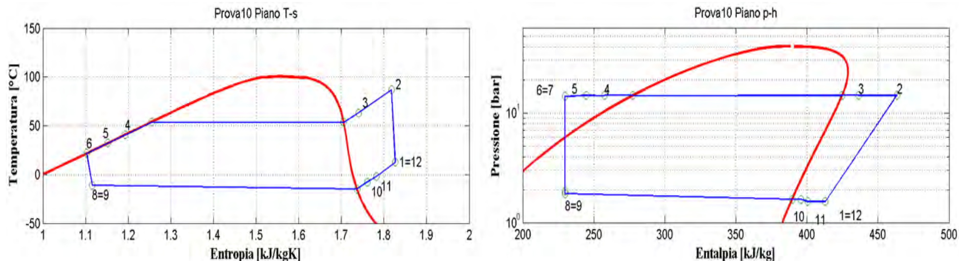
Figura 2.12: Piani T-s e p-h per la prova effettuata nelle condizioni 10 in modalità pompa di calore per il prototipo operante con R134a.
