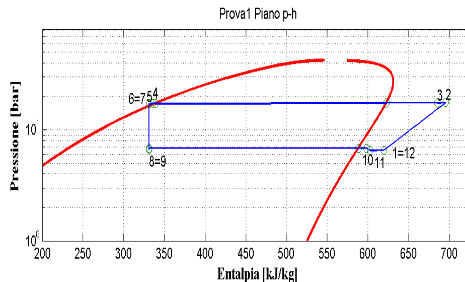
Figura 9.42: Piani T-s e p-h per la prova effettuata nelle condizioni 1 in modalità macchina frigorifera per il prototipo a propano (R290).
