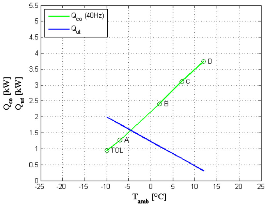
Figura 8.3: Andamento in funzione della temperatura esterna della potenza termica fornita dalla pompa di calore con compressore a 40 Hz (in verde) e quella richiesta dall'utenza (in blu).
