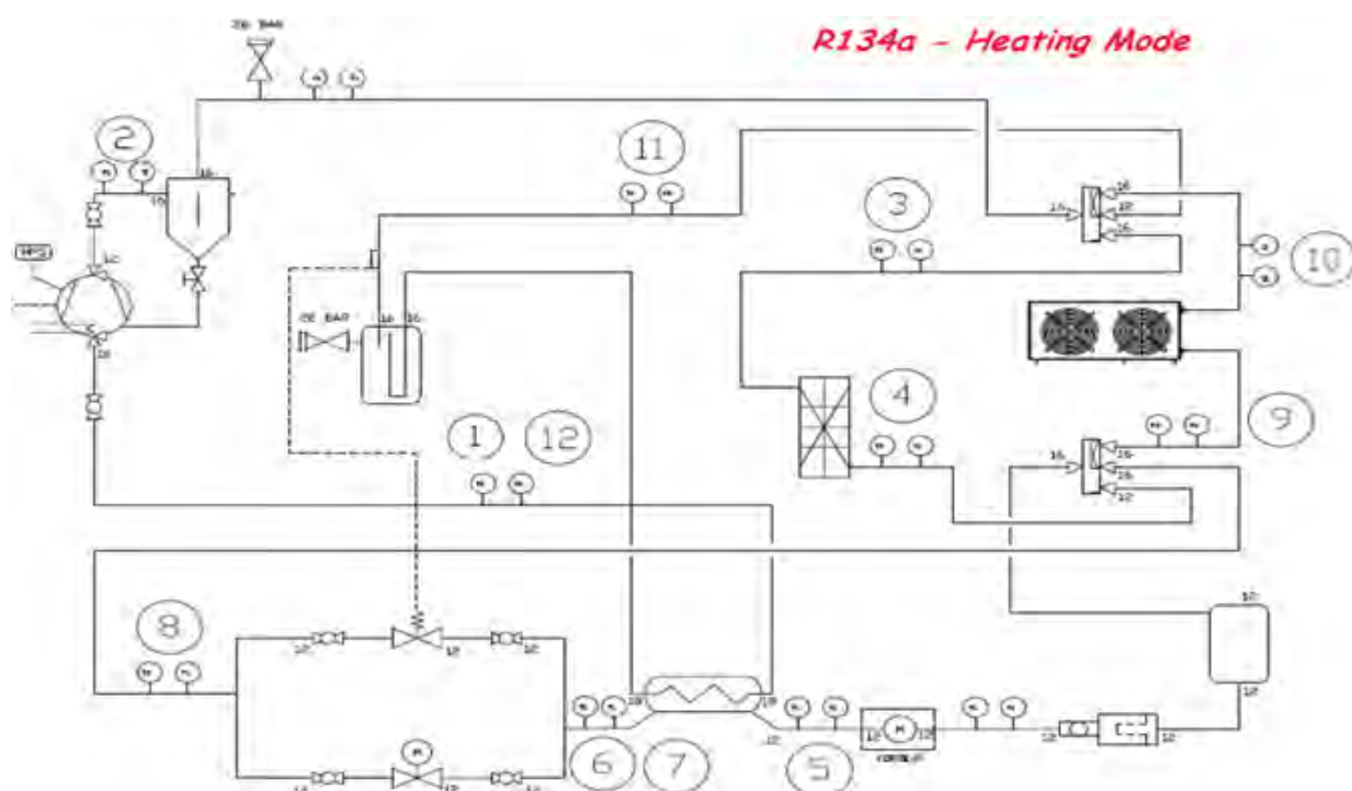
Figura 2.2: Schema impianto prototipo elaborante R134a in modalità pompa di calore.
