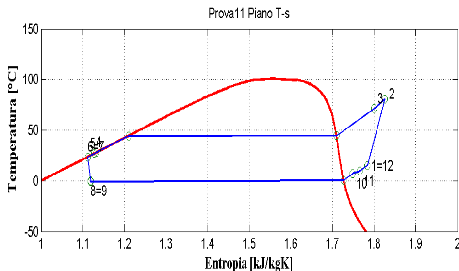
Figura 2.53: Piani T-s e p-h per la prova effettuata nelle condizioni 11 in modalità macchina frigorifera per il prototipo elaborante R134a.
