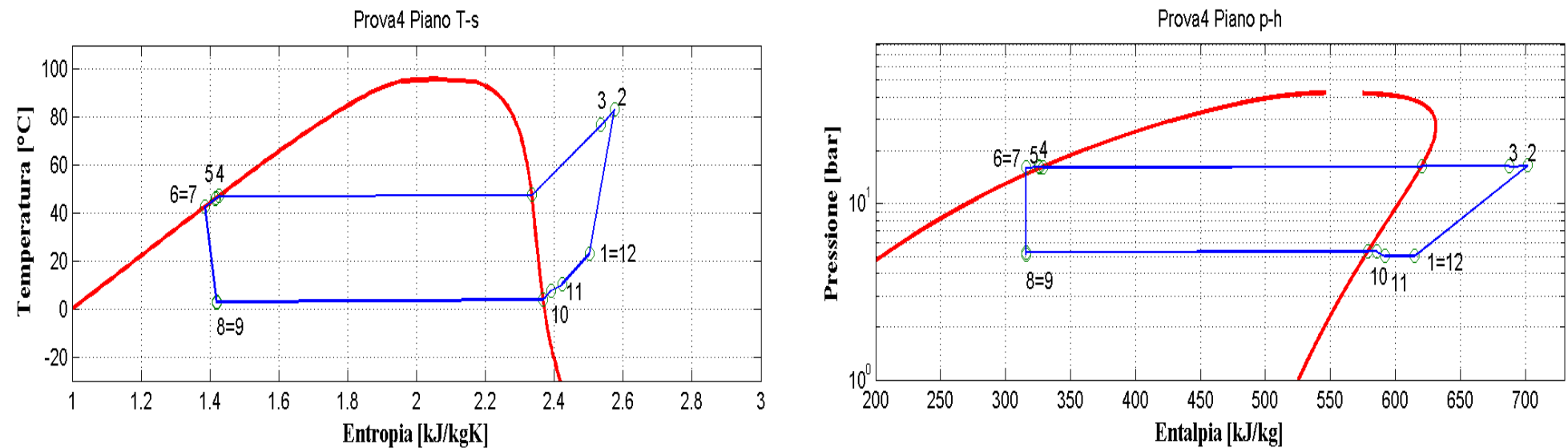
Figura 9.45: Piani T-s e p-h per la prova effettuata nelle condizioni 4 in modalità macchina frigorifera per il prototipo a propano (R290).
