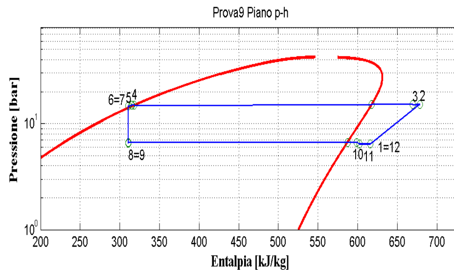
Figura 9.50: Piani T-s e p-h per la prova effettuata nelle condizioni 9 in modalità macchina frigorifera per il prototipo a propano (R290).
