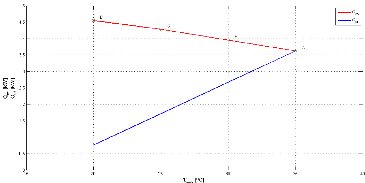
Figura 13.2: Andamento in funzione della temperatura esterna della potenza frigo fornita dalla macchina frigorifera elaborante R290 (in rosso) e quella richiesta dall'utenza (in blu).
