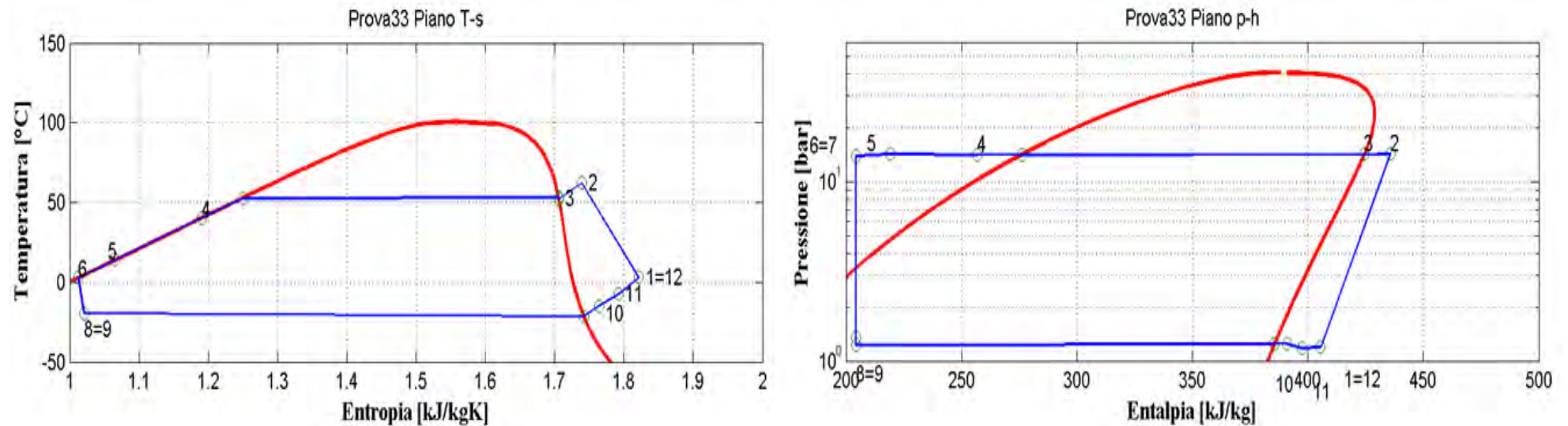
Figura 2.35: Piani T-s e p-h per la prova effettuata nelle condizioni 33 in modalità pompa di calore per il prototipo operante con R134a.
