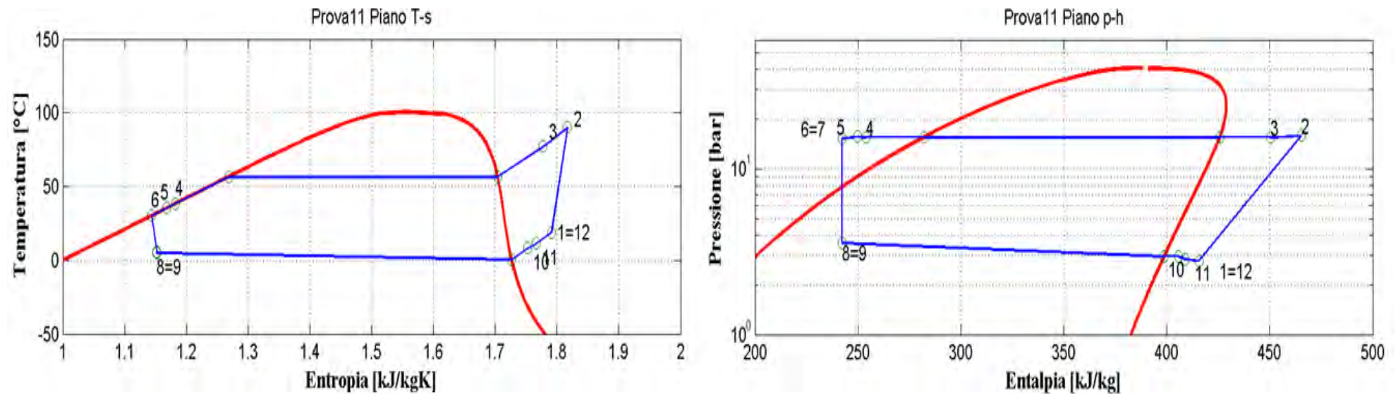
Figura 2.13: Piani T-s e p-h per la prova effettuata nelle condizioni 11 in modalità pompa di calore per il prototipo operante con R134a.
