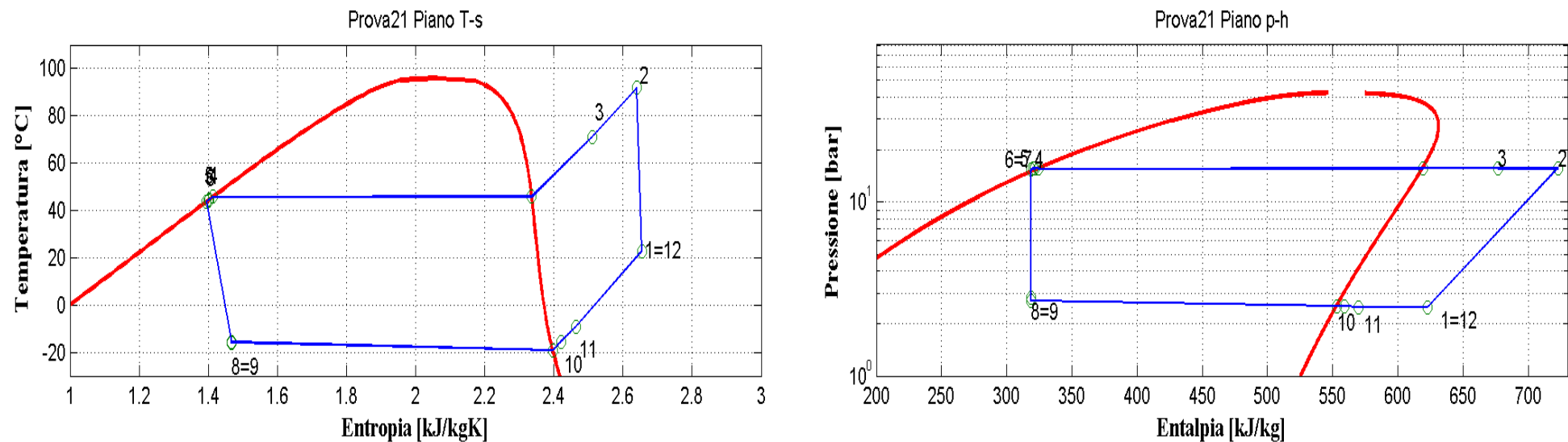
Figura 9.22: Piani T-s e p-h per la prova effettuata nelle condizioni 21 in modalità pompa di calore per il prototipo operante con R290.
