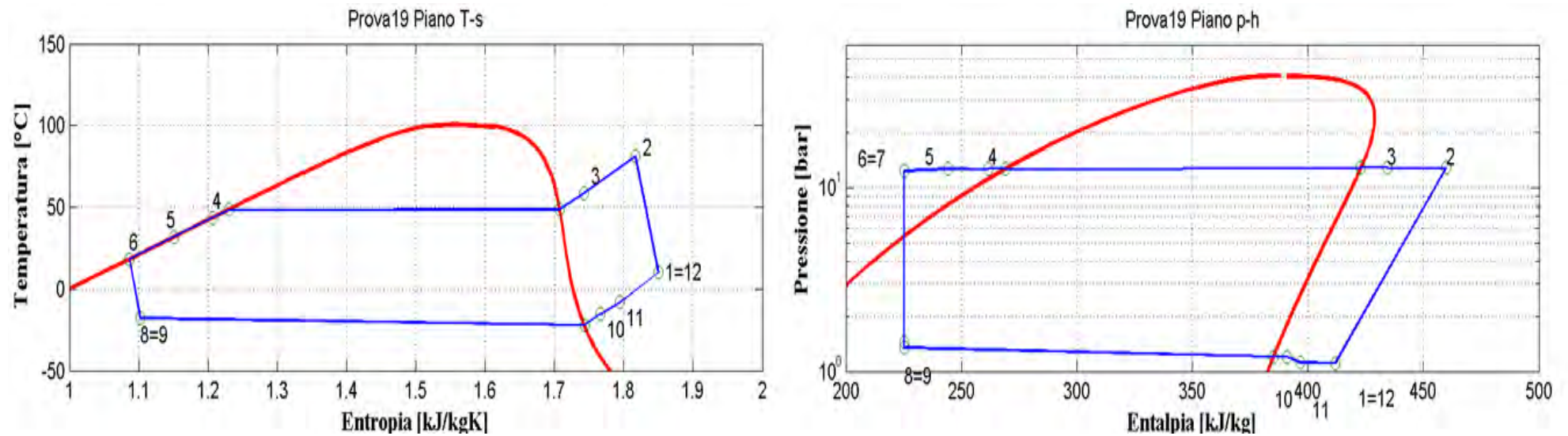
Figura 2.21: Piani T-s e p-h per la prova effettuata nelle condizioni 19 in modalità pompa di calore per il prototipo operante con R134a.
