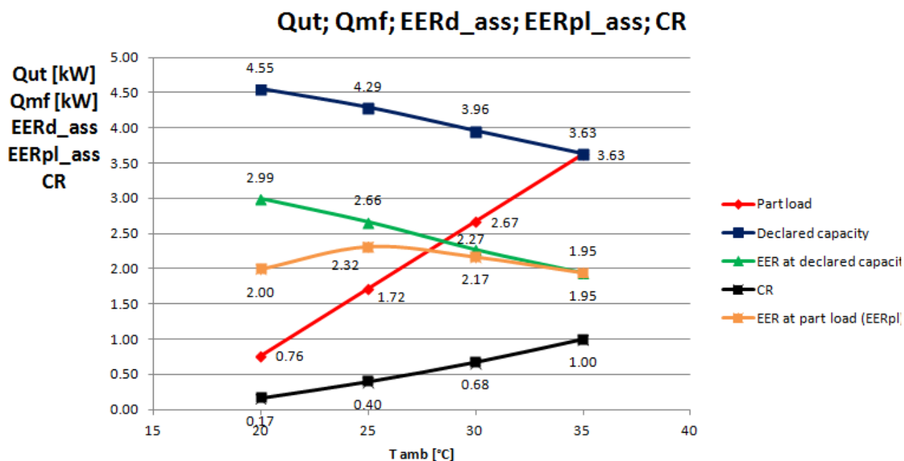
Figura 13.3: Andamento in funzione della temperatura esterna della potenza frigorifera fornita dalla macchina frigo (in blu), della potenza richiesta dall'utenza (in rosso), del rapporto di capacità CR (in nero), dell'EER dichiarato della macchina frigo (in verde) e dell'EER a carico parziale (in arancione), questi ultimi valutati considerando come spesa energetica la potenza elettrica assorbita dall'intero impianto
