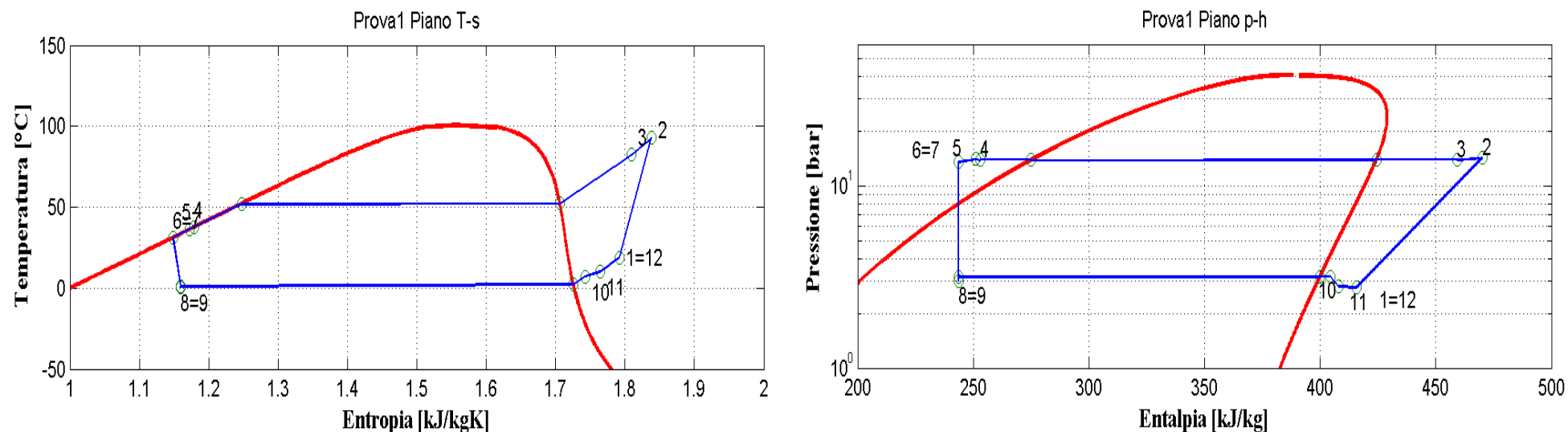
Figura 2.43: Piani T-s e p-h per la prova effettuata nelle condizioni 1 in modalità macchina frigorifera per il prototipo elaborante R134a.
