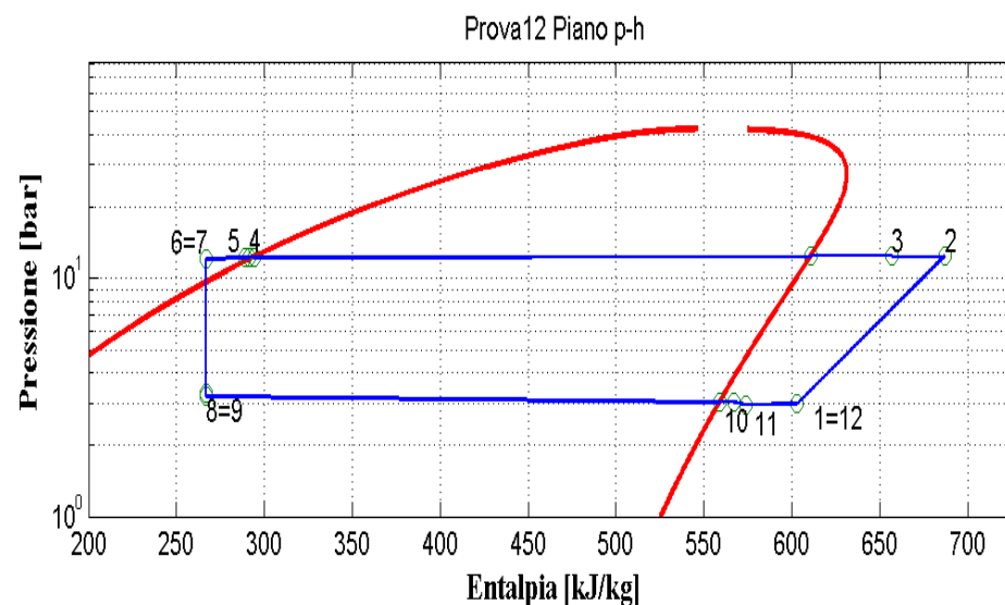
Figura 9.13: Piani T-s e p-h per la prova effettuata nelle condizioni 12 in modalità pompa di calore per il prototipo operante con R290.
