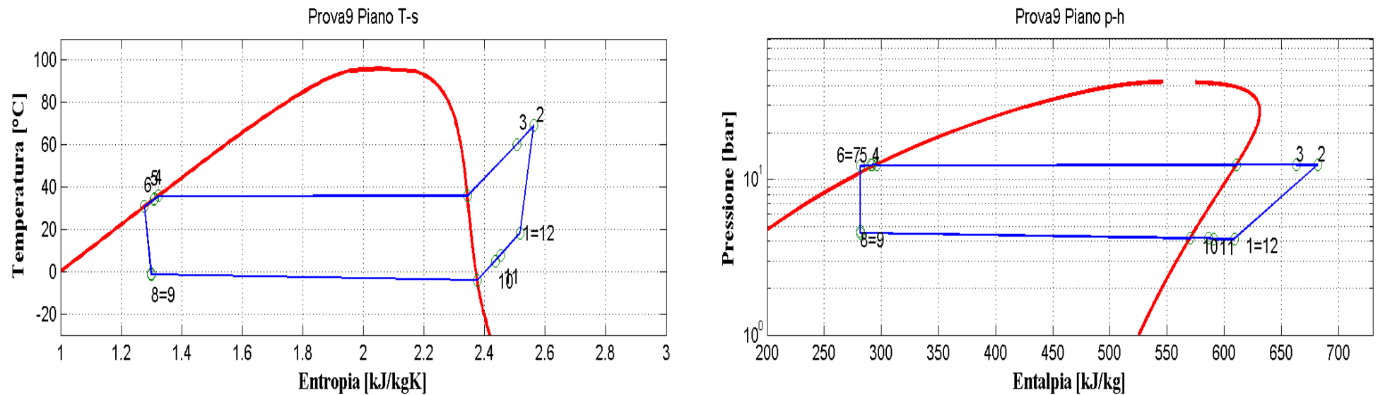
Figura 9.10: Piani T-s e p-h per la prova effettuata nelle condizioni 9 in modalità pompa di calore per il prototipo operante con R290.
