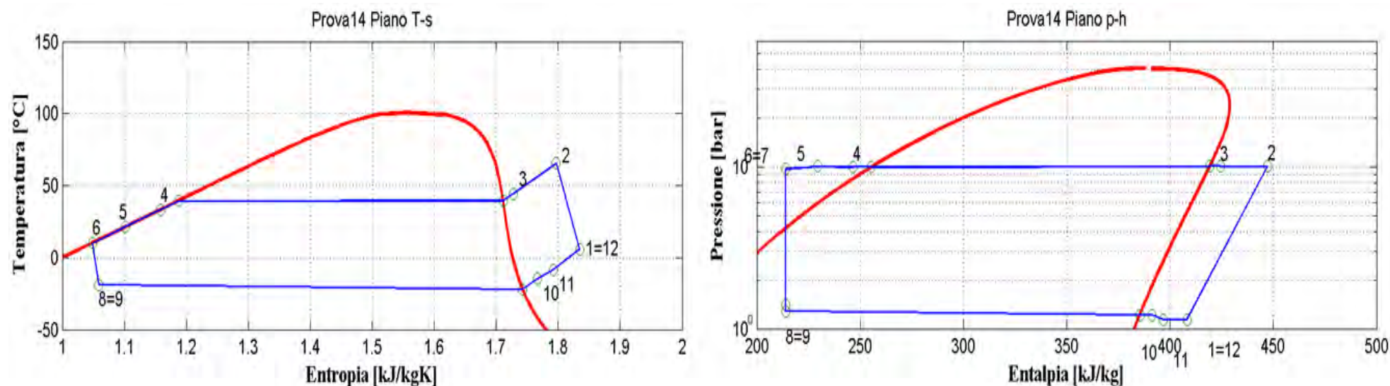
Figura 2.16: Piani T-s e p-h per la prova effettuata nelle condizioni 14 in modalità pompa di calore per il prototipo operante con R134a.
