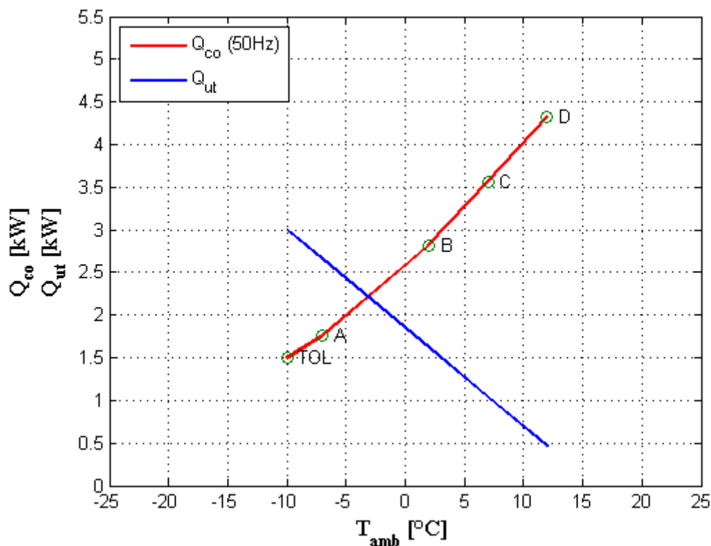
Figura 8.1: Andamento in funzione della temperatura esterna della potenza termica fornita dalla pompa di calore a R134a (in rosso) e quella richiesta dalla nuova utenza (in blu).
