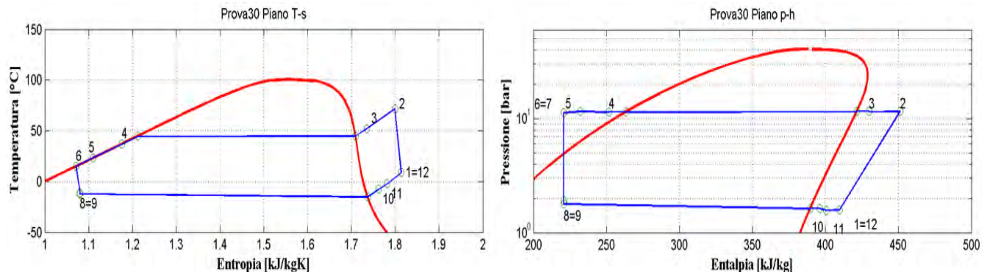
Figura 2.32: Piani T-s e p-h per la prova effettuata nelle condizioni 30 in modalità pompa di calore per il prototipo operante con R134a.
