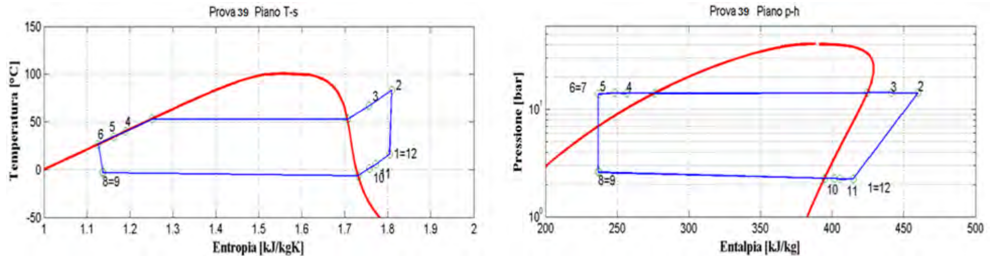
Figura 2.41: Piani T-s e p-h per la prova effettuata nelle condizioni 39 in modalità pompa di calore per il prototipo operante con R134a.
