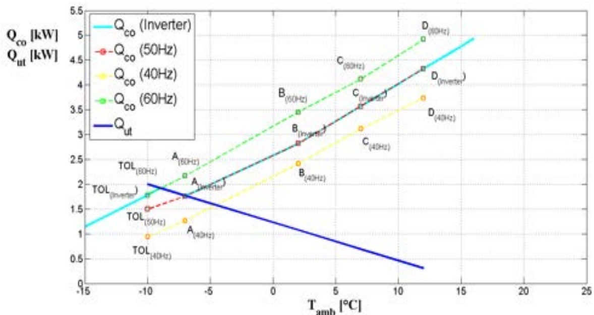
Figura 8.8: Andamento in funzione della temperatura esterna della potenza termica fornita dalla pompa di calore elaborante R134a con compressore funzionante con inverter tra 60 e 50 Hz (curva in azzurro), e quella richiesta dall'utenza (curva in blu).
