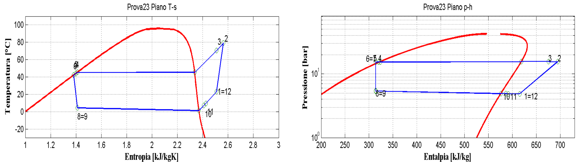
Figura 9.24: Piani T-s e p-h per la prova effettuata nelle condizioni 23 in modalità pompa di calore per il prototipo operante con R290.
