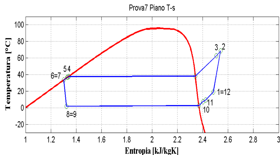
Figura 9.48: Piani T-s e p-h per la prova effettuata nelle condizioni 7 in modalità macchina frigorifera per il prototipo a propano (R290).
