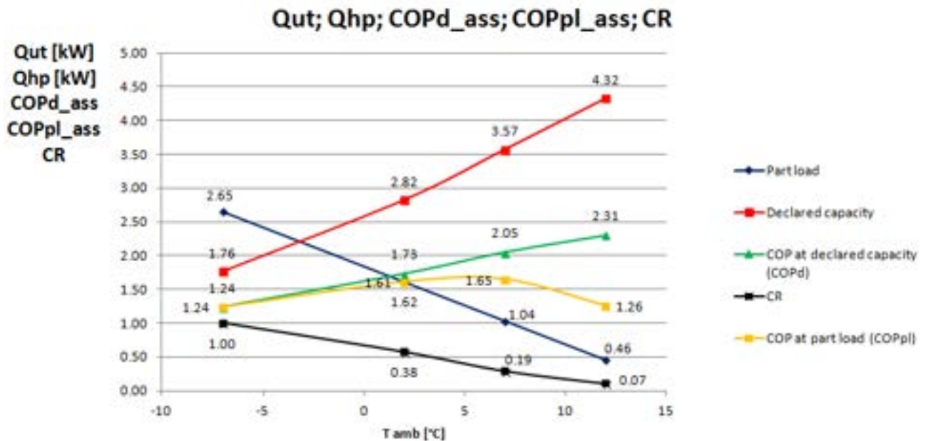
Figura 8.2: Andamento in funzione della temperatura esterna della potenza termica fornita dalla pompa di calore a R134a (in rosso), della potenza richiesta dalla nuova utenza (in blu), del rapporto di capacità CR (in nero), del COP dichiarato della pompa di calore (in verde) e del COP a carico parziale (in giallo) questi ultimi valutati considerando come spesa energetica la potenza elettrica assorbita dall'intero impianto
