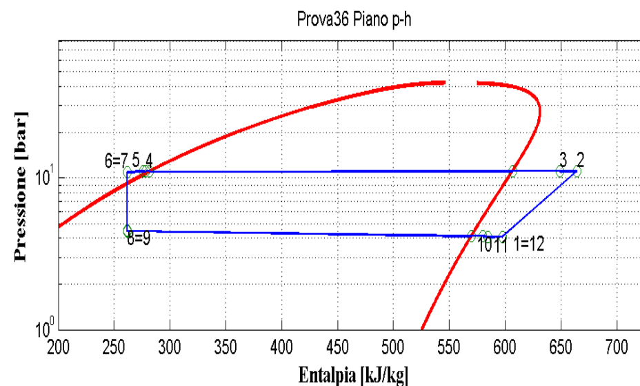
Figura 9.37: Piani T-s e p-h per la prova effettuata nelle condizioni 36 in modalità pompa di calore per il prototipo operante con R290.
