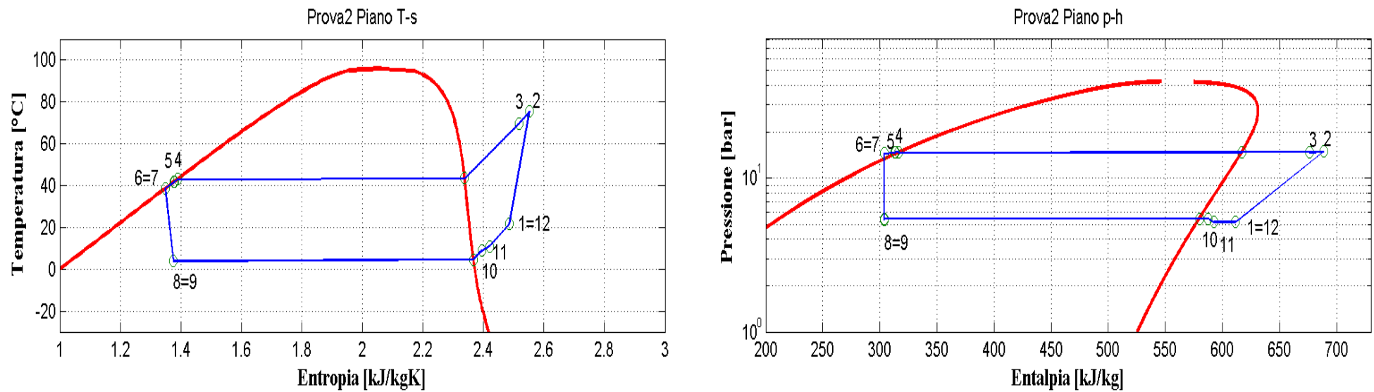
Figura 9.43: Piani T-s e p-h per la prova effettuata nelle condizioni 2 in modalità macchina frigorifera per il prototipo a propano (R290).
