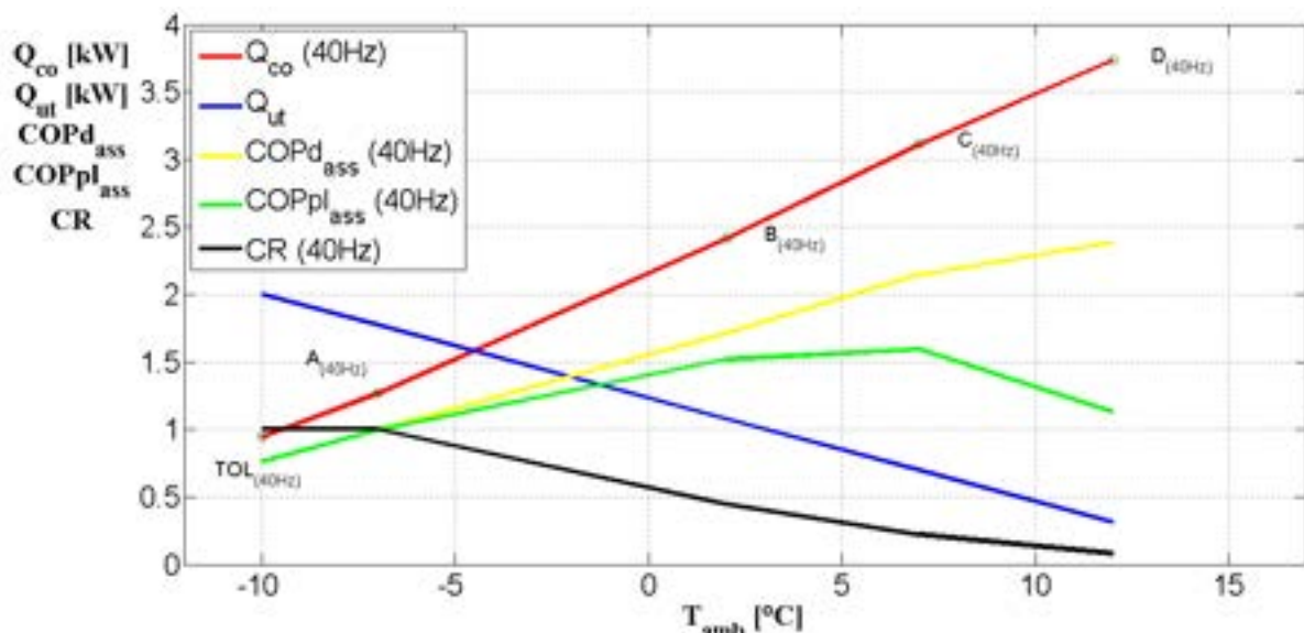
Figura 8.4: Andamento in funzione della temperatura esterna della potenza termica fornita dalla pompa di calore con compressore a 40 Hz operante con R134a (in rosso), quella richiesta dall'nuova utenza (in blu), del COP dichiarato della pompa di calore (in giallo), del COP a carico parziale (in verde) e del fattore CR (in nero)
