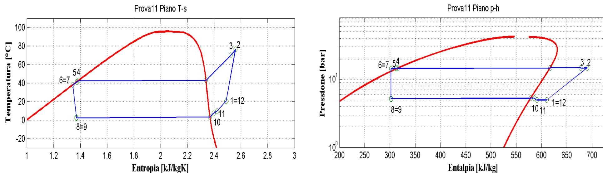
Figura 9.52: Piani T-s e p-h per la prova effettuata nelle condizioni 11 in modalità macchina frigorifera per il prototipo a propano (R290).
