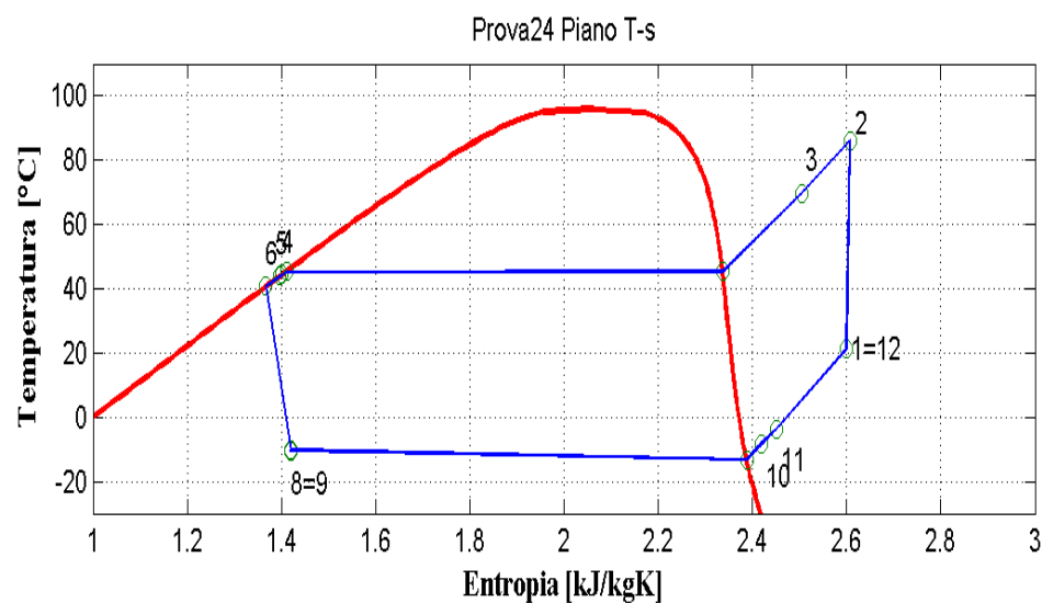
Figura 9.25: Piani T-s e p-h per la prova effettuata nelle condizioni 24 in modalità pompa di calore per il prototipo operante con R290.
