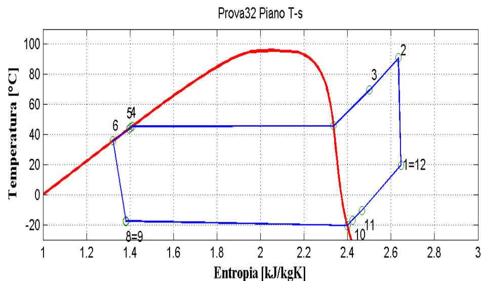
Figura 9.33: Piani T-s e p-h per la prova effettuata nelle condizioni 32 in modalità pompa di calore per il prototipo operante con R290.
