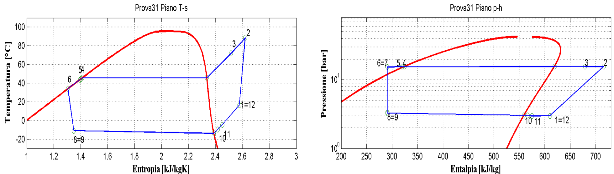
Figura 9.32: Piani T-s e p-h per la prova effettuata nelle condizioni 31 in modalità pompa di calore per il prototipo operante con R290.
