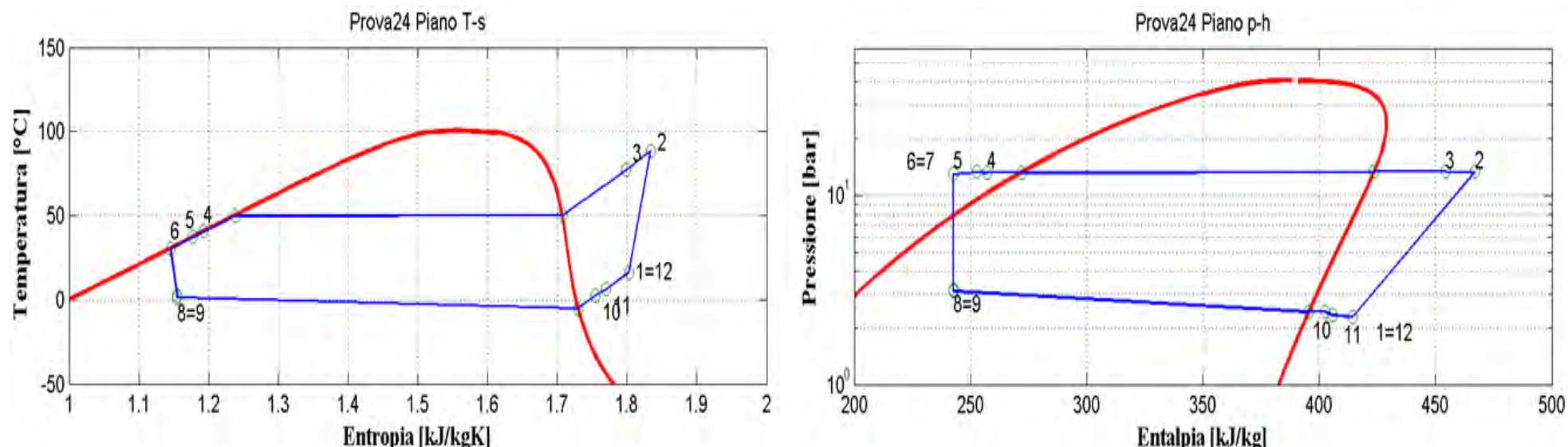
Figura 2.26: Piani T-s e p-h per la prova effettuata nelle condizioni 24 in modalità pompa di calore per il prototipo operante con R134a.
