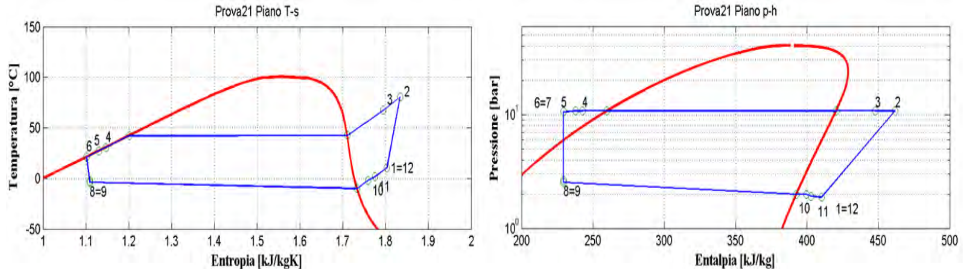
Figura 2.23: Piani T-s e p-h per la prova effettuata nelle condizioni 21 in modalità pompa di calore per il prototipo operante con R134a.
