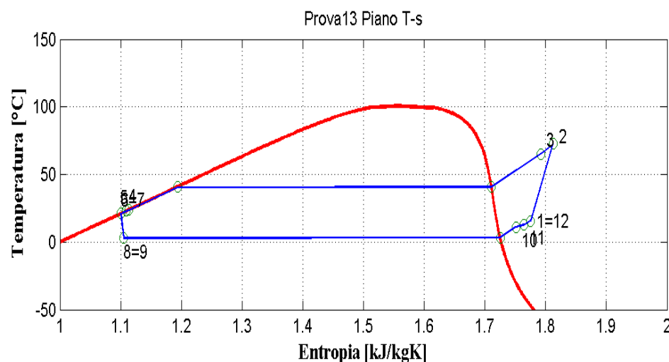
Figura 2.55: Piani T-s e p-h per la prova effettuata nelle condizioni 13 in modalità macchina frigorifera per il prototipo elaborante R134a.
