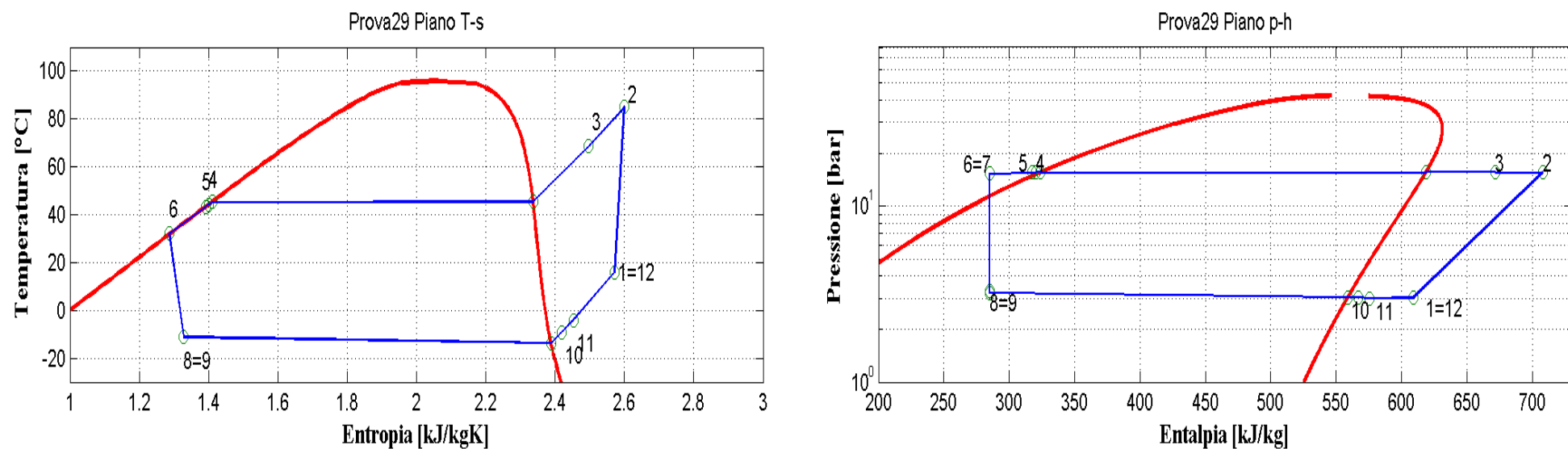
Figura 9.30: Piani T-s e p-h per la prova effettuata nelle condizioni 29 in modalità pompa di calore per il prototipo operante con R290.
