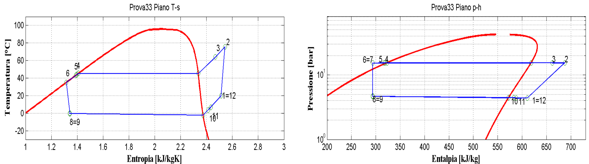
Figura 9.34: Piani T-s e p-h per la prova effettuata nelle condizioni 33 in modalità pompa di calore per il prototipo operante con R290.
