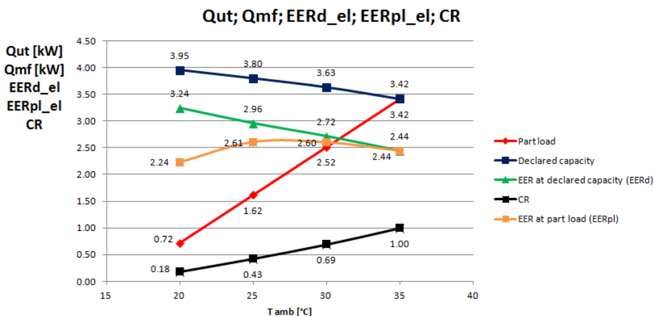
Figura 6.4: Andamento in funzione della temperatura esterna della potenza frigorifera fornita dalla macchina frigo (in blu), della potenza richiesta dall'utenza (in rosso), del rapporto di capacità CR (in nero), dell'EER dichiarato della macchina frigo (in verde) e dell'EER a carico parziale (in arancione), questi ultimi valutati considerando come spesa energetica la potenza elettrica assorbita dal solo compressore
