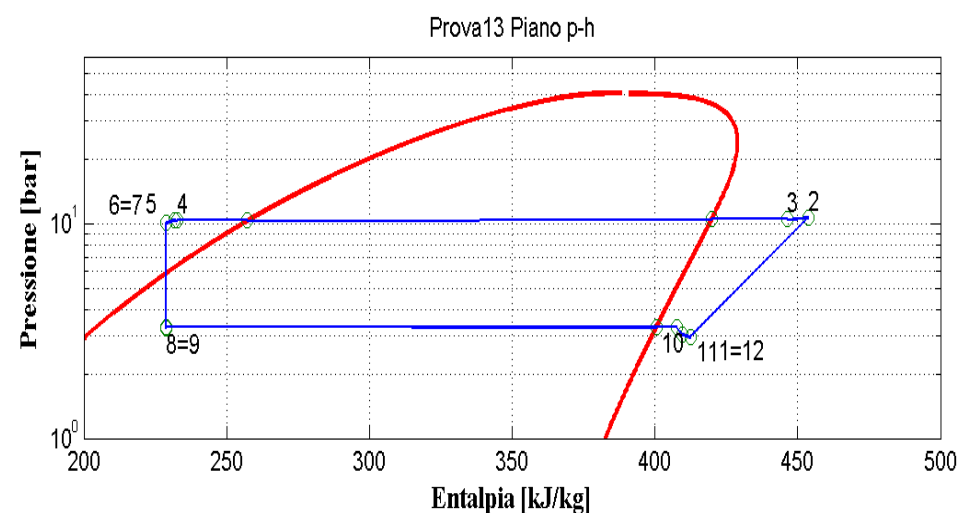
Figura 2.55: Piani T-s e p-h per la prova effettuata nelle condizioni 13 in modalità macchina frigorifera per il prototipo elaborante R134a.
