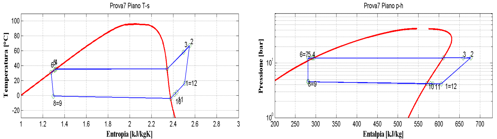
Figura 9.8: Piani T-s e p-h per la prova effettuata nelle condizioni 7 in modalità pompa di calore per il prototipo operante con R290.
