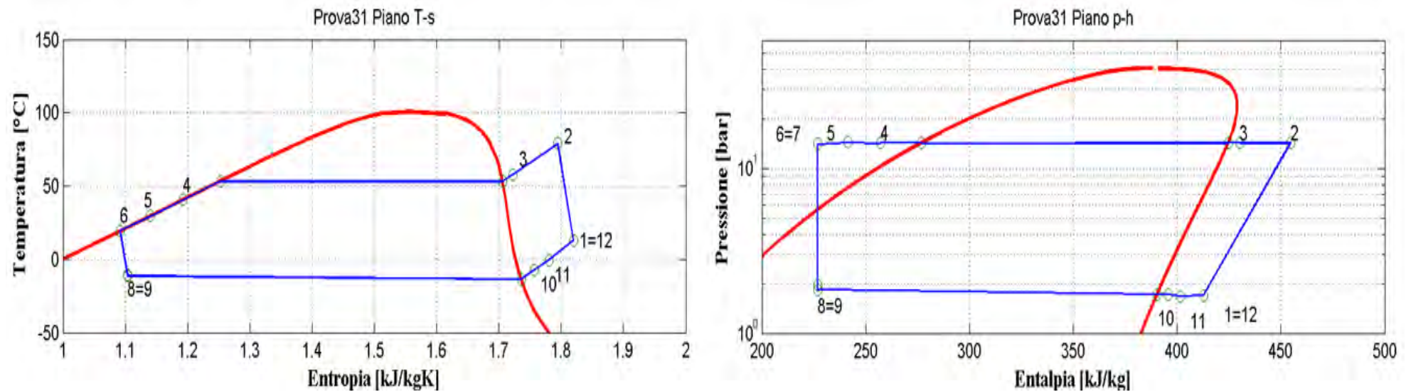
Figura 2.33: Piani T-s e p-h per la prova effettuata nelle condizioni 31 in modalità pompa di calore per il prototipo operante con R134a.
