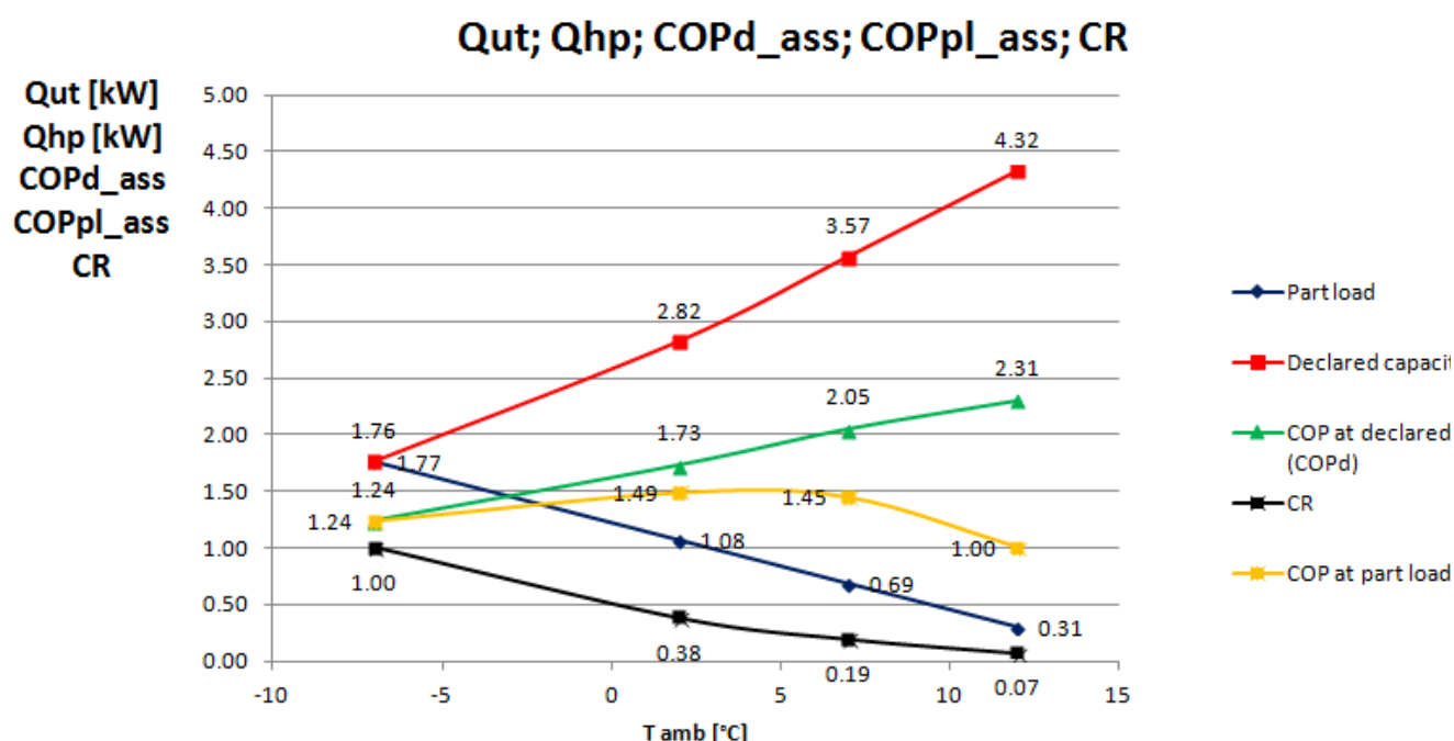
Figura 4.3: Andamento in funzione della temperatura esterna della potenza termica fornita dalla pompa di calore a R134a (in rosso), della potenza richiesta dall'utenza (in blu), del rapporto di capacità CR (in nero), del COP dichiarato della pompa di calore (in verde) e del COP a carico parziale (in giallo) questi ultimi valutati considerando come spesa energetica la potenza elettrica assorbita dall'intero impianto.
