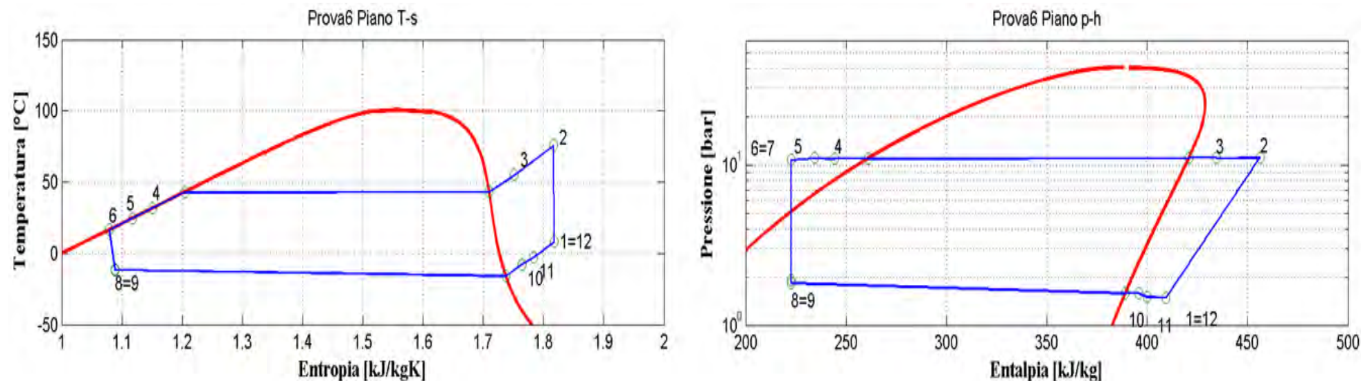
Figura 2.8: Piani T-s e p-h per la prova effettuata nelle condizioni 6 in modalità pompa di calore per il prototipo operante con R134a.
