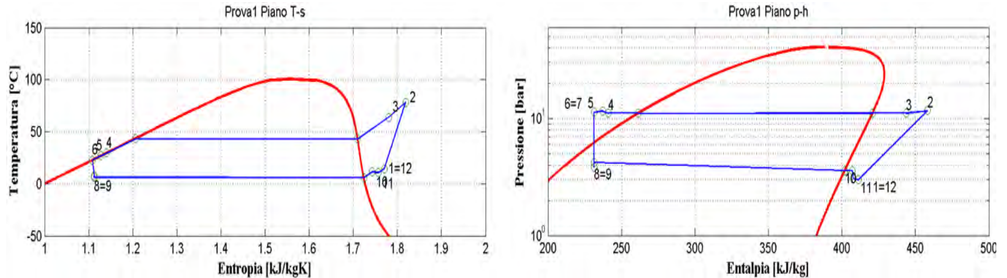
Figura 2.3: Piani T-s e p-h per la prova effettuata nelle condizioni 1 in modalità pompa di calore per il prototipo operante con R134a.
