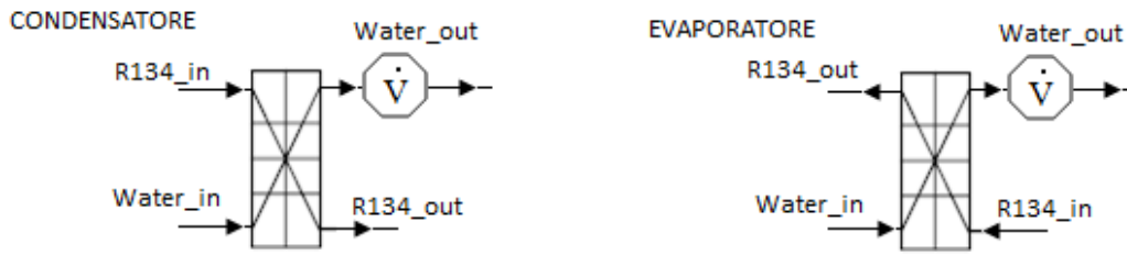
Figura 2.1: Posizione del misuratore di portata volumetrica dell'acqua.
