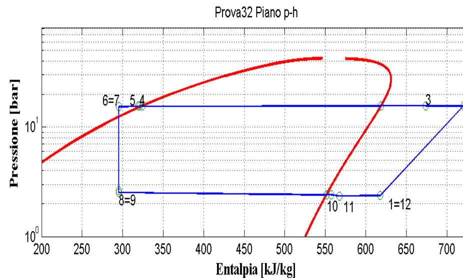
Figura 9.33: Piani T-s e p-h per la prova effettuata nelle condizioni 32 in modalità pompa di calore per il prototipo operante con R290.
