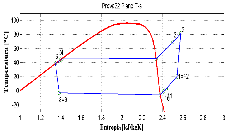
Figura 9.23: Piani T-s e p-h per la prova effettuata nelle condizioni 22 in modalità pompa di calore per il prototipo operante con R290.
