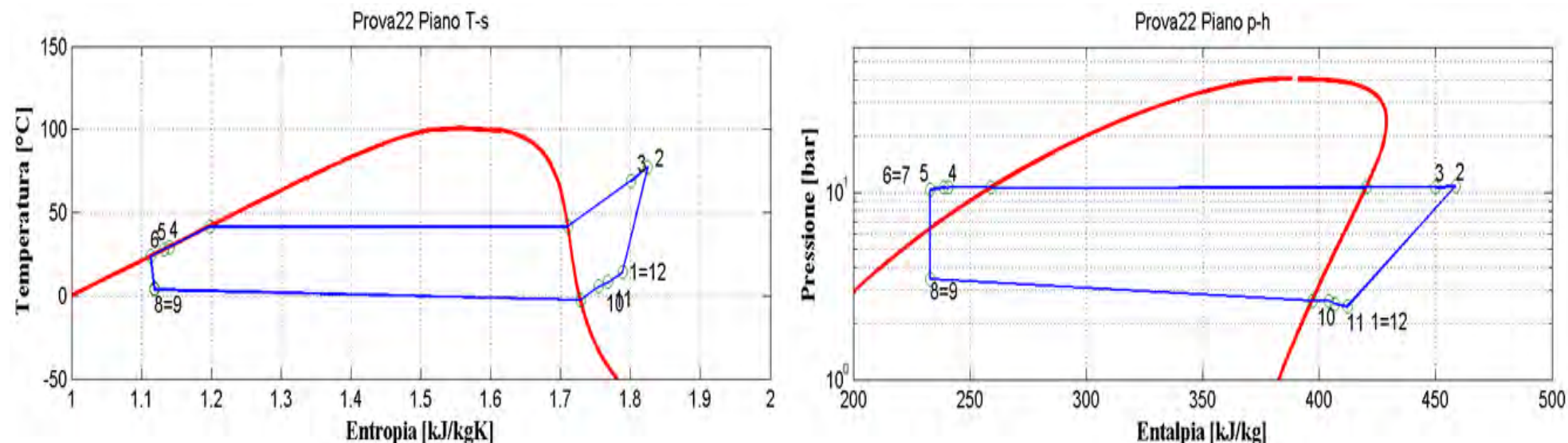
Figura 2.24: Piani T-s e p-h per la prova effettuata nelle condizioni 22 in modalità pompa di calore per il prototipo operante con R134a.
