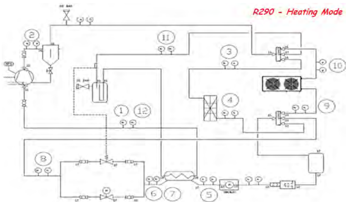
Figura 9.1: Schema d'impianto del prototipo operante con propano (R290) in modalità pompa di calore.
