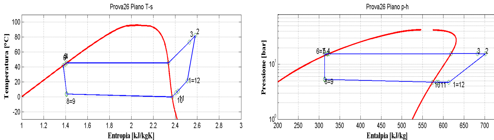
Figura 9.27: Piani T-s e p-h per la prova effettuata nelle condizioni 26 in modalità pompa di calore per il prototipo operante con R290.
