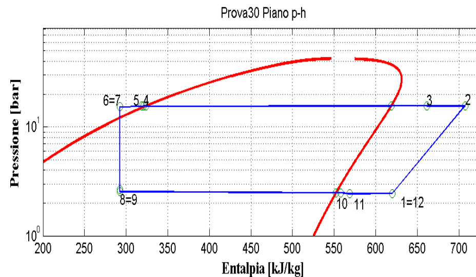
Figura 9.31: Piani T-s e p-h per la prova effettuata nelle condizioni 30 in modalità pompa di calore per il prototipo operante con R290.
