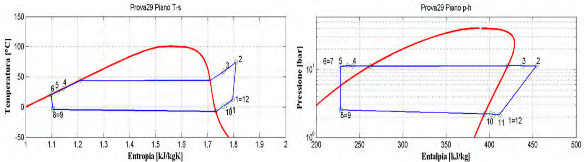
Figura 2.31: Piani T-s e p-h per la prova effettuata nelle condizioni 29 in modalità pompa di calore per il prototipo operante con R134a.
