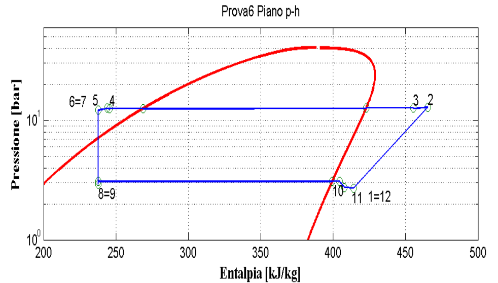
Figura 2.48: Piani T-s e p-h per la prova effettuata nelle condizioni 6 in modalità macchina frigorifera per il prototipo elaborante R134a.
