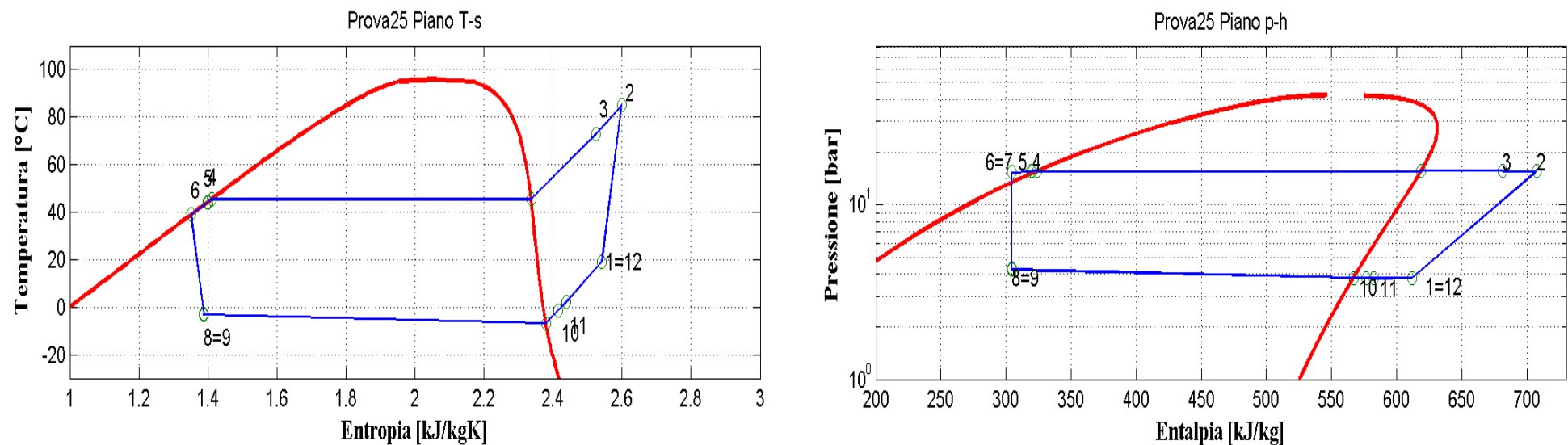
Figura 9.26: Piani T-s e p-h per la prova effettuata nelle condizioni 25 in modalità pompa di calore per il prototipo operante con R290.
