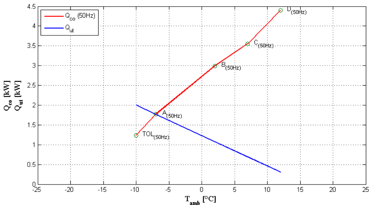
Figura 11.2: Andamento in funzione della temperatura esterna della potenza termica fornita dalla pompa di calore elaborante R290 (in rosso) e quella richiesta dall'utenza (in blu).
