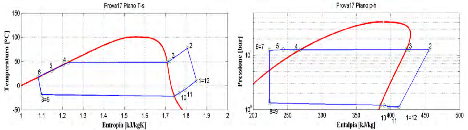
Figura 2.19: Piani T-s e p-h per la prova effettuata nelle condizioni 17 in modalità pompa di calore per il prototipo operante con R134a.
