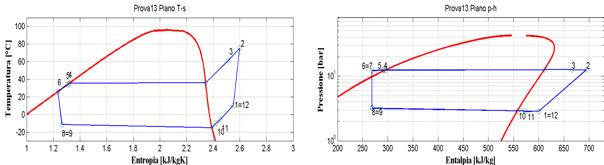
Figura 9.14: Piani T-s e p-h per la prova effettuata nelle condizioni 13 in modalità pompa di calore per il prototipo operante con R290.
