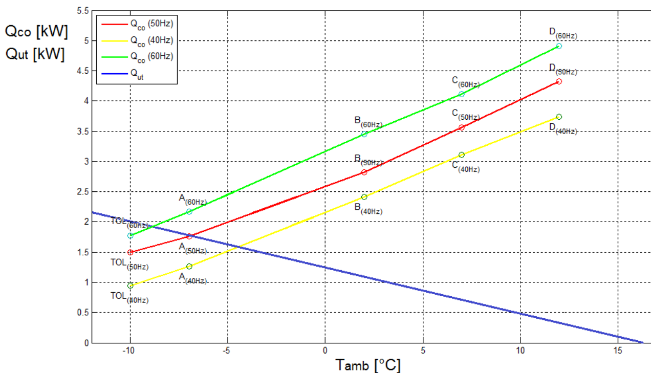
Figura 8.7: Andamento in funzione della temperatura esterna della potenza termica fornita dalla pompa di calore a R134a con compressore rispettivamente a 40Hz (in giallo), a 50 Hz (in rosso), a 60 Hz (in verde), e quella richiesta dall'utenza (in blu).
