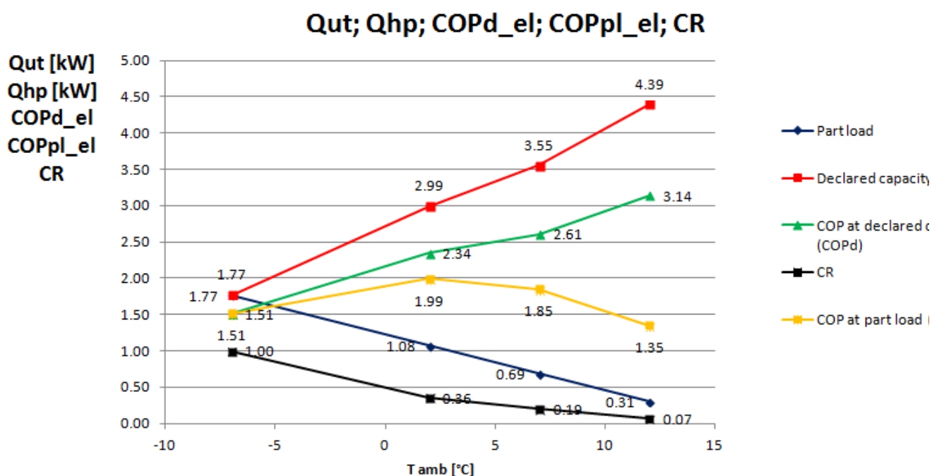
Figura 11.4: Andamento in funzione della temperatura esterna della potenza termica fornita dalla pompa di calore a propano (in rosso), della potenza richiesta dall'utenza (in blu), del rapporto di capacità C_R (in nero), del COP dichiarato della pompa di calore (in verde) e del COP a carico parziale (in giallo) questi ultimi valutati considerando come spesa energetica la potenza elettrica assorbita dal solo compressore.
