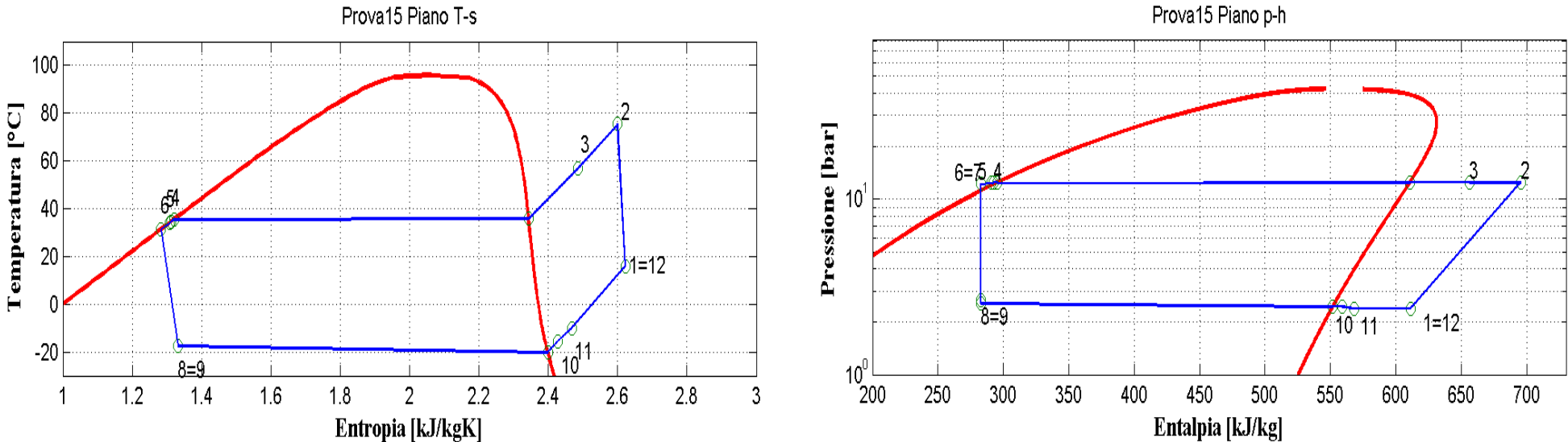
Figura 9.16: Piani T-s e p-h per la prova effettuata nelle condizioni 15 in modalità pompa di calore per il prototipo operante con R290.
