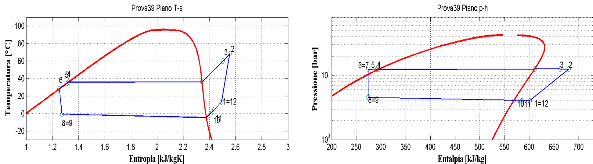
Figura 9.40: Piani T-s e p-h per la prova effettuata nelle condizioni 39 in modalità pompa di calore per il prototipo operante con R290.
