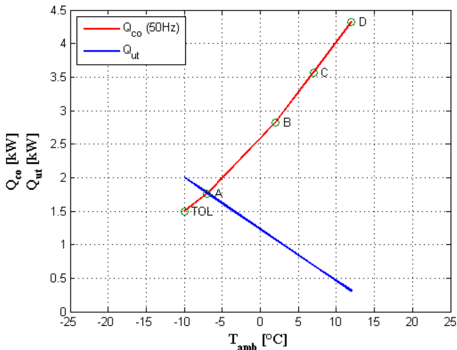
Figura 4.2: Andamento in funzione della temperatura esterna della potenza termica fornita dalla pompa di calore elaborante R134a (in rosso) e quella richiesta dall'utenza (in blu).
