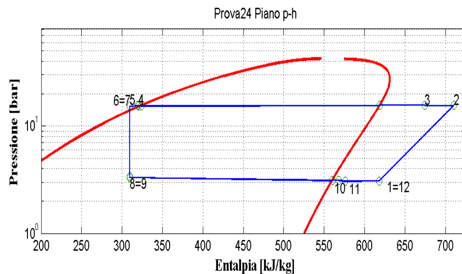
Figura 9.25: Piani T-s e p-h per la prova effettuata nelle condizioni 24 in modalità pompa di calore per il prototipo operante con R290.
