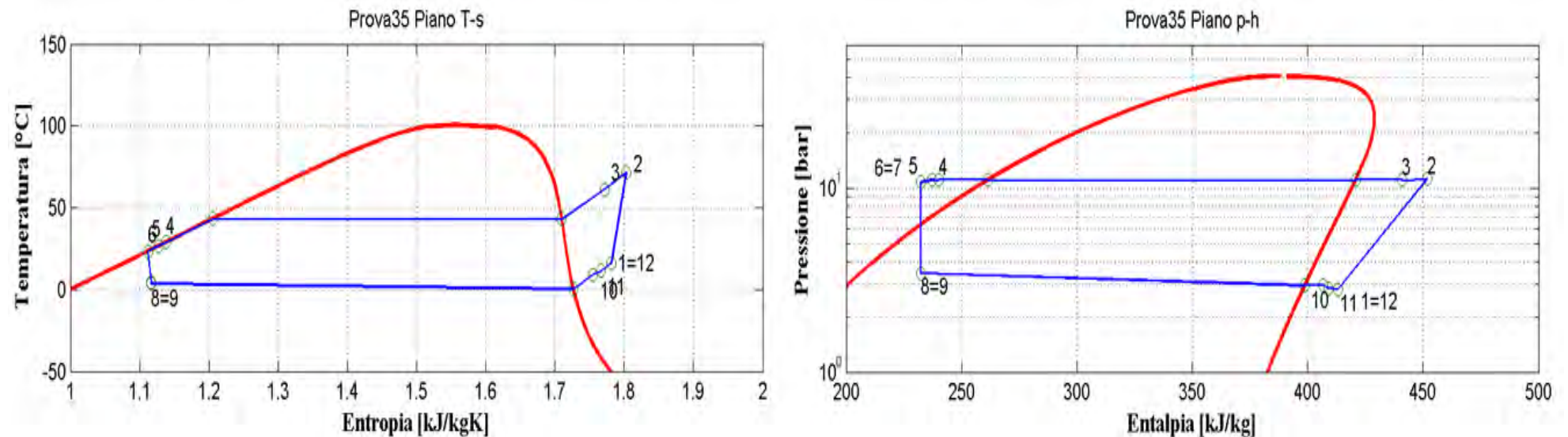
Figura 2.37: Piani T-s e p-h per la prova effettuata nelle condizioni 35 in modalità pompa di calore per il prototipo operante con R134a.
