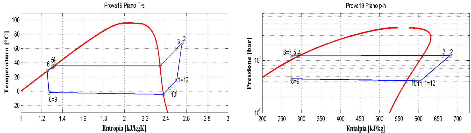
Figura 9.20: Piani T-s e p-h per la prova effettuata nelle condizioni 19 in modalità pompa di calore per il prototipo operante con R290.
