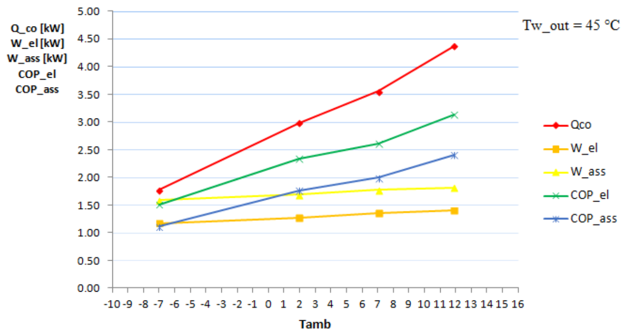
Fig. 11.1: Andamento della \dot{Q}_{co} , W_{el} , W_{ass} , COP_{el} , COP_{ass} al variare della temperatura ambiente per una fissata temperature dell'acqua in uscita dallo scambiatore per il prototipo a propano (R290).
