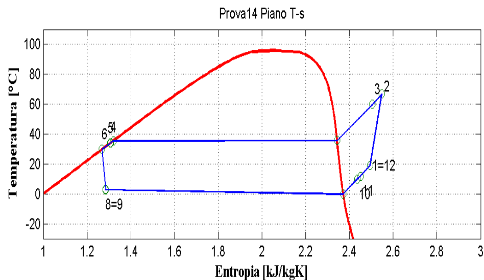
Figura 9.15: Piani T-s e p-h per la prova effettuata nelle condizioni 14 in modalità pompa di calore per il prototipo operante con R290.
