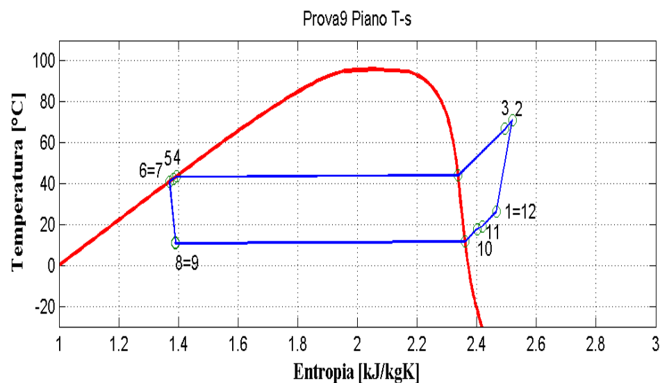
Figura 9.50: Piani T-s e p-h per la prova effettuata nelle condizioni 9 in modalità macchina frigorifera per il prototipo a propano (R290).
