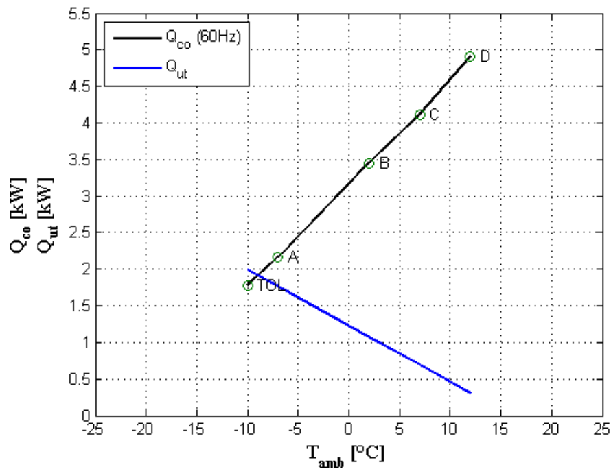
Figura 8.5: Andamento in funzione della temperatura esterna della potenza termica fornita dalla pompa di calore a R134a con compressore a 60 Hz (in nero) e quella richiesta dall'utenza (in blu).
