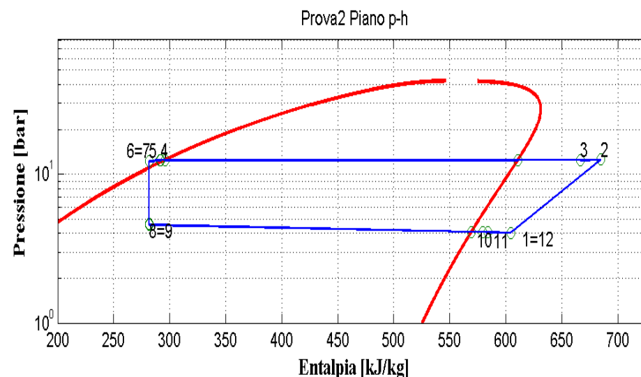
Figura 9.3: Piani T-s e p-h per la prova effettuata nelle condizioni 2 in modalità pompa di calore per il prototipo operante con R290.
