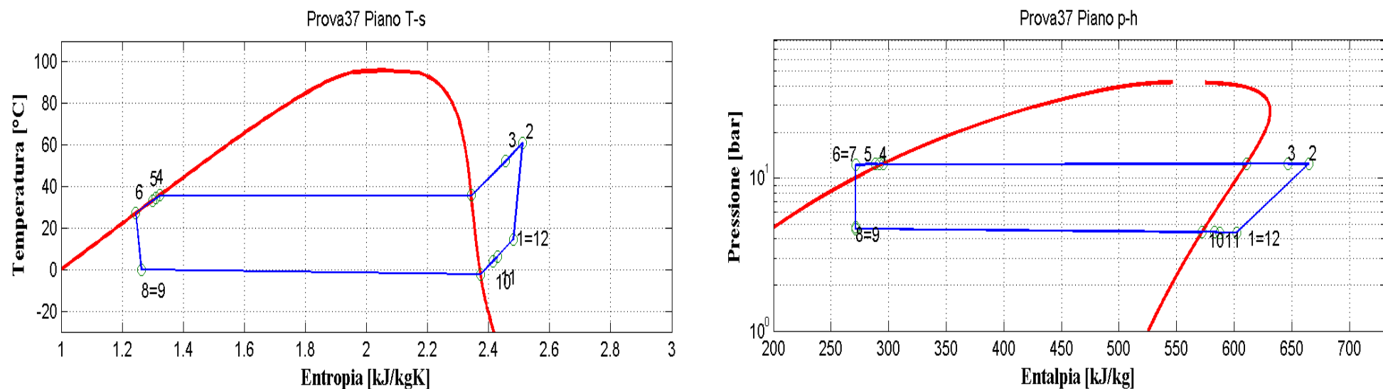
Figura 9.38: Piani T-s e p-h per la prova effettuata nelle condizioni 37 in modalità pompa di calore per il prototipo operante con R290.
