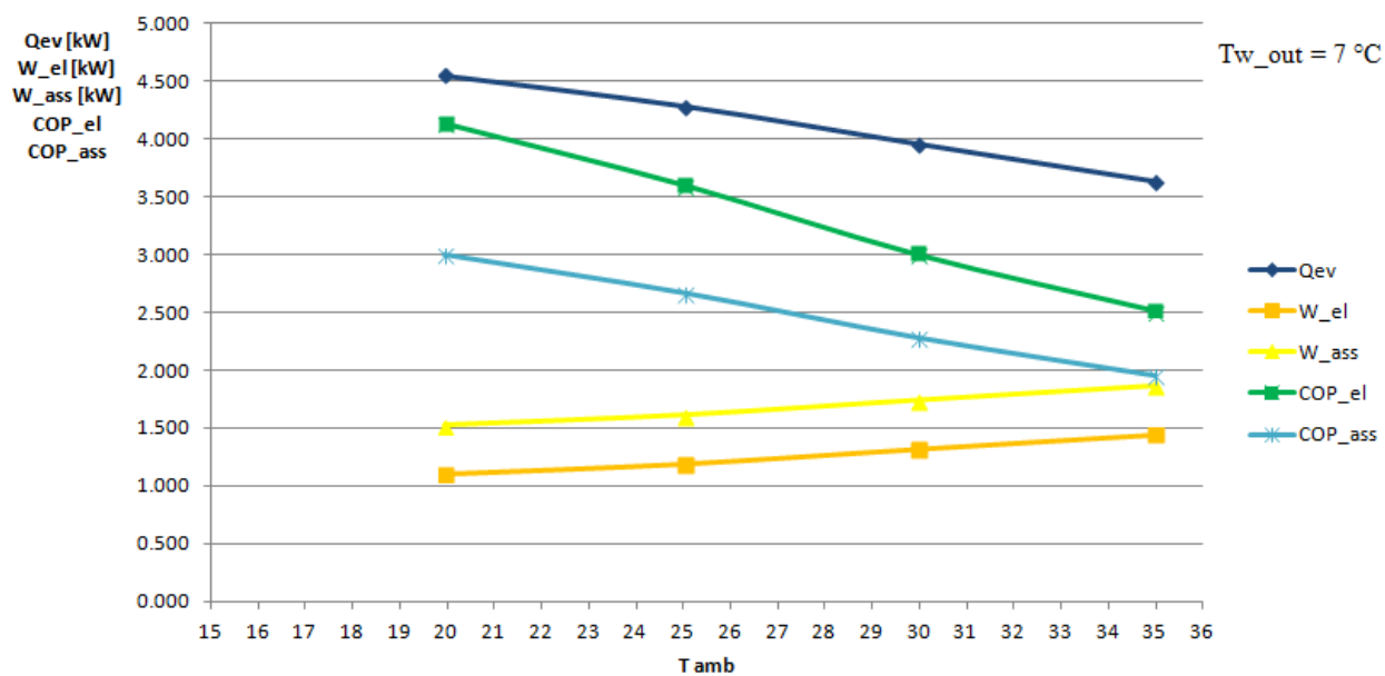
Figura 13.1: Andamento della \dot{Q}_{ev} , W_{el} , W_{ass} , COP_{el} , COP_{ass} al variare della temperatura ambiente per una fissata temperature dell'acqua in uscita dallo scambiatore per il prototipo operante con R290 in modalità macchina frigorifera.
