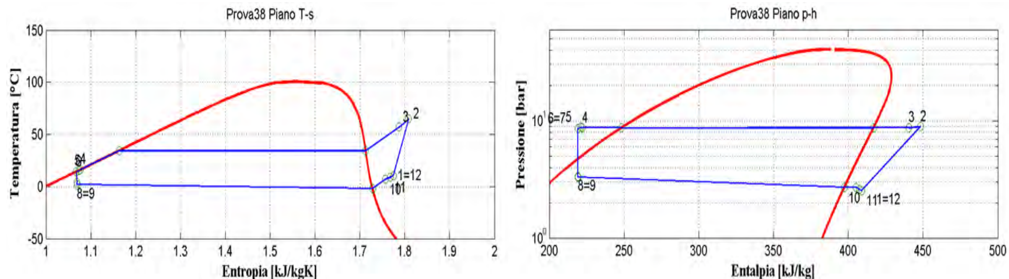
Figura 2.40: Piani T-s e p-h per la prova effettuata nelle condizioni 38 in modalità pompa di calore per il prototipo operante con R134a.
