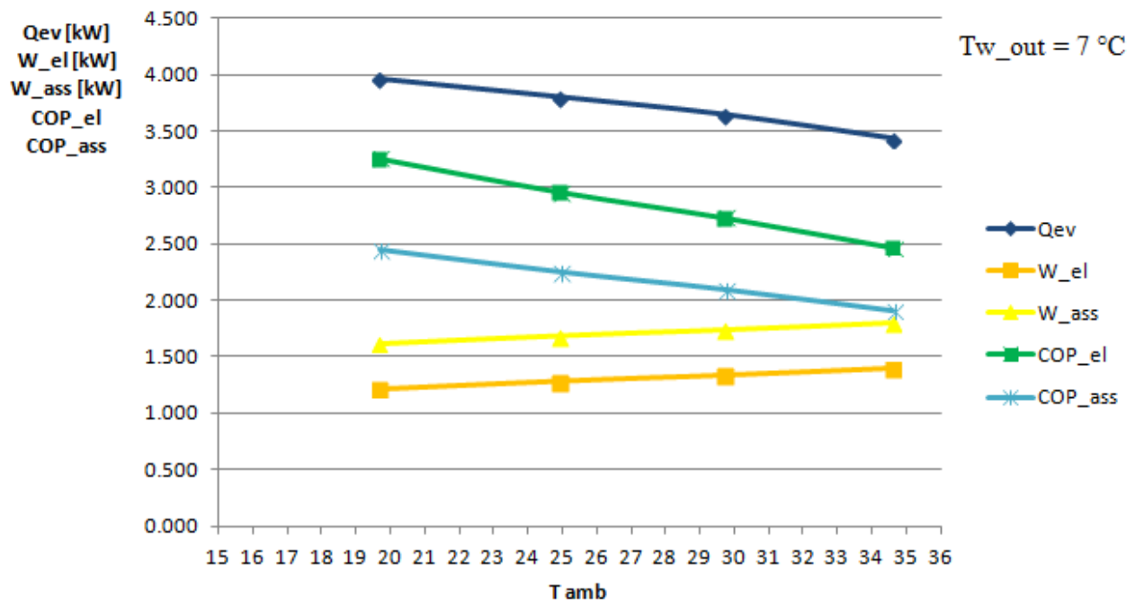
Fig. 6.1: Andamento della \dot{Q}_{ev} , W_{el} , W_{ass} , COP_{el} , COP_{ass} al variare della temperatura ambiente per una fissata temperature dell'acqua in uscita dallo scambiatore per il prototipo operante con R134a in modalità macchina frigorifera.
