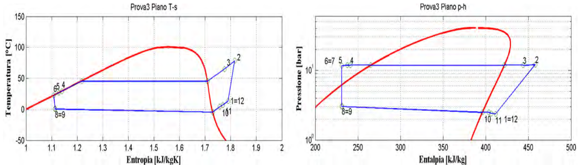
Figura 2.5: Piani T-s e p-h per la prova effettuata nelle condizioni 3 in modalità pompa di calore per il prototipo operante con R134a.
