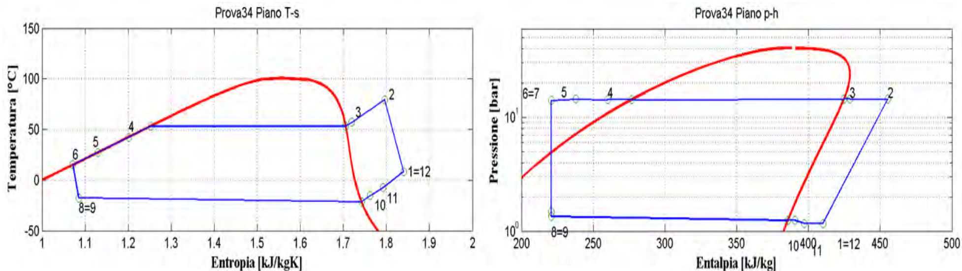
Figura 2.36: Piani T-s e p-h per la prova effettuata nelle condizioni 34 in modalità pompa di calore per il prototipo operante con R134a.
