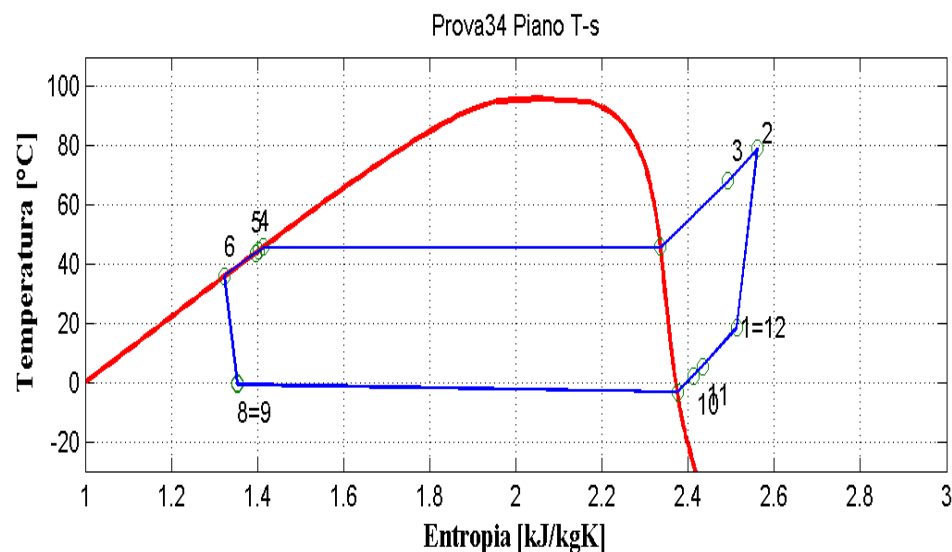
Figura 9.35: Piani T-s e p-h per la prova effettuata nelle condizioni 34 in modalità pompa di calore per il prototipo operante con R290.
