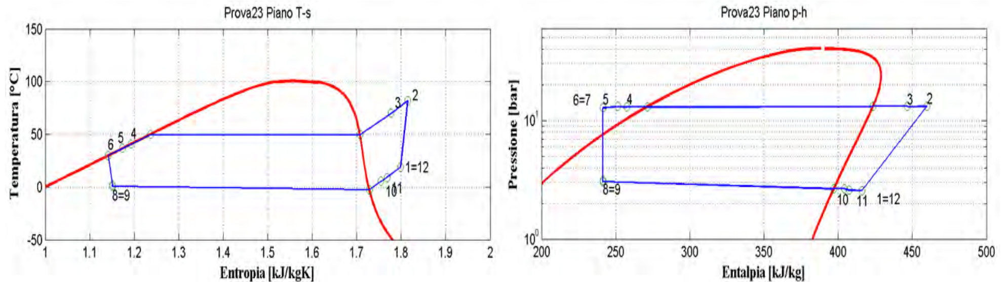
Figura 2.25: Piani T-s e p-h per la prova effettuata nelle condizioni 23 in modalità pompa di calore per il prototipo operante con R134a.
