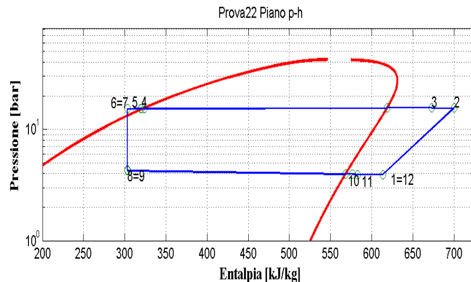
Figura 9.23: Piani T-s e p-h per la prova effettuata nelle condizioni 22 in modalità pompa di calore per il prototipo operante con R290.
