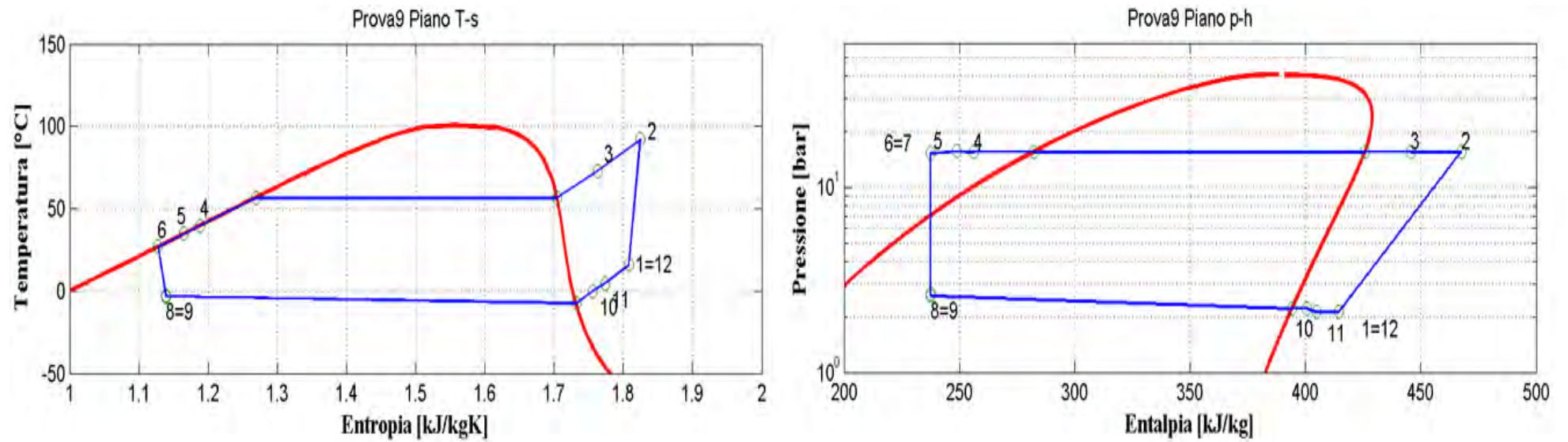
Figura 2.11: Piani T-s e p-h per la prova effettuata nelle condizioni 9 in modalità pompa di calore per il prototipo operante con R134a.
