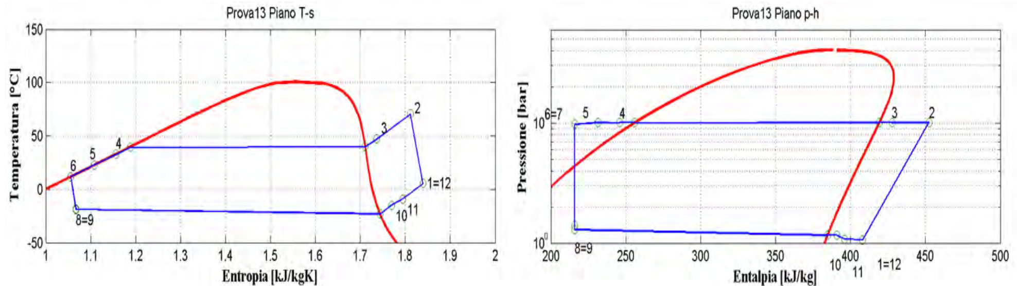
Figura 2.15: Piani T-s e p-h per la prova effettuata nelle condizioni 13 in modalità pompa di calore per il prototipo operante con R134a.
