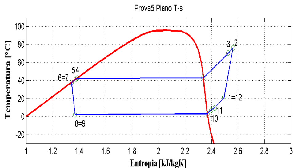
Figura 9.46: Piani T-s e p-h per la prova effettuata nelle condizioni 5 in modalità macchina frigorifera per il prototipo a propano (R290).
