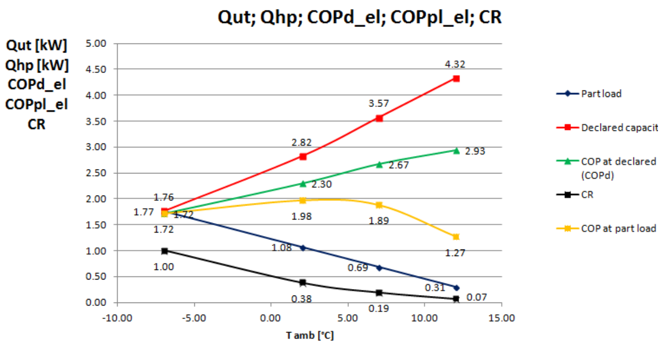
Figura 4.4: Andamento in funzione della temperatura esterna della potenza termica fornita dalla pompa di calore a R134a (in rosso), della potenza richiesta dall'utenza (in blu), del rapporto di capacità CR (in nero), del COP dichiarato della pompa di calore (in verde) e del COP a carico parziale (in giallo) questi ultimi valutati considerando come spesa energetica la potenza elettrica assorbita dal solo compressore.
