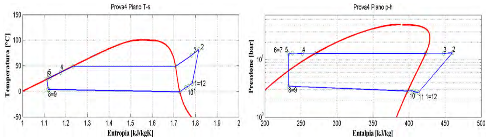
Figura 2.6: Piani T-s e p-h per la prova effettuata nelle condizioni 4 in modalità pompa di calore per il prototipo operante con R134a.
