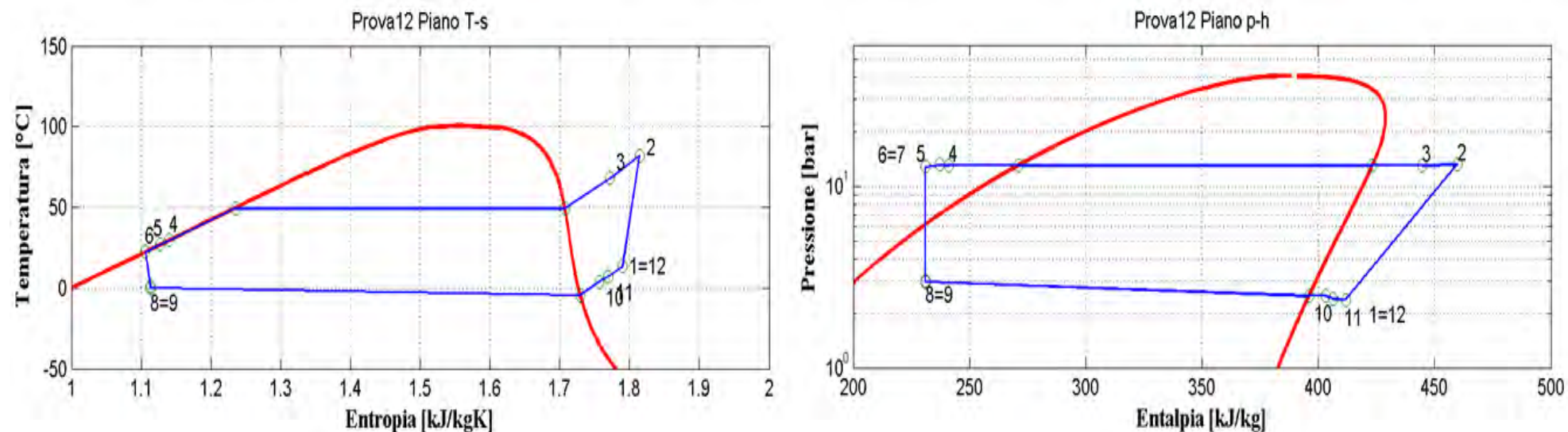
Figura 2.14: Piani T-s e p-h per la prova effettuata nelle condizioni 12 in modalità pompa di calore per il prototipo operante con R134a.
