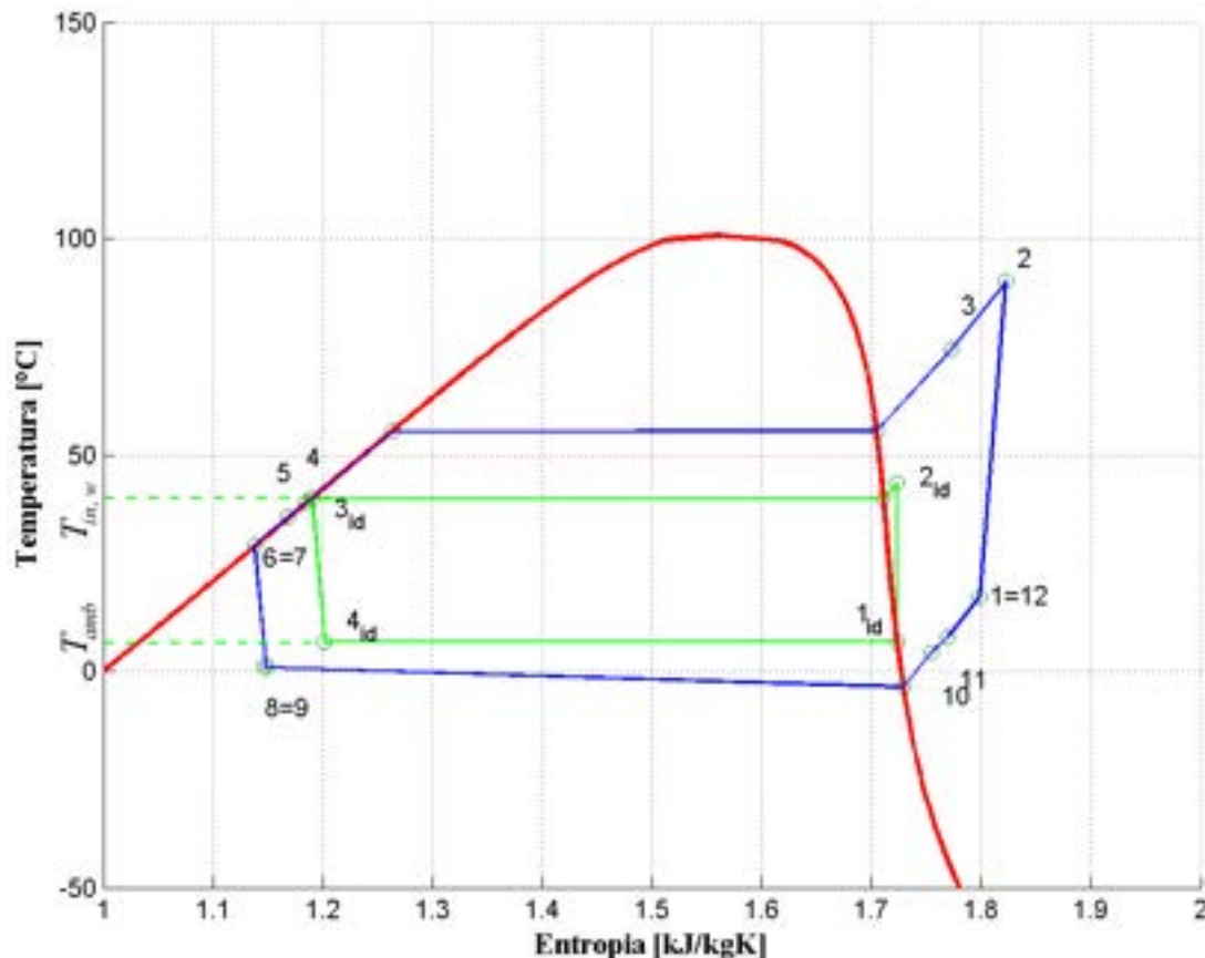
Figura 17.1: Confronto sul piano T-s tra il ciclo reale (in blu), ottenuto considerando componenti e fluido reali, e il ciclo ideale (in verde), ottenuto considerando compressore e scambiatori di calore ideali e pressioni di condensazione ed evaporazione corrispondenti alle temperature al contorno, nel caso di pompa di calore
