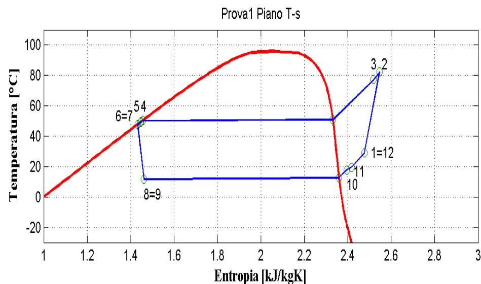
Figura 9.42: Piani T-s e p-h per la prova effettuata nelle condizioni 1 in modalità macchina frigorifera per il prototipo a propano (R290).
