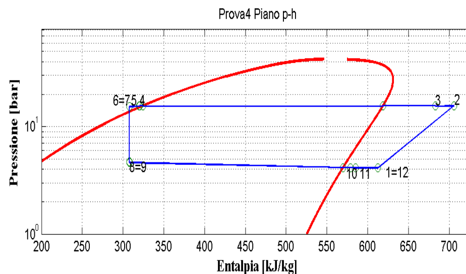
Figura 9.5: Piani T-s e p-h per la prova effettuata nelle condizioni 4 in modalità pompa di calore per il prototipo operante con R290.
