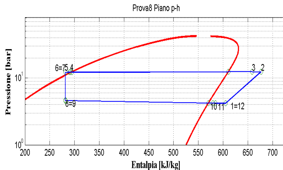
Figura 9.9: Piani T-s e p-h per la prova effettuata nelle condizioni 8 in modalità pompa di calore per il prototipo operante con R290.
