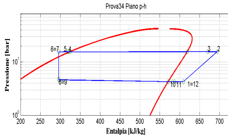
Figura 9.35: Piani T-s e p-h per la prova effettuata nelle condizioni 34 in modalità pompa di calore per il prototipo operante con R290.
