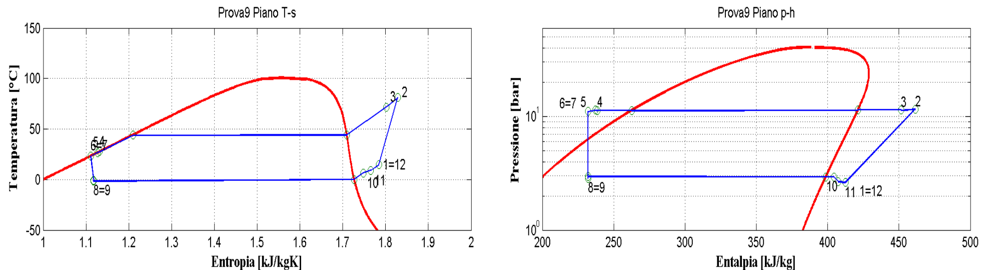
Figura 2.51: Piani T-s e p-h per la prova effettuata nelle condizioni 9 in modalità macchina frigorifera per il prototipo elaborante R134a.
