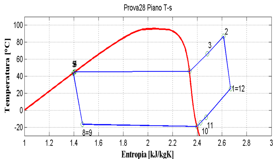
Figura 9.29: Piani T-s e p-h per la prova effettuata nelle condizioni 28 in modalità pompa di calore per il prototipo operante con R290.
