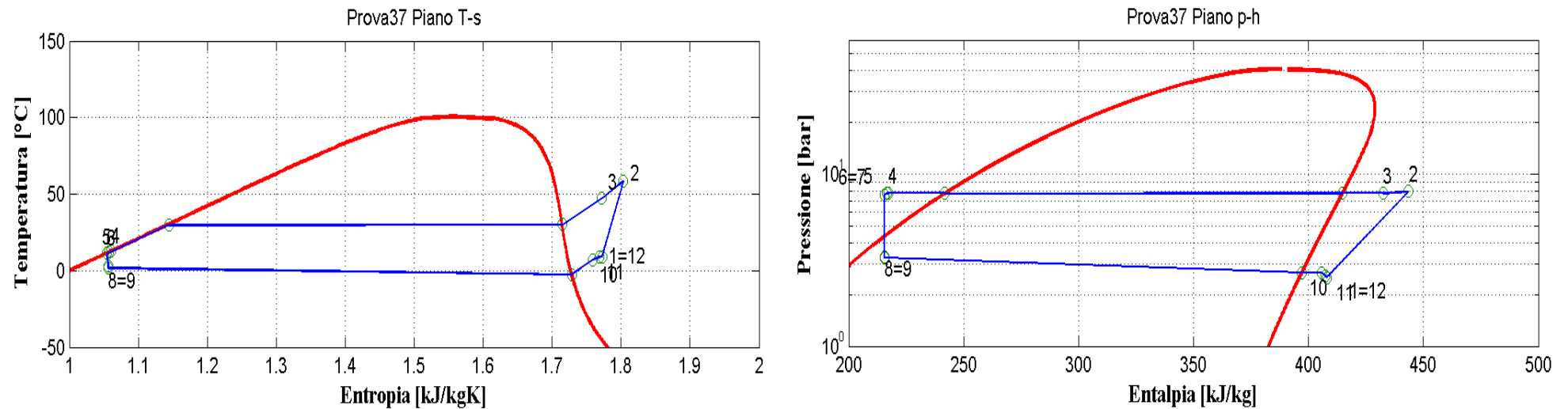
Figura 2.39: Piani T-s e p-h per la prova effettuata nelle condizioni 37 in modalità pompa di calore per il prototipo operante con R134a.
