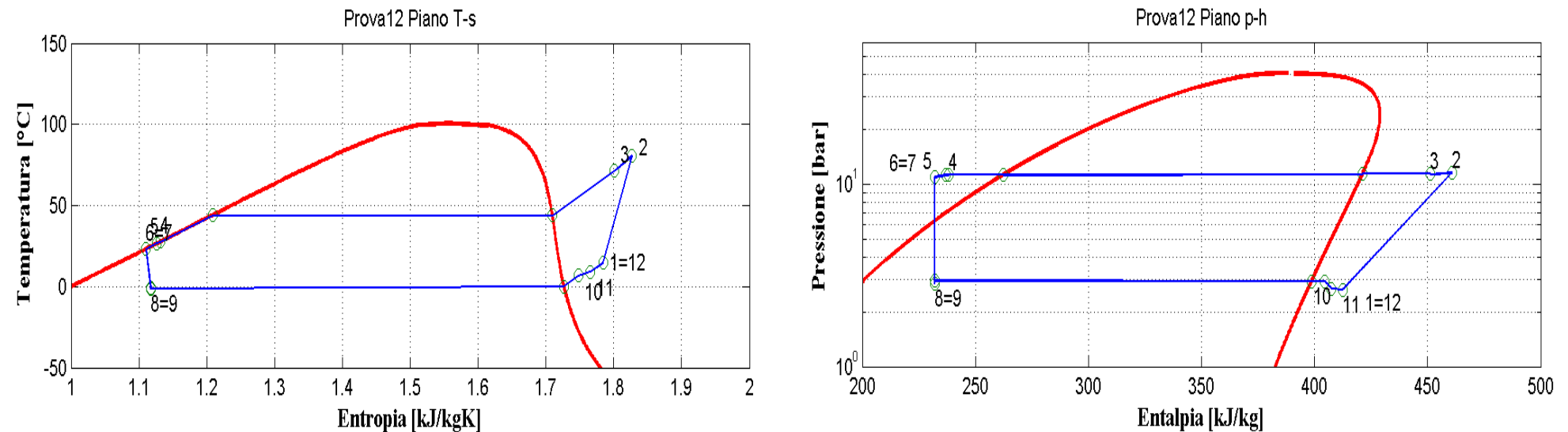
Figura 2.54: Piani T-s e p-h per la prova effettuata nelle condizioni 12 in modalità macchina frigorifera per il prototipo elaborante R134a.
