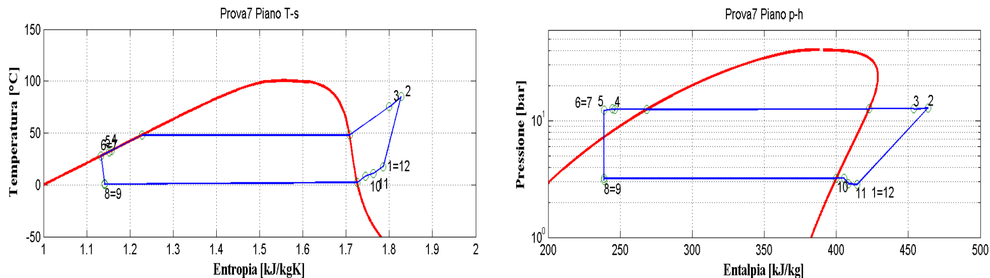
Figura 2.49: Piani T-s e p-h per la prova effettuata nelle condizioni 7 in modalità macchina frigorifera per il prototipo elaborante R134a.
