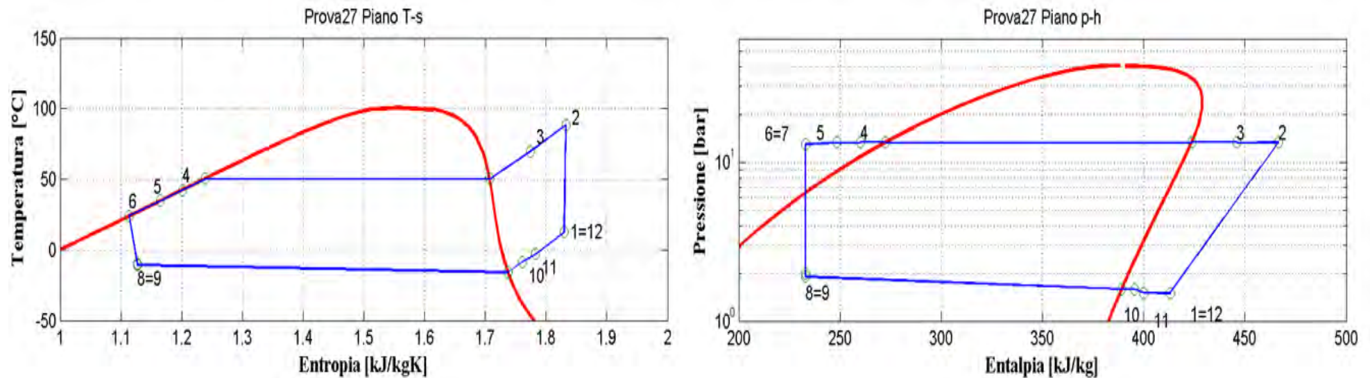
Figura 2.29: Piani T-s e p-h per la prova effettuata nelle condizioni 27 in modalità pompa di calore per il prototipo operante con R134a.
