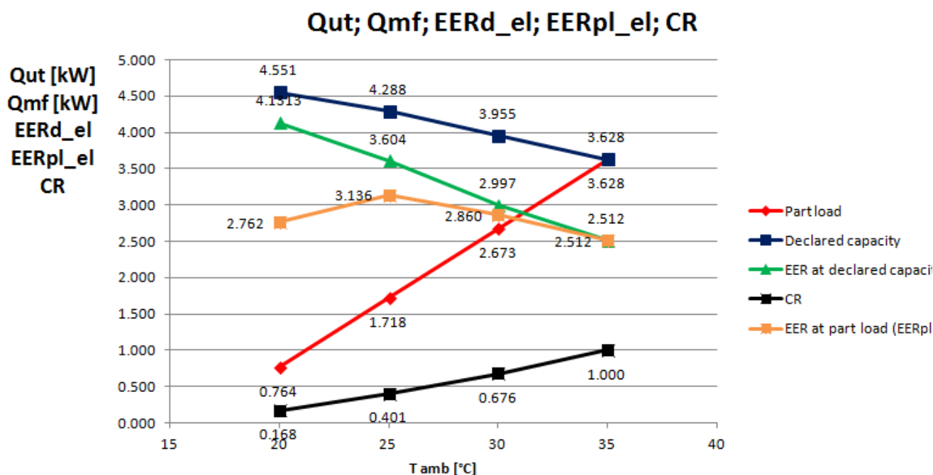
Figura 13.4: Andamento in funzione della temperatura esterna della potenza frigorifera fornita dalla macchina frigo a propano (in blu), della potenza richiesta dall'utenza (in rosso), del rapporto di capacità CR (in nero), dell'EER dichiarato della macchina frigo (in verde) e dell'EER a carico parziale (in arancione), questi ultimi valutati considerando come spesa energetica la potenza elettrica assorbita dal solo compressore
