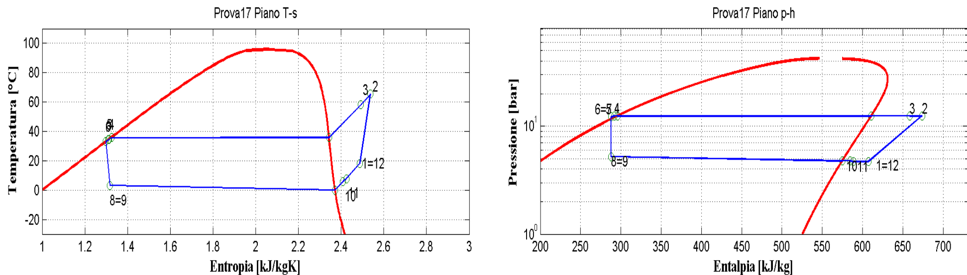
Figura 9.18: Piani T-s e p-h per la prova effettuata nelle condizioni 17 in modalità pompa di calore per il prototipo operante con R290.
