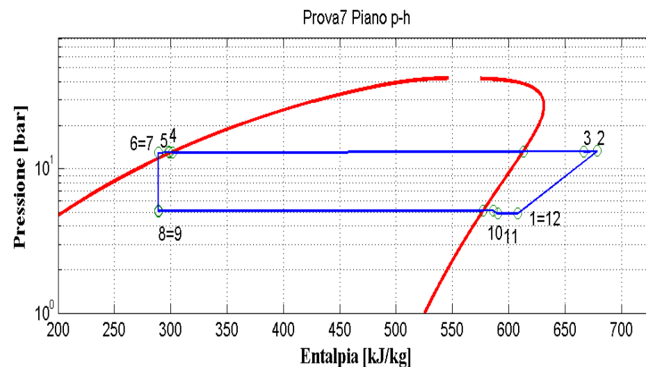
Figura 9.48: Piani T-s e p-h per la prova effettuata nelle condizioni 7 in modalità macchina frigorifera per il prototipo a propano (R290).
