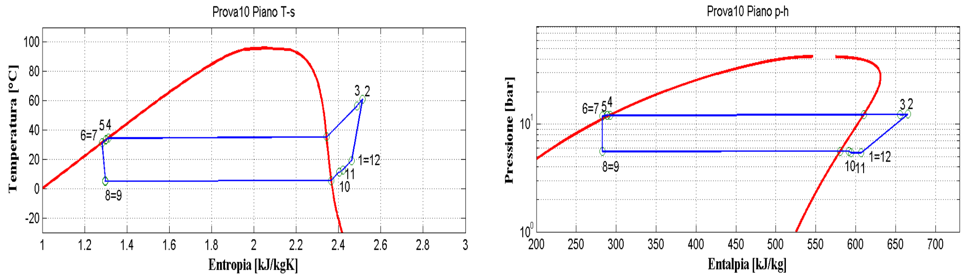
Figura 9.51: Piani T-s e p-h per la prova effettuata nelle condizioni 10 in modalità macchina frigorifera per il prototipo a propano (R290).
