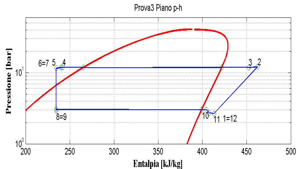
Figura 2.45: Piani T-s e p-h per la prova effettuata nelle condizioni 3 in modalità macchina frigorifera per il prototipo elaborante R134a.
