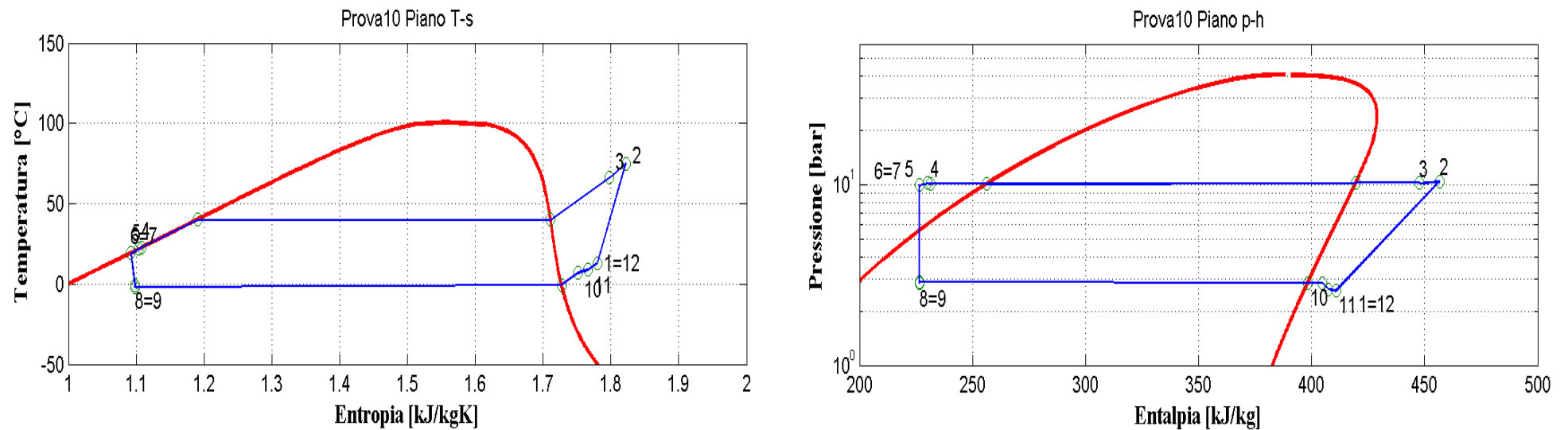
Figura 2.52: Piani T-s e p-h per la prova effettuata nelle condizioni 10 in modalità macchina frigorifera per il prototipo elaborante R134a.
