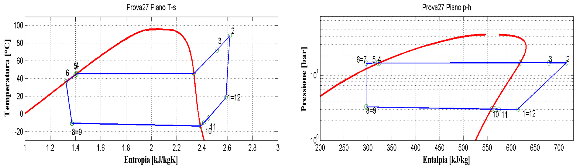
Figura 9.28: Piani T-s e p-h per la prova effettuata nelle condizioni 27 in modalità pompa di calore per il prototipo operante con R290.
