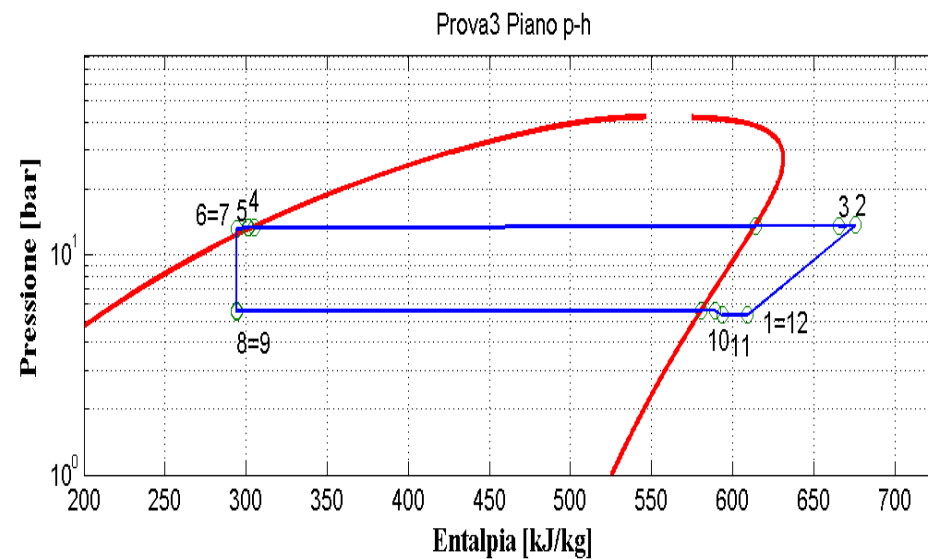
Figura 9.44: Piani T-s e p-h per la prova effettuata nelle condizioni 3 in modalità macchina frigorifera per il prototipo a propano (R290).
