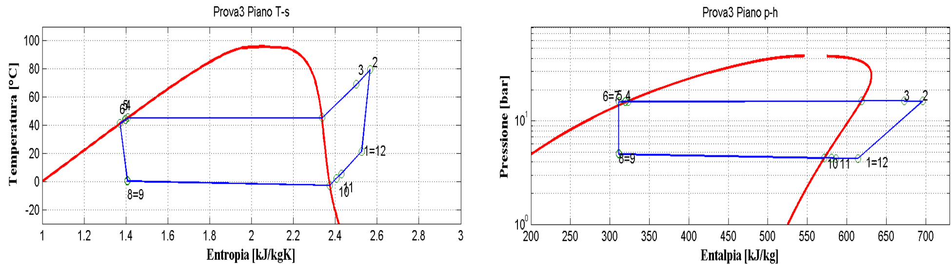
Figura 9.4: Piani T-s e p-h per la prova effettuata nelle condizioni 3 in modalità pompa di calore per il prototipo operante con R290.
