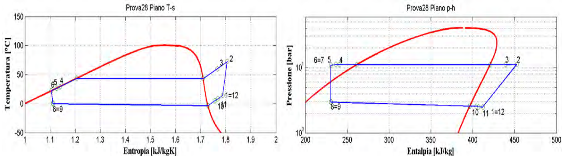
Figura 2.30: Piani T-s e p-h per la prova effettuata nelle condizioni 28 in modalità pompa di calore per il prototipo operante con R134a.
