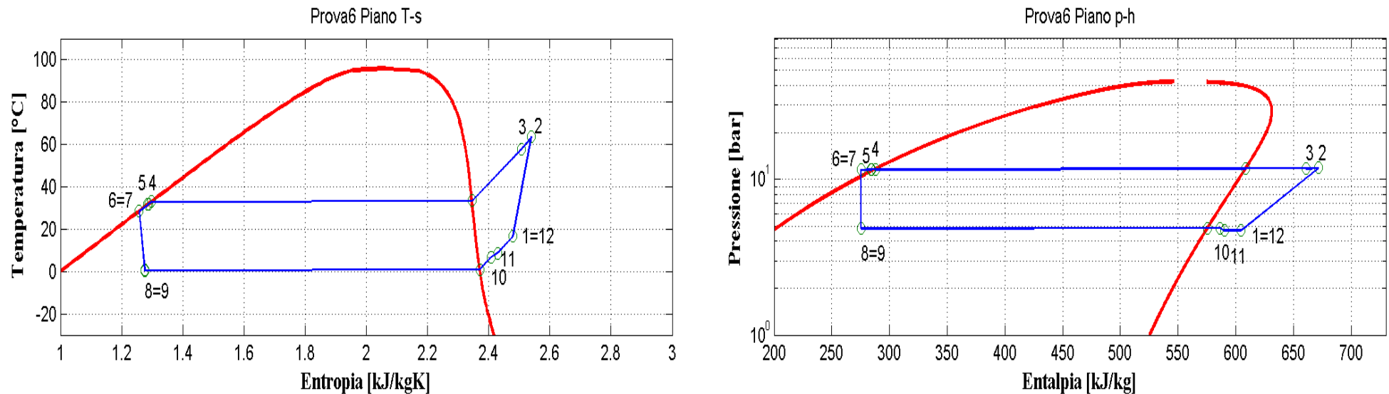
Figura 9.47: Piani T-s e p-h per la prova effettuata nelle condizioni 6 in modalità macchina frigorifera per il prototipo a propano (R290).
