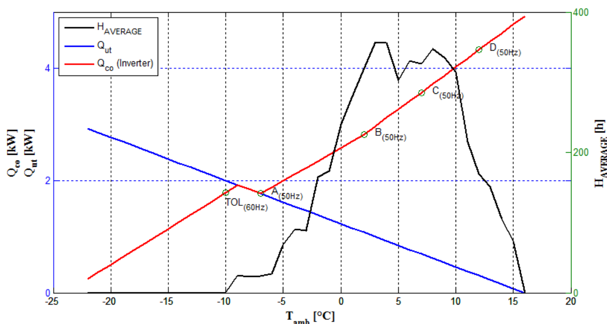
Figura 8.10: Andamento in funzione della temperatura esterna della potenza termica fornita dalla pompa di calore elaborante R134a con compressore funzionante con inverter tra 60 e 50 Hz (in rosso), quella richiesta dall'utenza (in blu), ed il numero di ore corrispondenti ad ogni bins.
