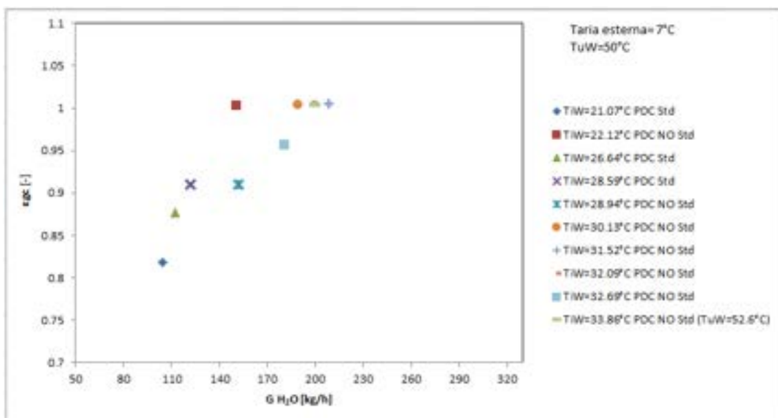
Figura 48. Efficienza del gas cooler in funzione della portata d'acqua.
