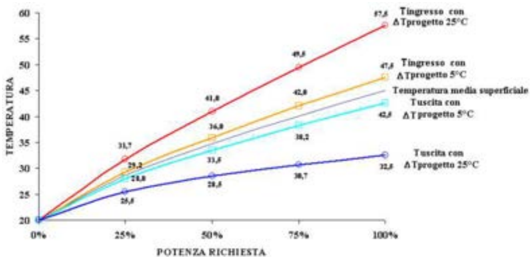
Figura 8. Andamento delle temperature di ingresso e di uscita in funzione del salto termico \Delta T .
