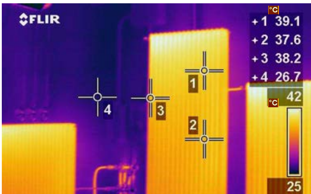
Figura 37. Analisi termografica dei terminali d'impianto installati.
