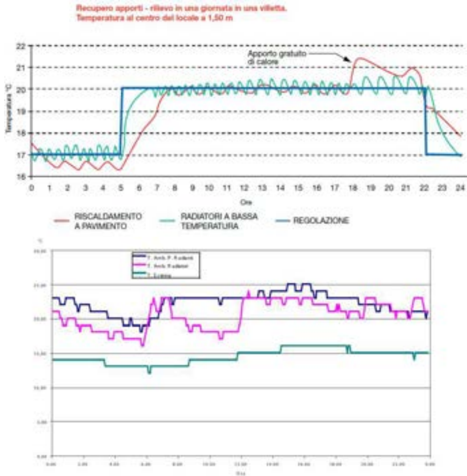
Figura 14. Andamento della temperatura ambiente con impianto a pannelli radianti e con impianto a radiatori in due differenti campagne di prova.
