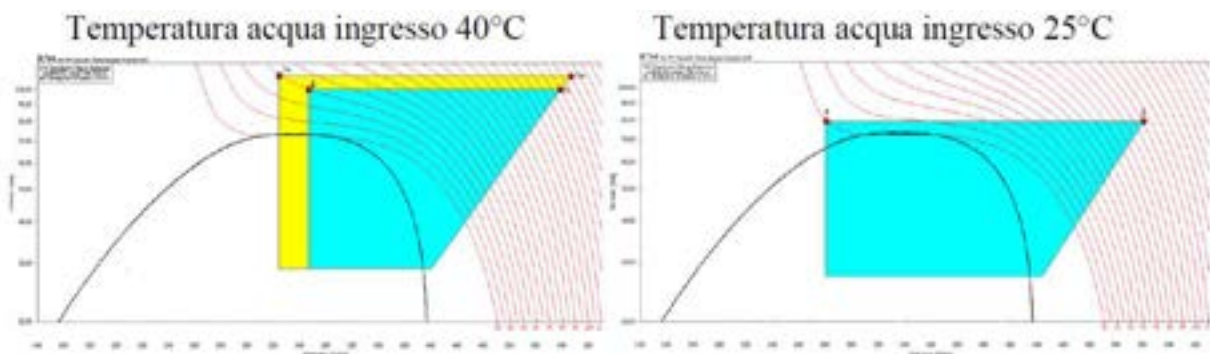
Figura 3. Cicli termodinamici per due diverse temperature dell'acqua in ingresso al gas cooler.
