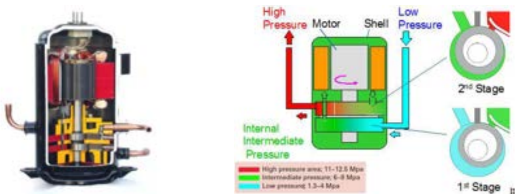
Figura 21. Compressore bistadio per CO 2
