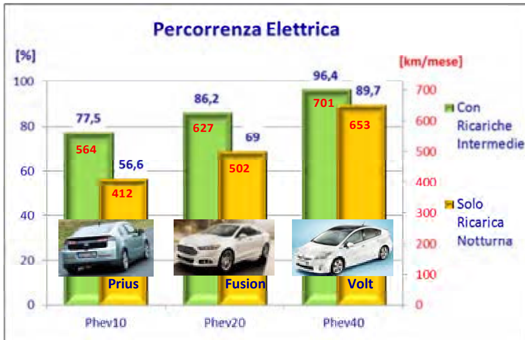
Figura 17 – Percorrenze elettriche in percentuale del totale ed in km percorsi nel mese per i 3 tipi di plug-in considerati. I valori mostrati sono ottenuti con ricarica solo notturna (giallo) e con ricariche intermedie (verde).
