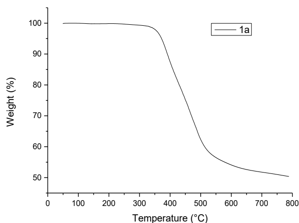
Figura 5. Analisi TGA per il polimero 1a.
