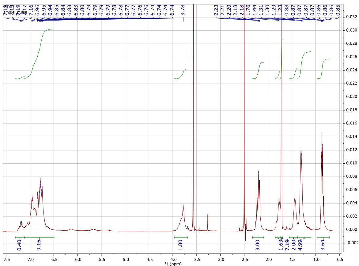
Figura 11. ^1\text{H} -NMR del polimero 1b.
