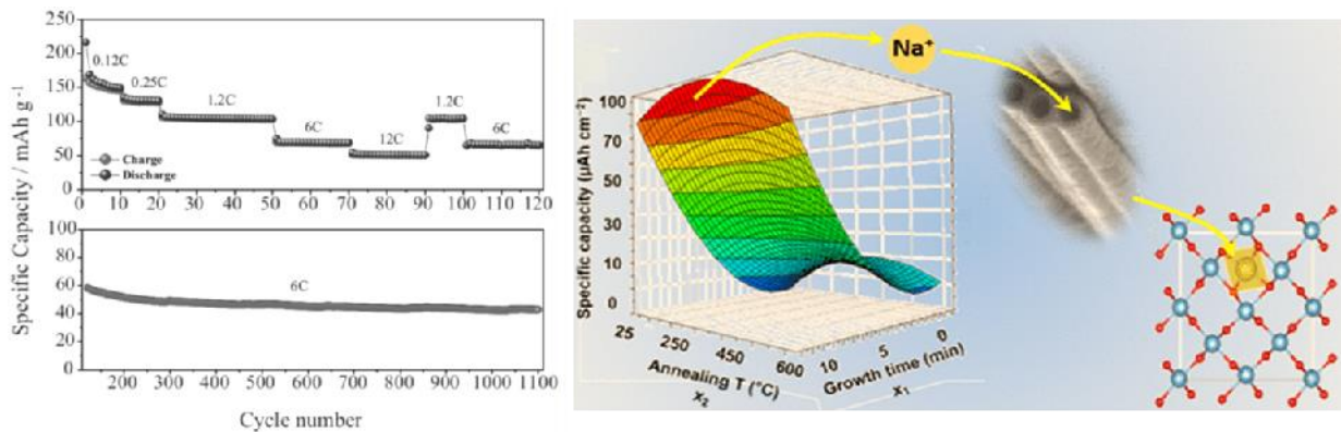
Figura 2. Sulla sinistra, ciclazione galvanostatica dei nanotubi di \text{TiO}_2 trattati a 450\text{ }^\circ\text{C} (fase anatasio) in cella su scala da laboratorio; sulla destra analisi computazionale mediante chemiometria e calcoli DFT.
