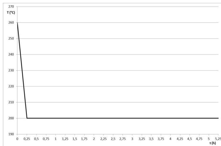
Figura 3- Andamento della temperatura del fluido termovettore nella fase di scarica
