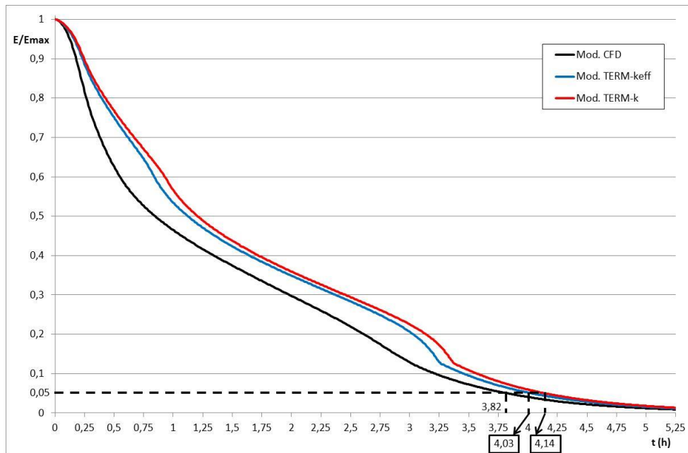
Figura 41- Fase di scarica - Energie termiche scaricate normalizzate con indicazione di t_{E5\%}
