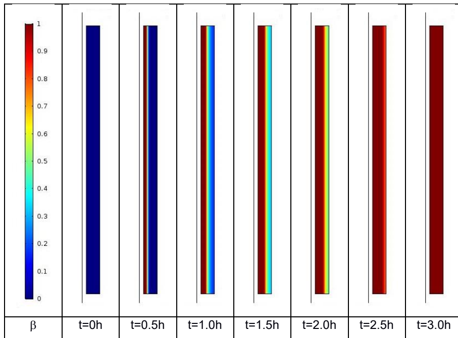
Figura 33- Mod. TERM-k, fase di carica - Frazione fusa del PCM in diversi istanti
