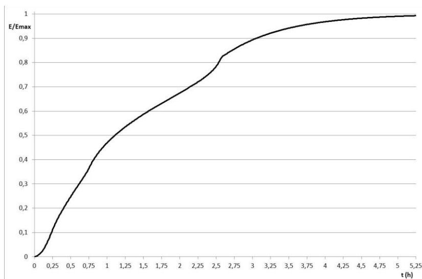
Figura 31- Mod. TERM-k, fase di carica - Evoluzione temporale dell'energia termica totale accumulata dal PCM, normalizzata
