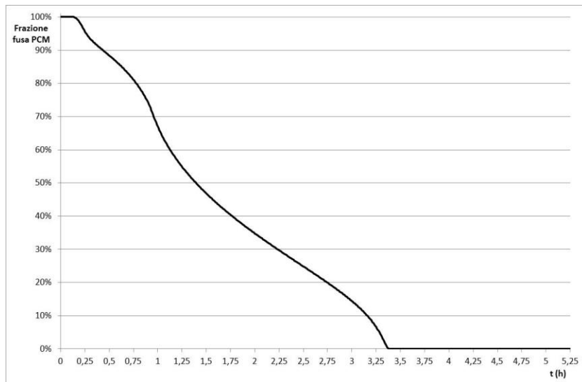
Figura 34- Mod. TERM-k, fase di scarica - Evoluzione temporale della frazione percentuale di massa fusa di PCM
