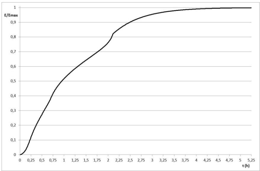
Figura 23- Mod. TERM-keff, fase di carica - Evoluzione temporale dell'energia termica totale accumulata dal PCM, normalizzata
