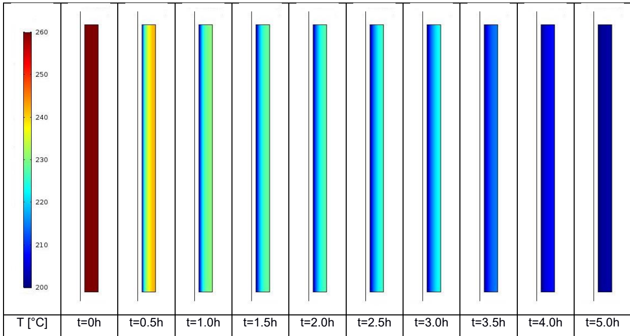
Figura 28- Mod. TERM-keff, fase di scarica - Campo termico nel PCM in diversi istanti
