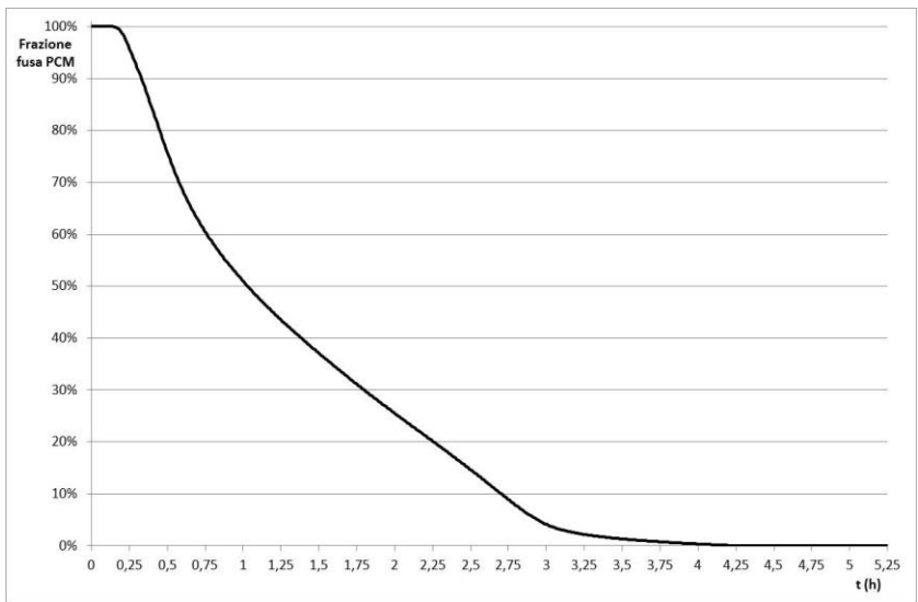
Figura 13- Mod. CFD, fase di scarica - Evoluzione temporale della frazione percentuale della massa fusa di PCM
