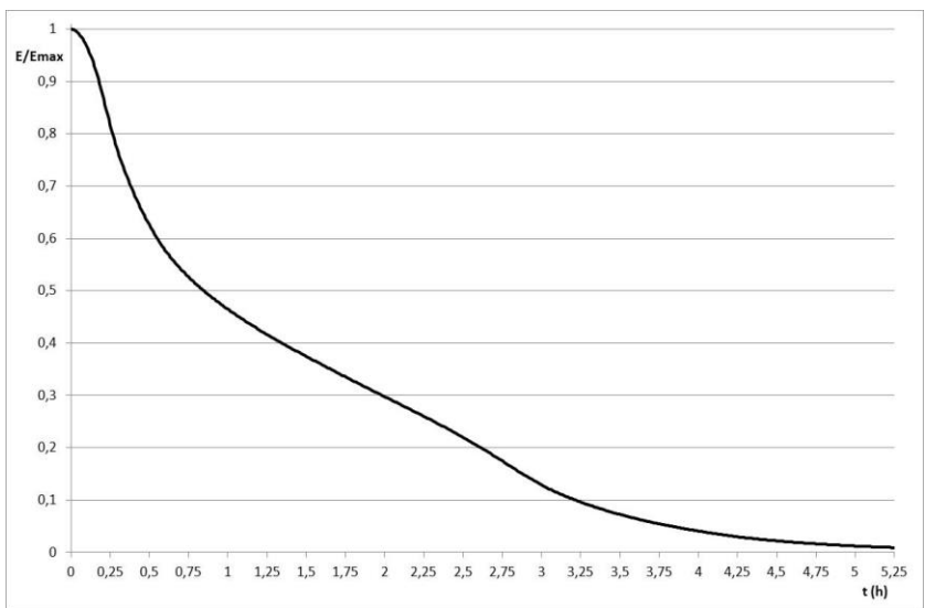
Figura 14- Mod. CFD, fase di scarica - Evoluzione temporale dell'energia termica totale accumulata dal PCM normalizzata
