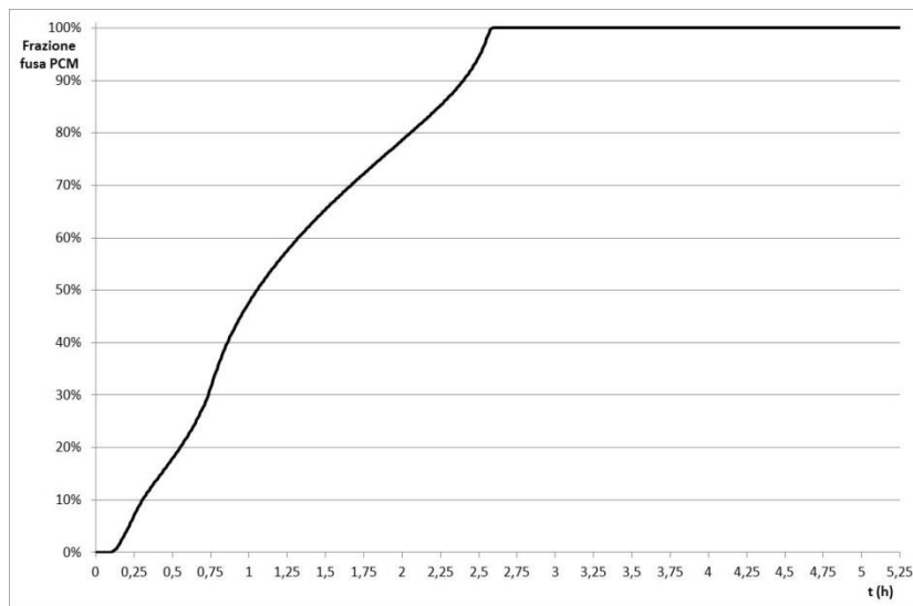
Figura 30- Mod. TERM-k, fase di carica - Evoluzione temporale della frazione percentuale della massa fusa di PCM
