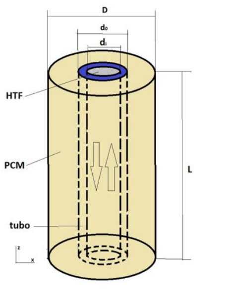
Figura 1- Singola unità cilindrica verticale di un sistema LHTES del tipo tube-and-shell
