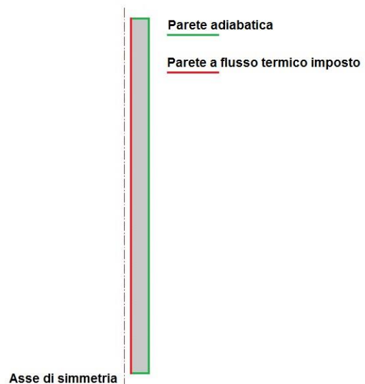
Figura 5- Mod. CFD - Condizioni al contorno
