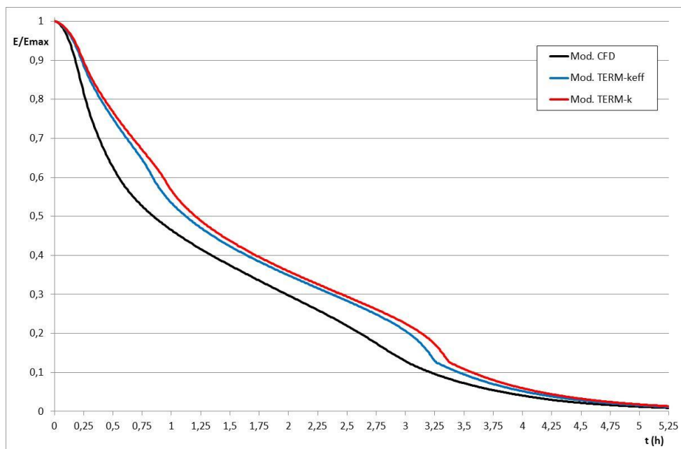
Figura 39- Fase di scarica - Andamento temporale delle energie termiche scaricate normalizzate, nei tre modelli
