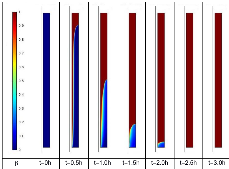
Figura 11- Mod. CFD, fase di carica - Frazione fusa del PCM in diversi istanti
