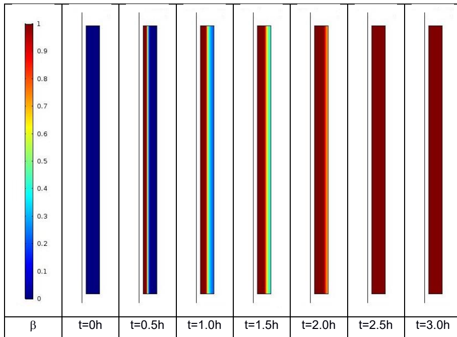
Figura 25- Mod. TERM-keff, fase di carica - Frazione fusa del PCM in diversi istanti
