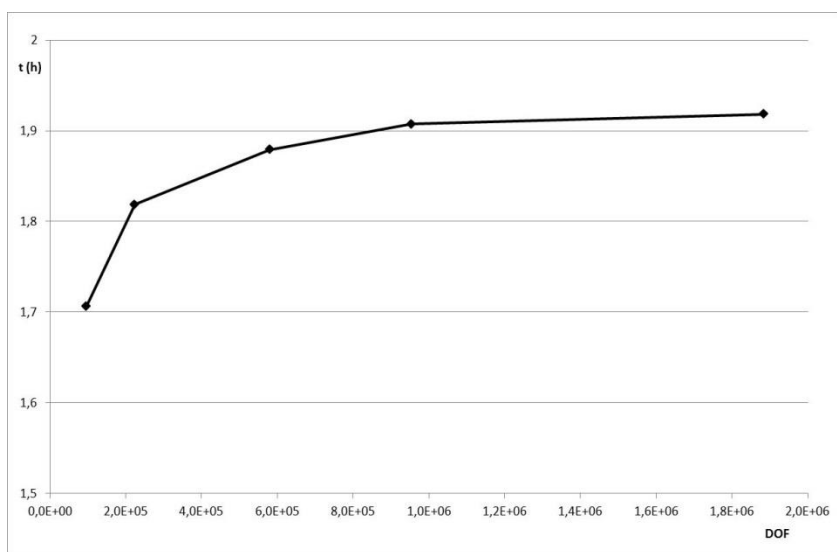
Figura 6- Andamento del tempo di carica t_{E95\%} in funzione del numero di gradi di libertà (DoF)
