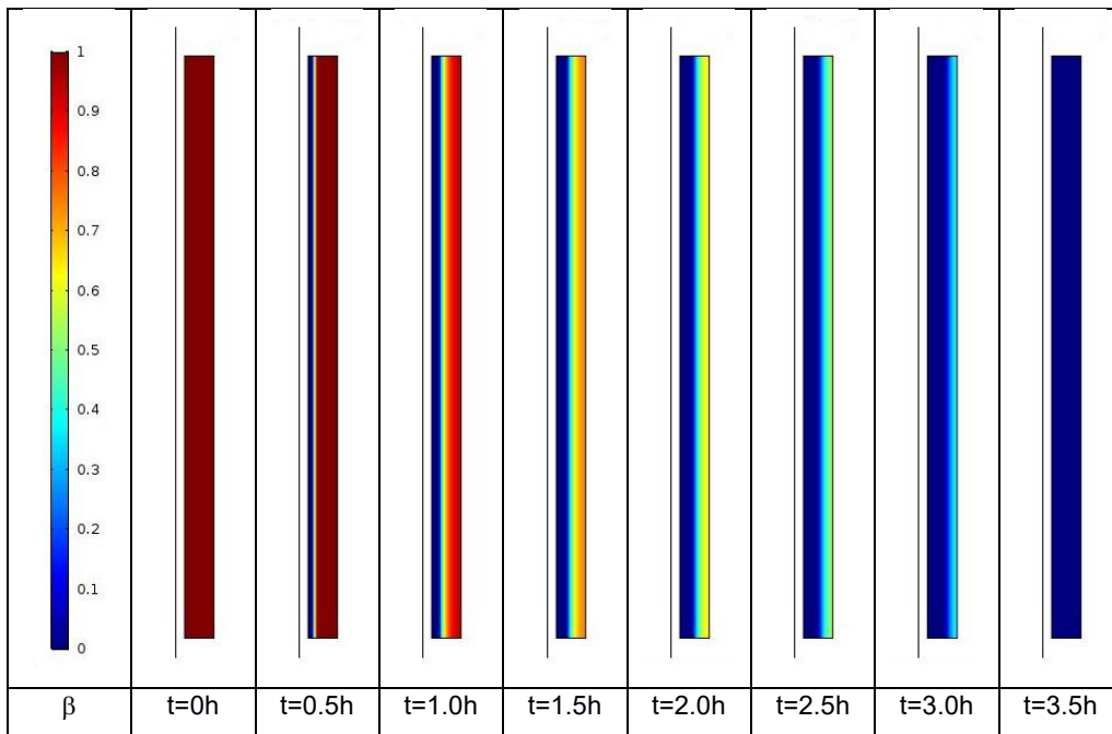
Figura 37- Mod. TERM-k, fase di scarica - Frazione fusa del PCM in diversi istanti
