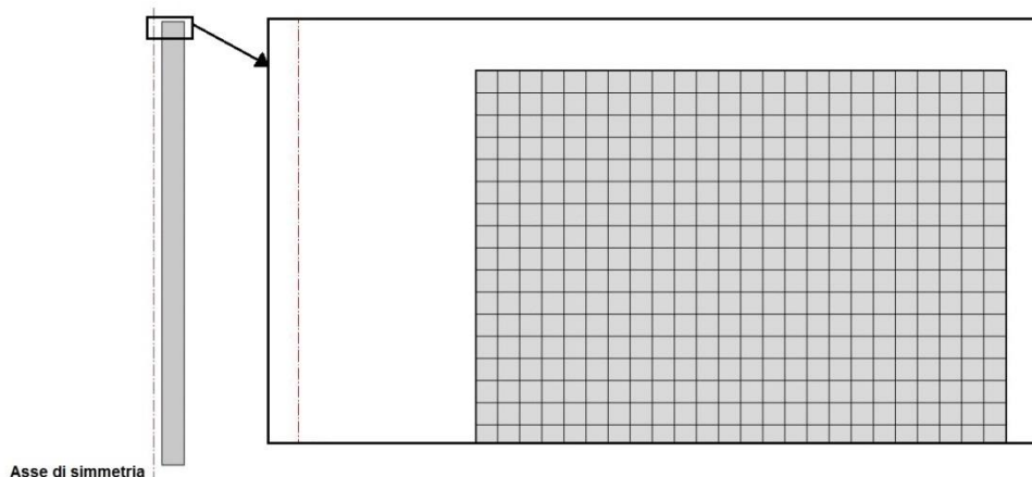
Figura 21- Mod. TERM-keff - Particolare del mesh
