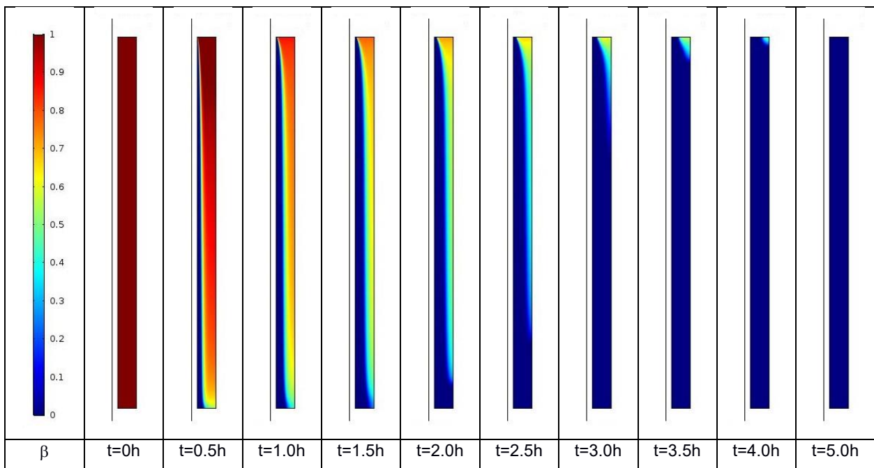
Figura 16- Mod. CFD, fase di scarica - Frazione fusa del PCM in diversi istanti
