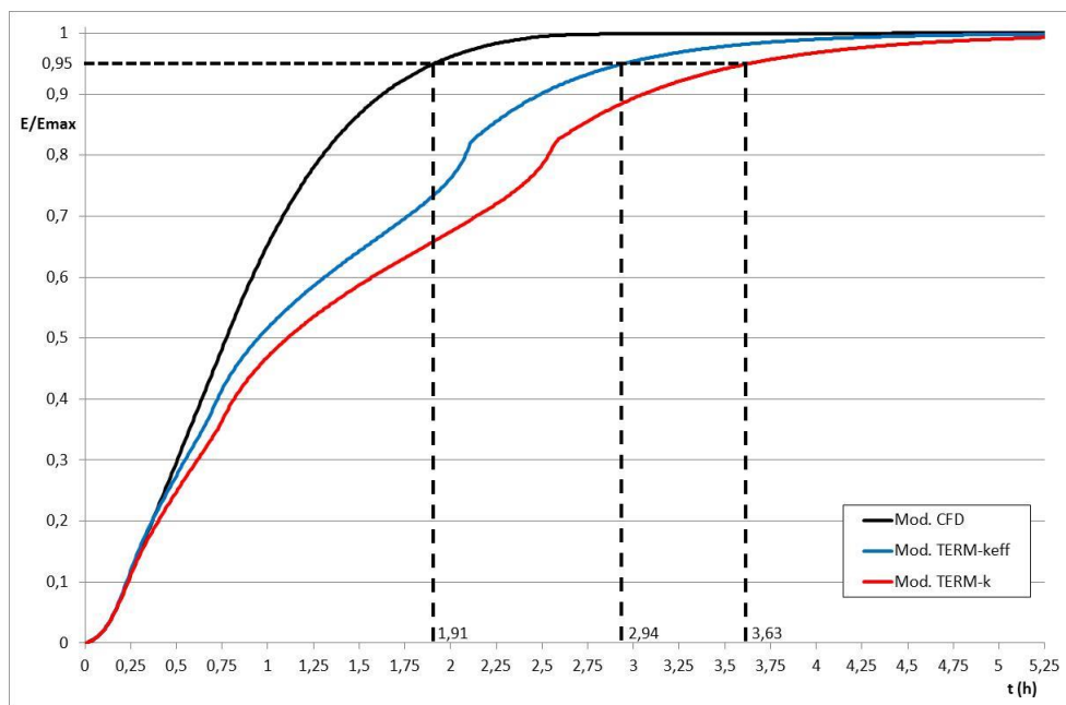
Figura 40- Fase di carica - Energie termiche accumulate normalizzate con indicazione di t_{E95\%}
