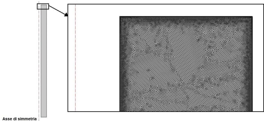
Figura 7- Mod. CFD - Particolare del mesh
