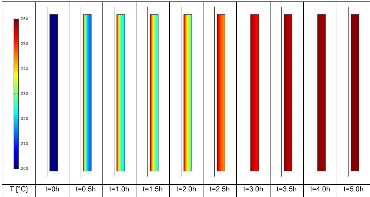
Figura 24- Mod. TERM-keff, fase di carica - Campo termico nel PCM in diversi istanti
