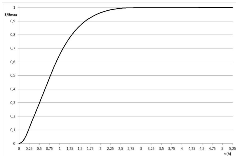
Figura 9- Mod. CFD, fase di carica - Evoluzione temporale dell'energia termica totale accumulata dal PCM normalizzata
