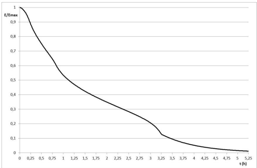
Figura 27- Mod. TERM-keff, fase di scarica - Evoluzione temporale dell'energia termica totale accumulata dal PCM, normalizzata
