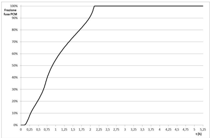
Figura 22- Mod. TERM-keff, fase di carica - Evoluzione temporale della frazione percentuale della massa fusa di PCM
