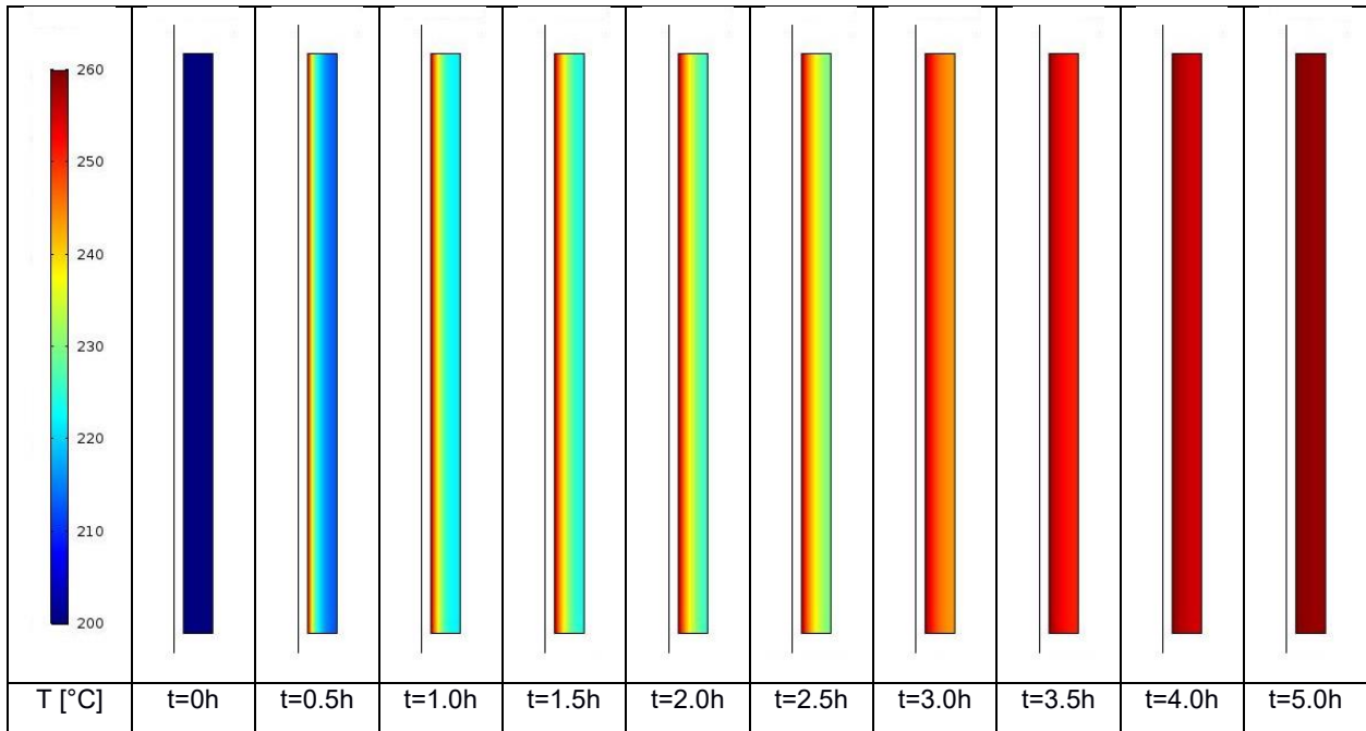
Figura 32- Mod. TERM-k, fase di carica - Campo termico nel PCM in diversi istanti
