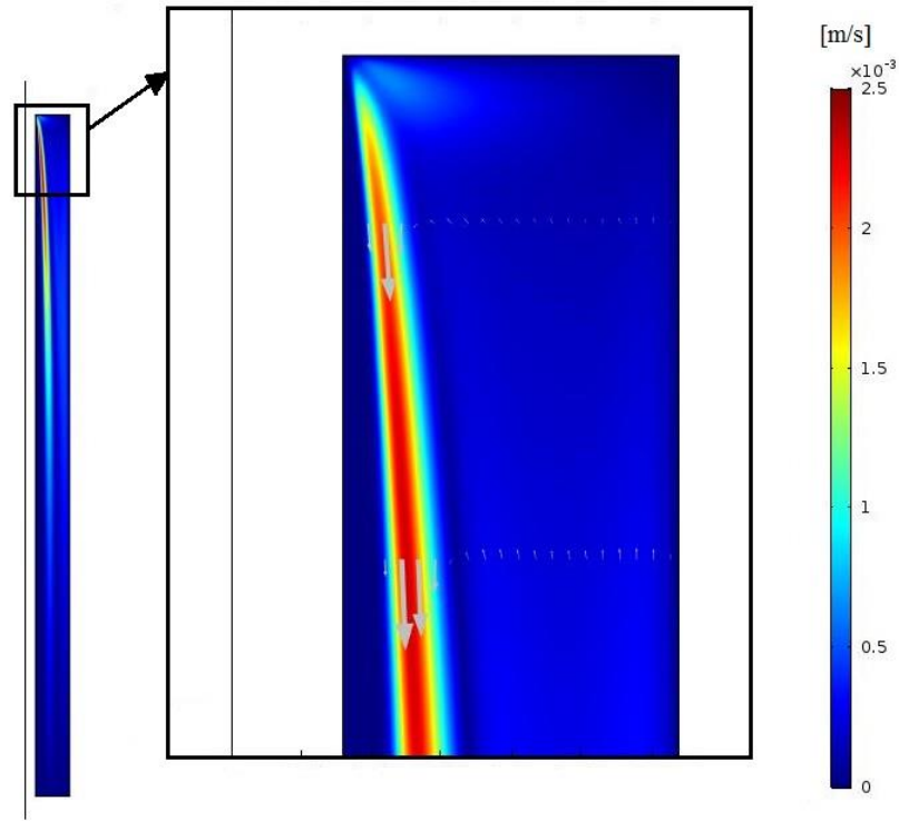
Figura 17- Mod. CFD, fase di scarica - Andamento delle velocità del PCM fuso all'istante t=1800 s
