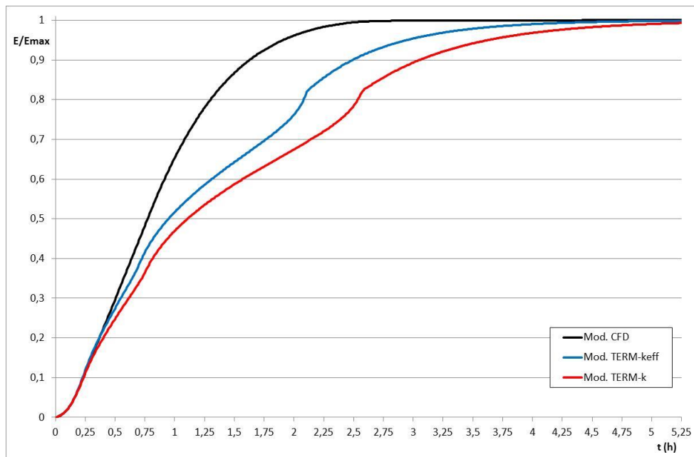
Figura 38- Fase di carica - Andamento temporale delle energie termiche accumulate normalizzate, nei tre modelli
