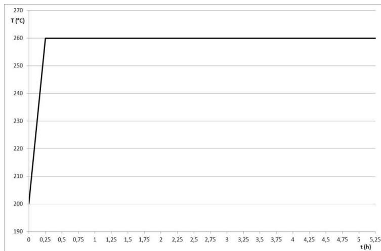
Figura 2- Andamento della temperatura del fluido termovettore nella fase di carica
