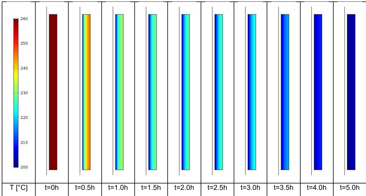
Figura 36- Mod. TERM-k, fase di scarica - Campo termico nel PCM in diversi istanti
