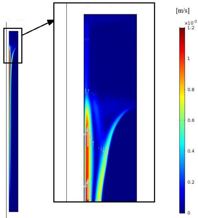
Figura 12- Mod. CFD, fase di carica - Andamento delle velocità del PCM fuso all'istante t=1800 s
