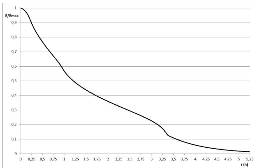
Figura 35- Mod. TERM-k, fase di scarica - Evoluzione temporale dell'energia termica totale accumulata dal PCM, normalizzata
