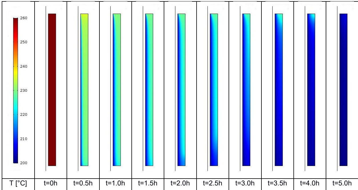
Figura 15- Mod. CFD, fase di scarica - Campo termico nel PCM in diversi istanti
