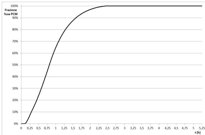
Figura 8- Mod. CFD, fase di carica - Evoluzione temporale della frazione percentuale della massa fusa di PCM
