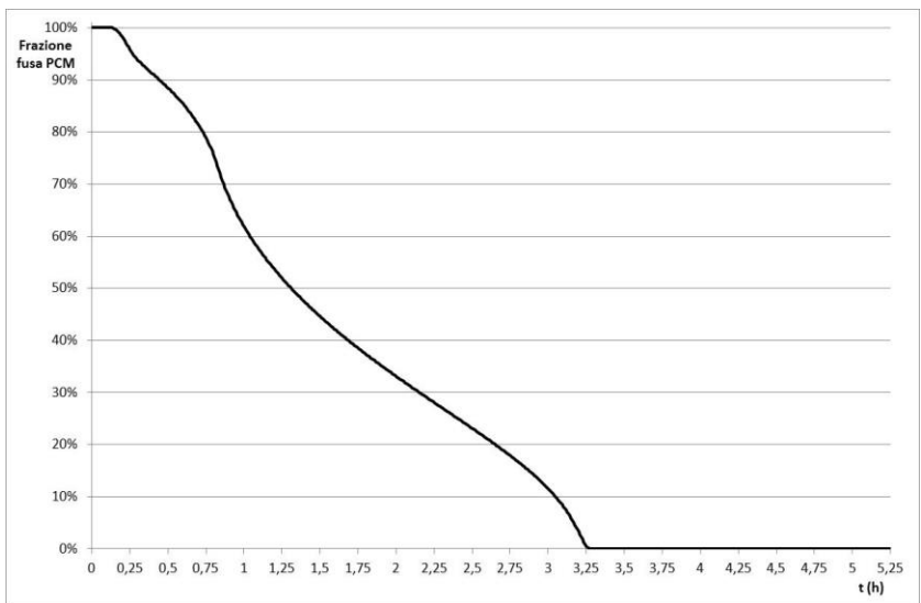
Figura 26- Mod. TERM-keff, fase di scarica - Evoluzione temporale della frazione percentuale della massa fusa di PCM
