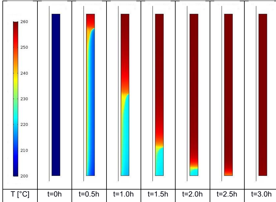
Figura 10- Mod. CFD, fase di carica - Campo termico nel PCM in diversi istanti
