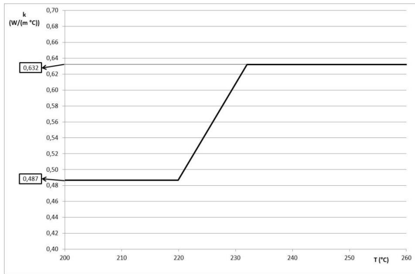
Figura 18- Mod. TERM-keff - Andamento di k del PCM in funzione della temperatura
