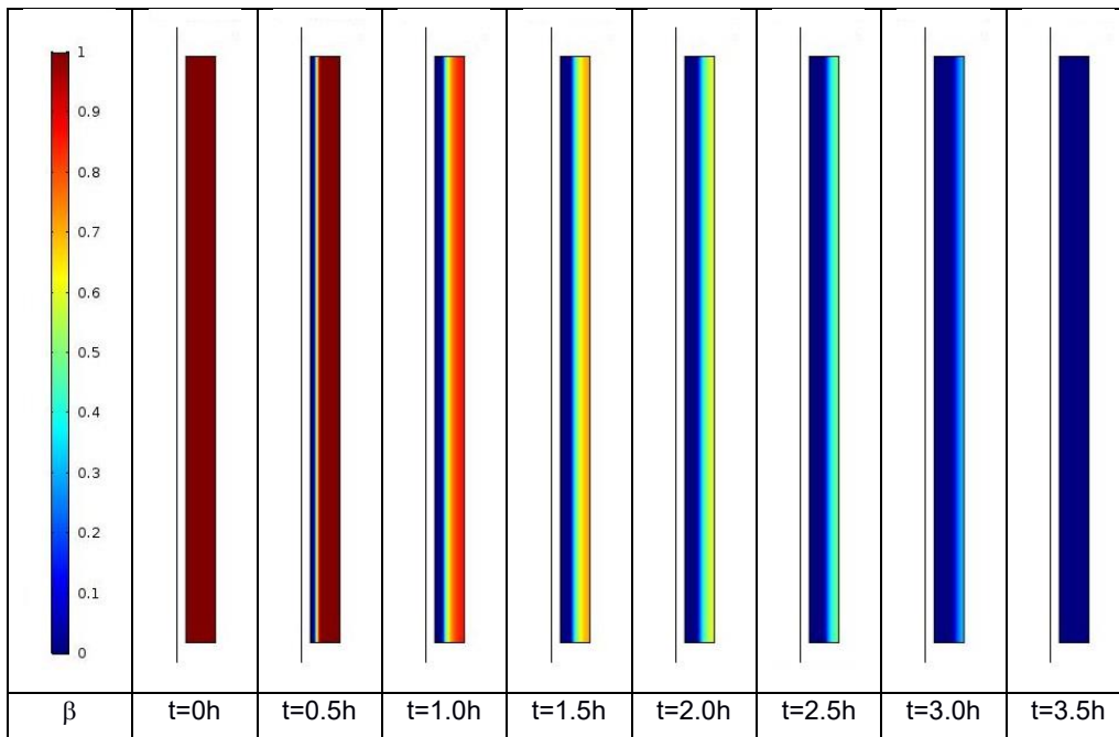
Figura 29- Mod. TERM-keff, fase di scarica - Frazione fusa del PCM in diversi istanti
