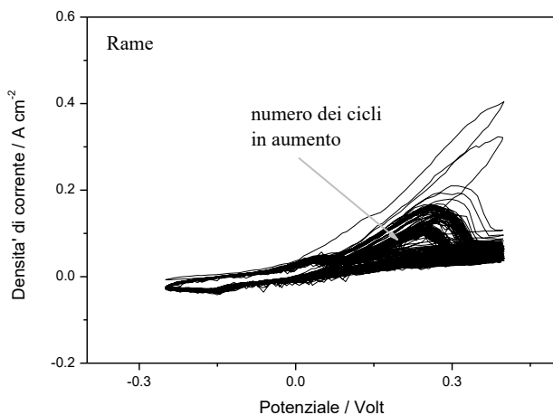
Figura 10 - Trattamento di condizionamento dell'elettrodo di rame. Scansione di potenziale fra -0.25V e +0.35V. Velocità di scansione 100 mV s -1 . Numero di cicli: 100.
