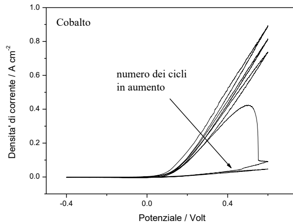
Figura 19 - Profilo voltammetrico del Cobalto dopo 4 ore di immersione. Scansione di potenziale fra -0.4V e +0.6V. Velocità di scansione: 5 mV s -1 . Numero di cicli: 5.
