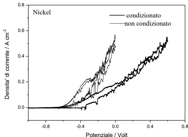
Figura 9 - Profilo voltammetrico del Nickel. Scansione di potenziale fra -1V e +0.6V (nickel condizionato) e fra -1V e 0 V (nickel non condizionato). Velocità di scansione: 5 mV s -1 . Numero di cicli: 2.
