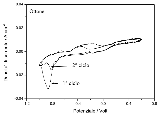
Figura 15 - Profilo voltammetrico dell'ottone dopo il trattamento di condizionamento. Scansione di potenziale fra -0.8V e +0.6V. Velocità di scansione: 5 mV s -1 . Numero di cicli: 2.
