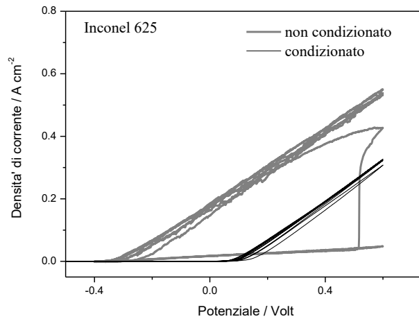
Figura 27 – Effetto del condizionamento sul profilo voltammetrico dell’Inconel 625 dopo 4 ore di immersione. Scansione di potenziale fra -0.6V e +0.6V. Velocità di scansione: 5 \text{ mV s}^{-1} . Numero di cicli: 5.
