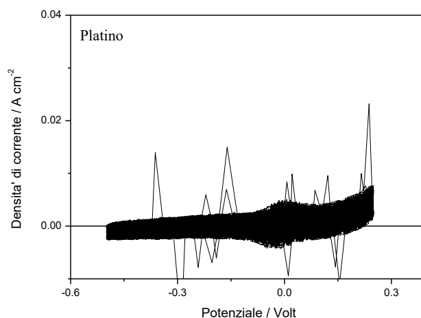
Figura 3 – Trattamento di condizionamento dell'elettrodo di platino. Scansione di potenziale fra -0.5V e +0.25V. Velocità di scansione 100 mV s -1 . Numero di cicli: 100.
