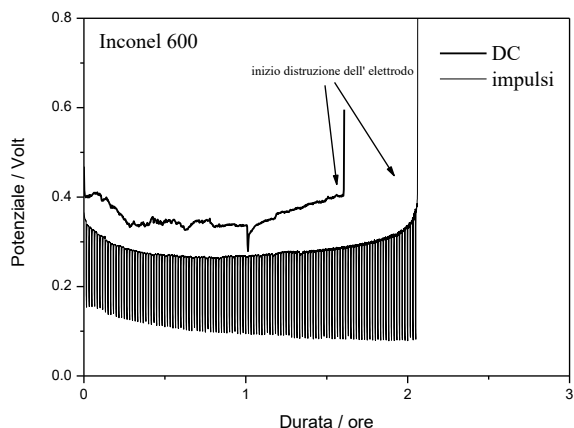
Figura 25 – Risultati dei test di polarizzazione galvanostatica sull’Inconel 600 in condizioni di corrente continua DC e ad impulsi. Corrente anodica applicata: 100 mA/ cm 2 .
