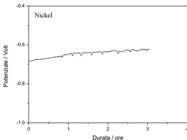
Figura 8 - Andamento nel tempo del potenziale di corrosione del Nickel.
