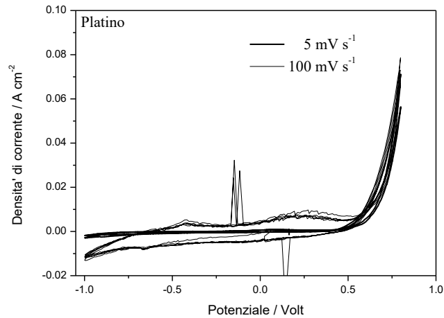
Figura 4 – Profilo voltammetrico del platino dopo il condizionamento. Scansione di potenziale fra -1V e +0.8V. Velocità di scansione: 5 e 100 mV s -1 . Numero di cicli: 5.
