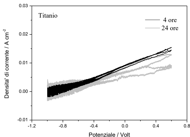
Figura 22 - Profilo voltammetrico del Titanio grado1 dopo 4 e 24 ore di immersione. Scansione di potenziale fra -1.0V e +0.6V. Velocità di scansione: 5 mV s -1 . Numero di cicli: 2.
