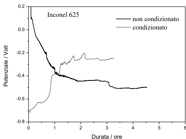
Figura 26 - Andamento nel tempo del potenziale di corrosione dell’Inconel 625: effetto del condizionamento. Condizionamento effettuato fra -0.5V e +0.2V, 100 mV s -1 , 100 cicli.
