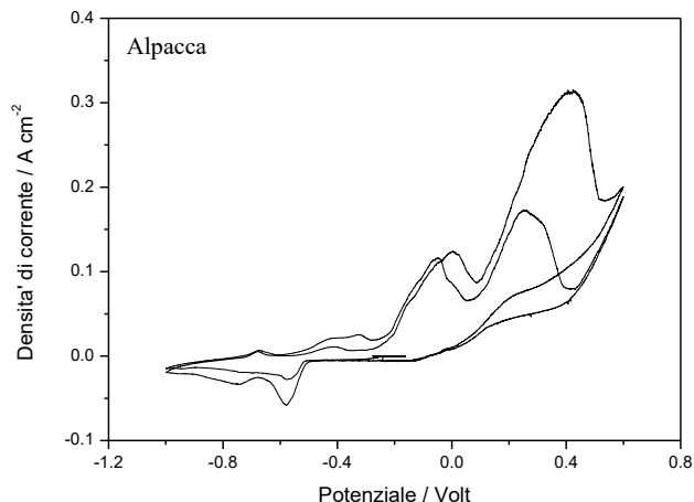
Figura 17 - Profilo voltammetrico della lega Alpacca dopo il trattamento di condizionamento. Scansione di potenziale fra -1.0V e +0.6V. Velocità di scansione: 5 mV s -1 . Numero di cicli: 2
