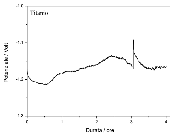
Figura 20 - Andamento nel tempo del potenziale di corrosione del Titanio grado 1.
