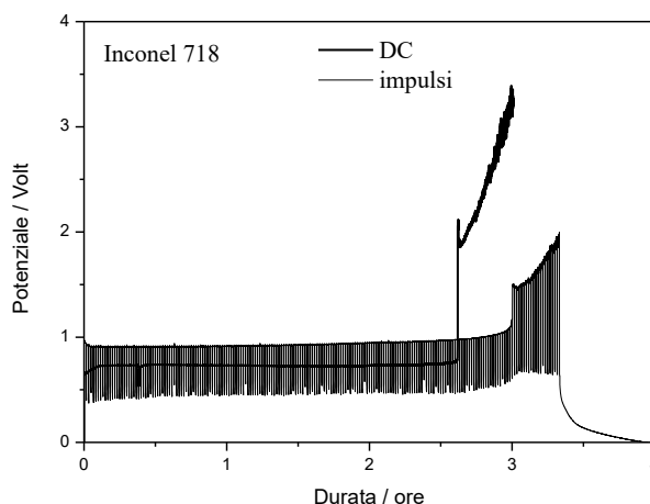
Figura 34 – Risultati dei test di polarizzazione galvanostatica sull’Inconel 718 in condizioni di corrente continua DC e ad impulsi. Corrente anodica applicata: 100 mA/ cm 2 .
