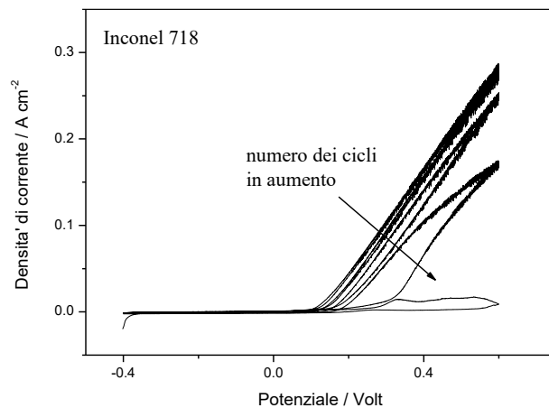
Figura 33 – Profilo voltammetrico dell’Inconel 718 dopo 4 ore di immersione. Scansione di potenziale fra -0.4V e +0.6V. Velocità di scansione: 5 mV s -1 . Numero di cicli: 5.
