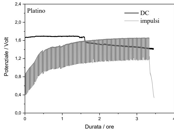
Figura 5 – Risultati dei test di polarizzazione galvanostatica in condizioni di corrente continua DC e ad impuls. Corrente anodica applicata: 100 mA/cm -2 .
