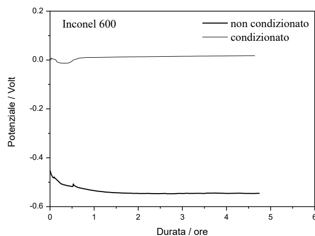
Figura 23 - Andamento nel tempo del potenziale di corrosione dell'Inconel 600: effetto del condizionamento. Condizionamento effettuato fra -0.5V e +0.2V , 100\text{ mV s}^{-1} , 100 cicli.
