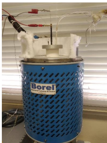
Figura 2 – Cella elettrochimica inserita nel forno tubolare. Sono visibili gli elettrodi collegati al potenziostato.
