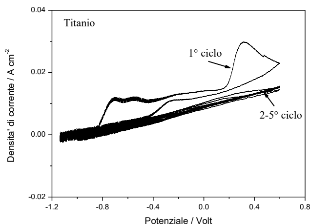
Figura 21 - Profilo voltammetrico del Titanio grado1 dopo 4 ore di immersione. Scansione di potenziale fra -1.0V e +0.6V. Velocità di scansione: 5 mV s -1 . Numero di cicli: 5.
