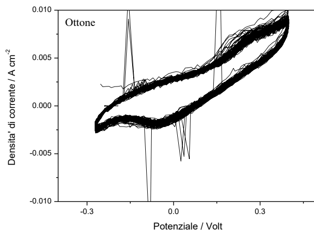
Figura 14 - Trattamento di condizionamento dell'elettrodo di ottone. Scansione di potenziale fra -0.25V e +0.35V. Velocità di scansione 100 mV s -1 . Numero di cicli: 100.
