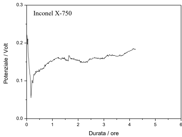
Figura 36 – Profilo voltammetrico dell'Inconel X-750 dopo 4 ore di immersione. Scansione di potenziale fra -0.4V e +0.6V. Velocità di scansione: 5 mV s -1 . Numero di cicli: 5.
