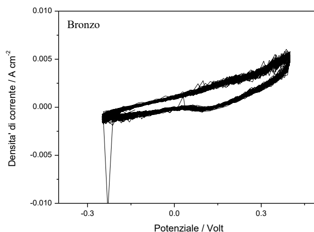
Figura 12 - Trattamento di condizionamento dell'elettrodo di bronzo. Scansione di potenziale fra -0.25V e +0.35V. Velocità di scansione 100 mV s -1 . Numero di cicli: 100.
