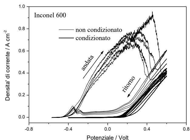
Figura 24 – Effetto del condizionamento sul profilo voltammetrico dell'Inconel 600 dopo 4 ore di immersione. Scansione di potenziale fra -0.6V e +0.6V . Velocità di scansione: 5\text{ mV s}^{-1} . Numero di cicli: 5.
