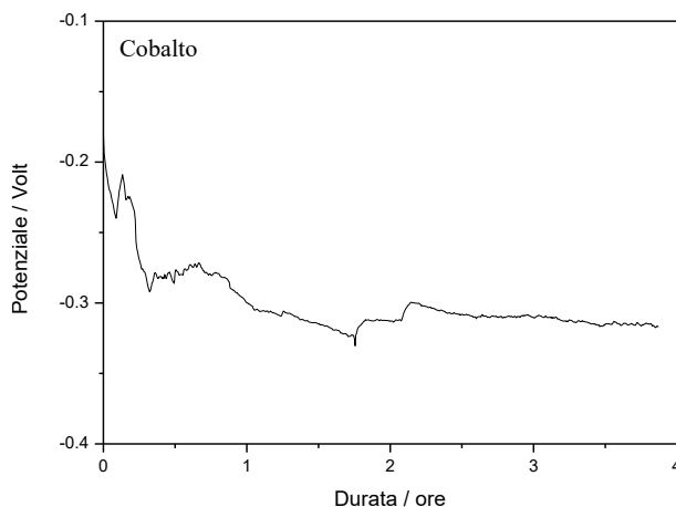
Figura 18 - Andamento nel tempo del potenziale di corrosione del cobalto.
