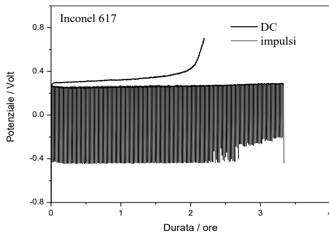
Figura 31 – Risultati dei test di polarizzazione galvanostatica sull’Inconel 617 in condizioni di corrente continua DC e ad impulsi. Corrente anodica applicata: 100 mA/ cm 2 .
