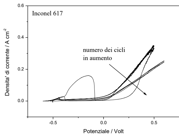
Figura 30 – Profilo voltammetrico dell'Inconel 617 dopo circa 6 ore di immersione. Scansione di potenziale fra -0.6V e +0.6V. Velocità di scansione: 5 mV s -1 . Numero di cicli: 5.
