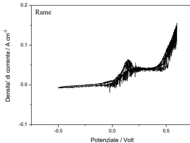
Figura 11 - Profilo voltammetrico del rame dopo il trattamento di condizionamento. Scansione di potenziale fra -0.5V e +0.6V. Velocità di scansione: 5 mV s -1 . Numero di cicli: 2.
