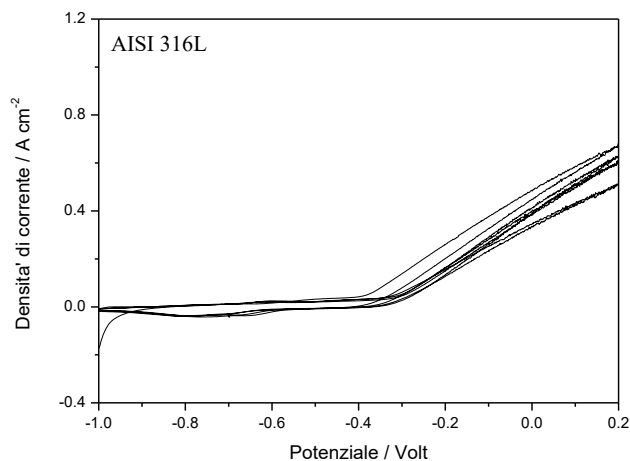
Figura 7 - Profilo voltammetrico dell'acciaio inox AISI 316L. Scansione di potenziale fra -1V e +0.2V. Velocità di scansione: 5 mV s -1 . Numero di cicli: 5.
