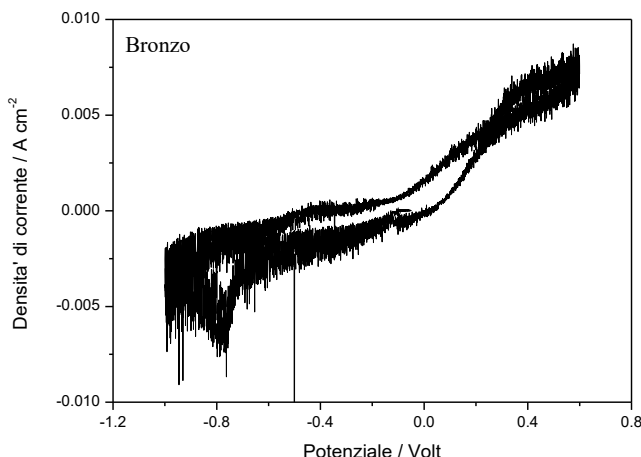
Figura 13 - Profilo voltammetrico del bronzo dopo il trattamento di condizionamento. Scansione di potenziale fra -1V e +0.6V. Velocità di scansione: 5 mV s -1 . Numero di cicli: 2.
