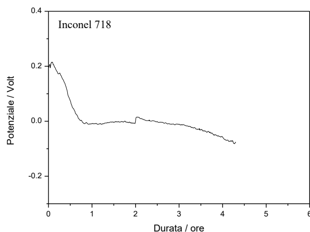
Figura 32 - Andamento nel tempo del potenziale di corrosione dell’Inconel 718. Elettrodo non condizionato.
