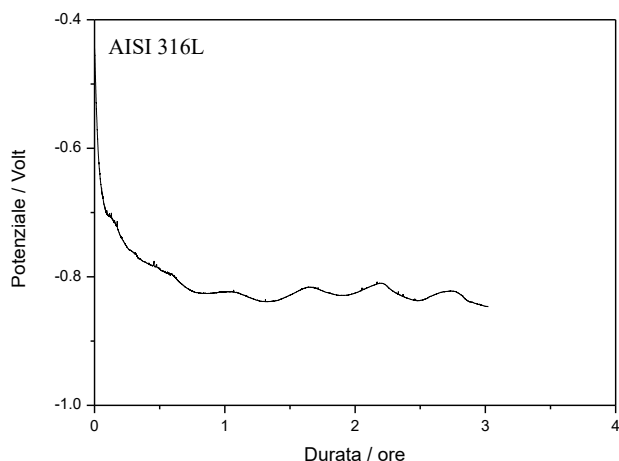
Figura 6 – Andamento nel tempo del potenziale di corrosione dell'acciaio inox AISI 316L.
