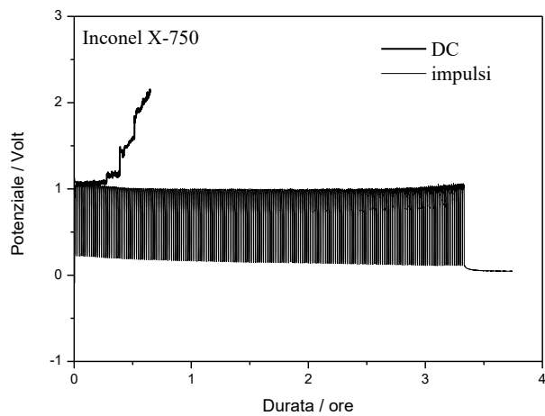
Figura 37 – Risultati dei test di polarizzazione galvanostatica sull'Inconel X-750 in condizioni di corrente continua DC e ad impulsi. Corrente anodica applicata: 100 mA/ cm -2 .
