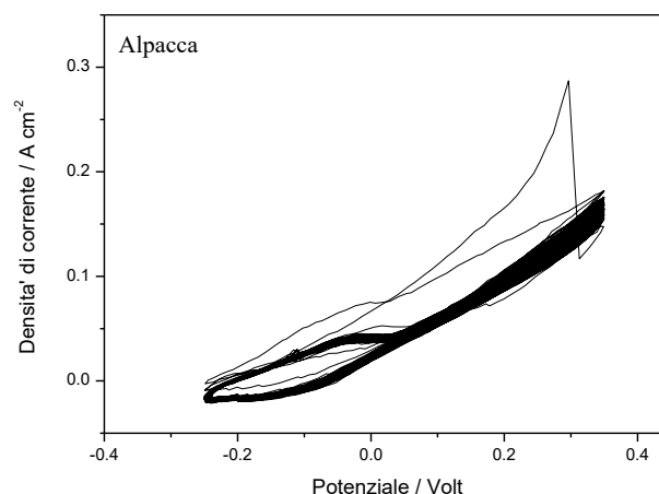
Figura 16 - Trattamento di condizionamento dell'elettrodo di Alpacca. Scansione di potenziale fra -0.25V e +0.35V. Velocità di scansione 100 mV s -1 . Numero di cicli: 100.
