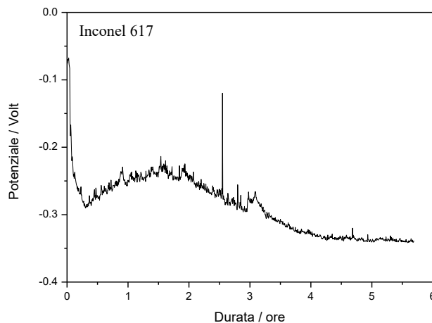
Figura 29 - Andamento nel tempo del potenziale di corrosione dell'Inconel 617. Elettrodo non condizionato.
