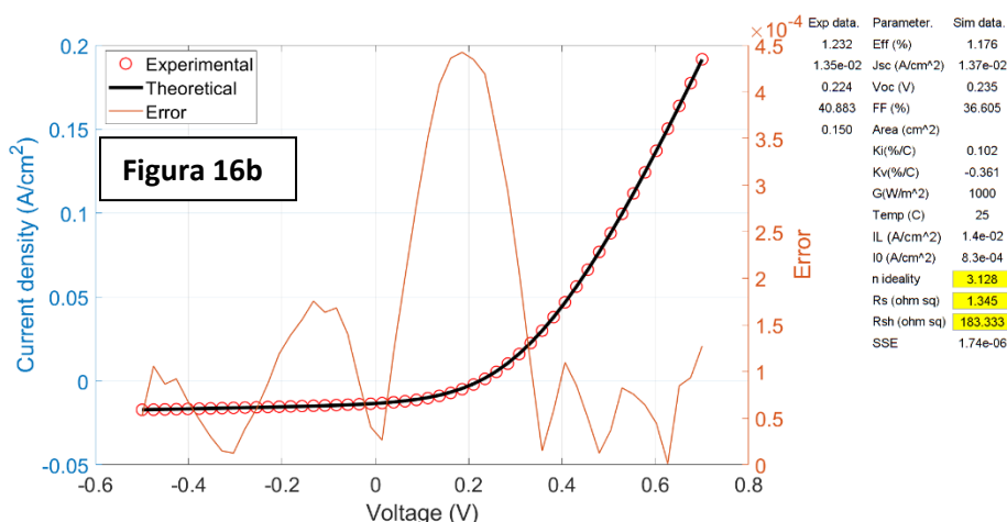
Figura 16. (a) fitting della curva al buio della cella di CZTS prodotta mediante film applicator; (b) fitting della curva sotto illuminazione della cella di CZTS prodotta mediante film applicator
