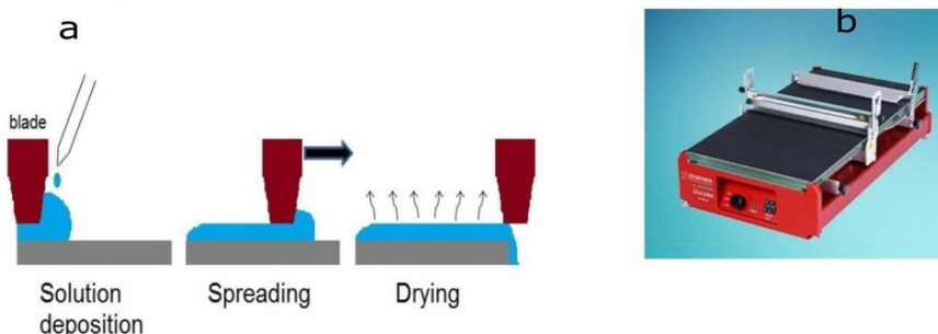
Figura 12. (a) schema di funzionamento della stesura della goccia mediante film applicator; (b) foto del film applicator utilizzato (Zehntner ZAA 2300) SCAPS del CZTS
