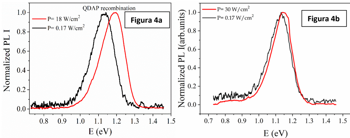
Figura 4. (a) misura PL a bassa temperatura ( T=14 K, \lambda_{\text{ex}}=805 nm, \Delta\lambda=6.6 nm) di un film di CZTS depositato su Mo-SLG; (b) misura PL a bassa temperatura ( T=14 K, \lambda_{\text{ex}}=805 nm, \Delta\lambda=6.6 nm) di CZTS depositato su FTO:Mo semitrasparente
