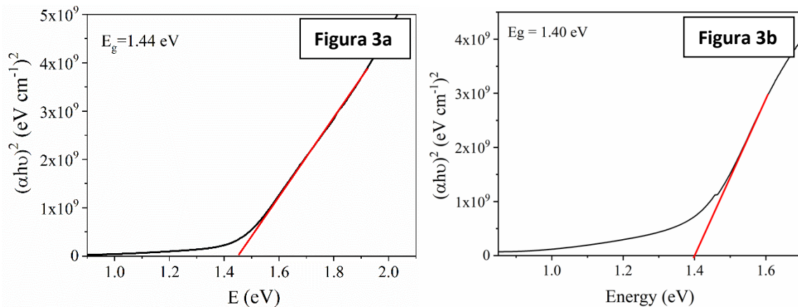
Figura 3. (a) Tauc's Plot di CZTS depositato su molibdeno; (b) Tauc's Plot di CZTS depositato su FTO:Mo semi-trasparente
