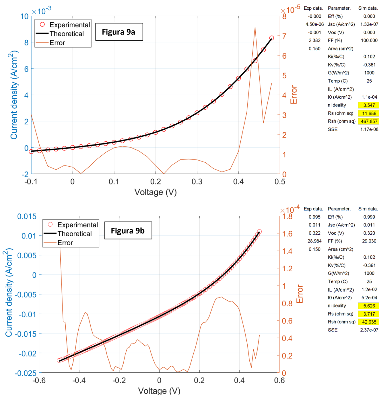
Figura 9. MATLAB fitting di curve J-V al buio e sotto illuminazione J-V (linea nera), misura sperimentale di curve J-V al buio e sotto illuminazione J-V (punti rossi) ed errore sul fitting (linea arancione) (dispositivo realizzato sul substrato FTO:Mo) . I risultati della interpolazione sono riportati nelle tabelle a fianco del grafico: (a) curva al buio; (b) curva sotto illuminazione.
