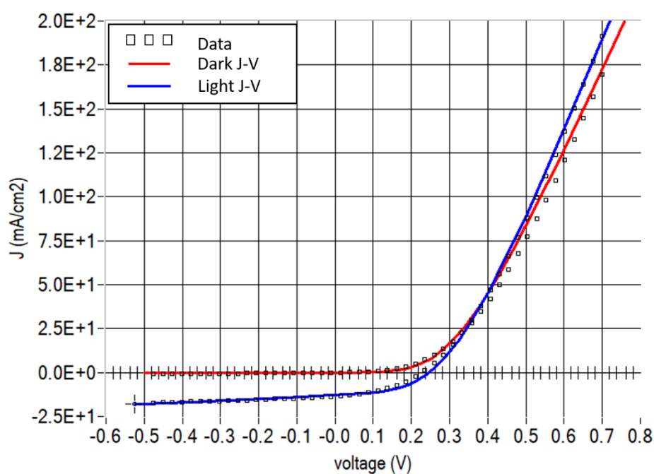
Figura 19. Risultato SCAPS della simulazione cella di CZTS prodotta mediante Film Applicator
