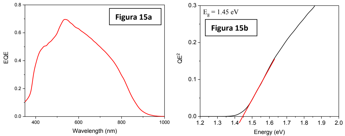
Figura 15. (a) curva EQE della cella di CZTS depositato su Mo-SLG mediante Film Applicator; (b) band gap calcolato da QE 2 = 1.45 eV
