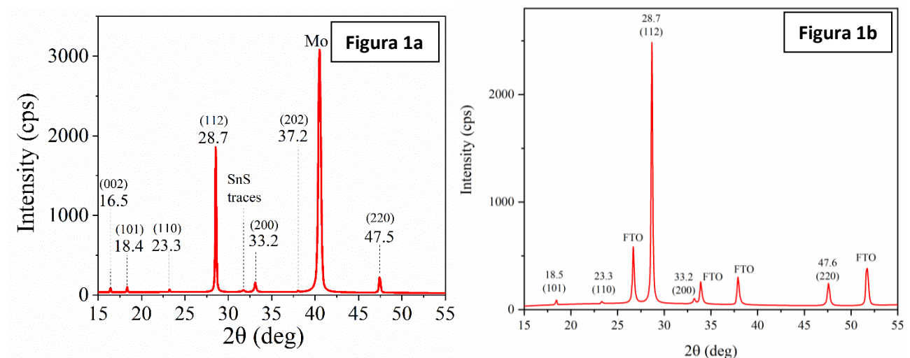
Figura 1. (a) XRD pattern di CZTS depositato su Mo-SLG; (b) XRD pattern di CZTS depositato su FTO:Mo semi-trasparente
