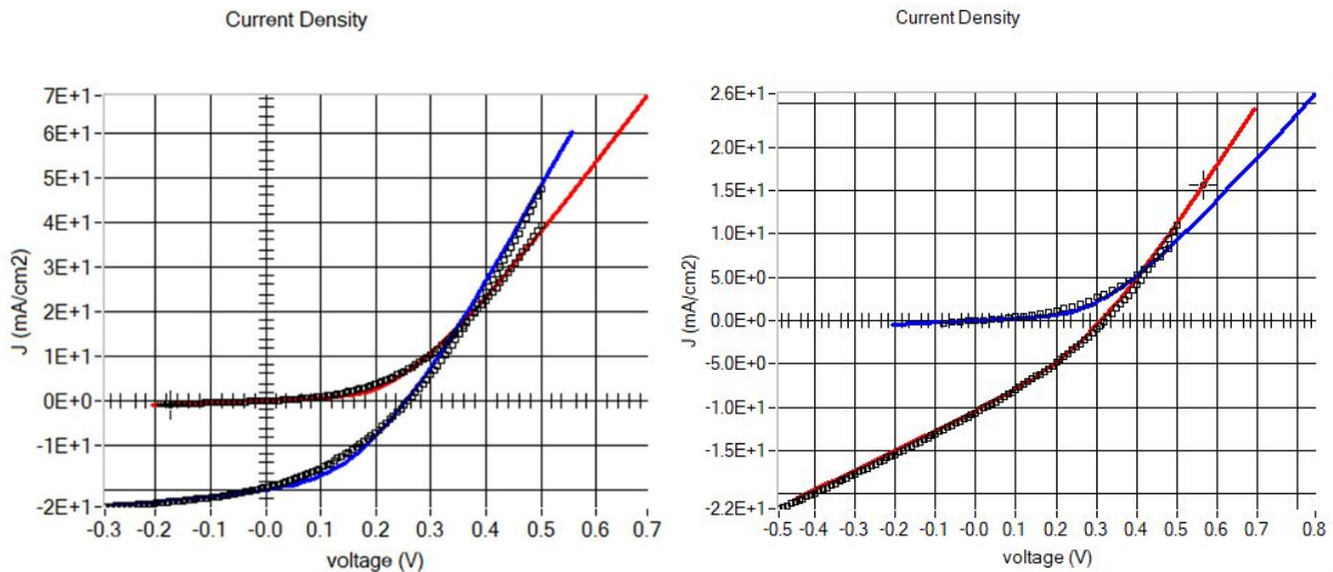
Figura 11. (a) simulazione della curva J-V di SCAPS del CZTS su Mo; (b) simulazione della curva J-V di SCAPS del CZTS su FTO:Mo; (Linea blu: curva sperimentale al buio; linea rossa: curva sperimentale sotto illuminazione frontale; tratteggio nero: curve al buio e sotto illuminazione simulate con SCAPS).
