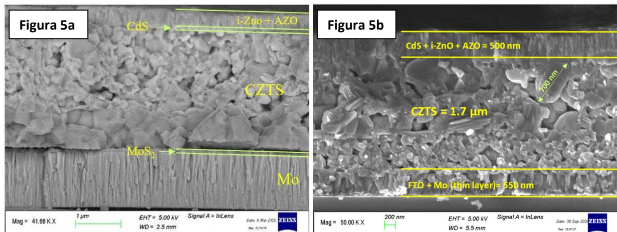
Figura 5. (a) Immagine SEM in sezione di CZTS depositato su Mo-SLG; (b) Immagine SEM in sezione di CZTS depositato su FTO:Mo semi-trasparente
