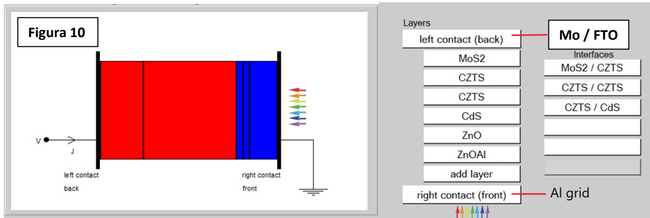
Figura 10. Architettura del dispositivo virtuale utilizzata nel software di simulazione SCAPS che replica l'architettura reale dei dispositivi prodotti; sono inoltre indicate le interfacce considerate.
