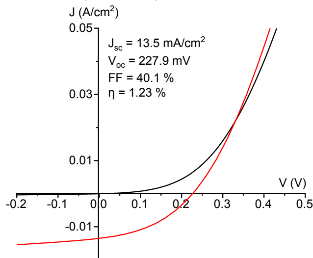
Figura 14. Curva J-V della cella di CZTS depositato su molibdeno mediante Film Applicator
