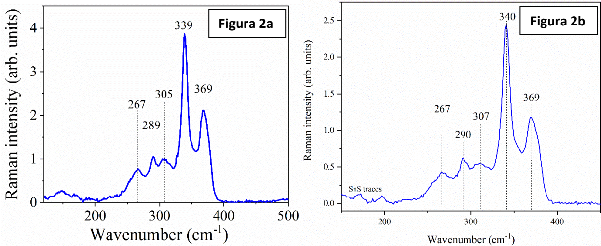
Figura 2. (a) spettro Raman di un tipico campione di CZTS cresciuto su film di molibdeno; (b) spettro Raman di CZTS depositato su substrato FTO:Mo semi-trasparente
