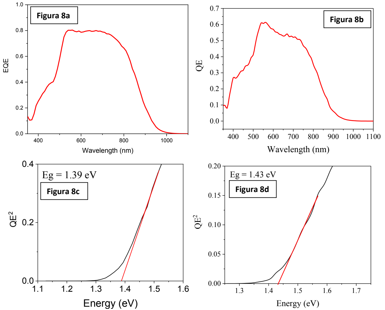
Figura 8. (a) misura EQE del dispositivo di CZTS depositato su Mo-SLG; (b) misura EQE del dispositivo bifacciale di CZTS depositato su FTO:Mo semi-trasparente; (c) band gap da QE² per la cella su Mo-SLG; (d) band gap da QE² per la cella su FTO:Mo semi-trasparente
