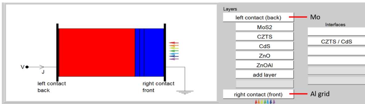
Figura 17. Architettura SCAPS della cella di CZTS prodotta mediante Film Applicator
