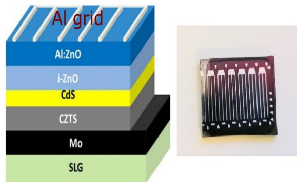
Figura 6. (sinistra) architettura di cella utilizzata; (destra) foto del dispositivo fotovoltaico ottenuto
