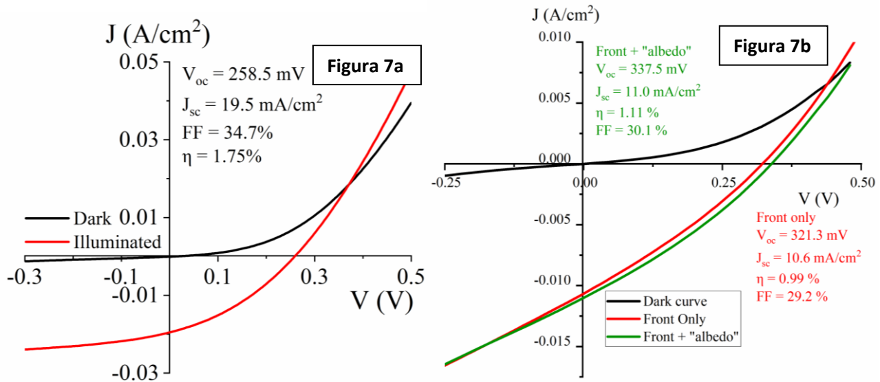
Figura 7. (a) misura J-V del dispositivo di CZTS depositato su molibdeno; (b) misura J-V del dispositivo bifacciale di CZTS depositato su FTO:Mo semi-trasparente
