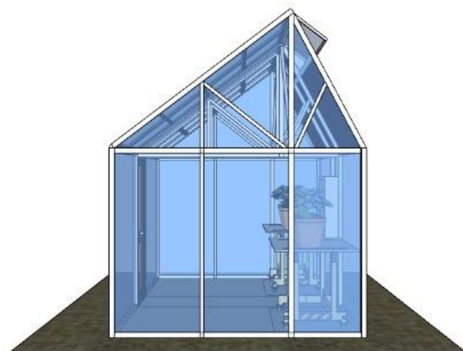
Figure 2.1.10: Immagine complessiva del prospetto laterale della serra, con dettaglio del sistema di ventilazione naturale affidato alla falda asimmetrica con apertura in alto lungo la parete nord.
