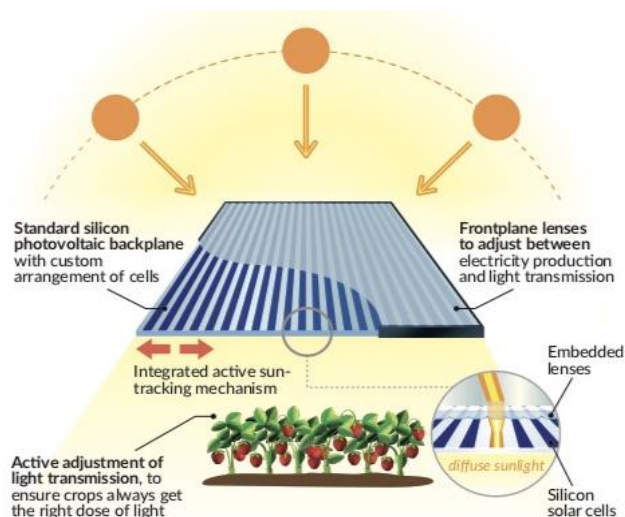
Figura 2.1.4: Il modulo agrivoltaico THEIA Insolight.
