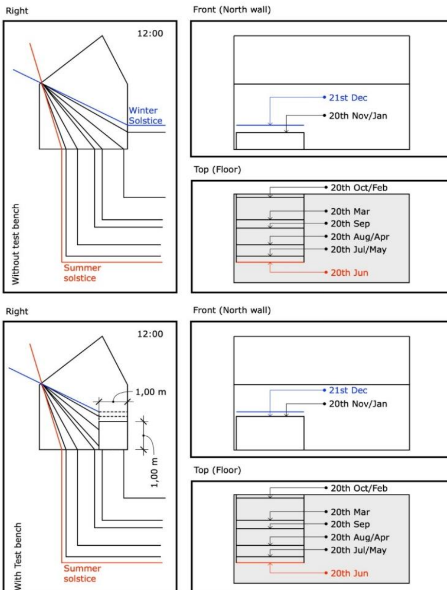
Figura 2.1.7: Studio dei percorsi solari nel corso dell'anno e relativi ombreggiamenti.
