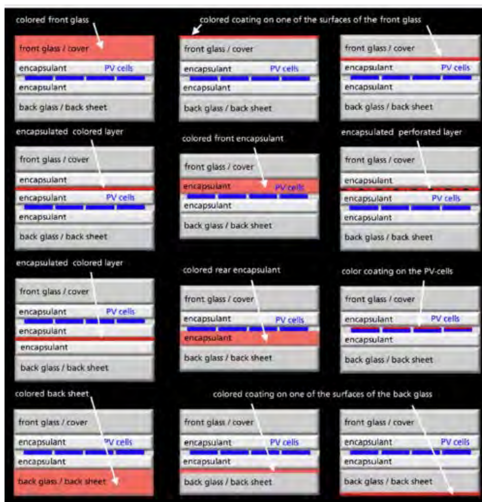
Figura 33. Possibili stratificazioni di moduli BIPV colorati, in cui si evidenziano le molte possibilità tecnologiche relative all'integrazione del colore, evidenziato in rosso [89].
