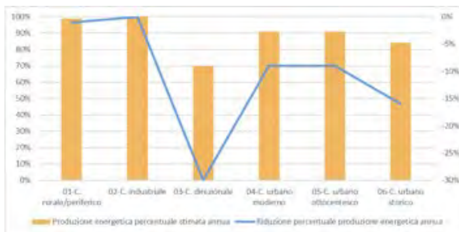
Figura 45. Variazione di produzione energetica di un sistema BIPV (tecnologia in silicio amorfo) in relazione ai diversi tipi di tessuto individuati. Sulla colonna sinistra è riportata la produzione energetica simulata; su quella destra, le riduzioni percentuali della produzione energetica stimata.
