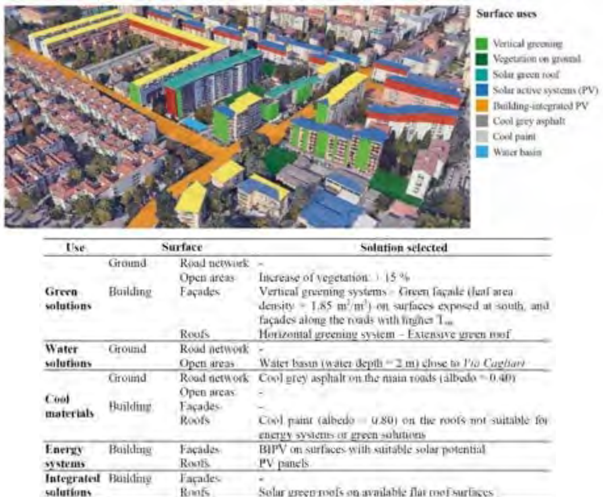
Figura 12. Approcci sistemici per l'integrazione di soluzioni fotovoltaiche sul costruito valutando le ricadute in ambito urbano in termini di resilienza climatica [56].
