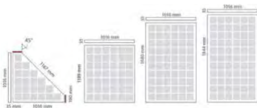
Figura 29. Moduli standard caratterizzati da diverse geometrie e dimensioni [Fonte: TRIENERGIA].
