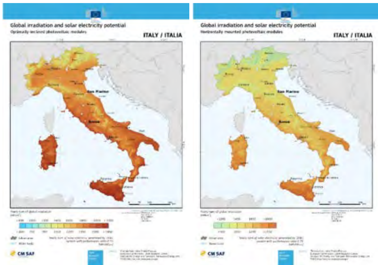
Figura 18. A sinistra, mappa dell'Italia che mostra la variazione della radiazione globale e potenziale elettricità prodotta da un impianto potenziale con inclinazione orizzontale. A destra, mappa dell'Italia che mostra la variazione della radiazione globale e potenziale elettricità prodotta da un impianto potenziale con inclinazione ottimale [Fonte grafici: https://re.jrc.ec.europa.eu/pvg_download/map_index.html ].
