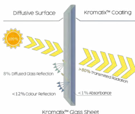
Figura 37. Schema di funzionamento del vetro a cui è applicato il filtro interferenziale Kromatix [Fonte: SWISSINSO].
