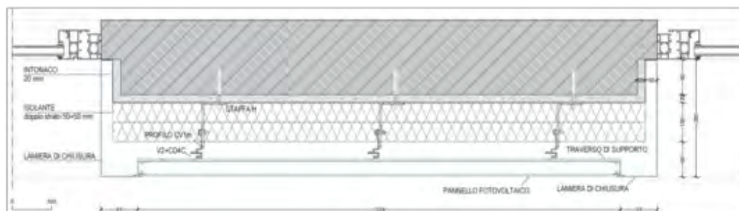
Prospetti Sud (con individuazione dei moduli FV) ed Est; particolare costruttivo della facciata ventilata in corrispondenza dei moduli fotovoltaici.
