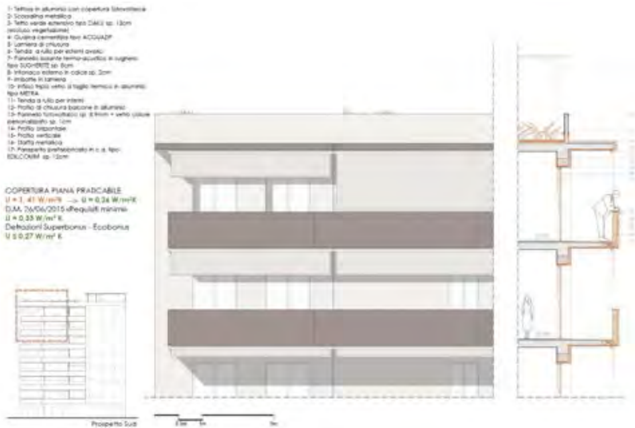
Figura 44. Integrazione di sistemi BIPV e controllo delle prestazioni termiche dell'involucro post retrofit (Elaborazione: C. Acquaviva).
