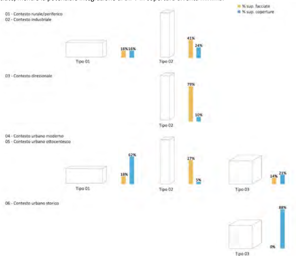
Figura 42. Variazione della percentuale media delle superfici idonee per l'installazione di sistemi BIPV suddivise per facciate e coperture in relazione ai tipi di edificio individuati nei diversi contesti urbani.
