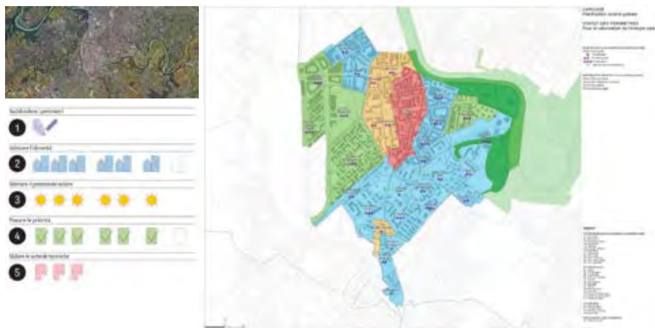
Figura 10. Il metodo in 5 step per l'identificazione delle aree idonee per integrazioni BIPV sperimentato nella città di Carouge [54].
