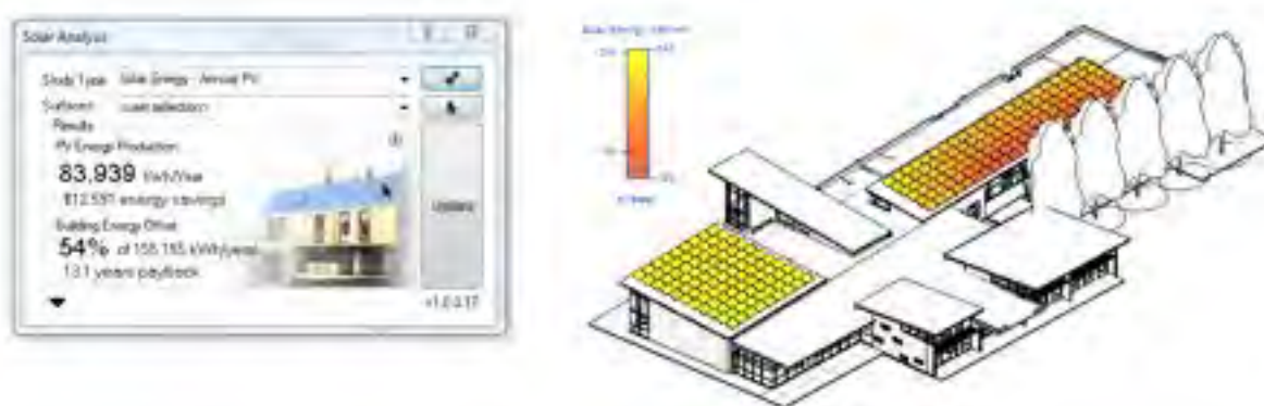
Figura 24. Finestra di dialogo del tool INSIGHT 360 - Solar Analysis durante la progettazione di un sistema fotovoltaico in copertura. Fonte grafici: https://blogs.autodesk.com/insight/pv-building-energy-offsets-with-insight-360-solar-analysis-2/ .
