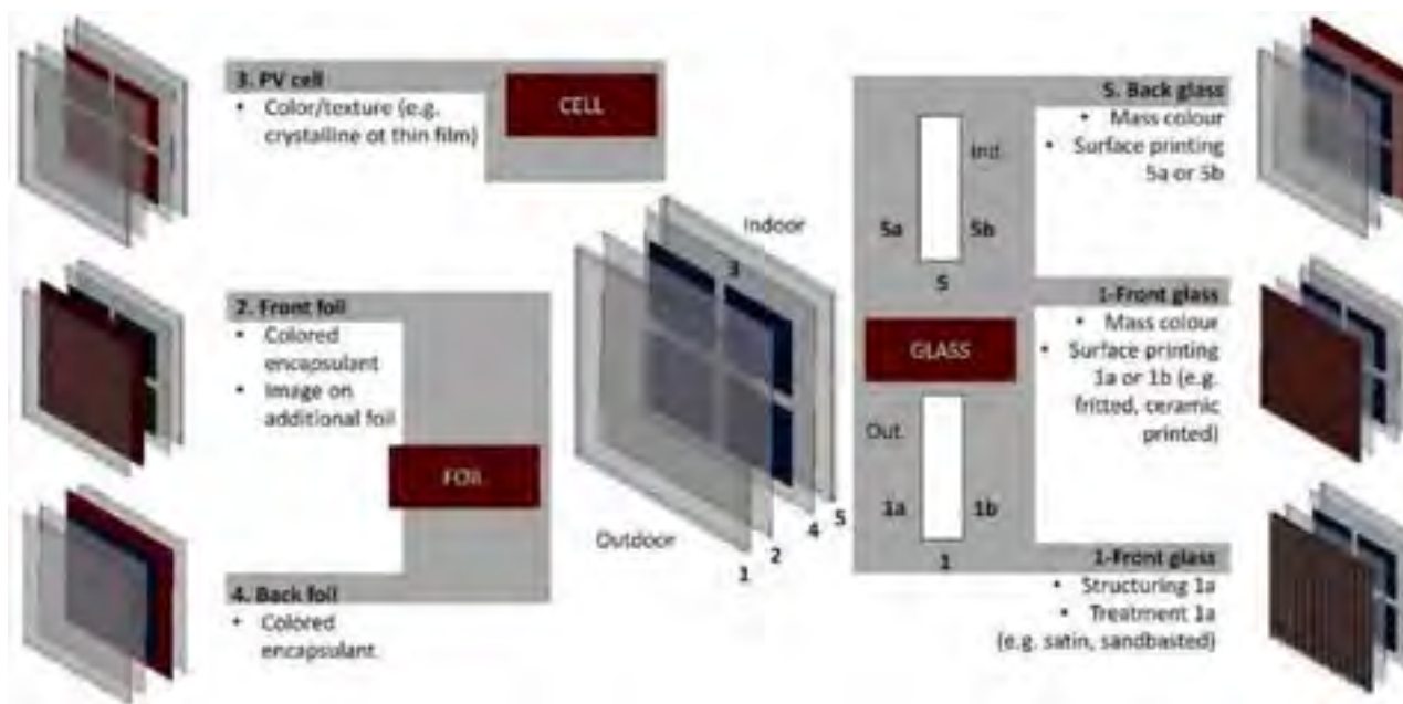
Figura 32. Possibilità di personalizzazione cromatica di un componente vetro-vetro BIPV per ottenere un aspetto colorato. Le celle possono essere visibili o nascoste [88].
