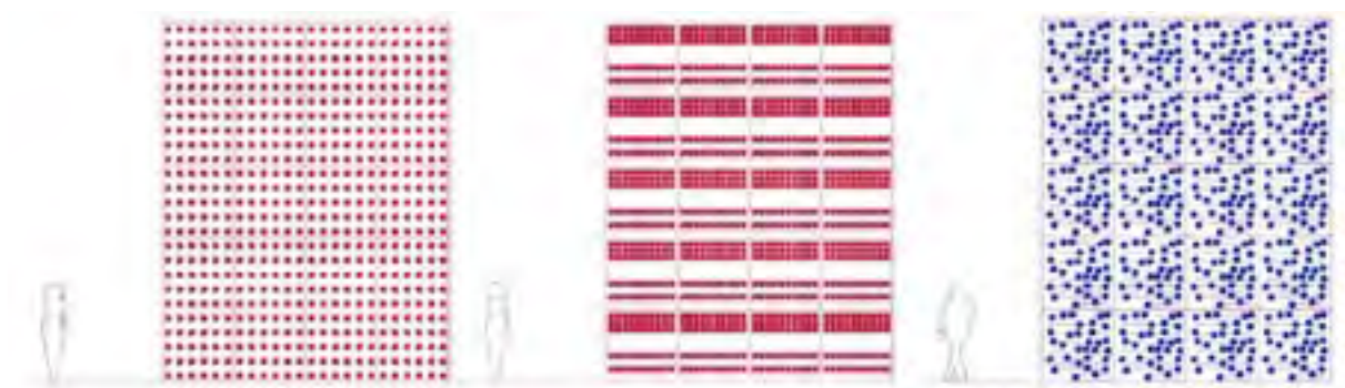
Figura 31. Confronto tra diverse possibilità progettuali dei pattern FV basate sulle geometrie: griglia ortogonale, strisce orizzontali parallele, random [90; 91].
