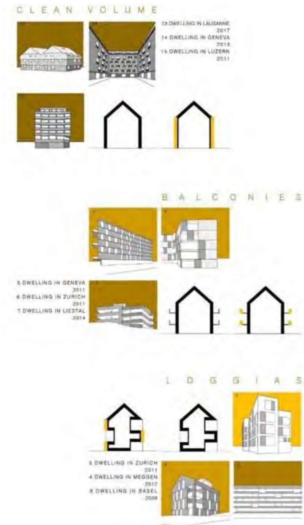
Figura 21. Schemi di morfologia di facciata e corrispondente integrazione BIPV [70].
