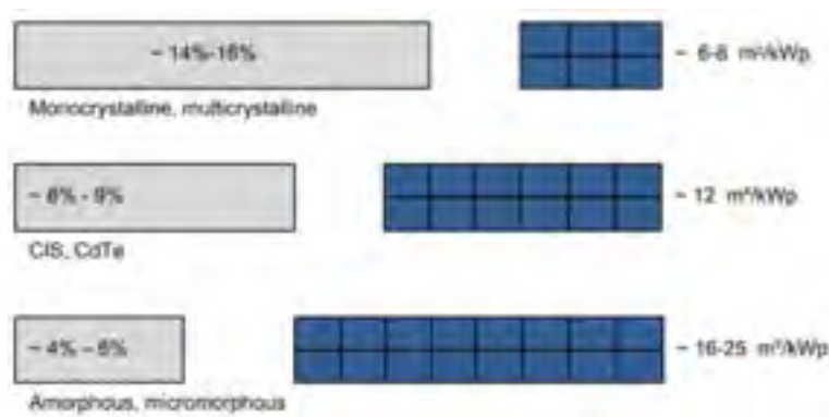
Figura 17. Variazione dello spazio richiesto per l'installazione di pannelli fotovoltaici in relazione all'efficienza di conversione dei moduli [Fonte grafici: SUPSI, ISACC].
