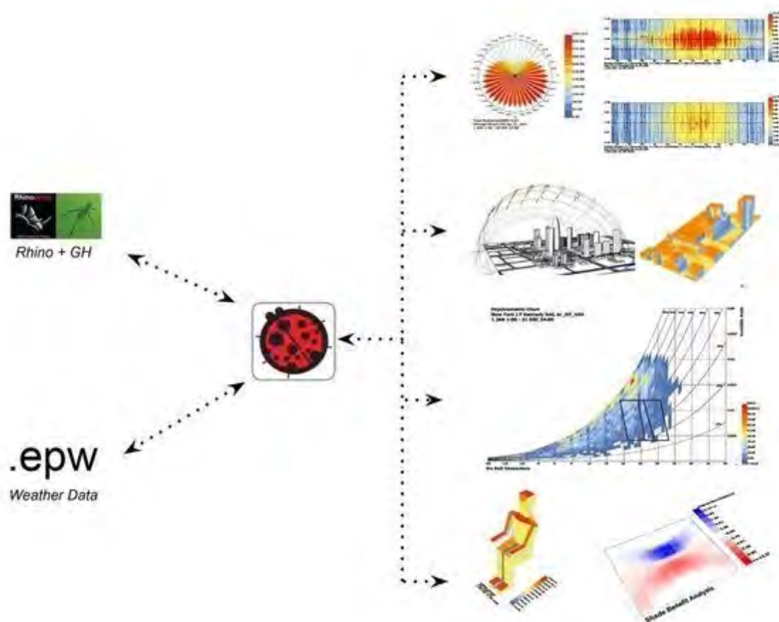
Figura 25. Dati di input e output del plugin Ladybug per Rhinoceros/Grasshoper. Fonte grafici: https://www.grasshopper3d.com/ .
