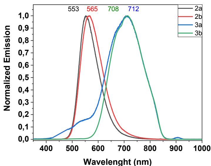
Figura 7. Spettri di fluorescenza per i polimeri 2a-2b e 3a-3b.
