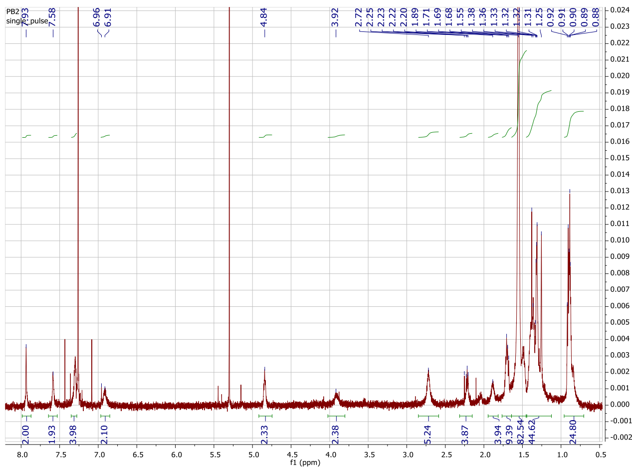
Figura 20. ^1\text{H} -NMR del Polimero 2b.
