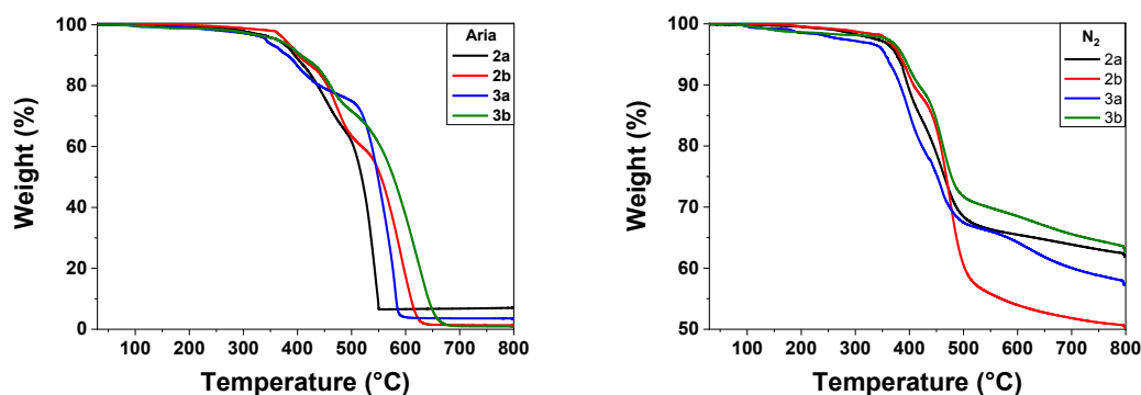
Figura 9. Analisi TGA in aria ed azoto per i polimeri 2a-2b e 3a-3b.
