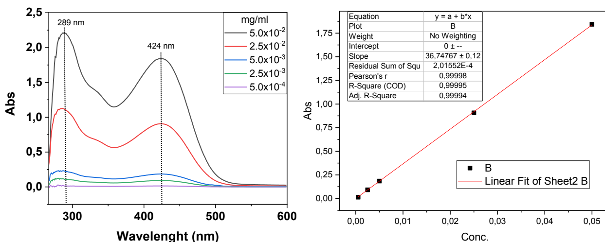
Figura 6. Spettri UV a concentrazione variabile per il polimero 2a e stima del coefficiente di assorbimento.
