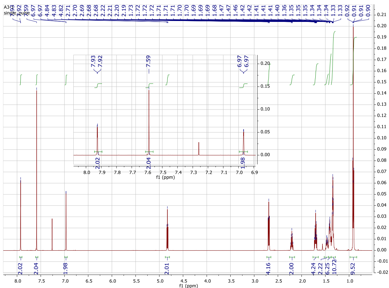
Figura 14. ^1\text{H} -NMR del Composto 9.
