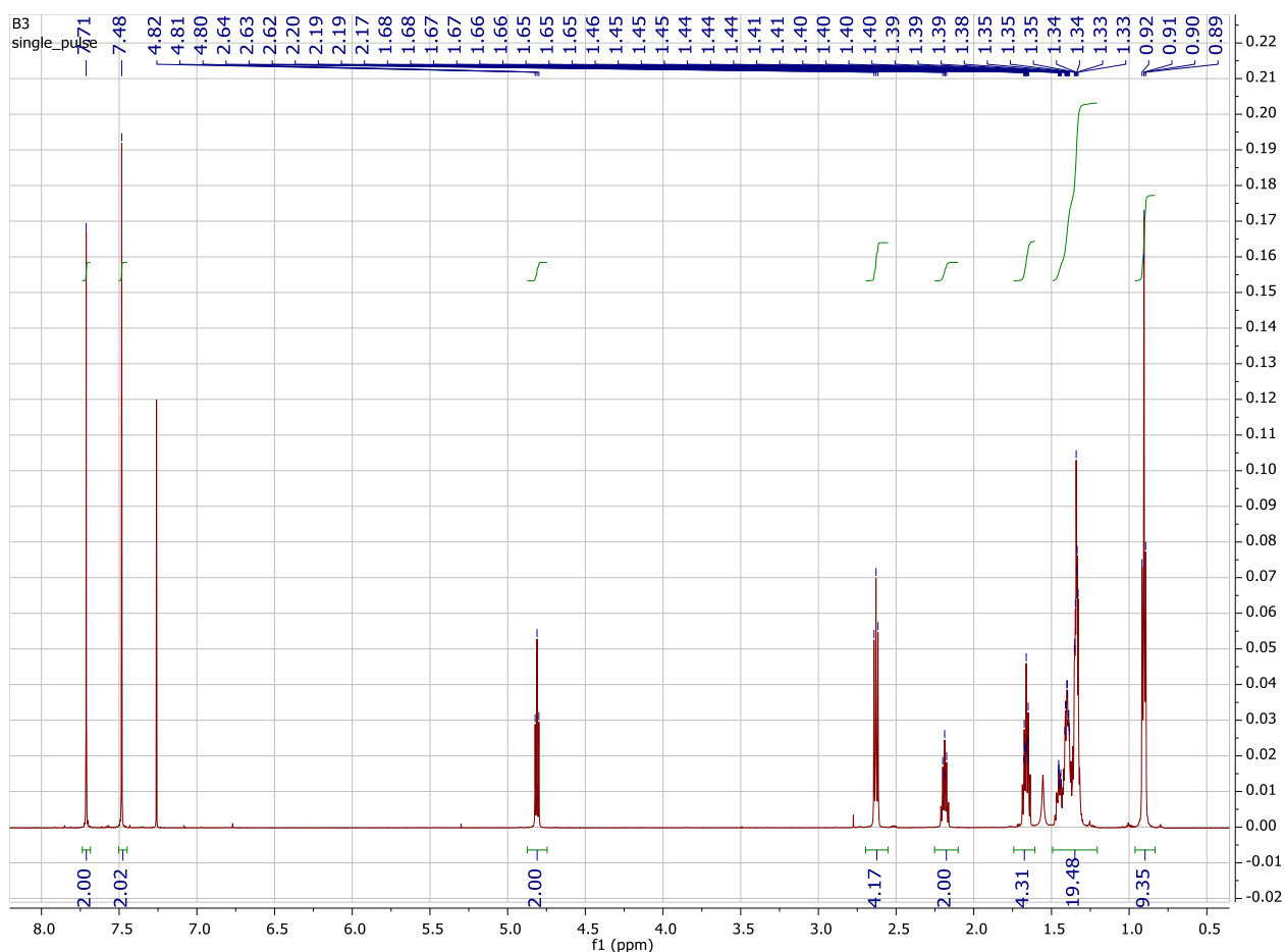
Figura 15. ^1\text{H} -NMR del Composto 10.
