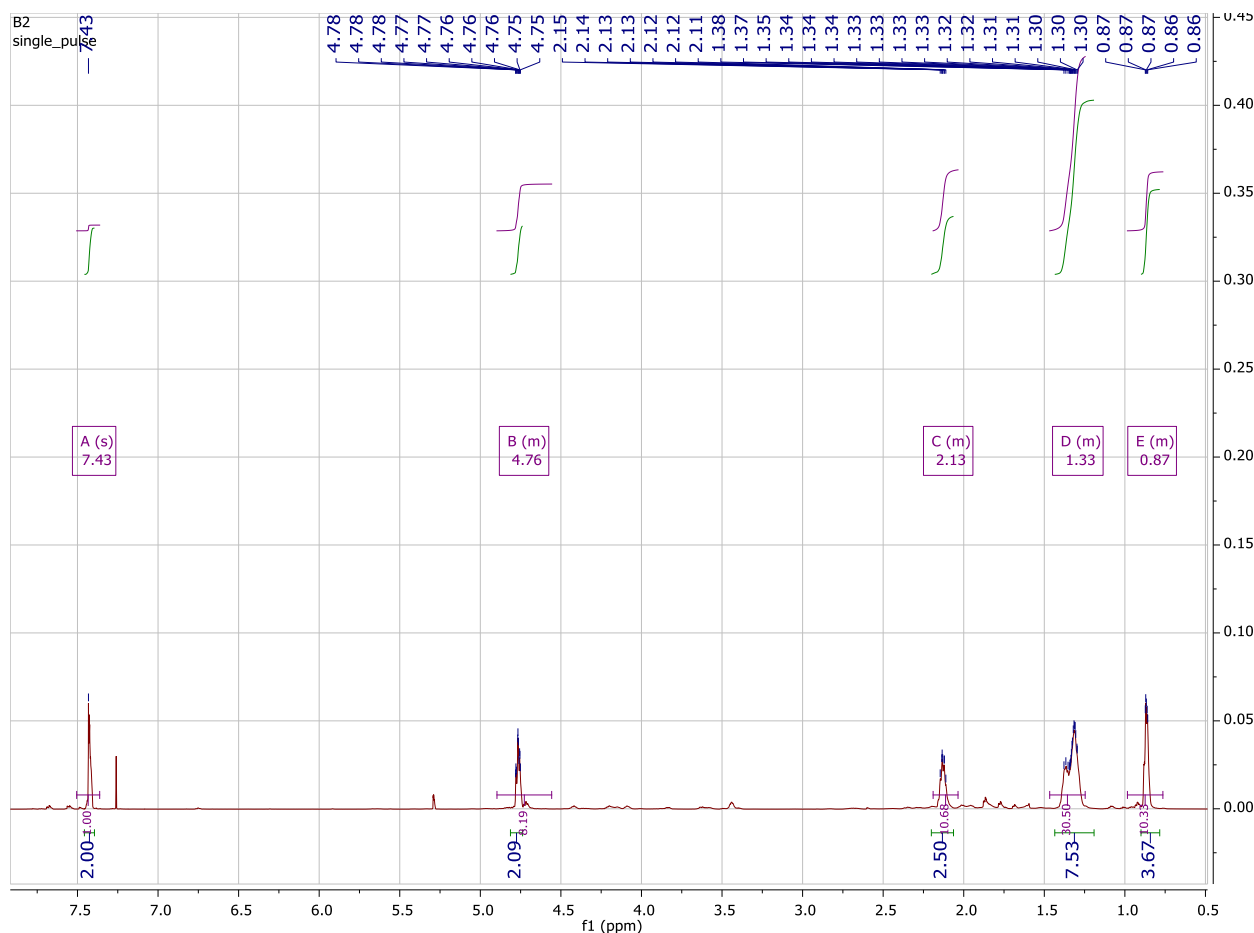
Figura 13. ^1\text{H} -NMR del Composto 8.
