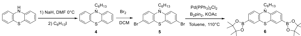
Figura 3. Preparazione del reagente fenotiazinico 6 per la sintesi dei polimeri 2.
