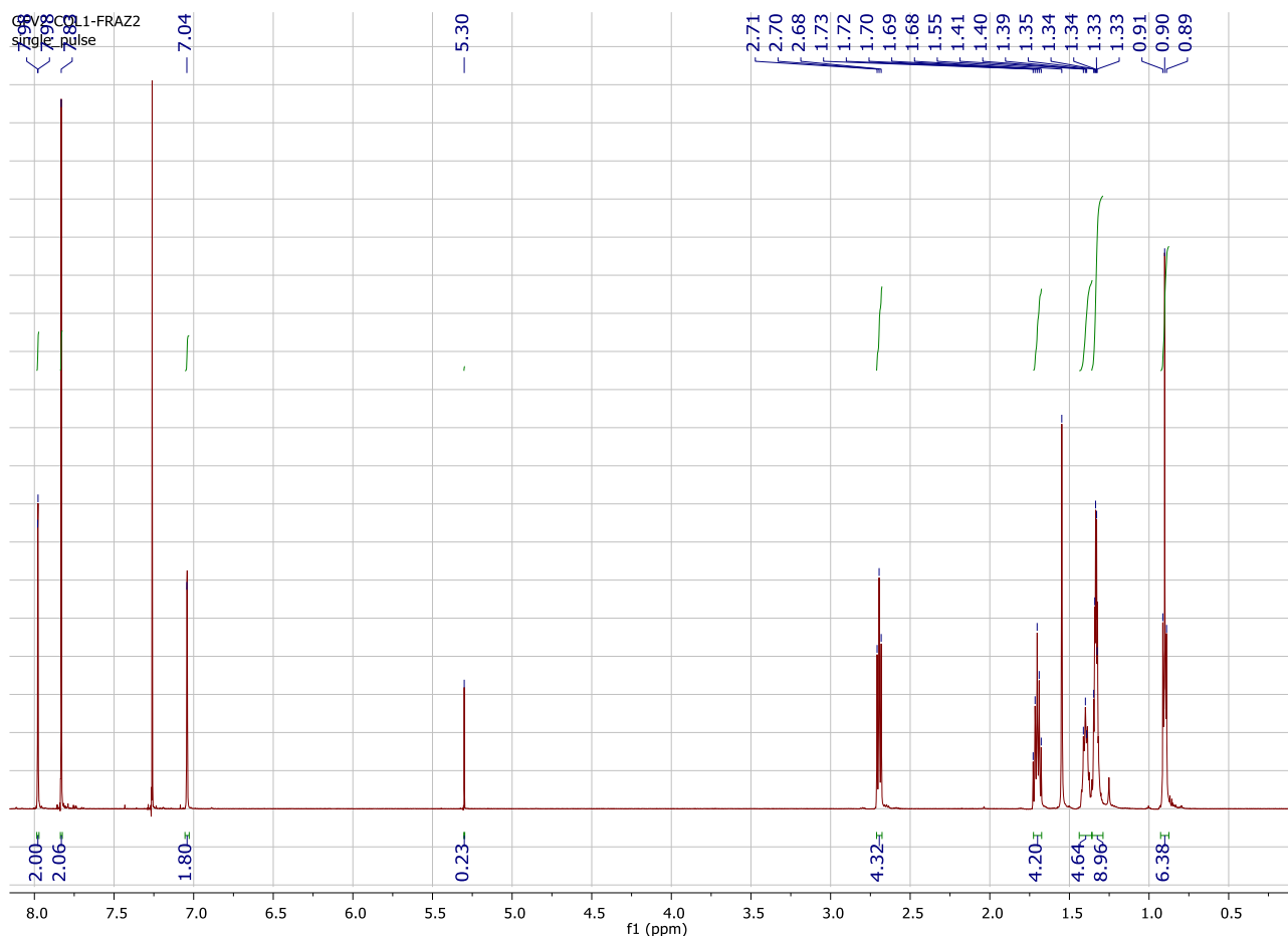
Figura 17. ^1\text{H} -NMR del Composto 12 .
