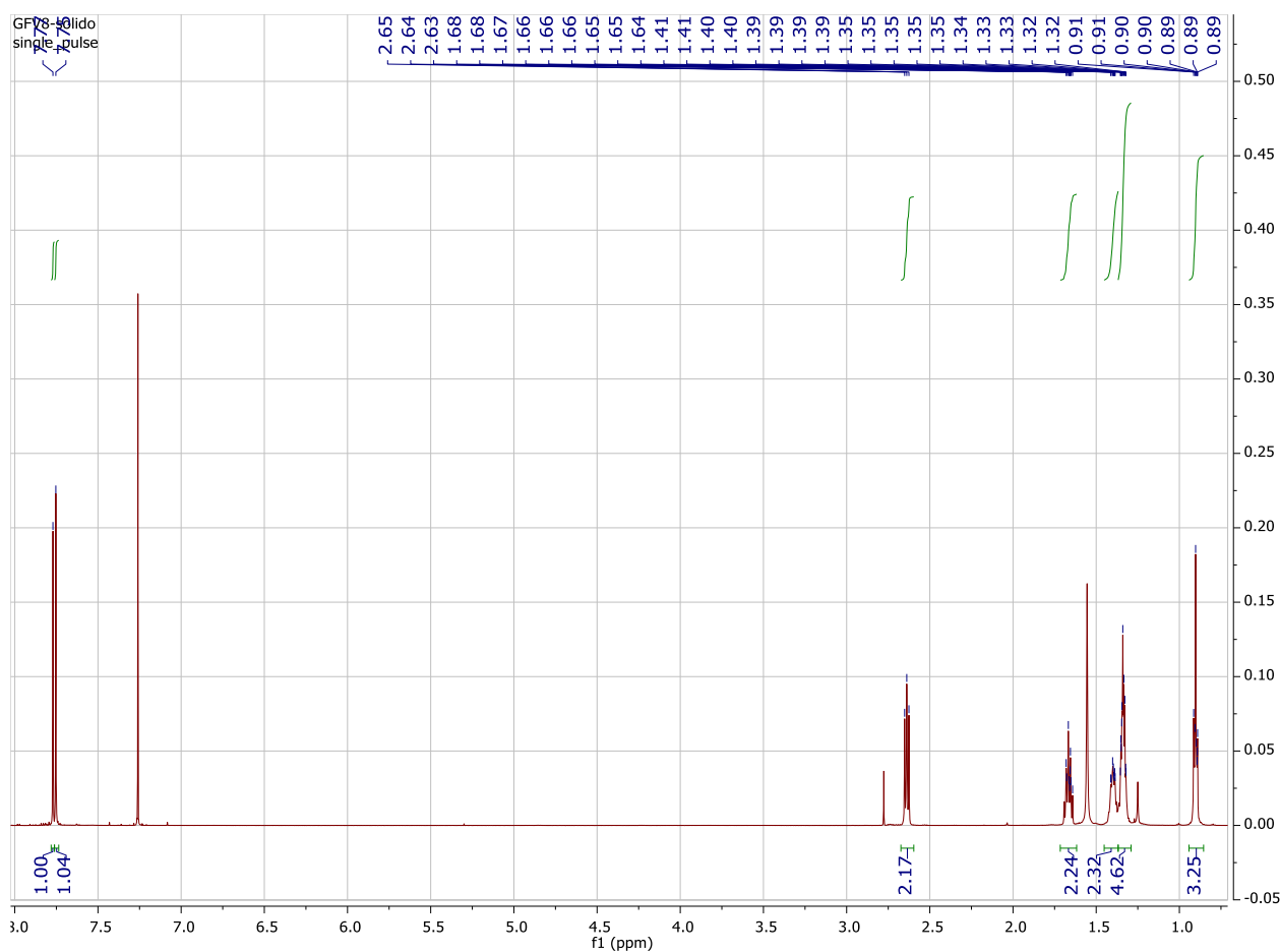
Figura 18. ^1\text{H} -NMR del Composto 13.
