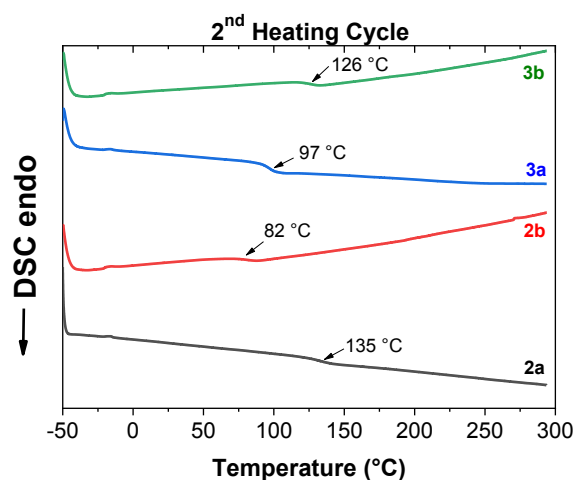
Figura 10. Analisi DSC in azoto per i polimeri 2a-2b e 3a-3b.
