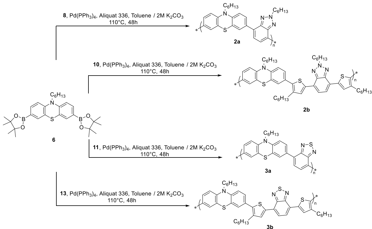
Figura 4. Preparazione dei polimeri 2a-2b e 3a-3b.
