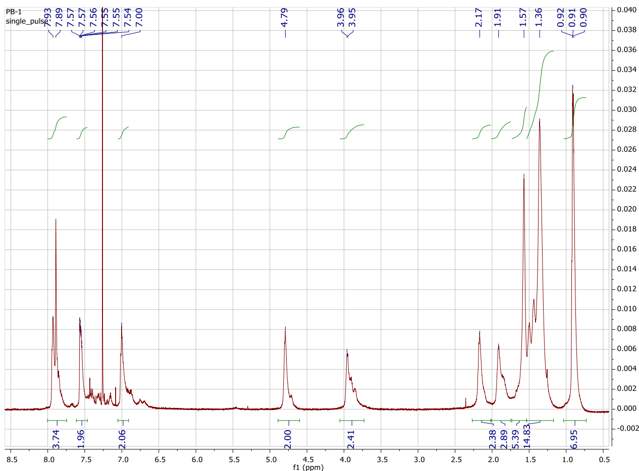
Figura 19. ^1\text{H} -NMR del Polimero 2a .
