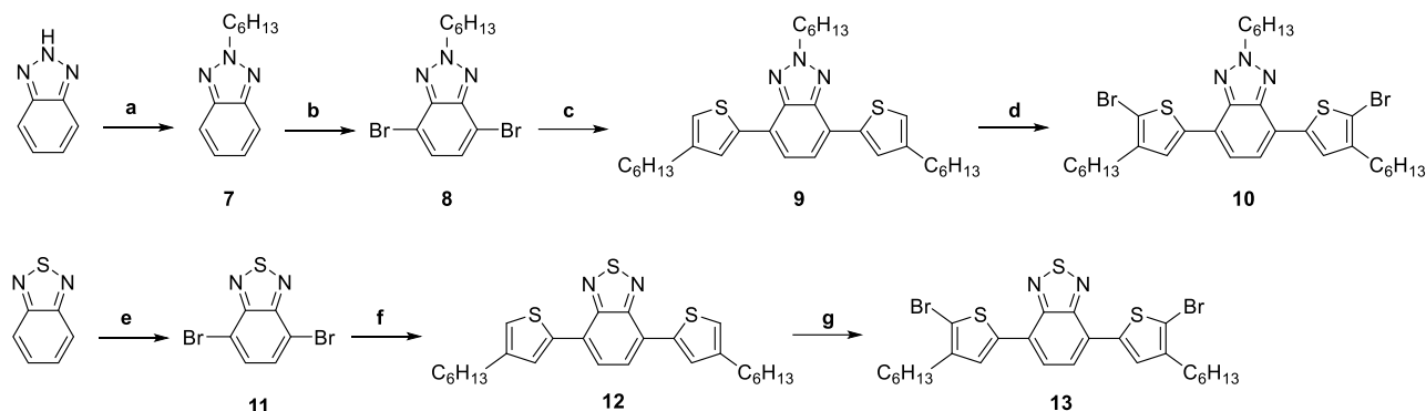
Figura 3. Preparazione degli intermedi accettori 7-13. Condizioni di reazione: a) t-BuOK, 1-bromoesano, MeOH, 80°C, 12h; b) Br 2 , HBr 48%, reflux, 6h; c) 2-(4-esil-2-tienil)-4,4,5,5-tetrametil-1,3,2-diossaborolano, Pd(PPh 3 ) 4 , Aliquat 336, toluene/2M K 2 CO 3 , 110°C, 24 h; d) NBS, DMF, 0°C, 1h; e) Br 2 , HBr 48%, reflux, 6h; f) 2-(4-esil-2-tienil)-4,4,5,5-tetrametil-1,3,2-diossaborolano, Pd(PPh 3 ) 4 , Aliquat 336, toluene/2M K 2 CO 3 , 110°C, 24 h; g) NBS, THF/DMF, 0°C, 2h.
