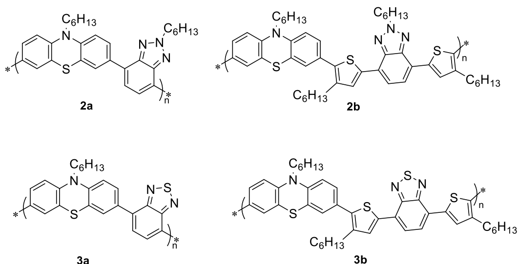
Figura 2. Strutture dei polimeri sintetizzati durante il secondo anno di progetto.
