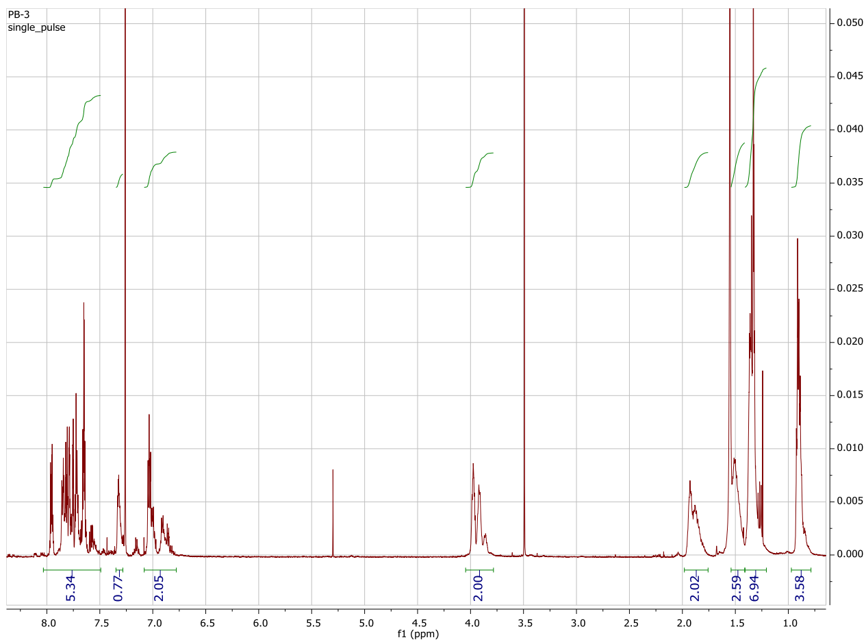
Figura 21. ^1\text{H} -NMR del Polimero 3a.
