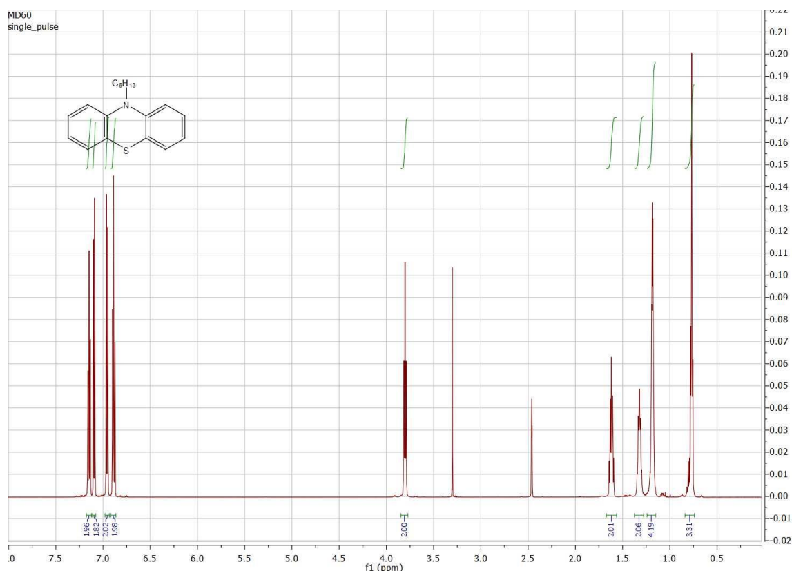
Figura 11. ^1\text{H} -NMR del Composto 4.
