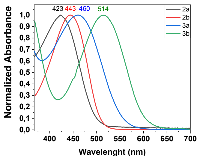
Figura 5. Spettri UV-visibile per i polimeri sintetizzati 2a-2b e 3a-3b.
