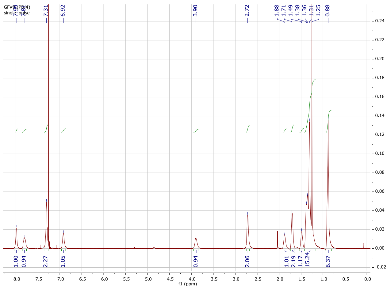
Figura 22. ^1\text{H} -NMR del Polimero 3b.
