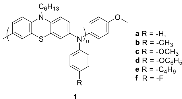
Figura. 1. Strutture dei polimeri preparati durante il primo anno.
