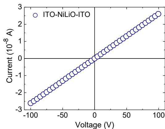
Figura 10. Grafico della misura I-V planare del contatto tra ITO e NiO:Li, essendo lineare il contatto è ohmico. L'inserto mostra lo schema del campione misurato.
