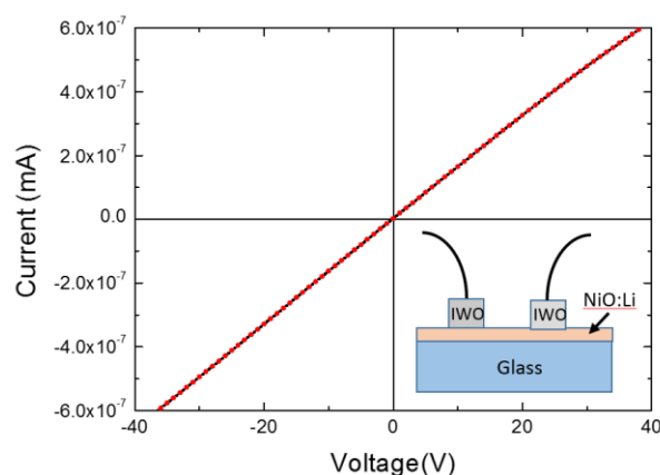
Figura 6. Misura I-V planare del contatto di IWO su film di NiO:Li, il contatto è ohmico.
