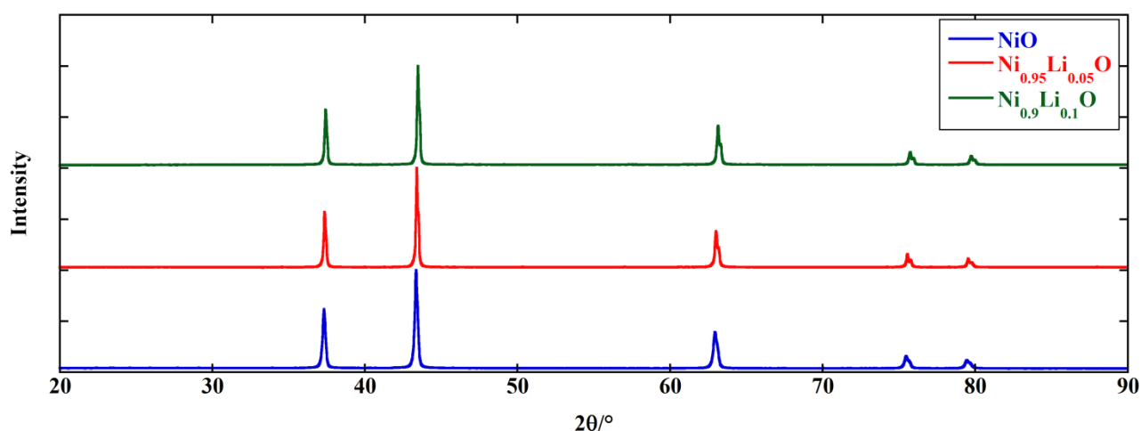
Figura 1. Diffrattogrammi di NiO puro e di NiO:Li con il 5% e 10% di Li in atomi di metallo.
