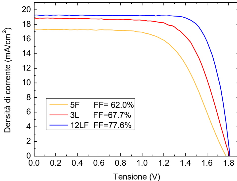
Figura 27: Caratteristiche J-V di celle tandem con la stessa cella in silicio cristallino e perovskiti a doppio catione con diversi dopanti per il PTAA: sali di litio e TBP (L), F4TCNQ (F) e la loro combinazione (LF)
