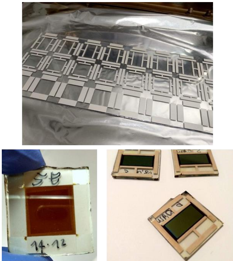
Figura 22: Layout utilizzati per definire le celle. Nella parte inferiore sono visibili il layout quadrato (sinistra) e il nuovo rettangolare (destra).
