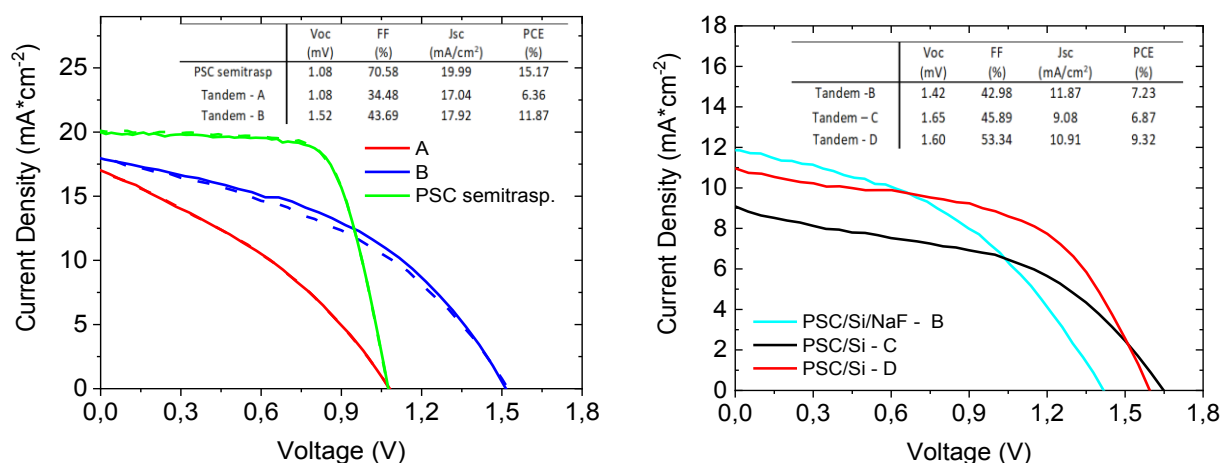
Figura 17: Curve caratteristiche J-V di dispositivi tandem perovskite /Si con cella in perovskite di tipo p-i-n. La curva J-V verde nel grafico a destra è relativa alla cella a singola giunzione in perovskite con contatto frontale semi-trasparente. Nelle tabelle sono inseriti i parametri fotovoltaici ricavati dalle curve JV.
