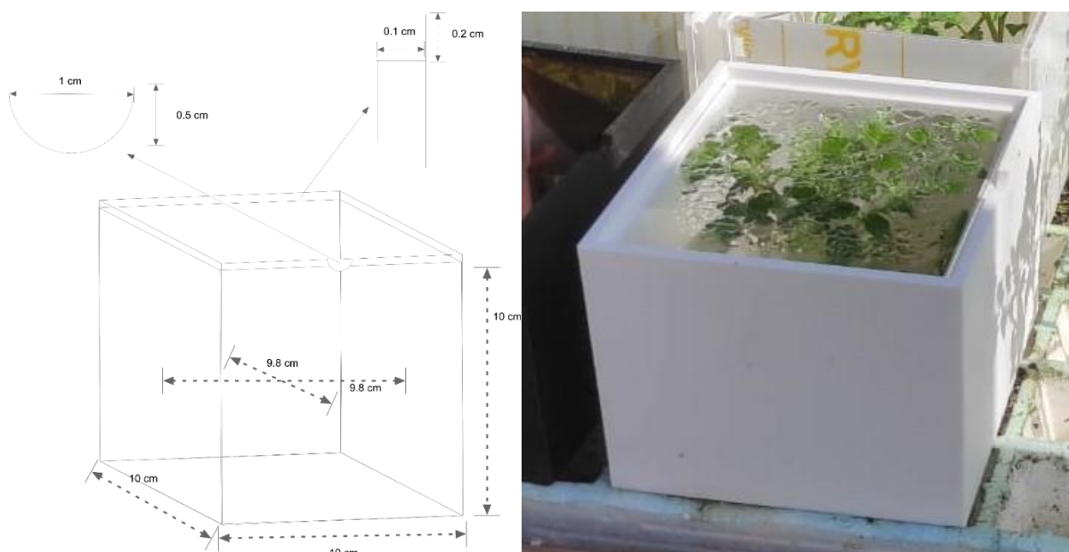
Figura 1 Box in polycarbonato progettato per la sperimentazione dei film sottili con relative misure (a sinistra). Prototipo reale di box in polycarbonato utilizzato in sperimentazione preliminare (a destra)
