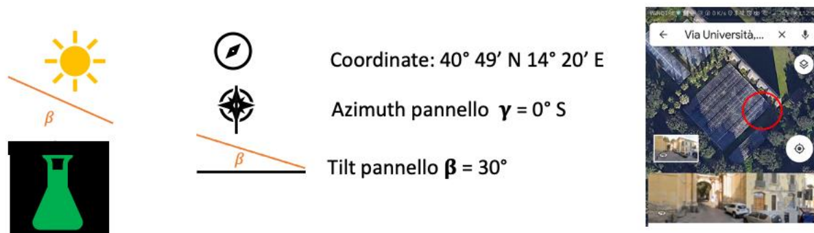
Figura 30 Schema sintetico dell'inclinazione e orientamento utilizzati risultanti di una simulazione di un pannello fotovoltaico alle coordinate della serra.
