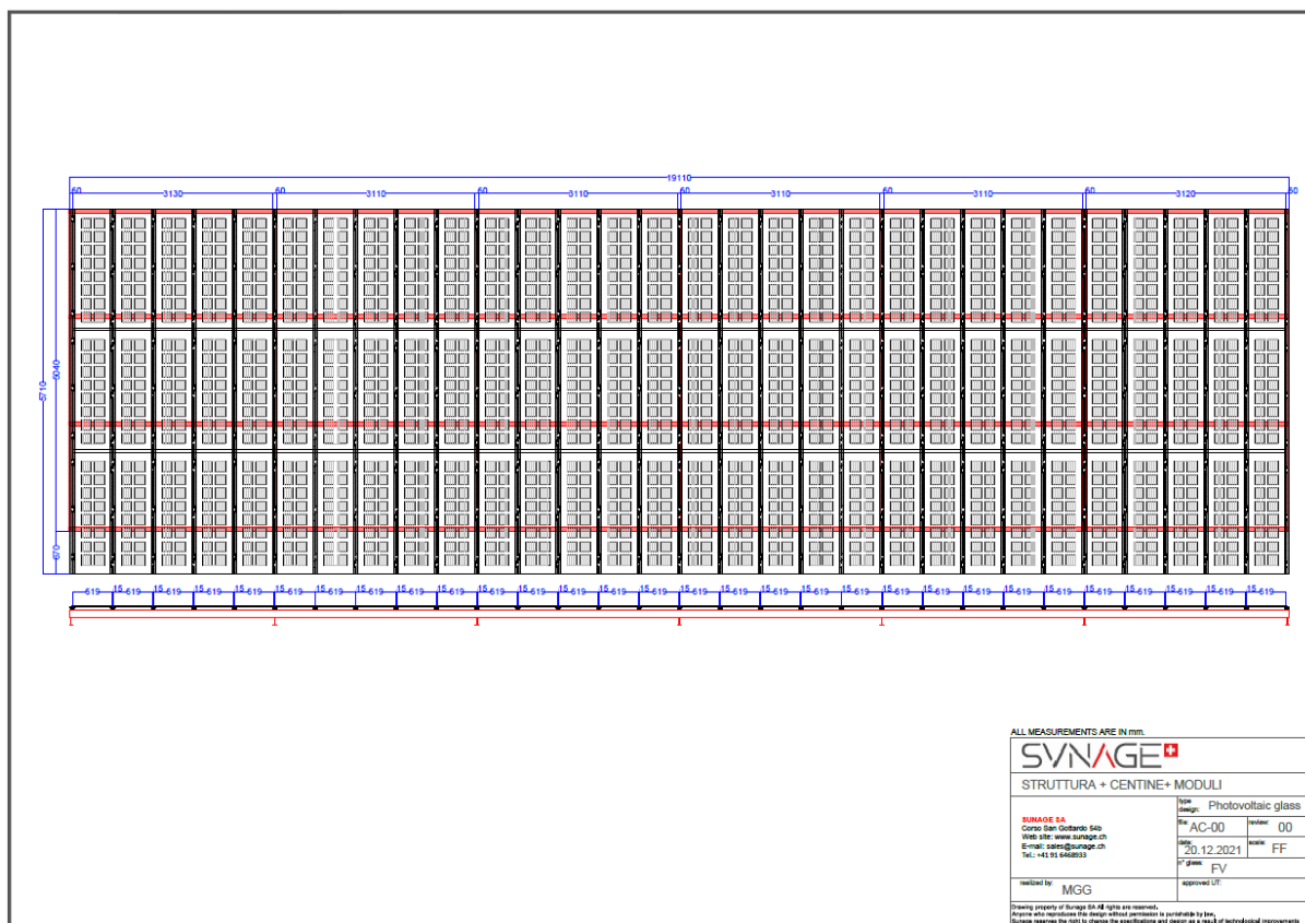
Figura 10 Dettaglio tecnico dell'intera copertura della falda sud con BIPV
