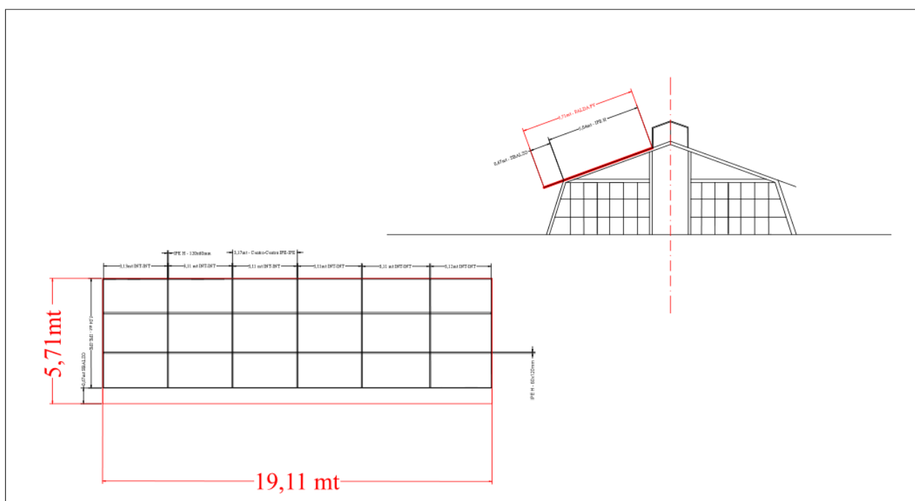
Figura 2 Rilievo architettonico della serra da ristrutturare. Dettaglio della falda sud oggetto dell’impianto fotovoltaico.
