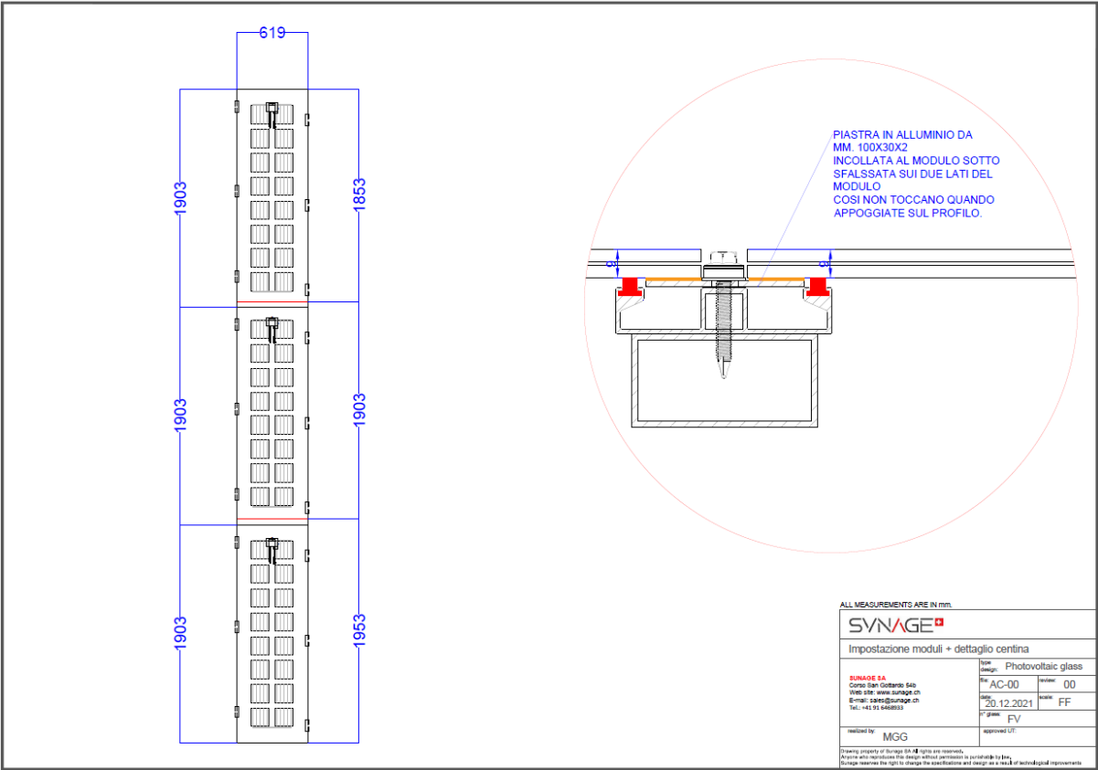
Figura 11 Dettaglio tecnico di una singola fila di pannelli BIPV e sistema di ancoraggio alla struttura
