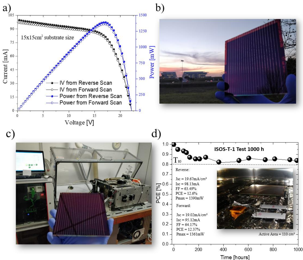
Figura 4 a) Curva I-V in e P-V del modulo campione in entrambe le scansioni (forward-reverse); b) foto del modulo campione con il rettorato in lontananza; c) foto del modulo campione con la tecnica blade/slot die utilizzata sia per la deposizione di NiOx che per la perovskite; d) stabilità termica del modulo per 1000 ore, con foto mostrante il modulo in forno.
