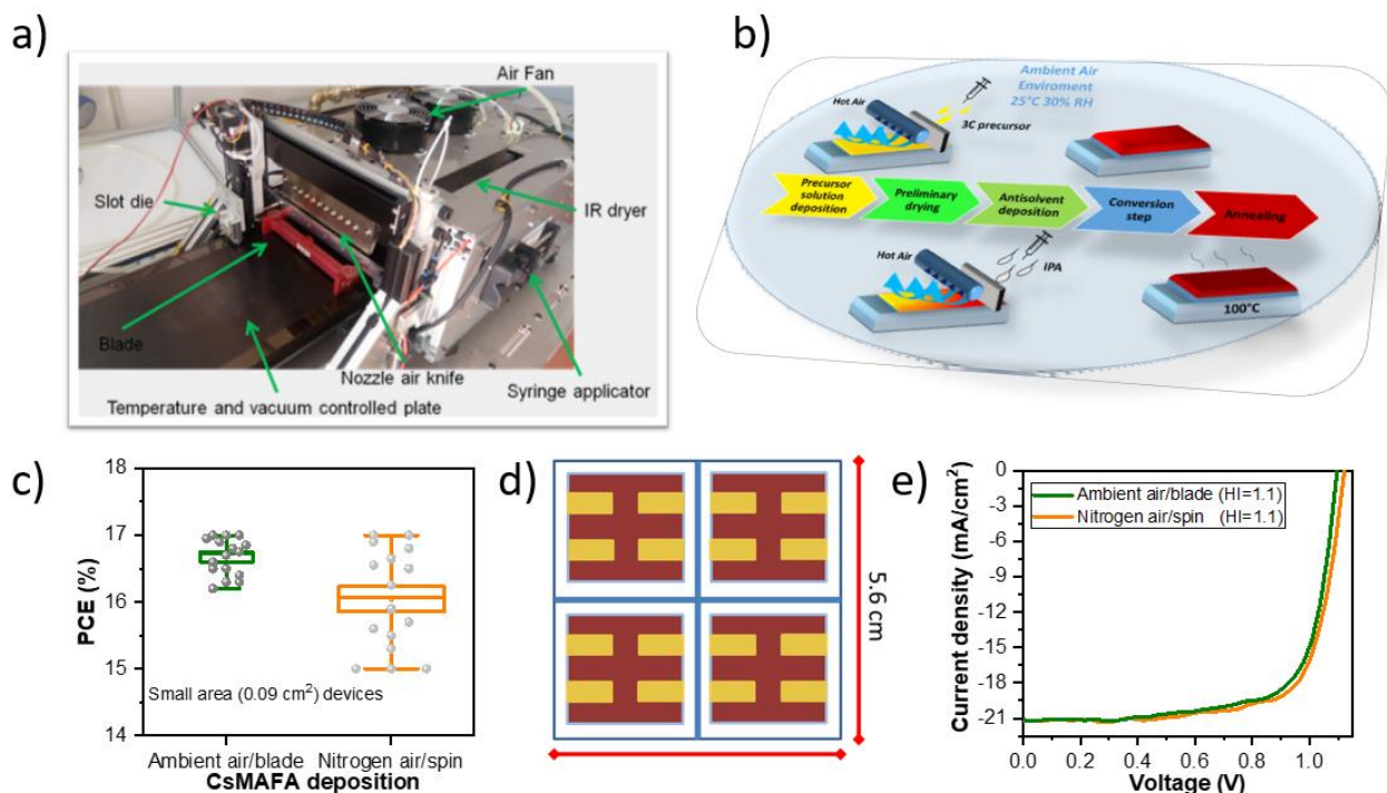
Figura 5 a) Immagine del sistema blade/slot die applicato per la deposizione della perovskite; b) schema del processo di deposizione della perovskite; c) confronto statistico delle performance ottenute con deposizione per blade/slot die fatta in aria e perovskite depositata con processo di spin coating in azoto; d) schema della geometria utilizzata per le celle di piccola area ( 0.1 \text{ cm}^2 ); e) confronto curve J-V delle due tecniche utilizzate (spin vs blade/slot die).
