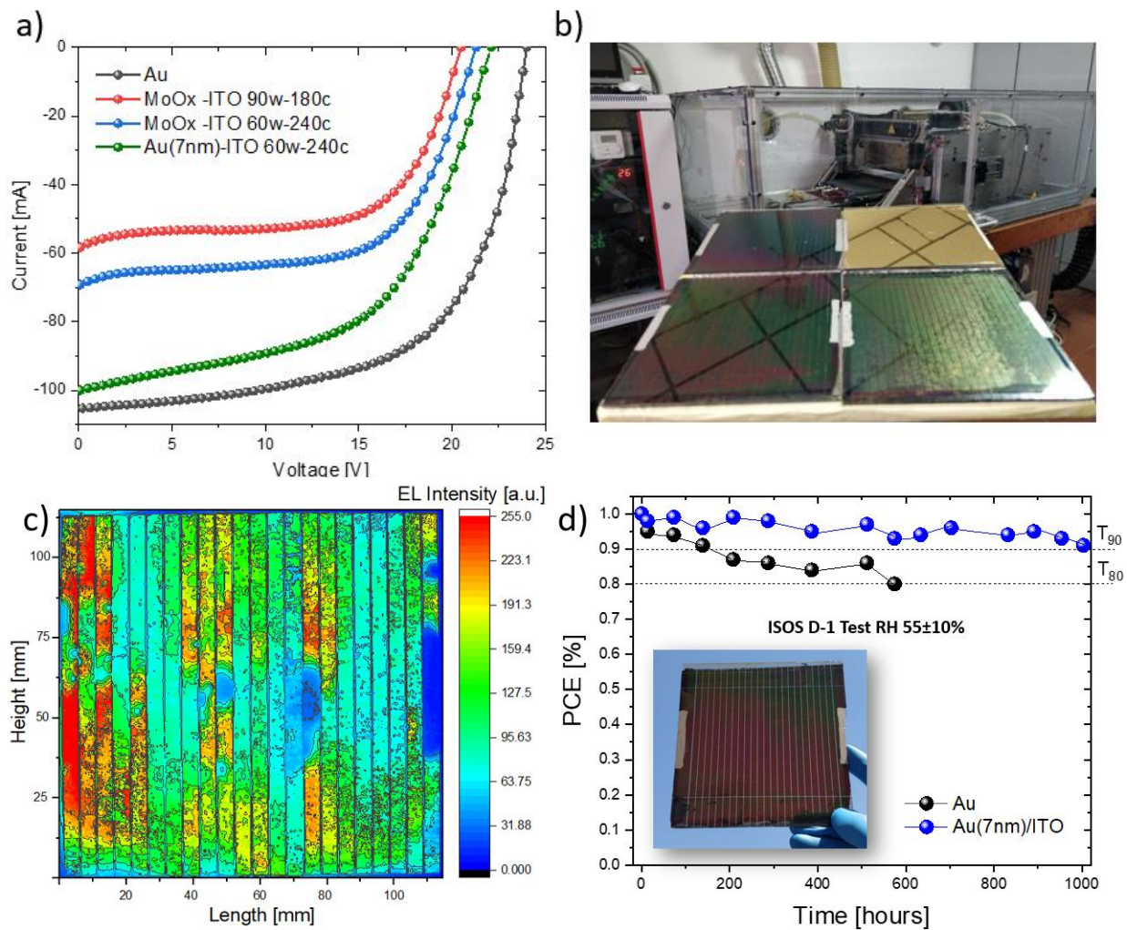
Figura 7 a) Curve I-V dei moduli campione n-i-p fabbricati; b) immagine dei moduli migliori fabbricati e nello sfondo la macchina per la deposizione dell'ETL, perovskite ed HTL; c) mappa di elettroluminescenza del modulo semi-trasparente con Au(7nm)/ITO come elettrodo superiore; d) confronto stabilità ambientale tra modulo opaco con oro e modulo semitrasparente con Au(7nm)/ITO.
