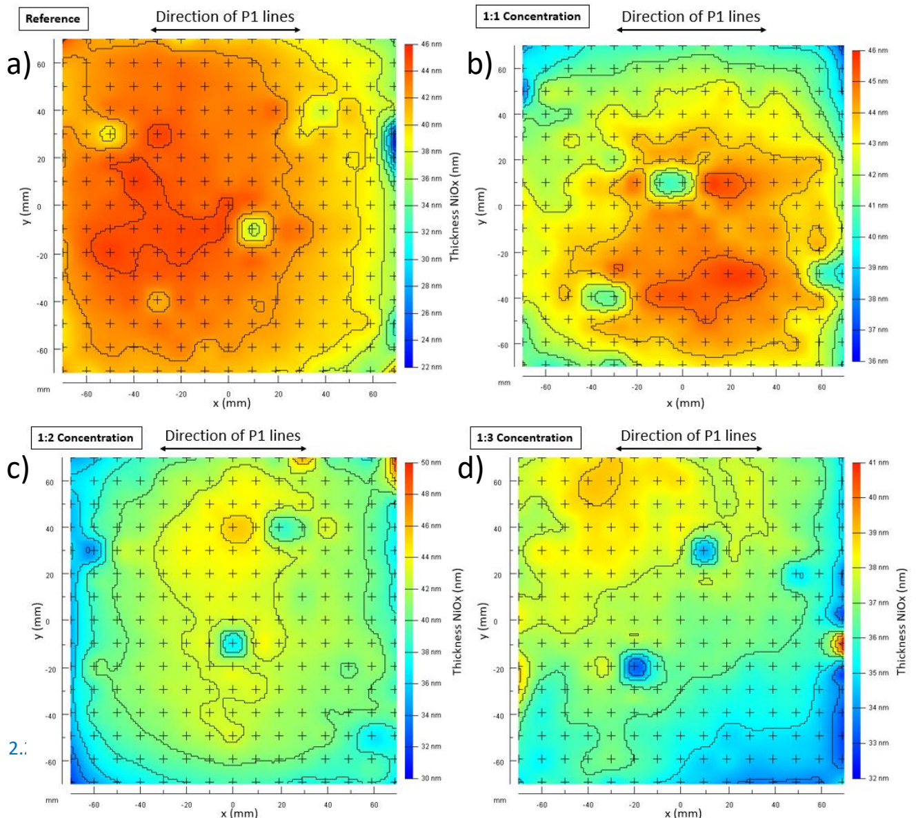
Figura 2 Mappe di Ellissometria di ossido di Nickel a diverse concentrazioni in soluzione; a) concentrazione di riferimento (reference) 0.15M; b) concentrazione con diluizione 1:1 (0.075M); c) concentrazione con diluizione 1:2 (0.05M); d) concentrazione con diluizione 1:3 (0.0375M).
