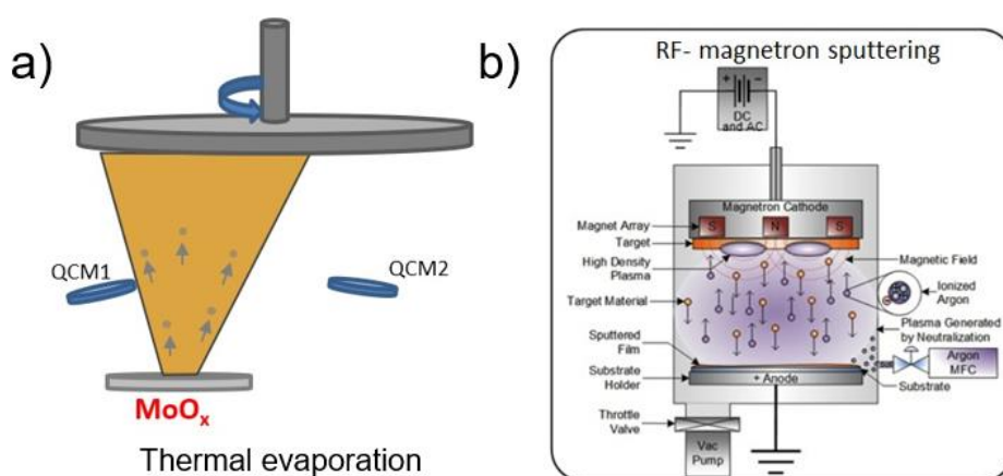
Figura 6 Schema delle due tecniche utilizzate per la fabbricazione dei moduli semi-trasparenti. a) schema della deposizione mediante evaporazione termica dell'ossido di molibdeno usato come buffer layer tra HTL e ITO; b) schema della deposizione di ITO avvenuta mediante tecnica di sputtering.
