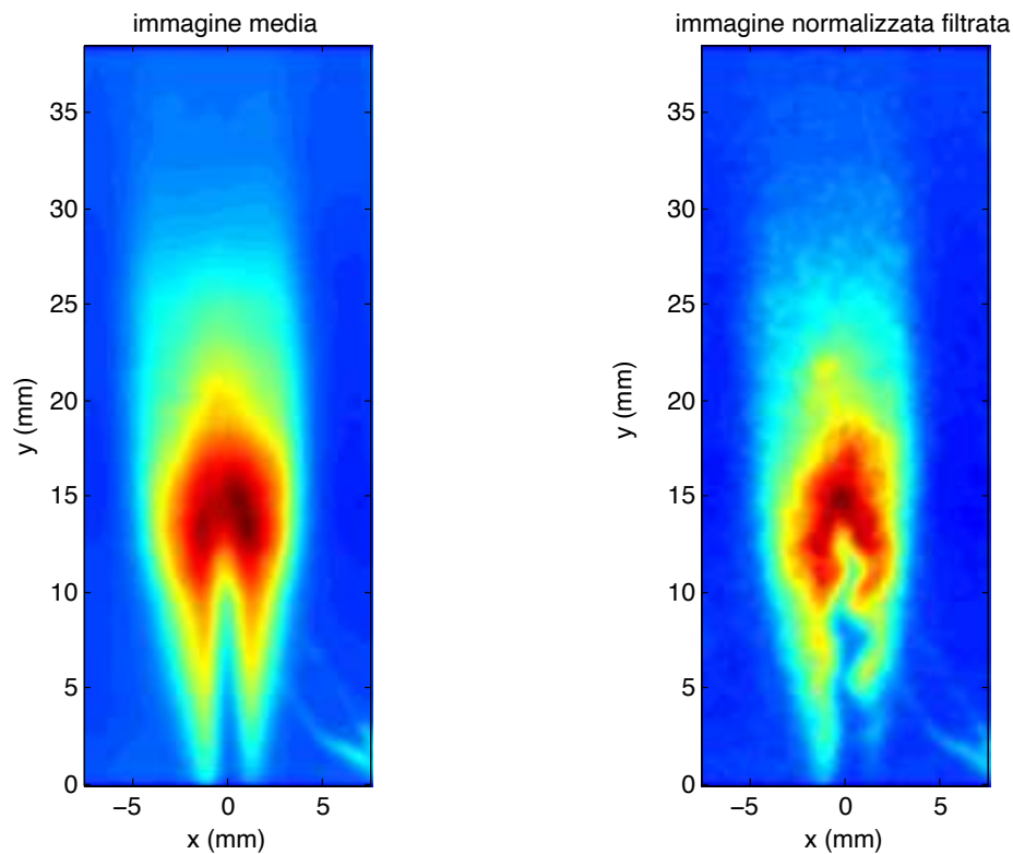
Figura 4 Fiamma esperimento 2. Sinistra, fiamma media. Destra, fiamma istantanea.
