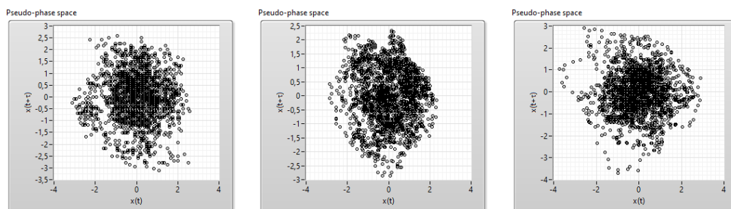
Figura 16 Spazio delle pseudo fasi per le configurazioni stabili 0% (metano puro), 50% e 60% di idrogeno, da sinistra verso destra. Segnale di pressione.
