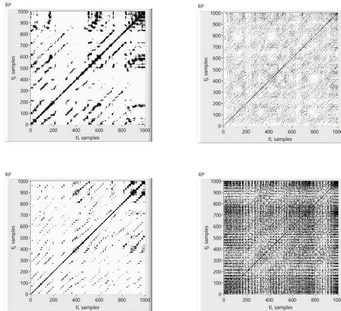
Figura 14 Recurrence plot fiamme stabili riportate in Tabella 3: prima riga, 0% idrogeno; seconda riga 60% di idrogeno. Prima colonna energia radiante, seconda colonna pressione.
