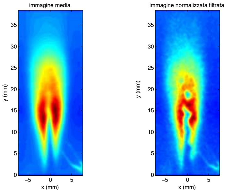
Figura 3 Fiamma esperimento 1. Sinistra, fiamma media. Destra, fiamma istantanea.
