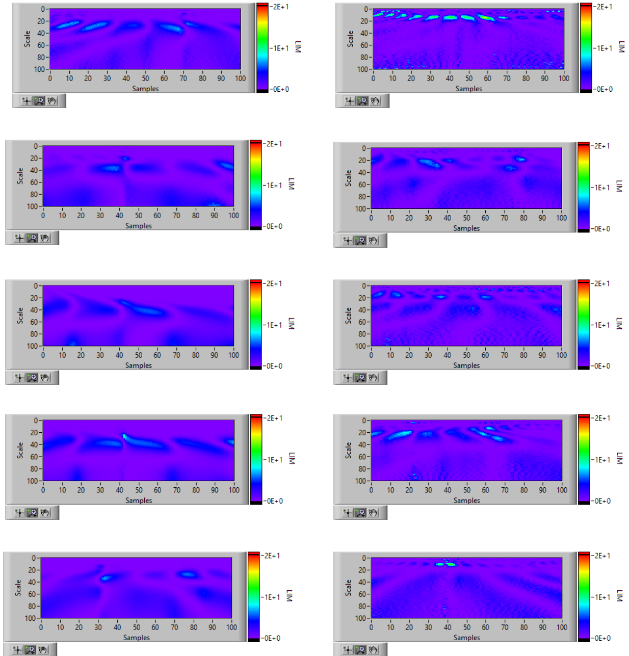
Figura 10 Scalogramma per le diverse configurazioni stabili elencate in Tabella 3. Prima colonna, segnale di chemiluminescenza nella banda del vicino infrarosso (900-2750 nm); seconda colonna, segnale di pressione. In ascissa è riportato il tempo di campionamento espresso in campioni, in ordinata la scala r del coefficiente wavelet w(r,t) , mentre i colori indicano il modulo di w(r,t) normalizzato con la sua varianza.
