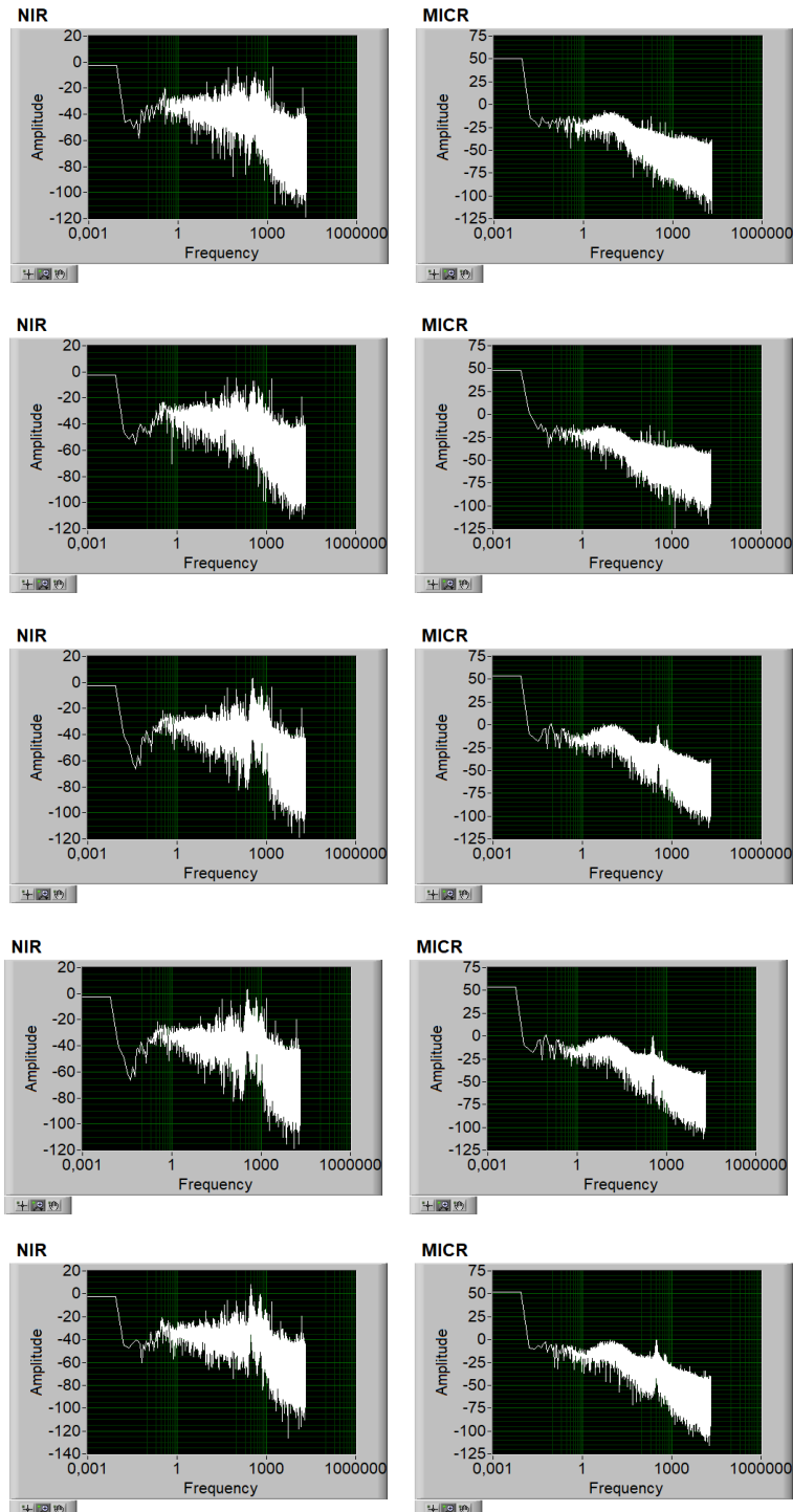
Figura 12 Analisi spettrale fiamme stabili nel regime di rumore di combustione, elencate in Tabella 3. Nella colonna di sinistra sono riportate le emissioni luminose nella banda del vicino infrarosso (900-2750 nm). In quella di destra il segnale registrato dal microfono.
