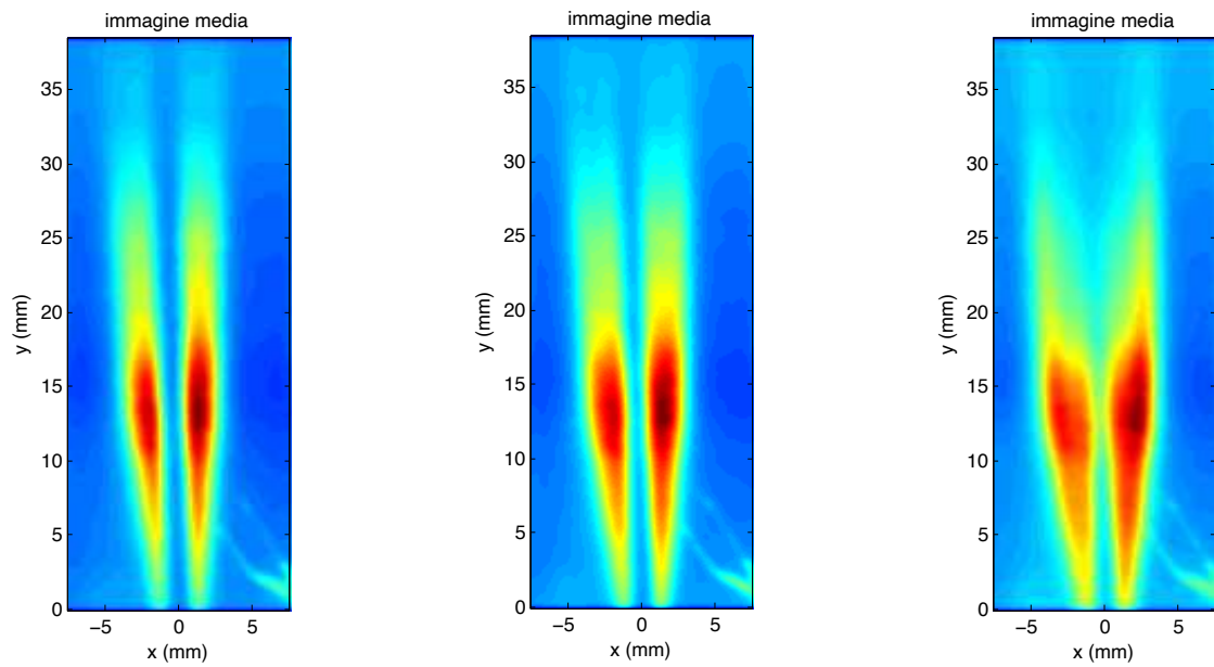
Figura 5 Fiamme medie relative agli esperimenti 3, 4, 5 da sinistra verso destra. Rapporto di equivalenza magro pari a 0.6 e tenore crescente di idrogeno, da sinistra verso destra, metano puro, 50% e 85% di idrogeno.
