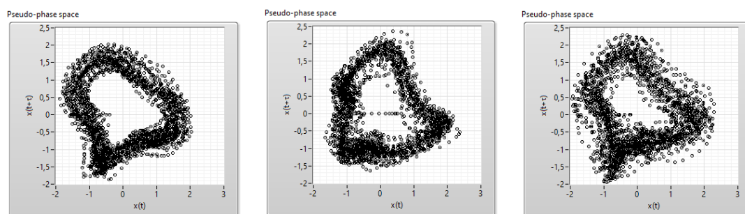
Figura 17 Spazio delle pseudo fasi per le configurazioni instabili 0% (metano puro), 50% e 60% di idrogeno, da sinistra verso destra. Segnale di pressione.
