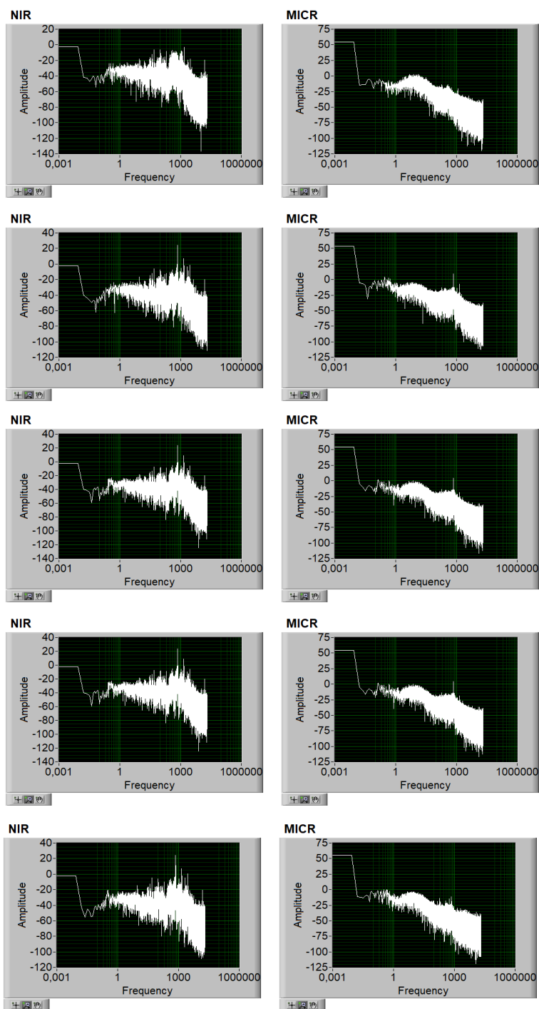
Figura 13 Analisi spettrale fiamme instabili nel regime di instabilità termoacustica, elencate in Tabella 4. Nella colonna di sinistra sono riportate le emissioni luminose nella banda del vicino infrarosso (900-2750 nm). In quella di destra il segnale registrato dal microfono.
