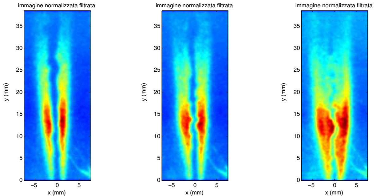
Figura 6 Fiamme istantanee relative agli esperimenti 3, 4, 5 da sinistra verso destra. Rapporto di equivalenza magro pari a 0.6 e tenore crescente di idrogeno, da sinistra verso destra, metano puro, 50% e 85% di idrogeno.
