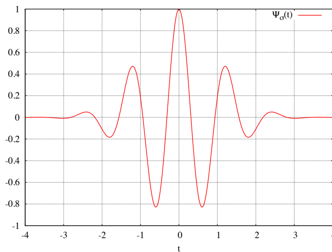
Figura 9 Mother wavelet di tipo Morlet.
