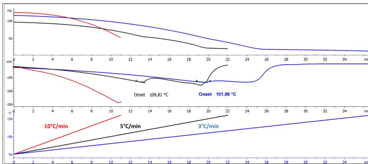
Figura 19 – Analisi TGA formazione dello ioduro di stagno, partendo da \text{SnO}_2 ed utilizzando HI 57% in peso: dall'alto verso il basso sono riportate le curve gravimetriche, le curve calorimetriche e le rampe di temperatura utilizzate (3°C/min, 5°C/min e 10°C/min, carrier gas \text{N}_2 40 Nml/min).
