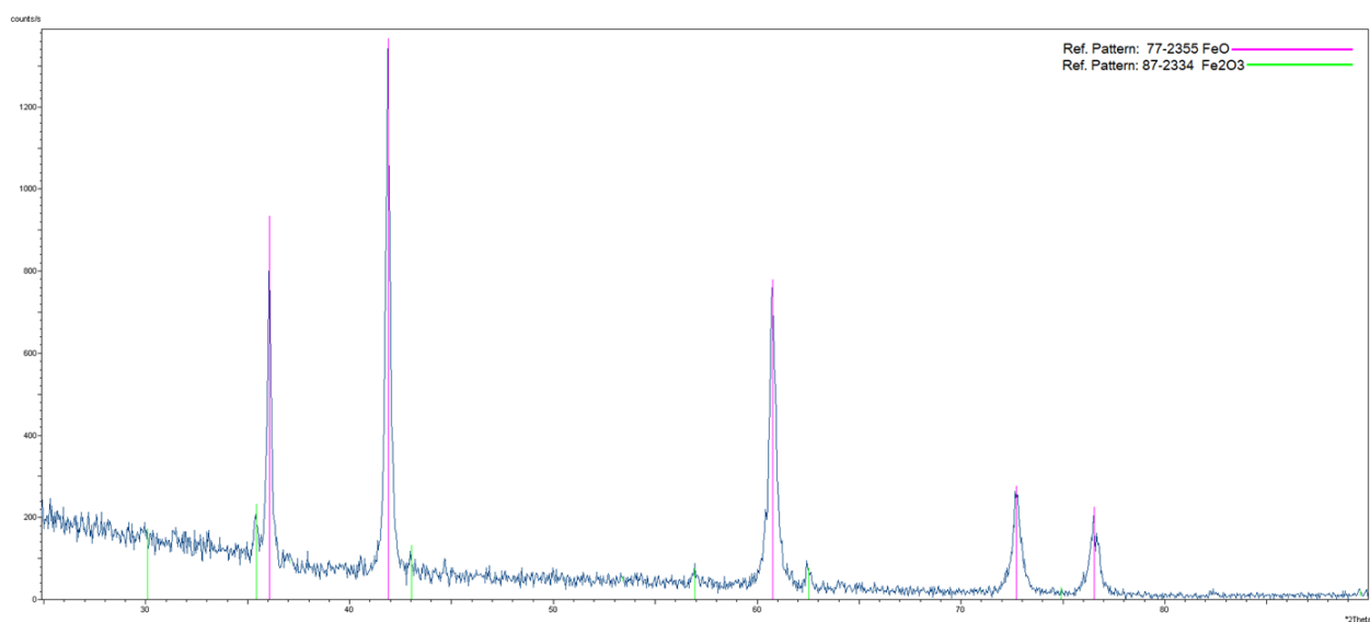
Figura 26– Diffrattogramma dello ioduro di ferro(II) commerciale utilizzato per produrre \text{FeI}_2
