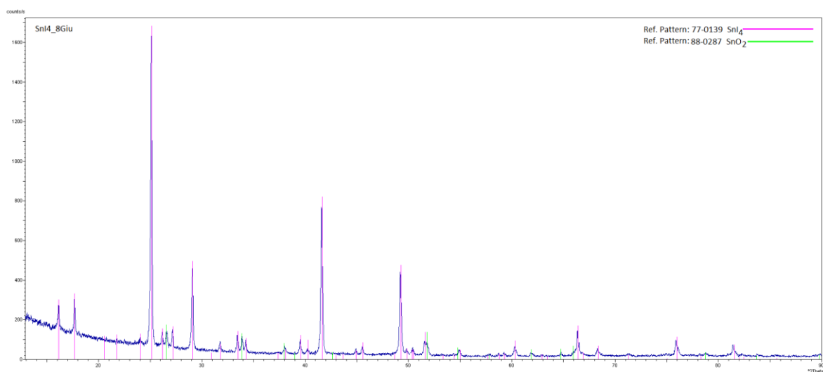
Figura 17 - Diffrattogramma del prodotto di sintesi in un reattore in pirex a livello di laboratorio dello ioduro di stagno (IV) a partire da \text{SnO}_2 e HI (Eq. 17) in maniera stechiometrica; dall'analisi si rileva la presenza sia di \text{SnI}_4 che di ossido di stagno (IV) non reagito.
