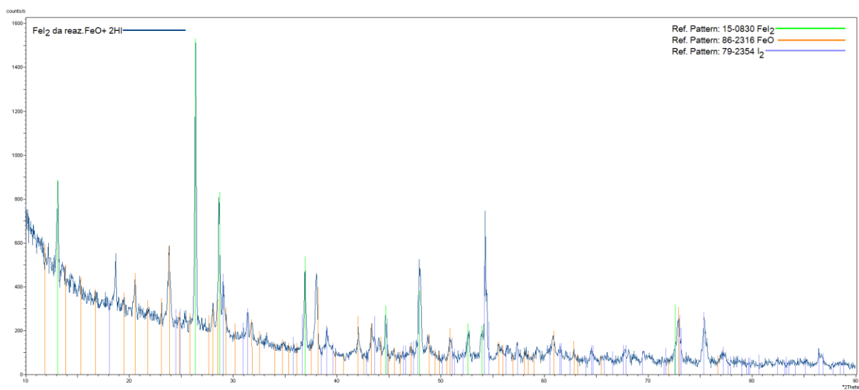
Figura 27– Diffrattogramma prodotto della reazione stechiometrica \text{FeO} + 2\text{HI} (al 57% in peso).
