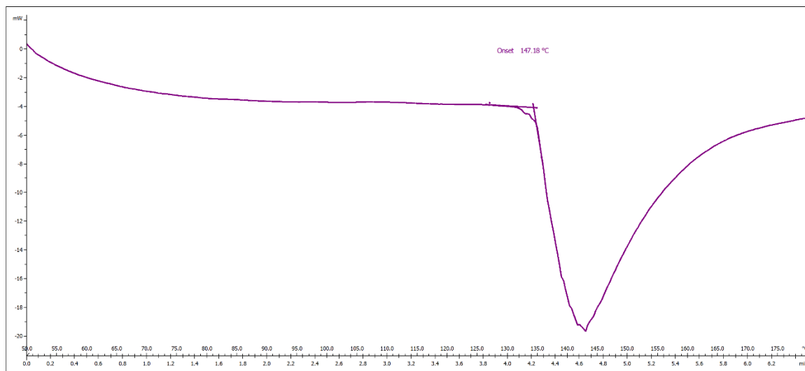
Figura 18 – DTA sul prodotto di sintesi del \text{SnI}_4 : il punto di fusione del prodotto ottenuto risulta uguale a circa 144°C, cioè l'onset previsto per l' \text{SnI}_4 (rampa 10°C/min/ carrier gas \text{N}_2 50 Nml/min)
