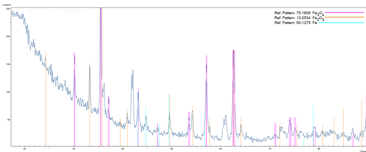
Figura 31– Diffratogramma prodotto della decomposizione termica di FeI 2 , contenente FeO residuo (flusso N 2 40 NmI/min).
