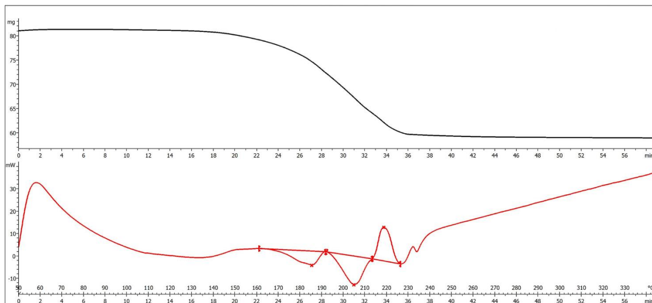
Figura 1 – TGA/DTA pattern della reazione stechiometrica di formazione del solfato di stagno partendo da Sn + 2H 2 SO 4 (carrier gas aria, 50 Nml/min)
