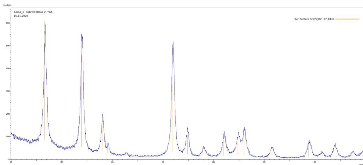
Figura 5 – Diffrattogramma del prodotto di decomposizione dello stagno solfato (partendo da \text{Sn} + 2\text{H}_2\text{SO}_4 ): l'analisi mostra la sola presenza di \text{SnO}_2
