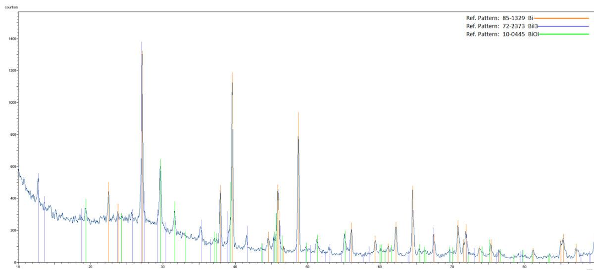
Figura 34– Diffrattogramma residuo reazione fra Bi e acido iodidrico (Bi:HI 1:3) ottenuto come illustrato in Figura 33.
