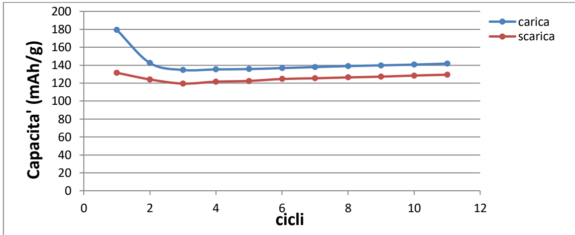
Fig. 6: Capacità specifica per una batteria al sodio con catodo a base di \text{Na}_{0.84}\text{Li}_{0.1}\text{Ni}_{0.27}\text{Mn}_{0.63}\text{O}_2 testato nell'intervallo di voltaggio tra 2.1V-4.5V
