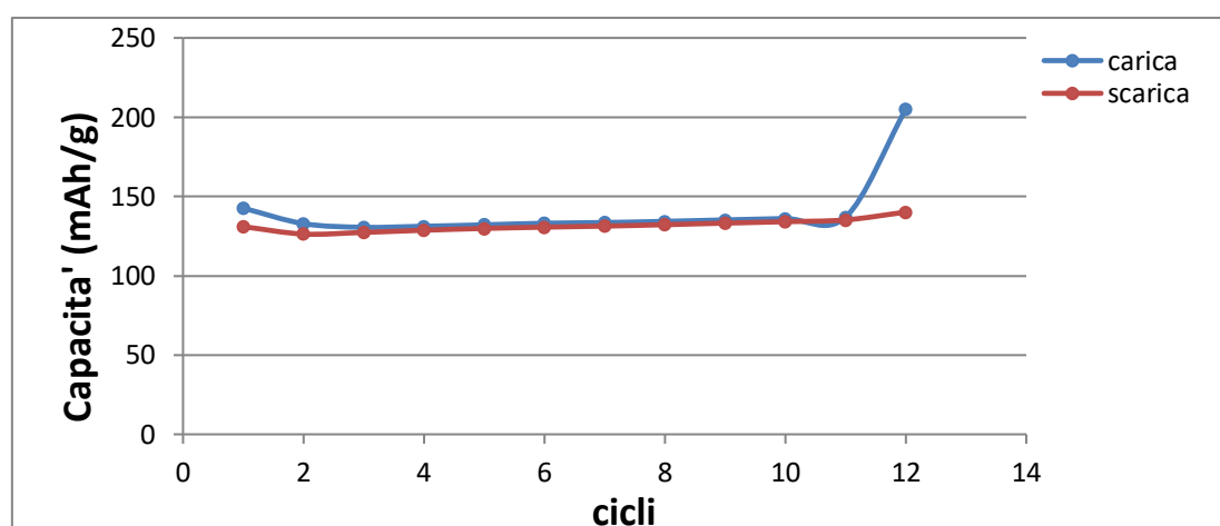
Fig. 10: Capacità specifica per una batteria con catodo a base di \text{Na}_{0.84}\text{Li}_{0.1}\text{Ni}_{0.27}\text{Mn}_{0.63}\text{O}_2 testato nell'intervallo di voltaggio tra 1.5V-4.5V
