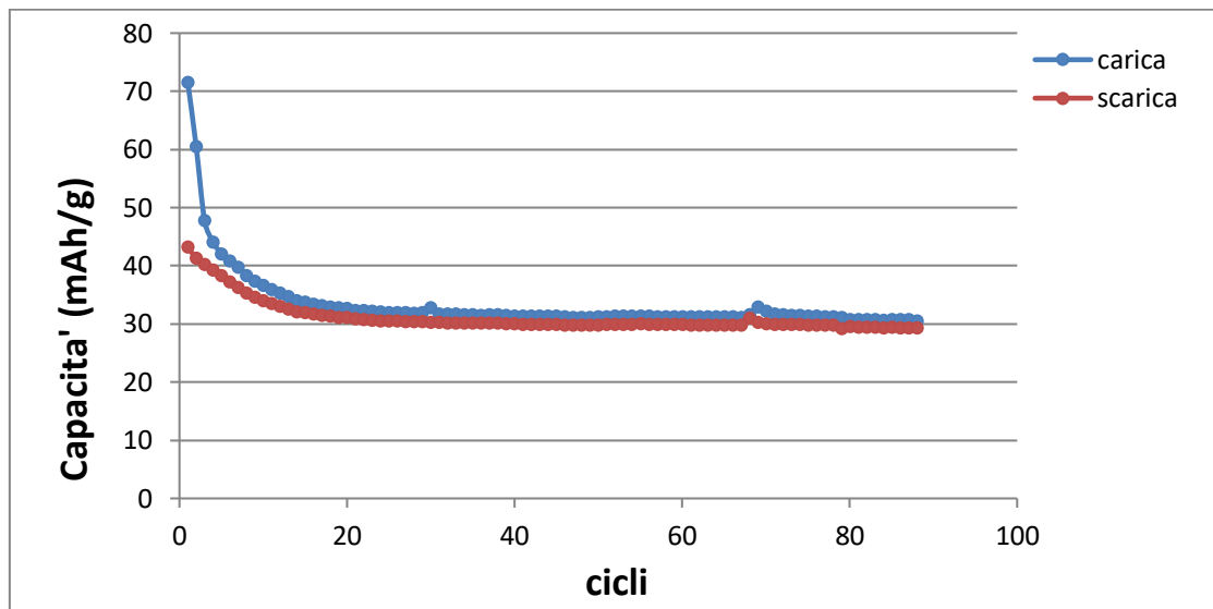
Fig. 14: capacità specifiche per una batteria al sodio con elettrolita \text{NaClO}_4 1M in EMITFSI
