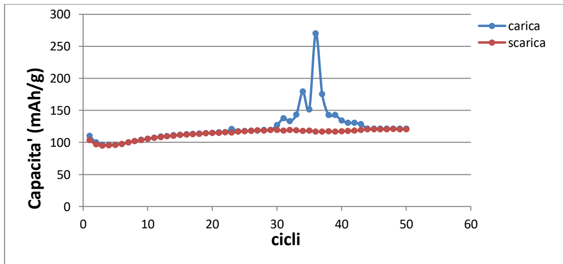
Fig. 8: Capacità specifica per una batteria al sodio con catodi a base di \text{Na}_{0.84}\text{Li}_{0.1}\text{Ni}_{0.27}\text{Mn}_{0.63}\text{O}_2 testato nell'intervallo di voltaggio tra 1.5V-4.1V
