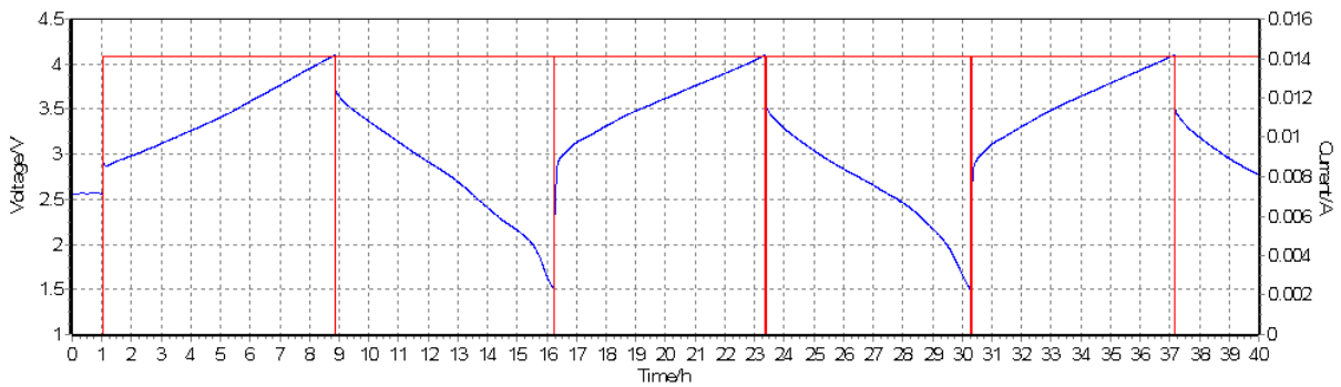
Fig. 7 ciclagioni galvanostatiche per una batteria al sodio con catodo a base di \text{Na}_{0.84}\text{Li}_{0.1}\text{Ni}_{0.27}\text{Mn}_{0.63}\text{O}_2 in un intervallo di voltaggio tra 1.5V-4.1V
