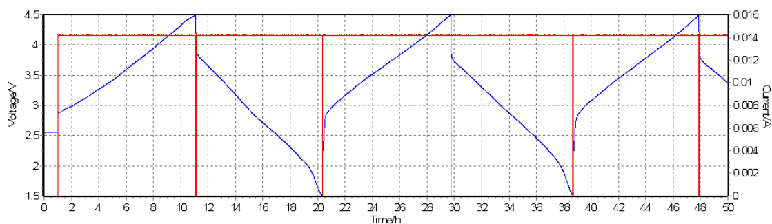
Fig. 9 ciclaggi galvanostatici per una batteria al sodio con catodo a base di \text{Na}_{0.84}\text{Li}_{0.1}\text{Ni}_{0.27}\text{Mn}_{0.63}\text{O}_2 in un intervallo di voltaggio tra 1.5V-4.5V
