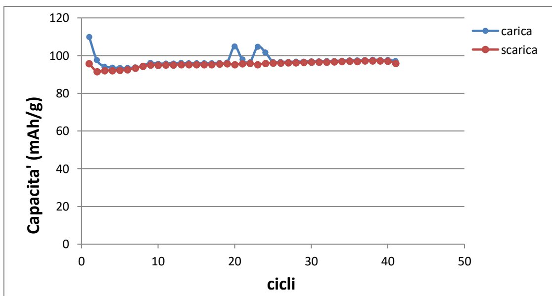
Fig. 2: Capacità specifica per una batteria al sodio con catodo a base di \text{Na}_{0.84}\text{Li}_{0.1}\text{Ni}_{0.27}\text{Mn}_{0.63}\text{O}_2 testato nell'intervallo di voltaggio tra 2.1V-4.1V
