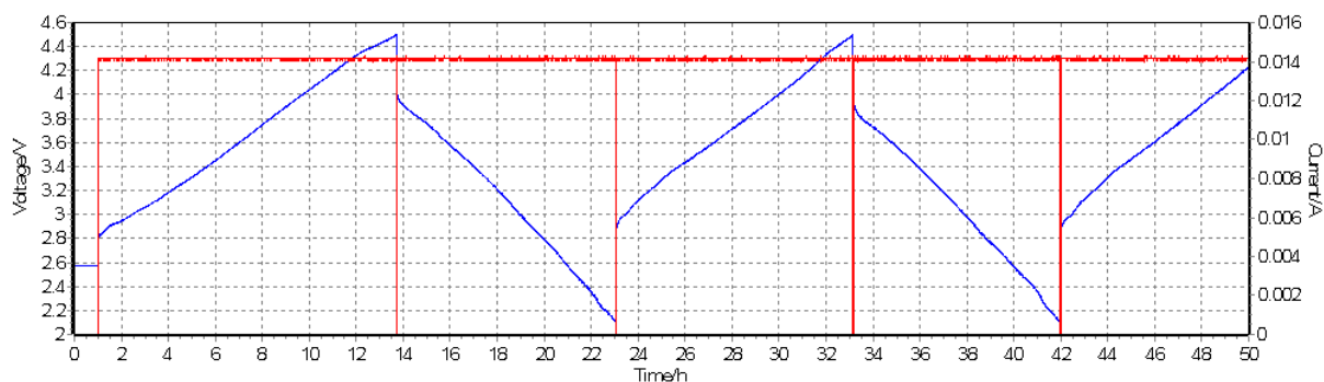
Fig. 5 ciclagioni galvanostatiche per una batteria al sodio con catodo a base di \text{Na}_{0.84}\text{Li}_{0.1}\text{Ni}_{0.27}\text{Mn}_{0.63}\text{O}_2 in un intervallo di voltaggio tra 2.1V-4.5V
