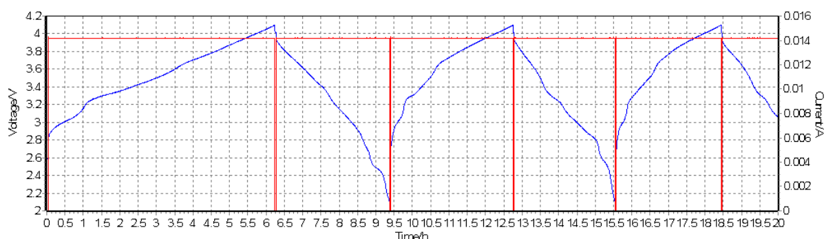
Fig. 11: ciclazioni galvanostatiche per una batteria al sodio con elettrolita \text{NaClO}_4 1M in EMIFS
