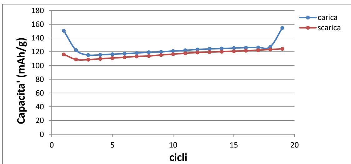
Fig. 4: Capacità specifica per una batteria al sodio con catodo a base di \text{Na}_{0.84}\text{Li}_{0.1}\text{Ni}_{0.27}\text{Mn}_{0.63}\text{O}_2 testato nell'intervallo di voltaggio tra 2.1V-4.3V
