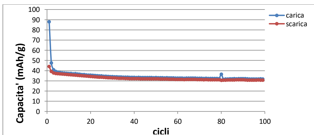
Fig. 12: capacità specifiche per una batteria al sodio con elettrolita \text{NaClO}_4 1M in EMIFS
