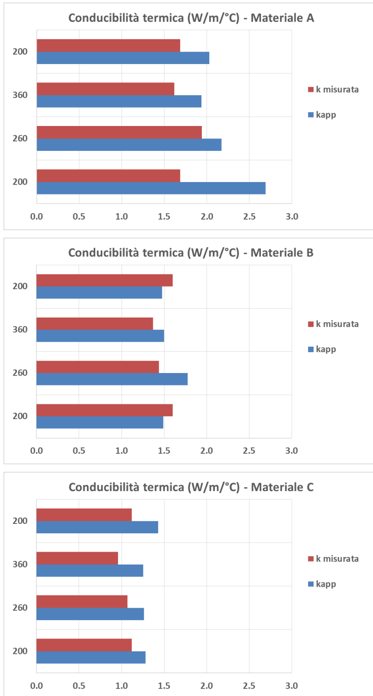
Figura 3-11 Conducibilità termica apparente e misurata in funzione del tipo di materiale e della temperatura operativa.
