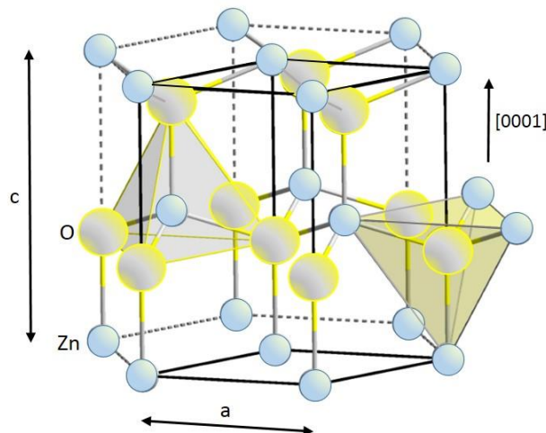
Figura 3. Struttura esagonale del cristallo di wurzite.
