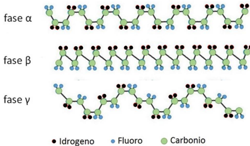
Figura 2. Conformazione molecolare delle fasi \alpha , \beta , \gamma del PVDF.
