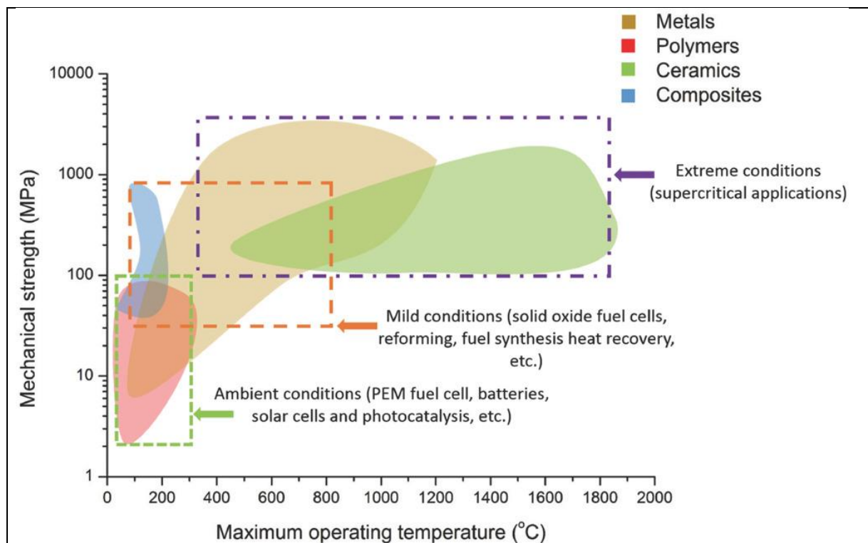
Figura 8. Confronto di materiali strutturali in AM in termini di resistenza meccanica e massima temperatura operativa [49].
