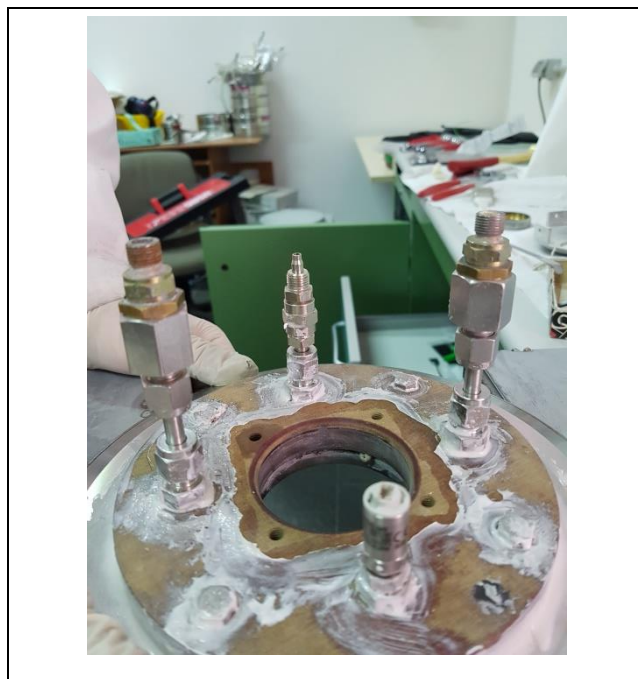
Figura 23. Alloggiamento di bachelite della torcia
