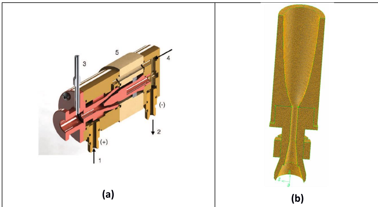
Figura 22. Estensione dell'ugello per il confinamento del plasma
