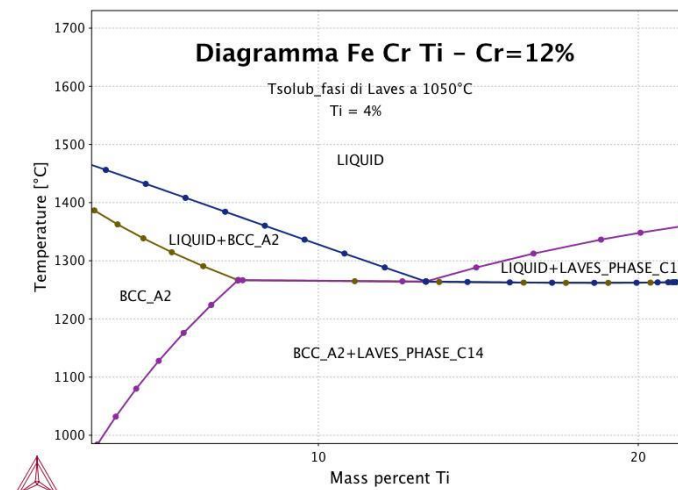
Figura 11 Diagramma pseudo-binario del sistema Fe 12 Cr xTi
