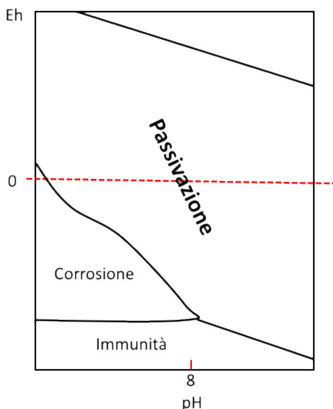
Figura 7 Schema del Diagramma di Pourbaix teorico del Titanio in acqua a 25°C
