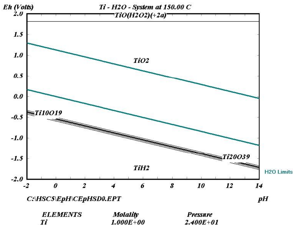
Figura 4 Diagramma di Pourbaix del Titanio in soluzione acquosa a 150°C e a pressione pari 24 bar
