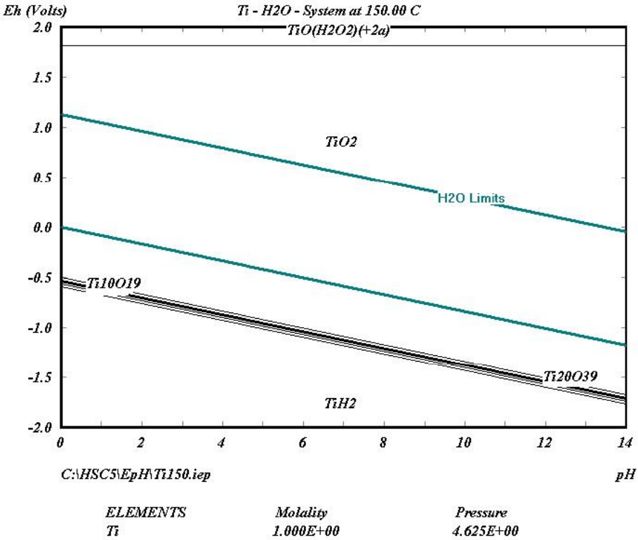
Figura 3 Diagramma di Pourbaix del Titanio in soluzione acquosa a 150°C e a pressione pari alla tensione di vapore dell'acqua alla stessa temperatura
