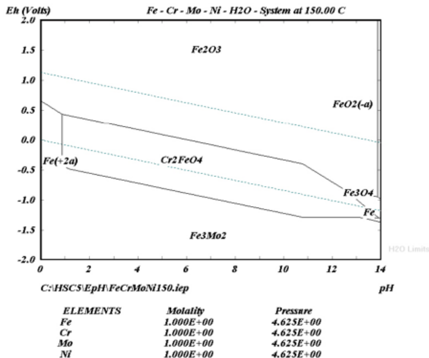
Figura 10 Diagramma di Pourbaix del sistema FeCrNiMo a 150°C - 4.62 bar in soluzione acquosa, nel quale si passa dalla Cromite ( \text{Cr}_2\text{FeO}_4 ) al dominio della magnetite ( \text{Fe}_3\text{O}_4 )
