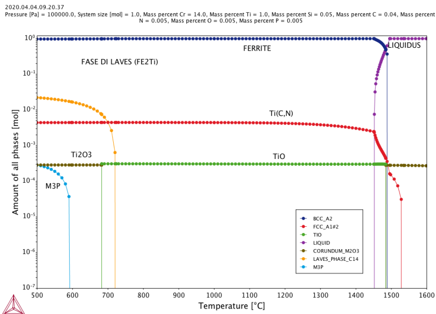
Figura 15 Stepped Calculation Graph (Thermocalc) relativo alla composizione con Ti = 1%
