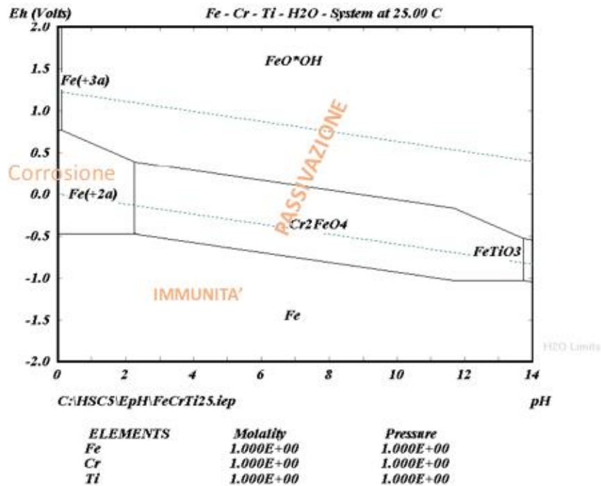
Figura 8 Diagramma di Pourbaix del sistema FeCrTi a 25°C- 1bar in soluzione acquosa
