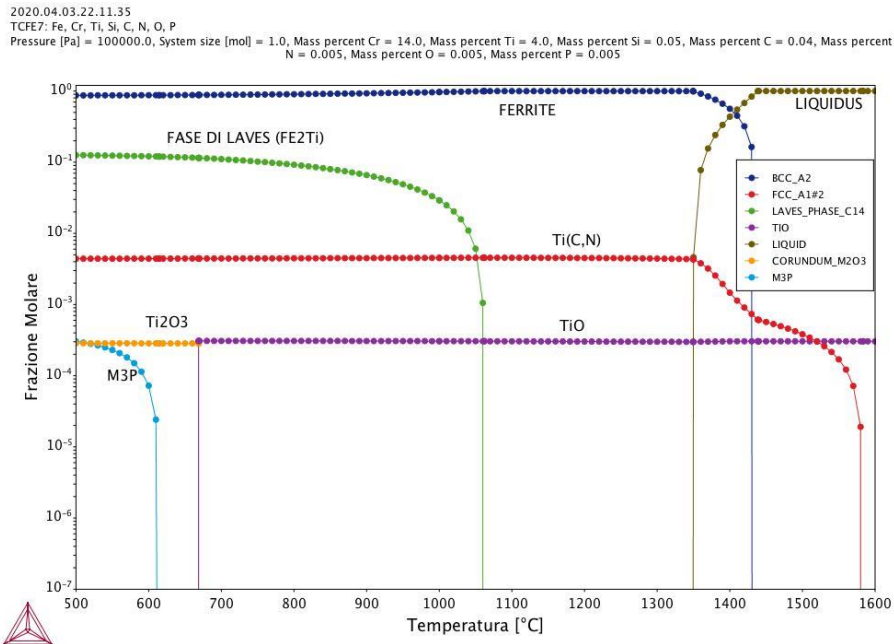
Figura 13 Stepped Calculation Graph (Thermocalc) relativo alla composizione desiderata
