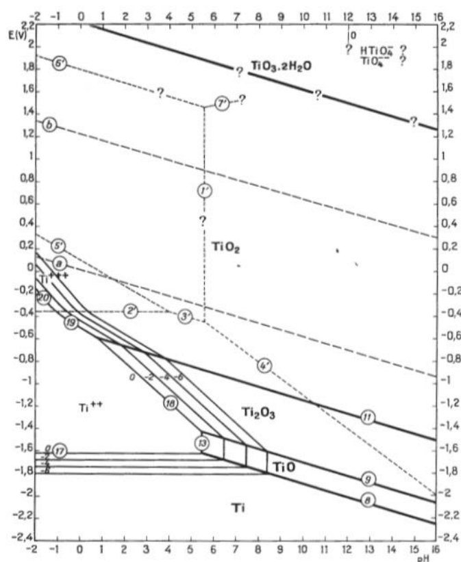
Figura 6 Diagramma di Pourbaix teorico del Titanio in acqua a 25°C [23]
