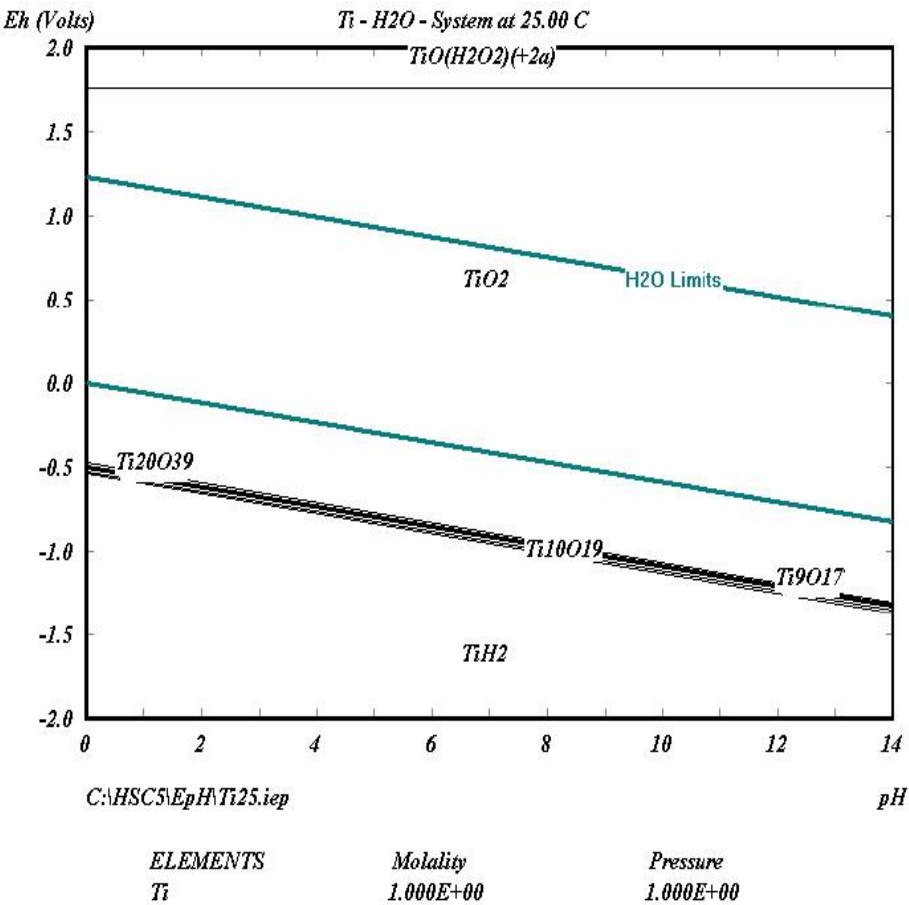
Figura 2 Diagramma di Pourbaix del Titanio in soluzione acquosa a 25°C e a pressione atmosferica
