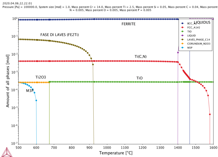
Figura 14 Stepped Calculation Graph (Thermocalc) relativo alla composizione con Ti = 2.5%
