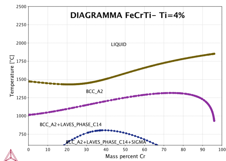
Figura 12 Diagramma pseudo-binario del sistema Fe 4Ti xCr
