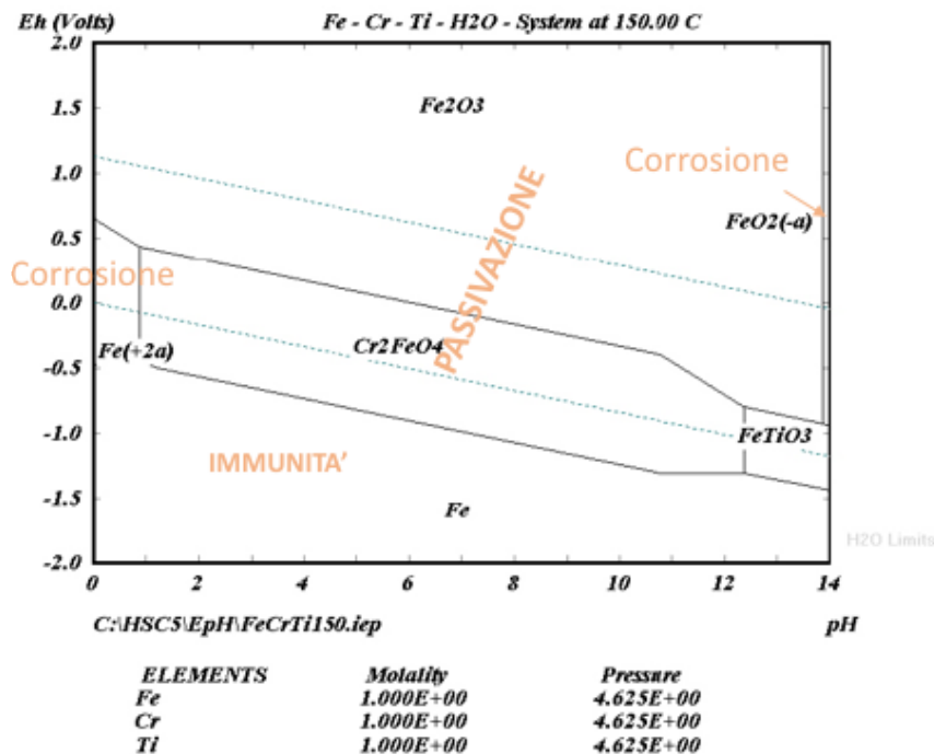
Figura 9 Diagramma di Pourbaix del sistema FeCrTi a 150°C - 4.62 bar in soluzione acquosa
