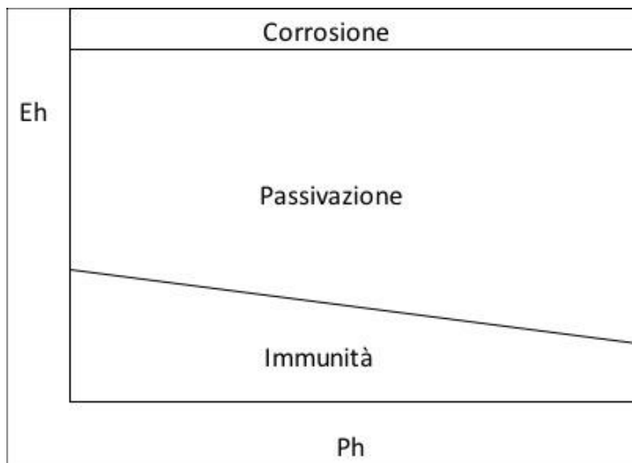
Figura 5 Schema del Diagramma di Pourbaix del Titanio in soluzione acquosa
