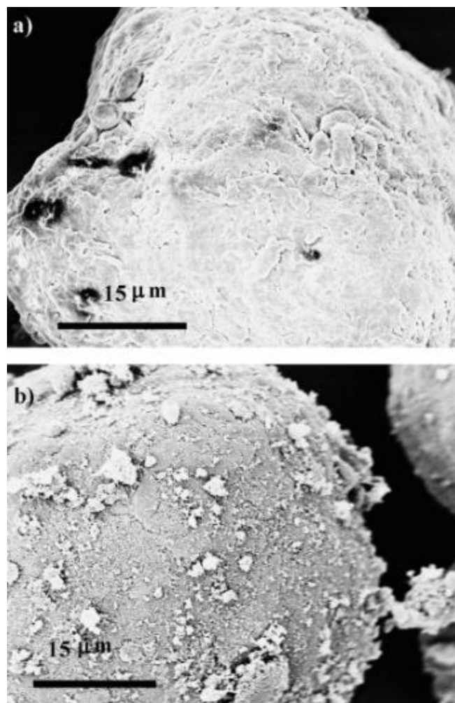
Figura 9 Immagini SEM di (a) polvere di Nylon-12 e (b) polvere di Nylon-12 miscelata con carbon black [94].
