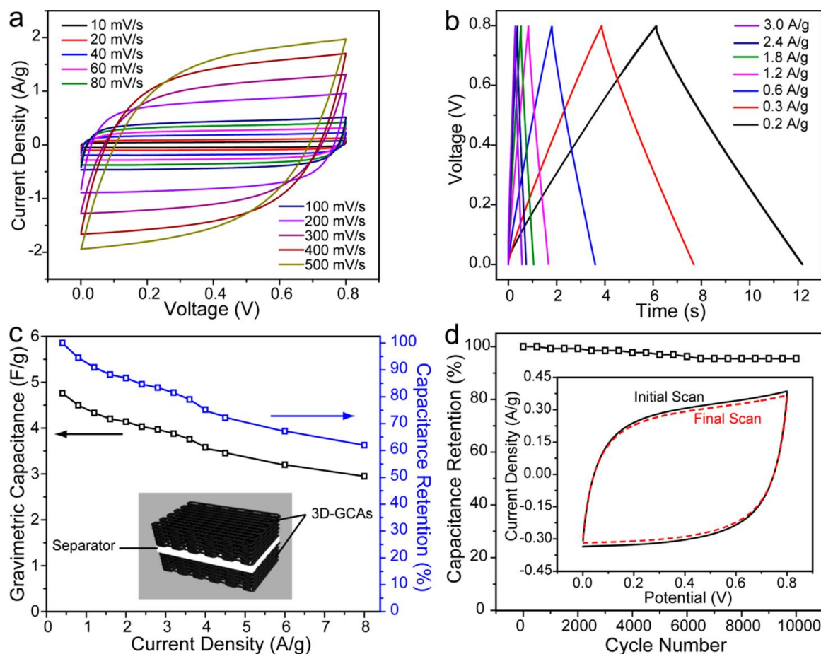
Figura 11 Performance elettrochimiche del dispositivo a base di grafene stampato in 3D (3D-GCA) [109].
