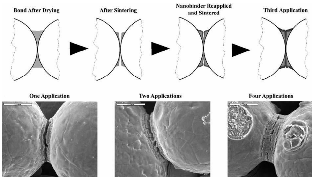
Figura 7 Illustrazione schematica della riparazione del legame mediante l'applicazione multipla di nanobinder ed immagini dei legami, sinterizzati a 700 °C, di campioni sottoposti ad un numero diverso di applicazioni di nanobinder ed essiccati tramite campo magnetico [91].
