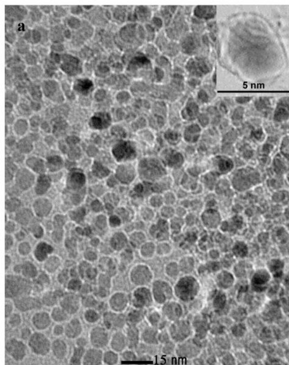
Figura 2 Immagini TEM di nanoparticelle costituite dalla lega FeCo ricoperte da pochi strati di grafene [88].
