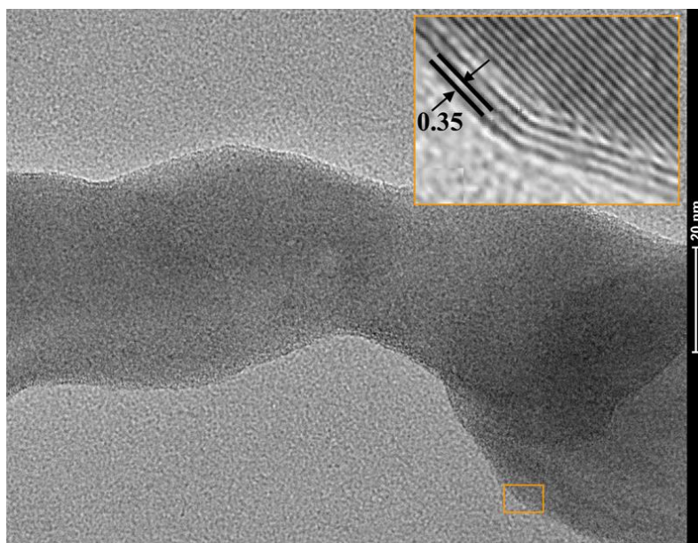
Figura 5 Immagine TEM di nanostrutture a base di carburo di silicio, sono evidenti i piani dei foglietti di grafene che ricoprono il materiale.
