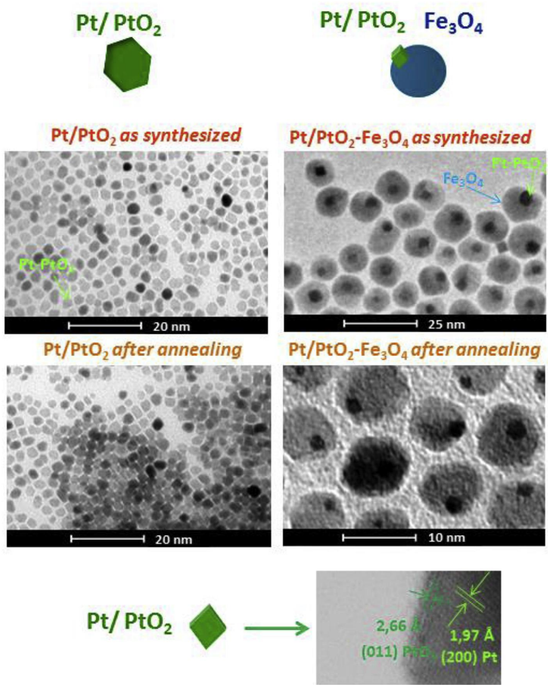
Figura 1 Immagini TEM di Pt/PtO 2 e Pt/PtO 2 -Fe 3 O 3 [87].
