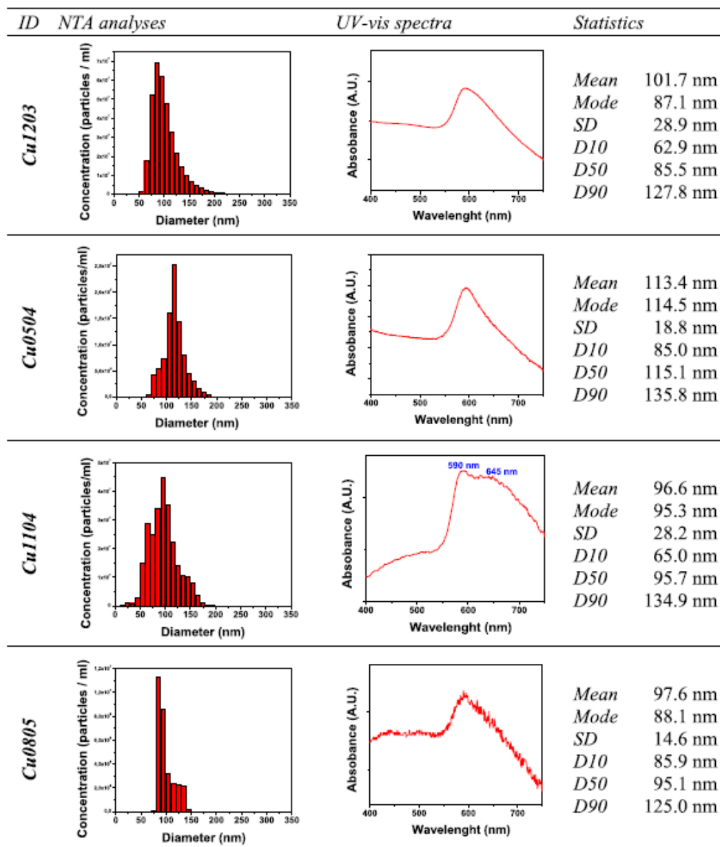
Figura 4 Analisi NTA di nanoparticelle di Cu realizzate in mezzi oleosi a diverse concentrazioni di precursori, agenti riducenti, olio e tensioattivi [89].
