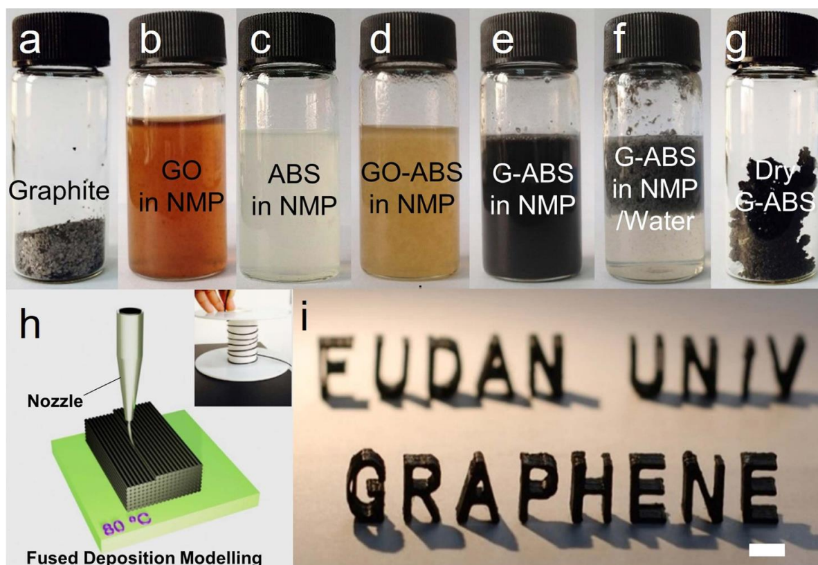
Figura 12 grafite (a); dispersioni di GO e ABS in solvente NMP (b,c); miscele omogenee di GO-ABS in NMP prima e dopo riduzione chimica, GO-ABS in sospensione durante riduzione chimica (d,e); Grafene-ABS ottenuto dopo separazione (f); polvere di Grafene-ABS dopo lavaggio ed asciugatura (g); illustrazione schematica del processo di stampa 3D tramite fused deposition modelling . L'inserto rappresenta l'avvolgimento di un filamento a base di grafene. Il filamento è stato depositato attraverso un ugello sopra un supporto riscaldato alla temperatura di 80 ° C (h); esempio di modello stampato in 3D tramite filamento composito G-ABS al 3,8% in peso, barra di scala: 1 cm (i) [80].
