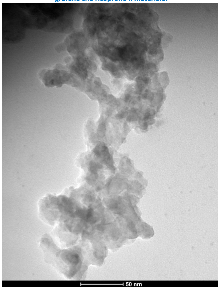
Figura 6 Immagine TEM di nanoparticelle di \text{TiO}_2 .
