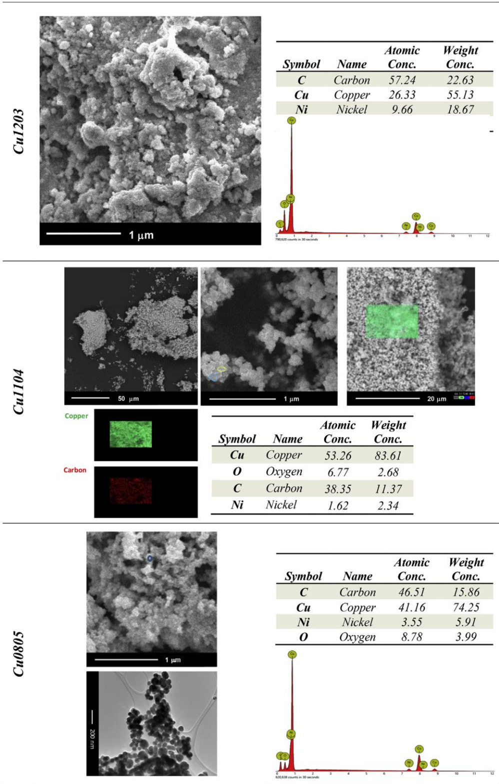
Figura 3 Immagini SEM e TEM di nanoparticelle di Cu realizzate in mezzi oleosi a diverse concentrazioni di precursori, agenti riducenti, olio e tensioattivi [89].
