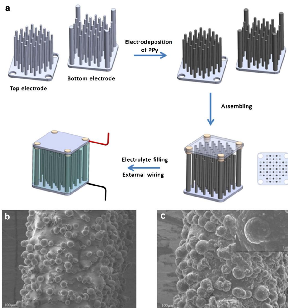
Figura 10 Procedura di realizzazione di elettrodi ed immagini SEM delle superfici prima e dopo il ricoprimento con polipirrolo [108].
