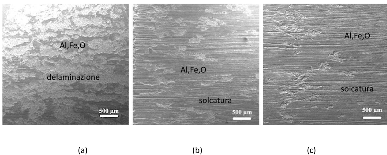
Figura 5: morfologia delle piste di usura (immagini SEM) sui pattini stazionari in lega A357 sottoposti a prove di strisciamento pattino su cilindro contro acciaio 100Cr6 (40 N, 0.3 \text{ m s}^{-1} ): (a) campione prodotto con tecnologie convenzionali, (b) campione SLM ottenuto in condizioni di massima produttività (SLM-1); (c) campione SLM con microstruttura ottimizzata (SLM-2).
